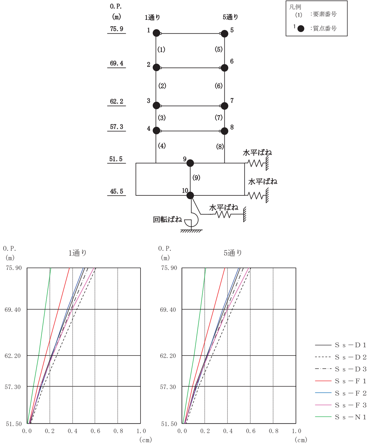
図 4-7 最大応答変位 (基準地震動 S s , EW 方向)
