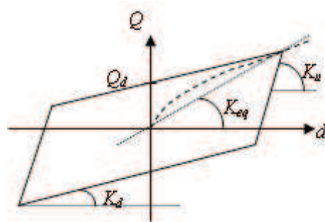
図 6.3.7-5 修正バイリニア型履歴
