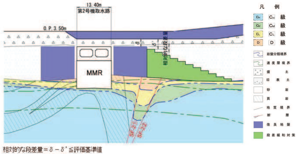
図 8.6-13 相対的な段差量の算出方法
