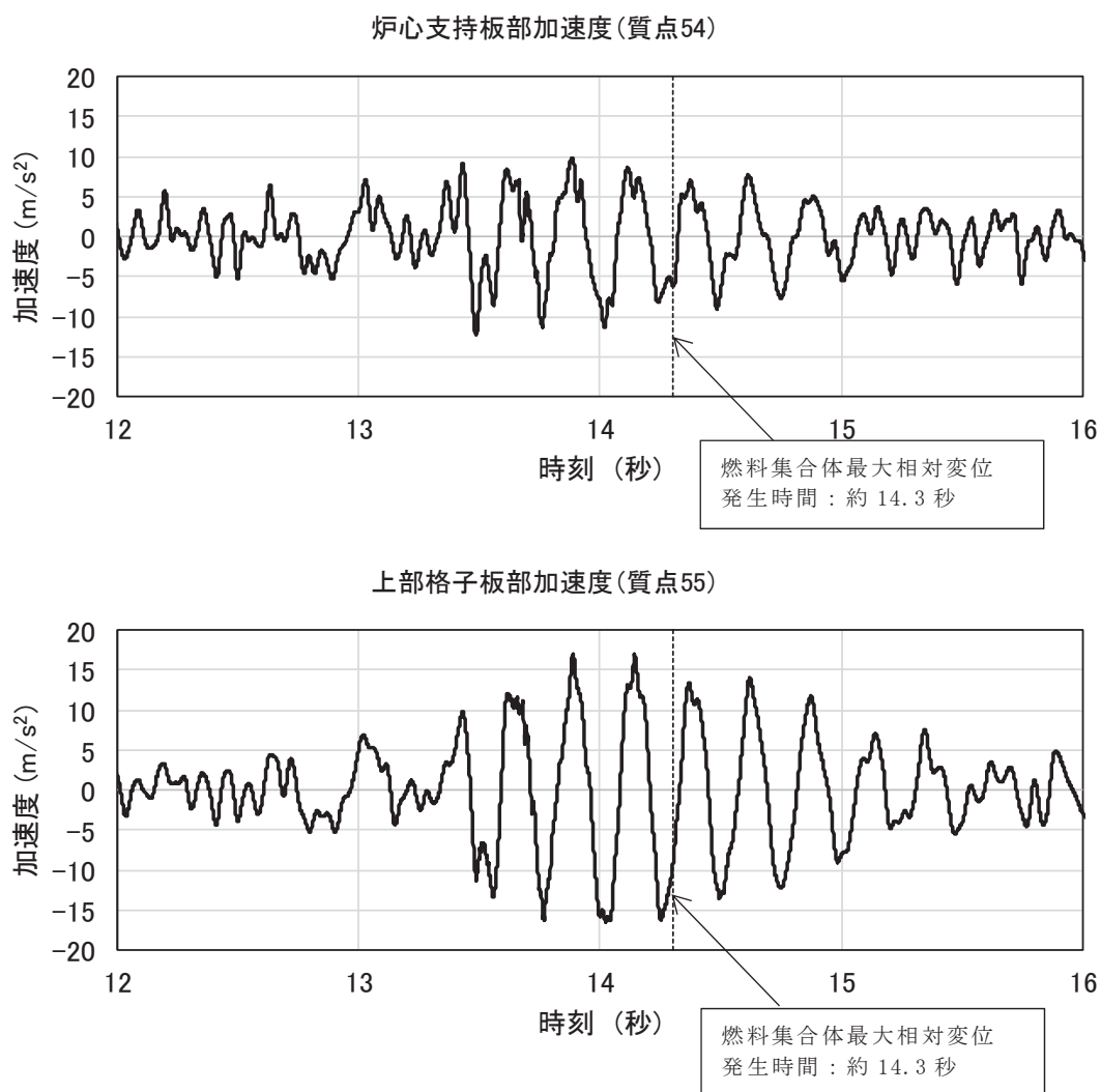
別紙 3 図 12 CR-IN に入力する加速度時刻歴データの比較
