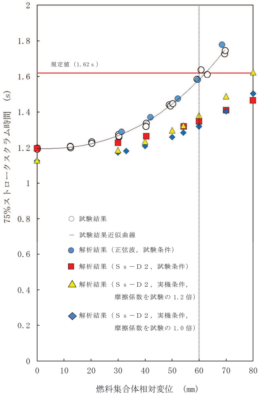
図 5-12 試験条件による制御棒挿入性解析結果
