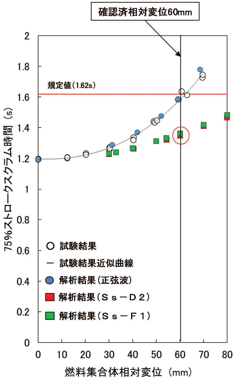
別紙 3 図 6 挿入性曲線の比較
