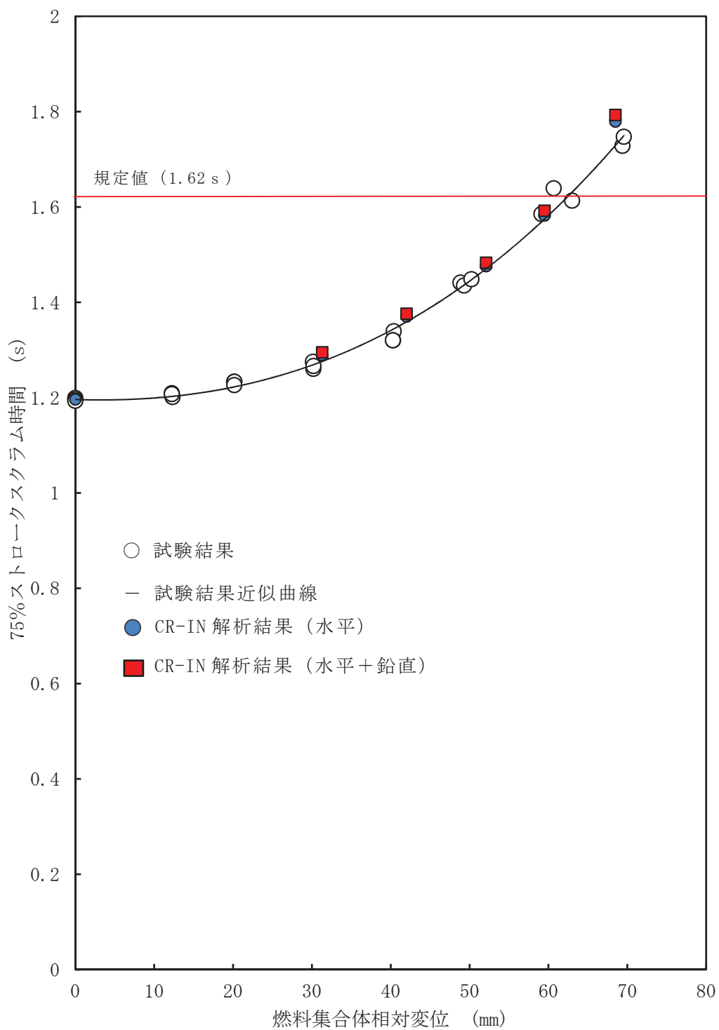
図 5-14 制御棒に対する鉛直方向加速度の影響確認結果
