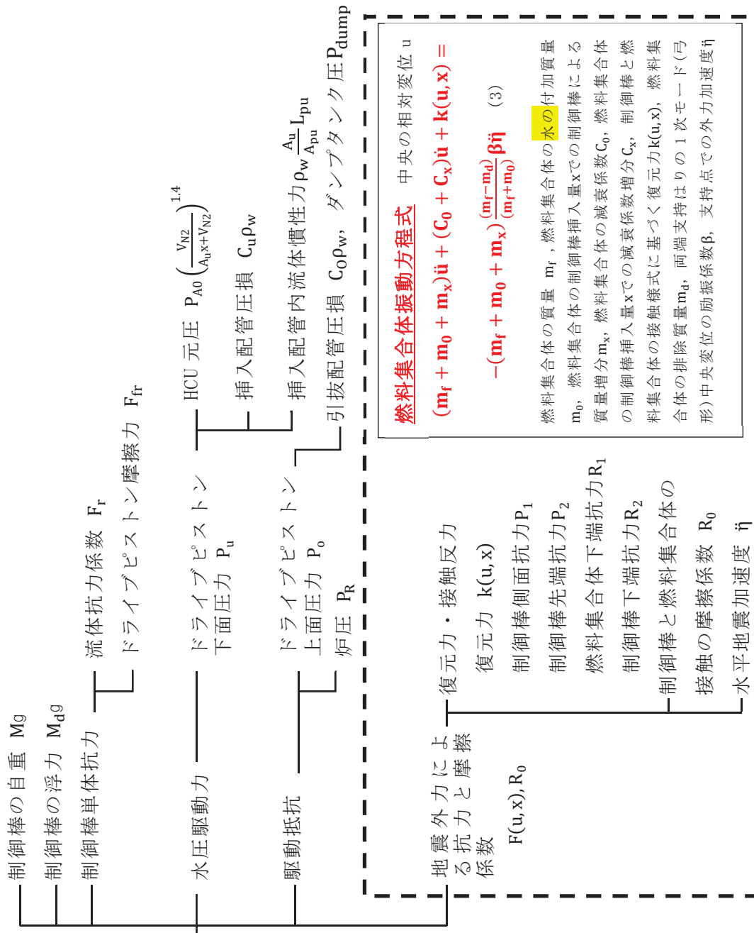
別紙 1 図 1 CR-IN に関係するパラメータ一覧 (点線内が地震外力に関係する項)
