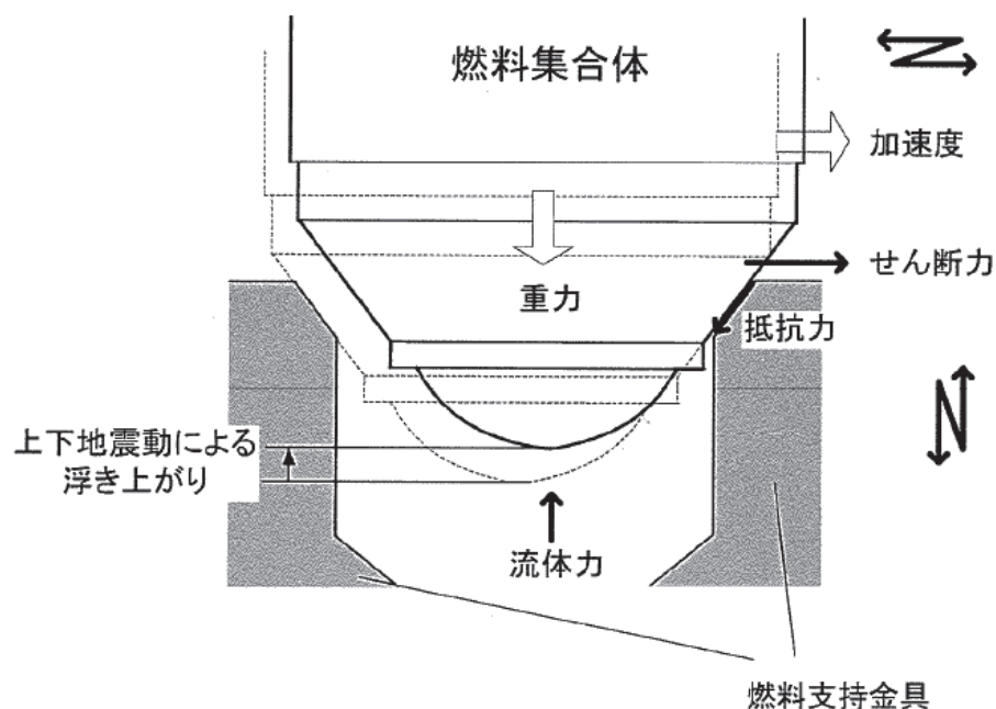
図 5-18 水平・鉛直方向加速度による浮上り検討概要図 (既往知見 (2) )
