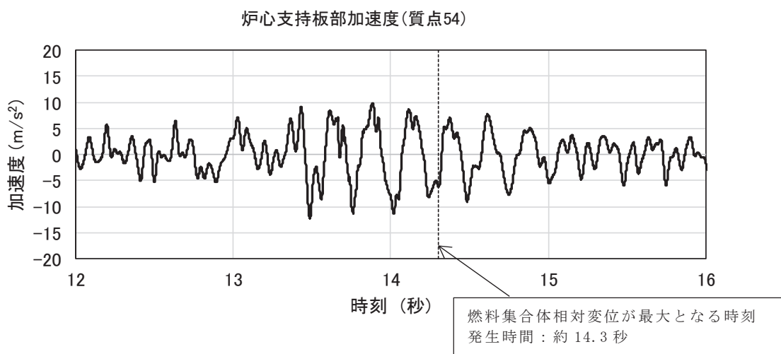
別紙 3 図 10 炉心支持板の加速度時刻歴 (S s - D 2)
