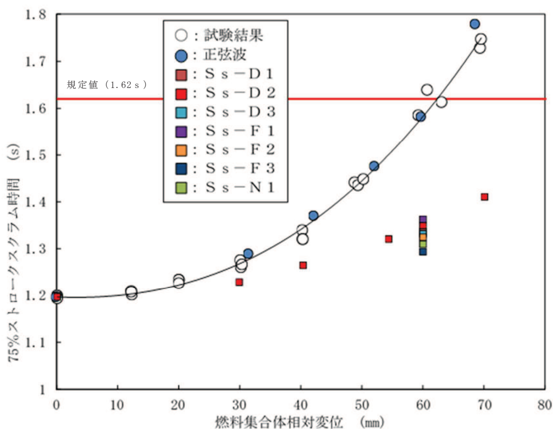
別添 3 図 3 S s - D 2 以外の基準地震動に対する制御棒挿入性解析結果
