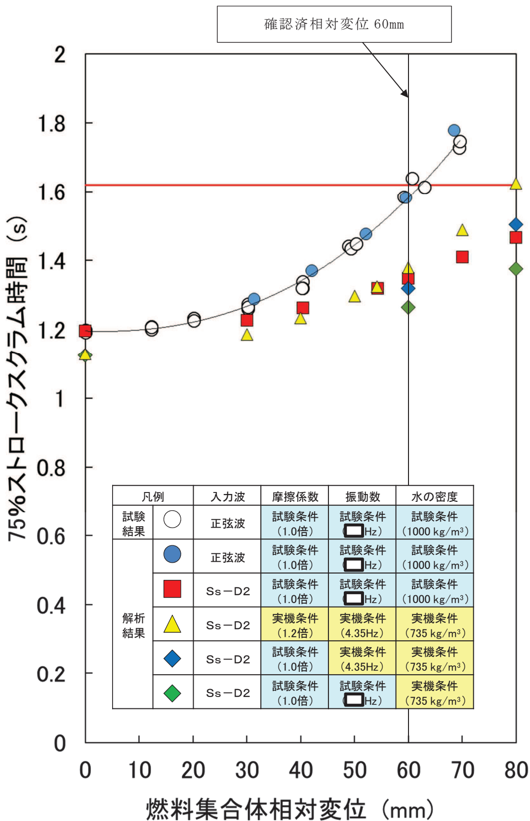
別添 4 図 1 実機及び試験条件における制御棒解析結果の比較
