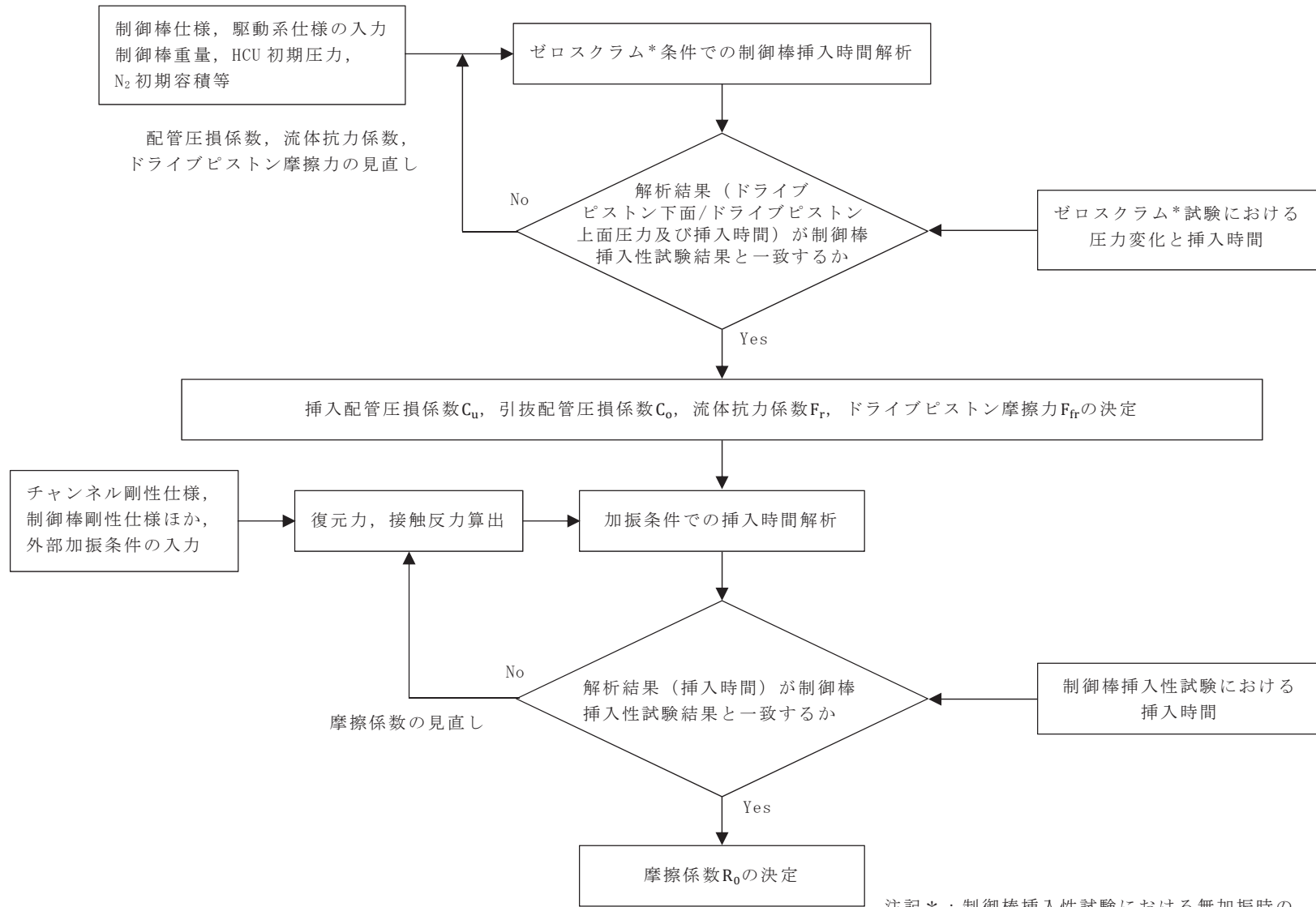
別添 1 図 1 CR-IN の各パラメータの設定フロー
