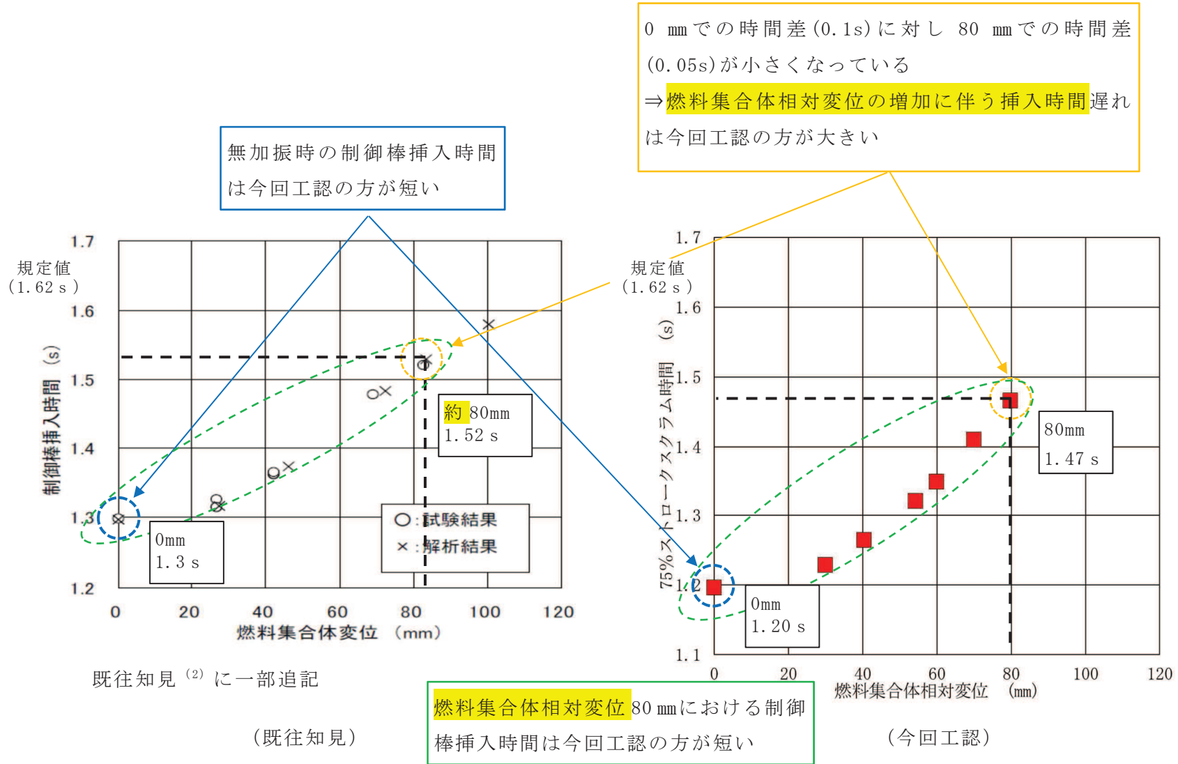
図 5-12 既往知見における制御棒挿入性解析結果との比較
