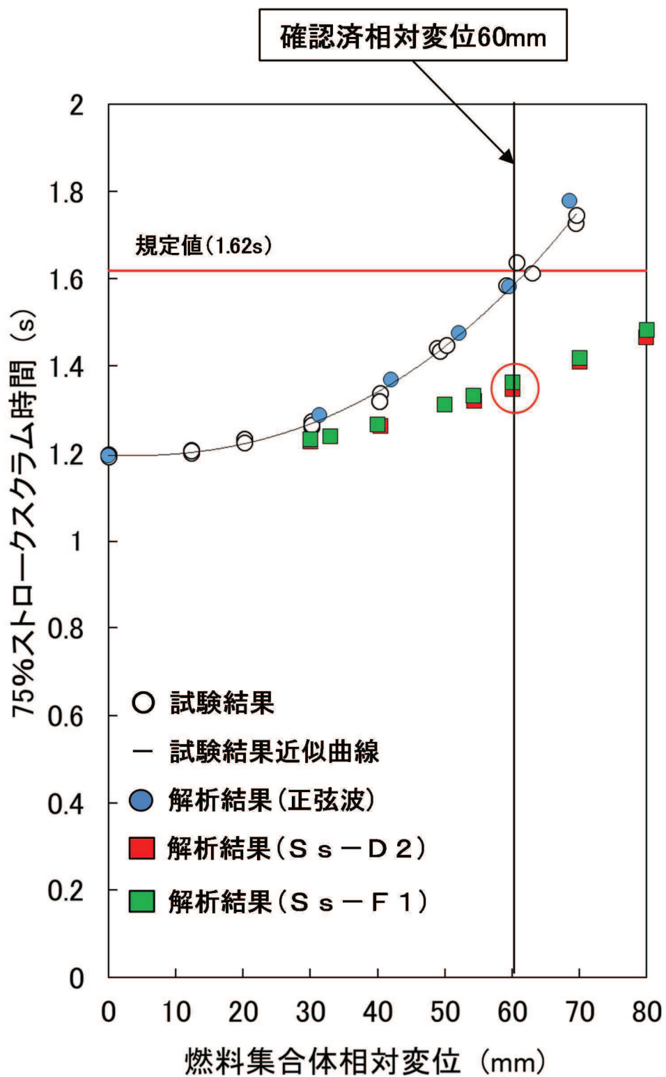
別添 3 図 5 挿入性曲線の比較
