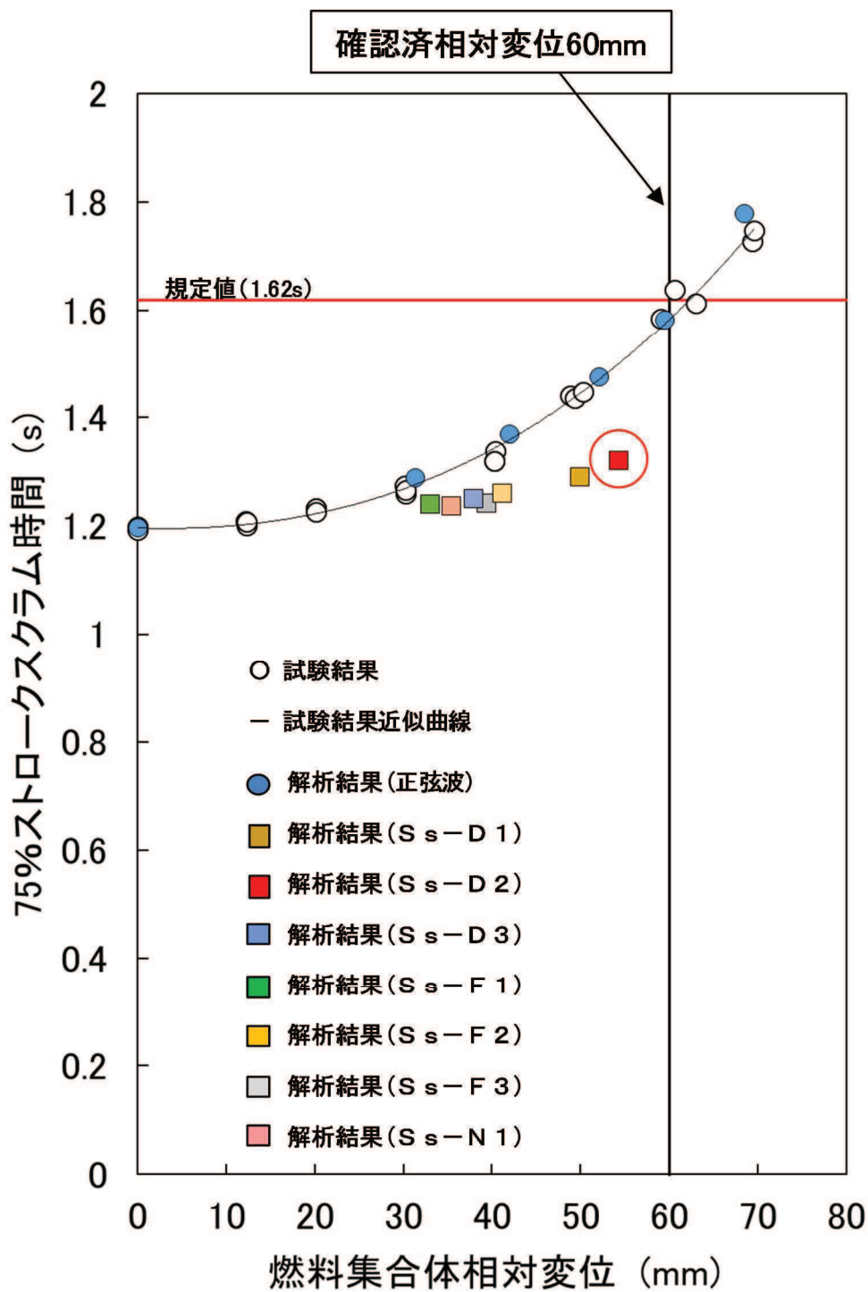
別添 3 図 1 各基準地震動に対する燃料集合体相対変位を用いた 制御棒挿入性解析結果
