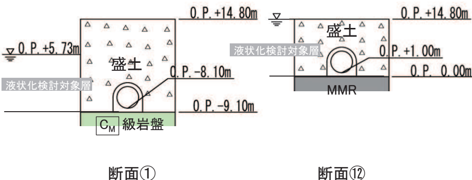
浮上り評価地質図
