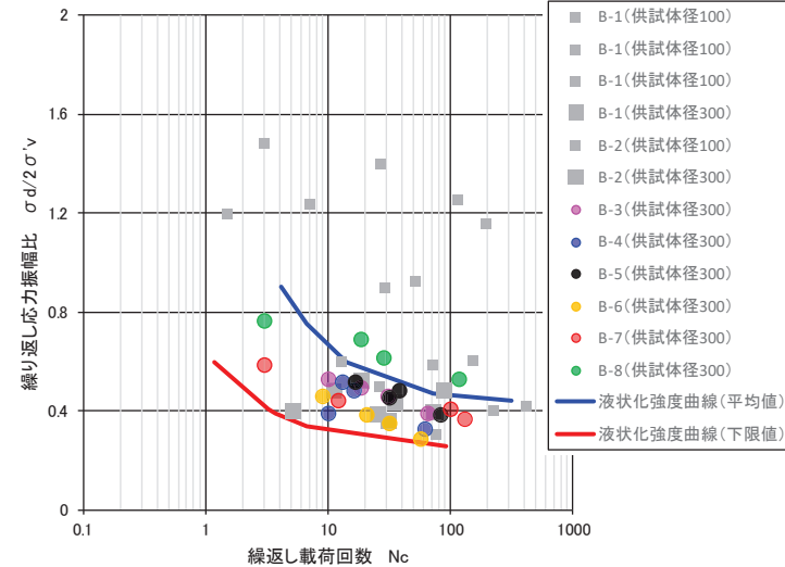
液状化強度特性(盛土)
