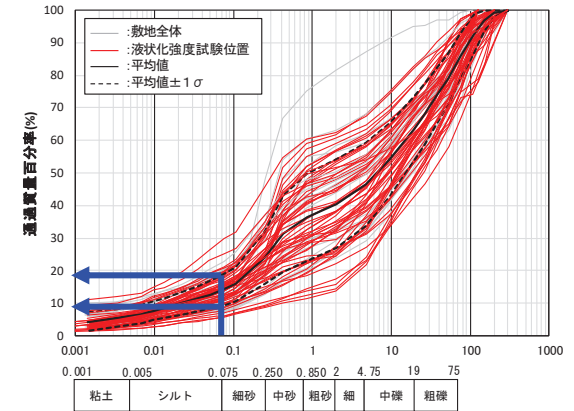
図2 粒径加積曲線*1
