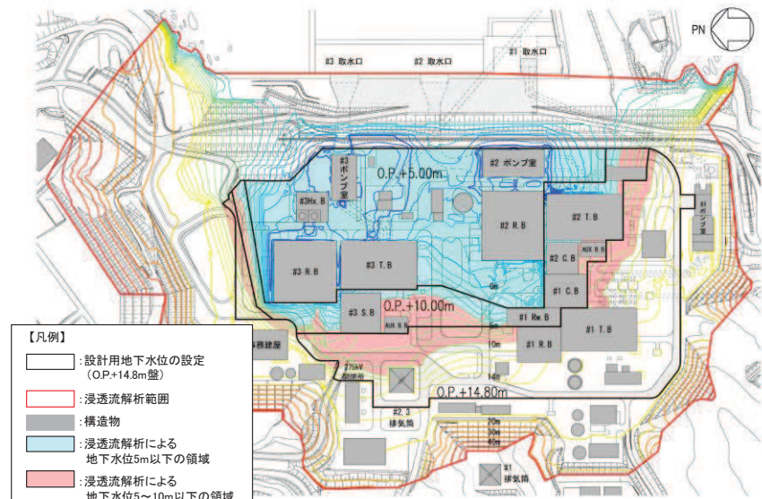
O.P.+14.8m盤の設計用地下水位
