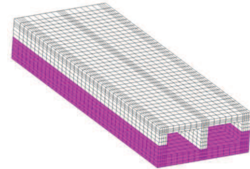
貯水機能を損なわないことの確認における評価対象範囲(着色部)
