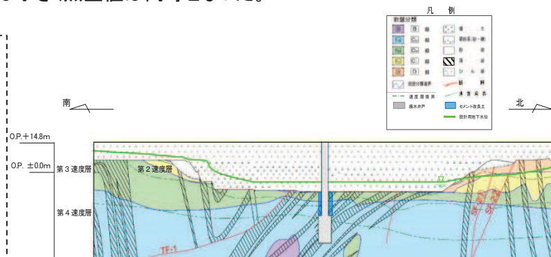
No.2揚水井戸地質断面図
