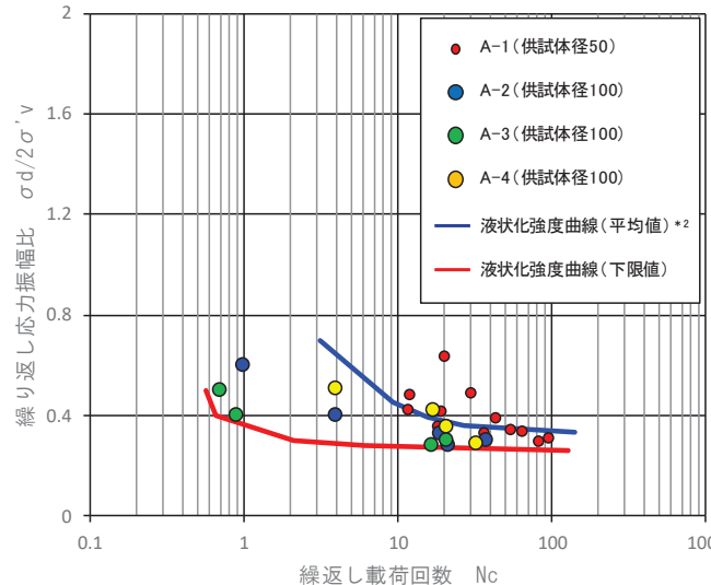
液状化強度特性(旧表土)
