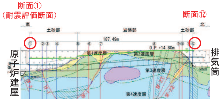
排気筒連絡ダクト地質縦断図
