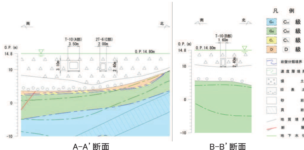
A-A' 断面
