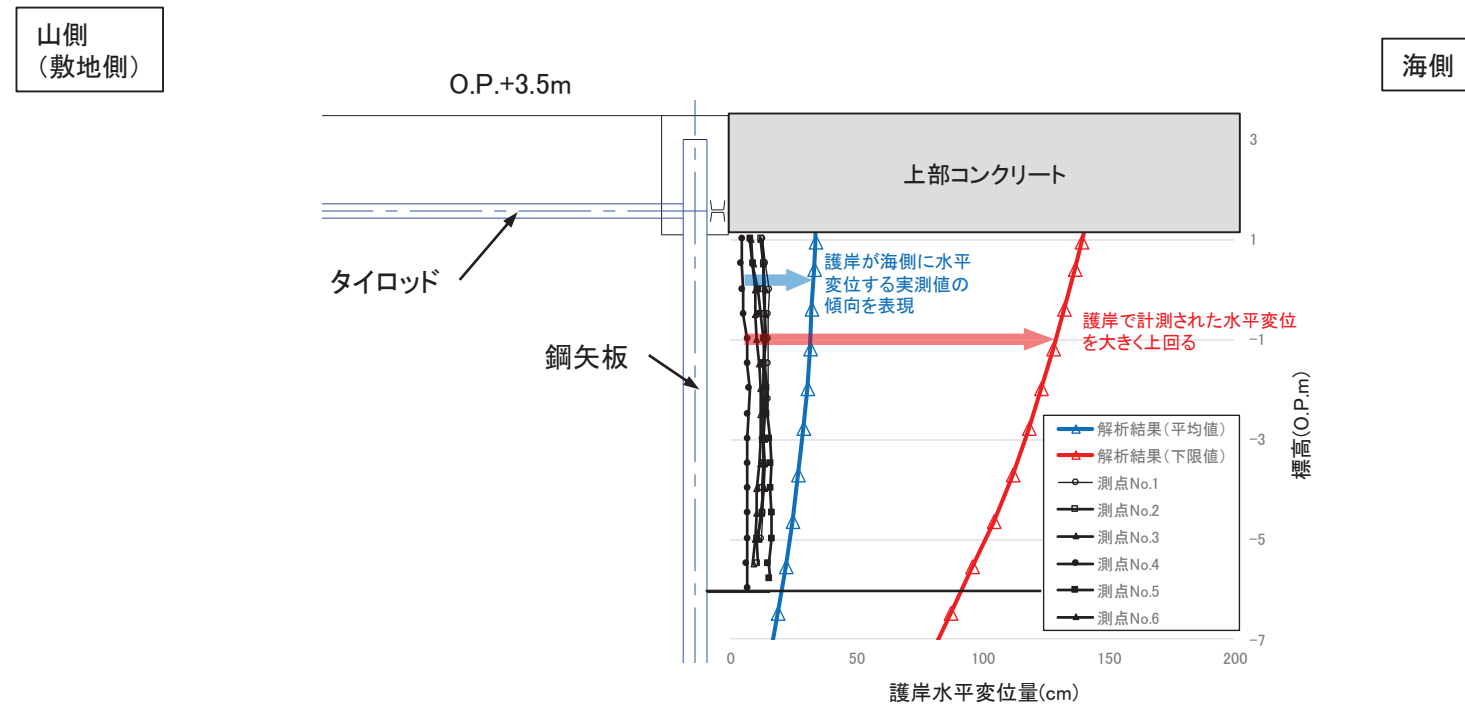
3.11地震の検証解析結果と矢板護岸の水平変位実測値の比較
