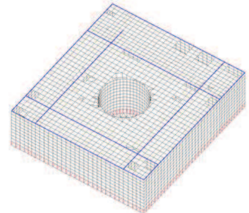
原子炉建屋基礎版 解析モデル
