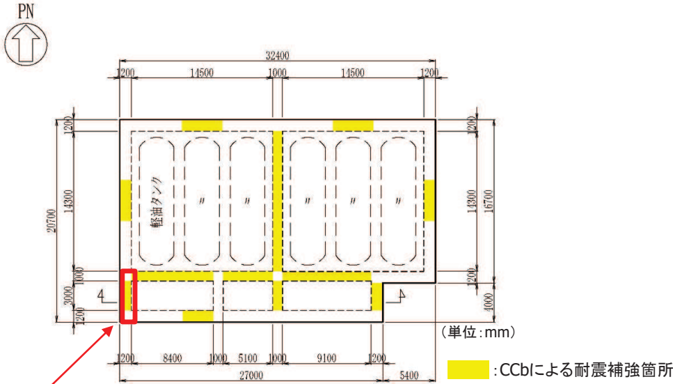
軽油タンク室平面図とCCb補強箇所
