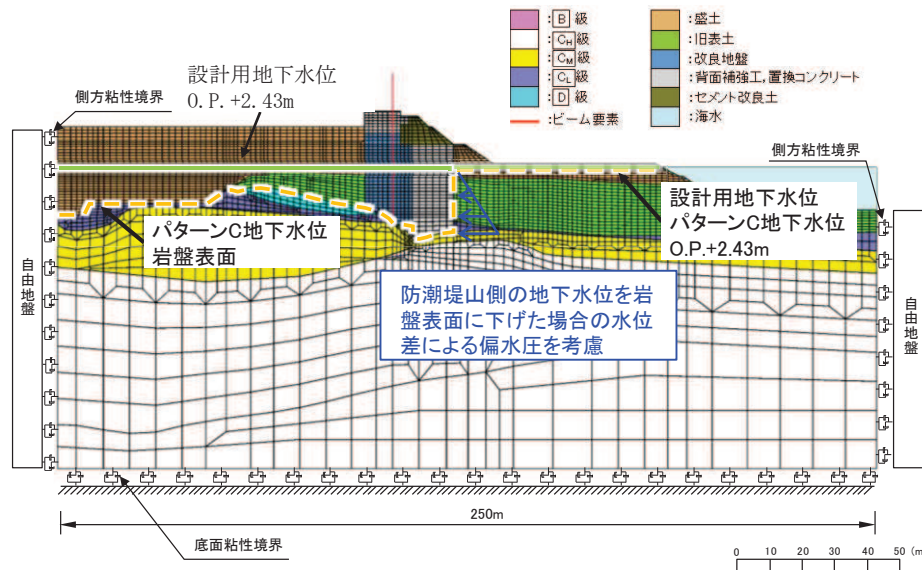
解析モデルと地下水位
