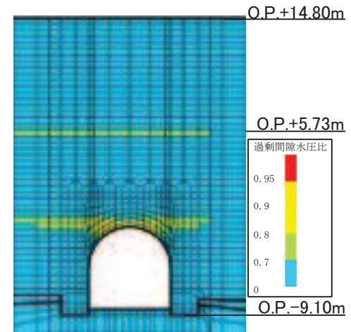
断面① 最大過剰間隙水圧比分布図
