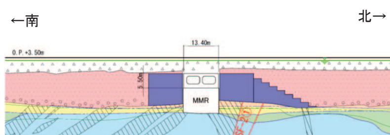
地質断面図(断面②)
