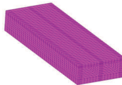
構造強度及び通水機能を有することの確認における評価対象範囲(全部材)
