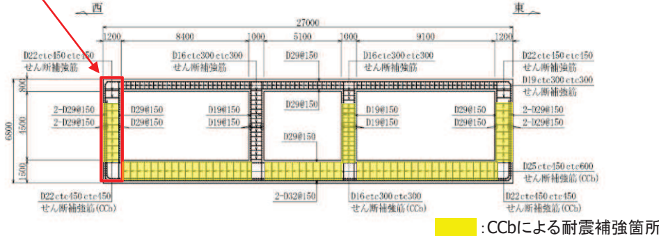
軽油タンク室縦断図とCCb補強箇所 (単位: mm)
