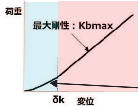
滑り変位とばね力の関係
