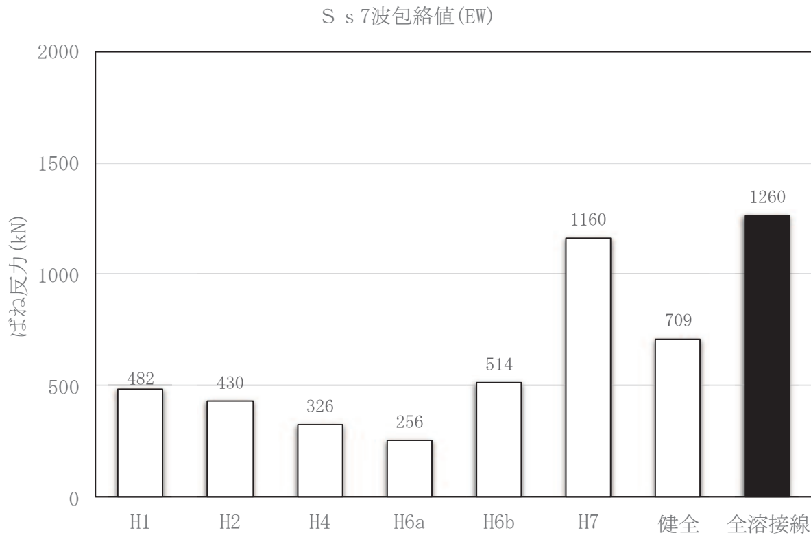
図 2-12 下部スタビライザ反力最大値の比較
