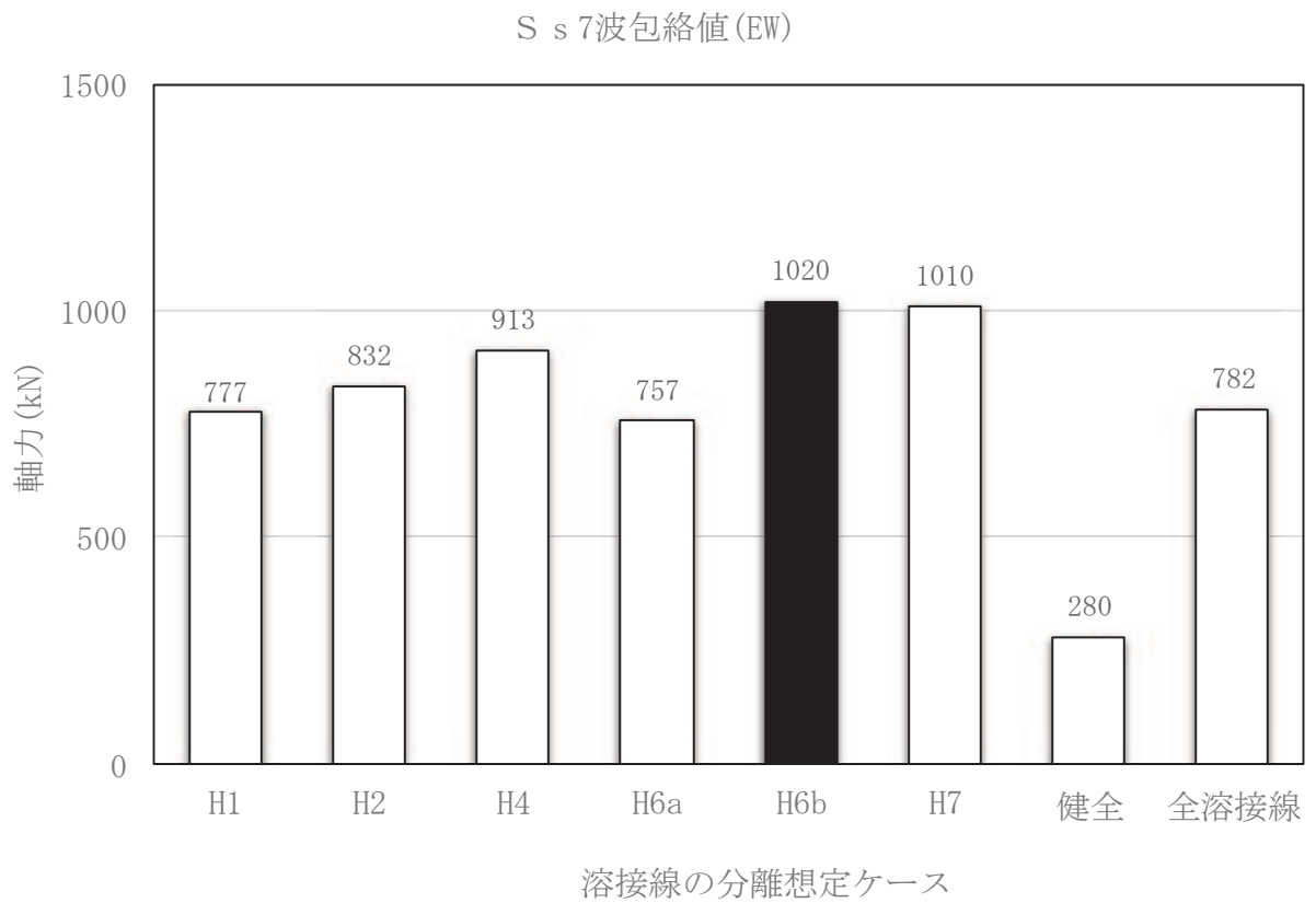
図 2-8 炉心シュラウド支持ロッド軸力最大値の比較
