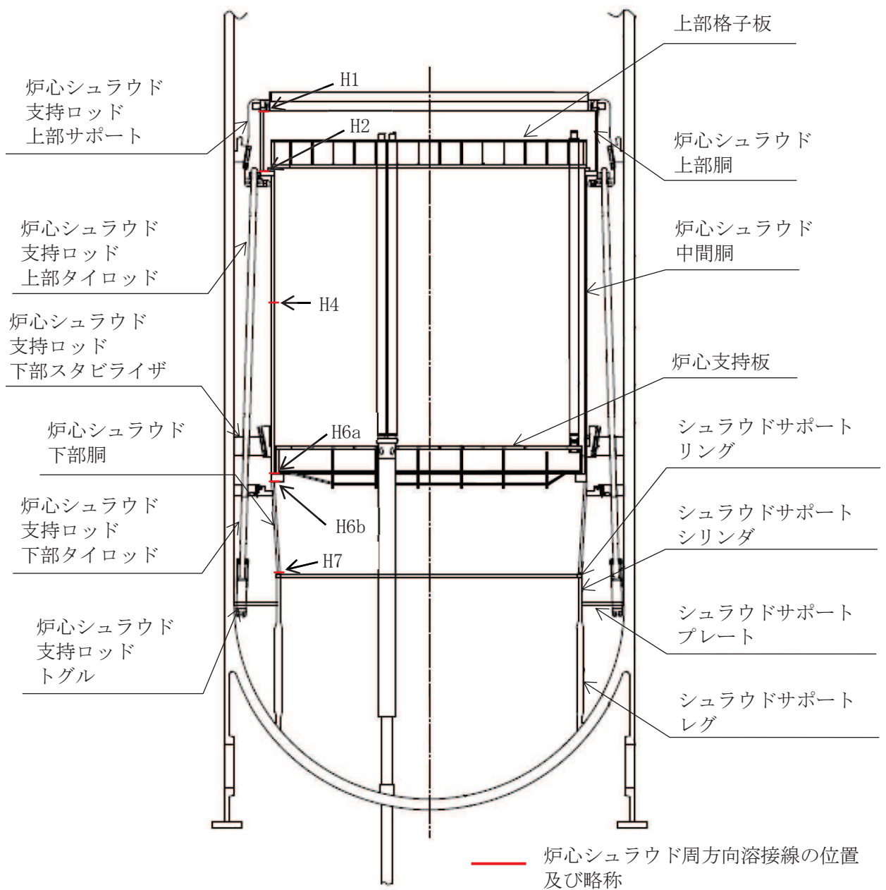
図 2-5 炉心シュラウド，炉心シュラウド支持ロッド及びシュラウドサポートの概略形状並びに炉心シュラウド周方向溶接線の位置
