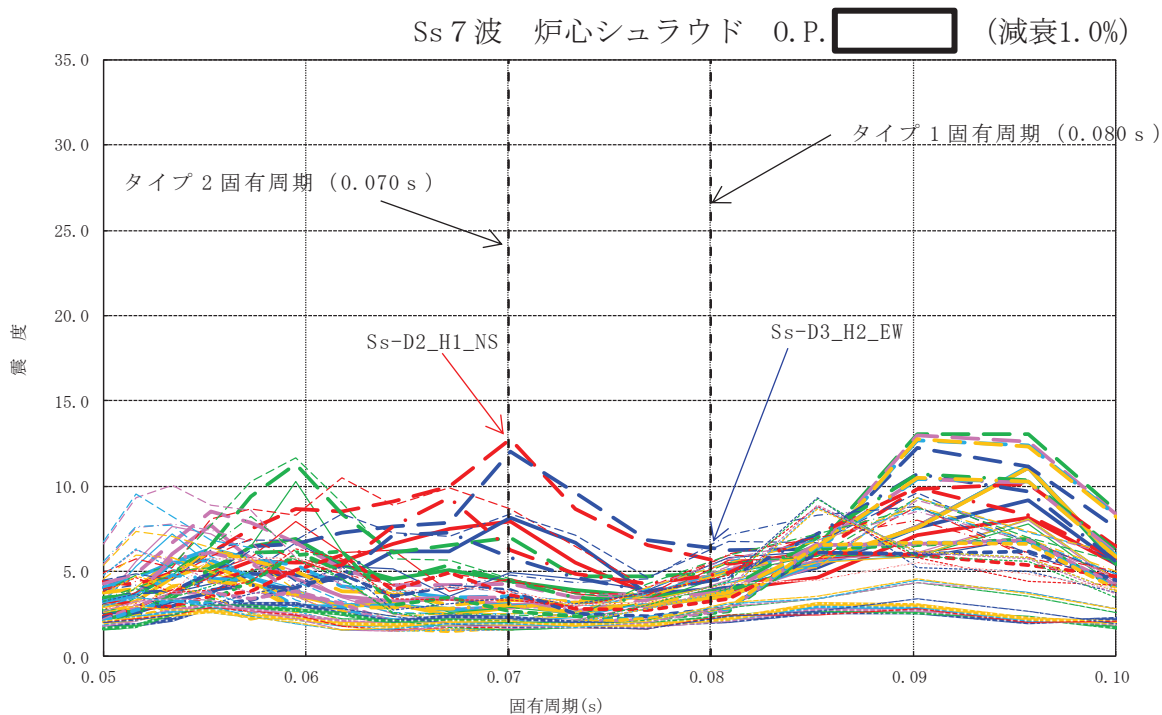
図 2-9 炉心シュラウド支持ロッド固有周期における床応答曲線最大値
