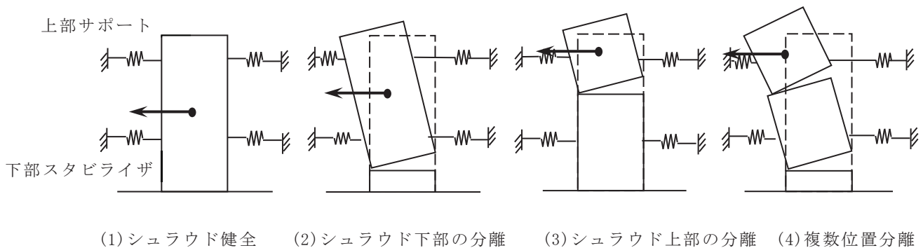
図 2-10 炉心シュラウドの分離想定概念図
