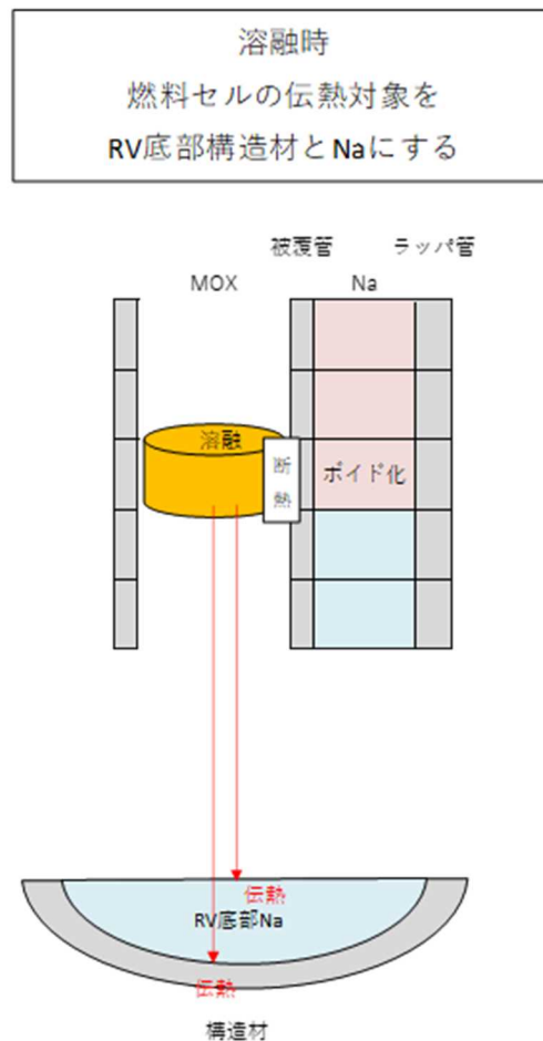
図1 溶融落下した燃料セルの伝熱モデル
