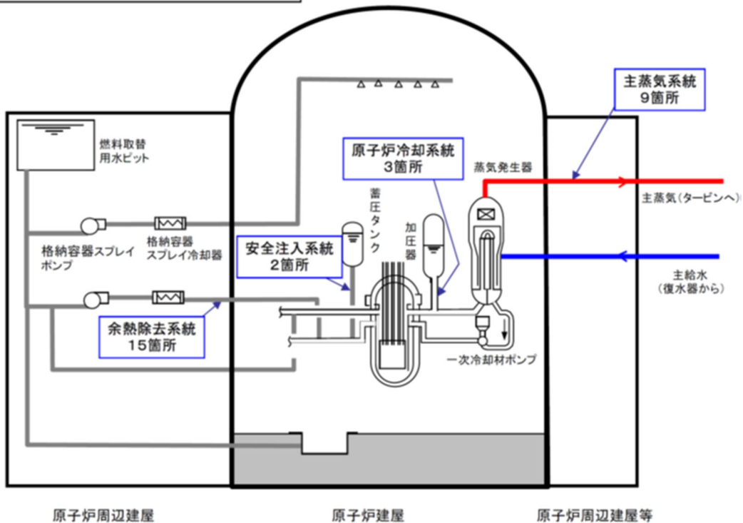
支持構造物を補強した系統の概要図
