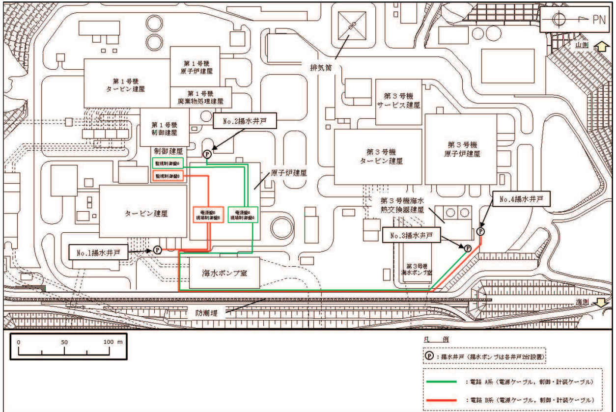
図6-1 電路の配置
