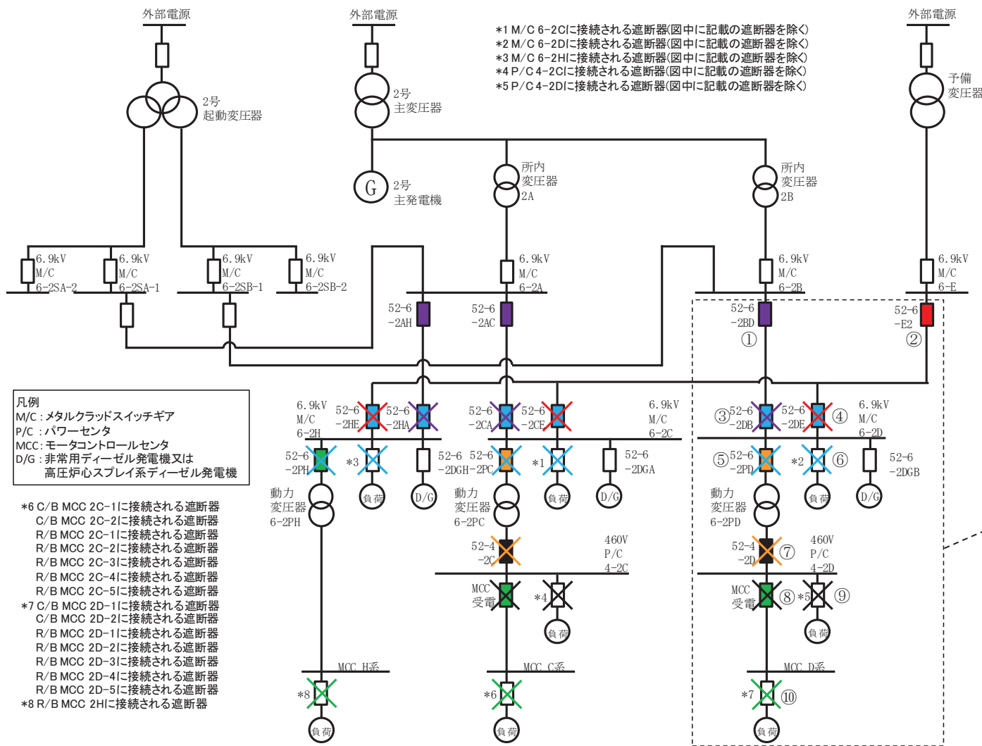
図 3.3 HEAF 対策が必要な電気盤系統図 (1/2)
