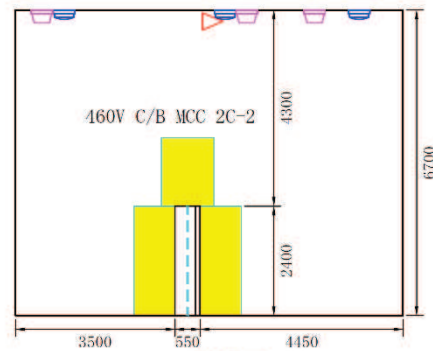
B-B' 断面
