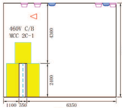
A-A' 断面
