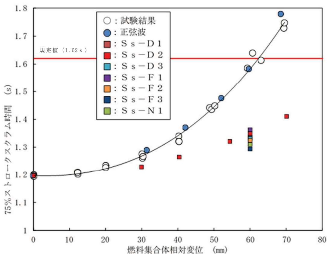
別添 3 図 2 S s - D 2 以外の基準地震動に対する制御棒挿入性解析結果
