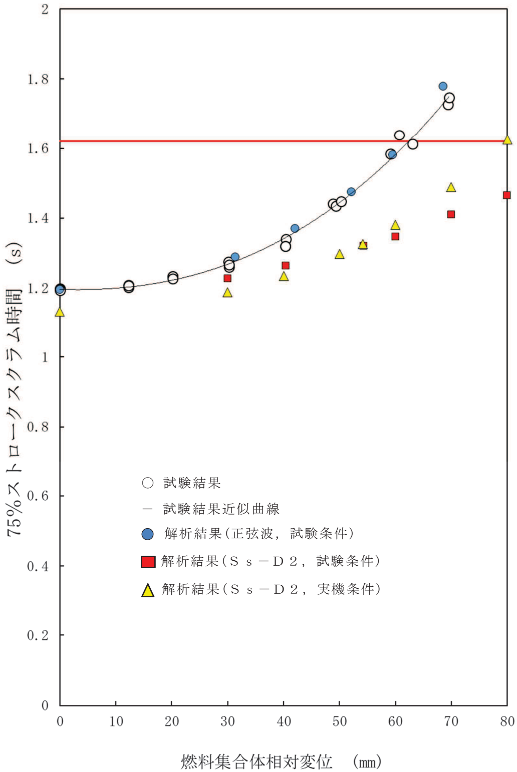
別添 4 図 1 実機及び試験条件における制御棒解析結果の比較
