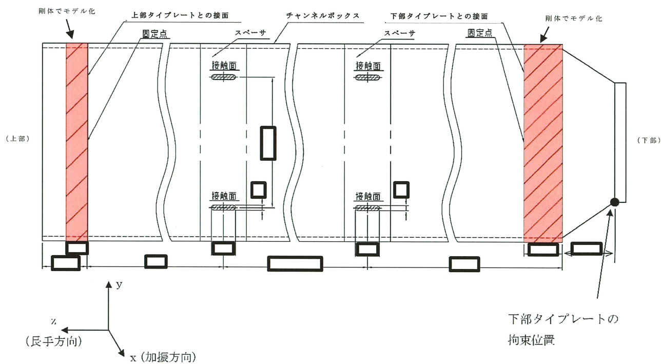
別添 7 図 3 燃料集合体の構造概略図
