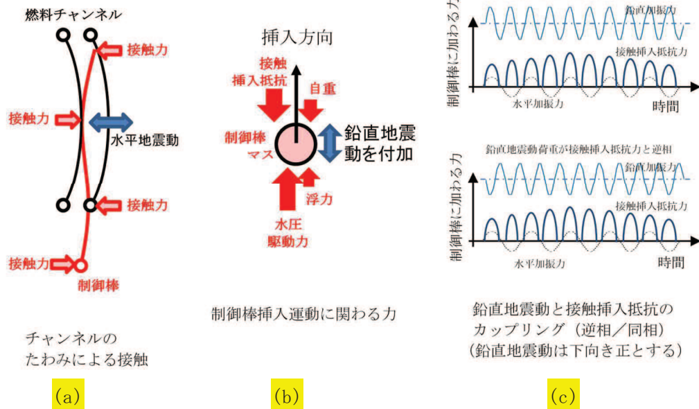
別紙 1 図 7 CR-IN による鉛直方向加速度の挿入時間への影響解析モデル
