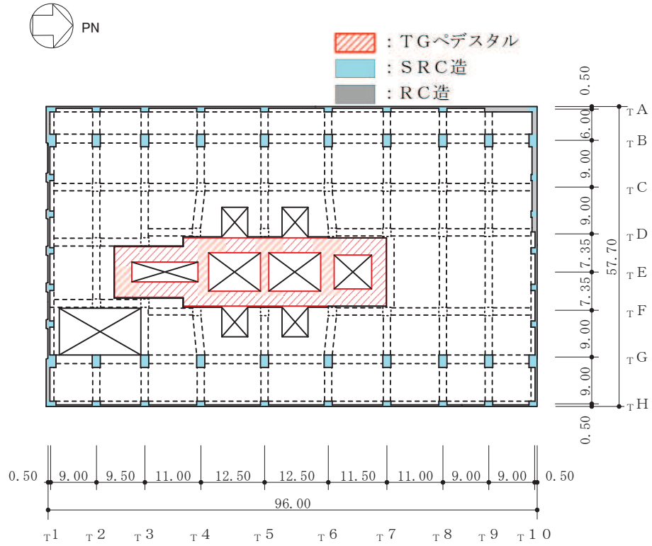
図 2-2(4) タービン建屋の概略平面図 (0.P. 24.8m)
