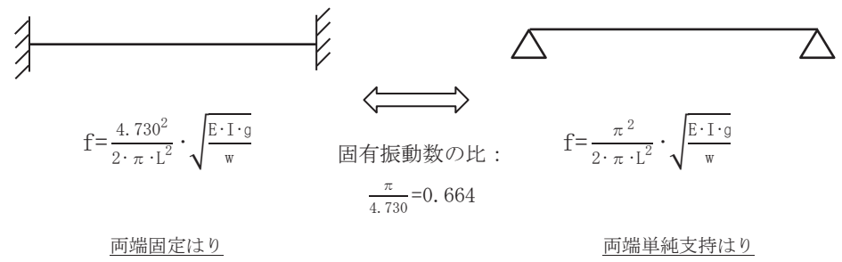
図2 境界条件の違いによる固有振動数の差異
