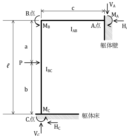
図2 支持架構モデル概略図
