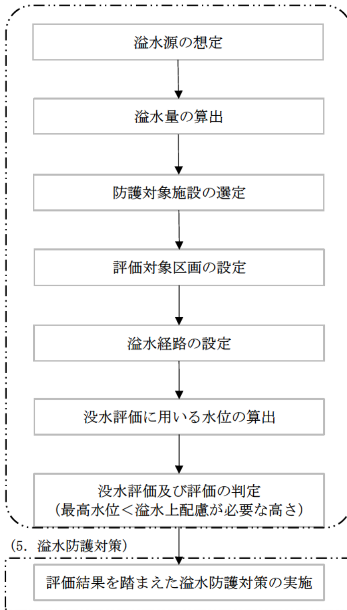
図-1 溢水防護対策の全体方針
