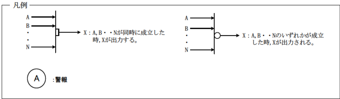
図-1-2-25 均質・ブレンド設備 インターロック (2号均質パージ系コールドトラップ) (圧力異常高又は温度異常高による加熱停止のインターロック)
