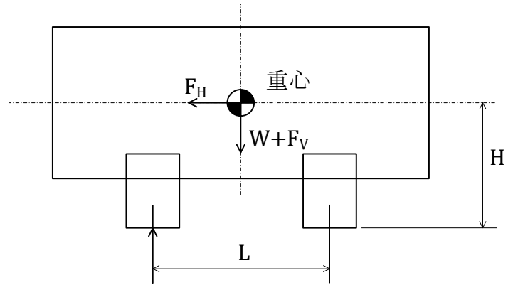
図6 脚部応力評価（設計基準を超える条件に対する設計）の計算モデル
