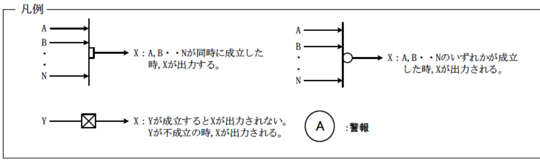
図-1-2-8(2/2) 均質・ブレンディング設備 インターロック (2号均質槽F) (地震発生時のUF 6 漏えい防止インターロック (緊急遮断弁閉, 加熱停止))
