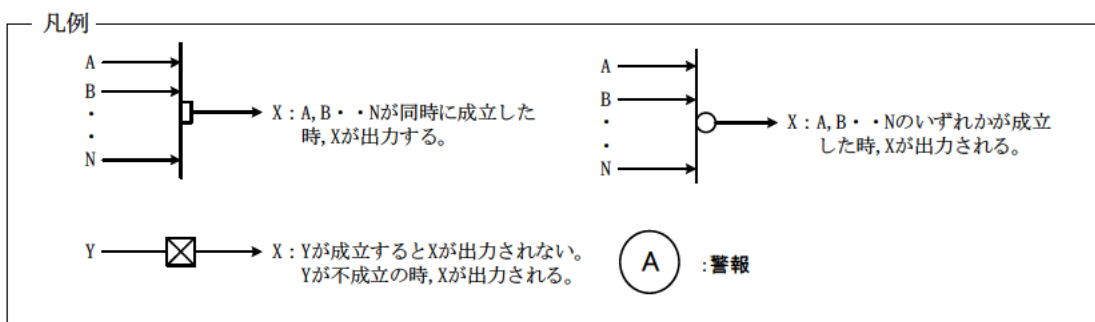
図-1-2-3(2/2) 均質・ブレンディング設備 インターロック (2号均質槽 F) (減圧槽故障による均質槽加熱停止インターロック)
