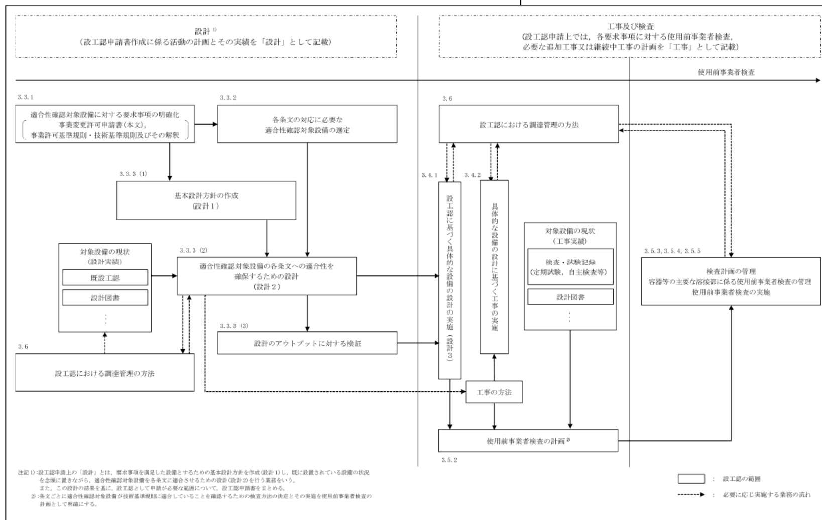
第3.2-1図 設工認として必要な設計、工事及び検査の流れ
