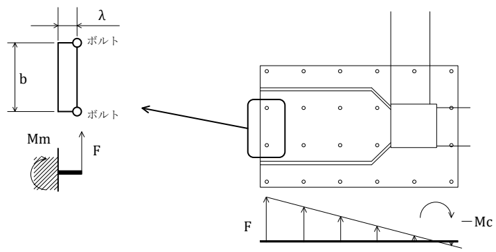
図3 後打ちプレートモデル概略図
