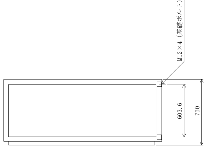
側面図
