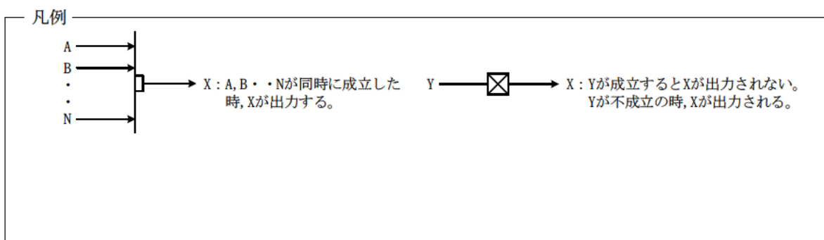
図-1-2-7(1/3) 均質・ブレンディング設備 インターロック (2号均質槽) (UF 6 シリンダ類交換時の誤操作防止のインターロック)
