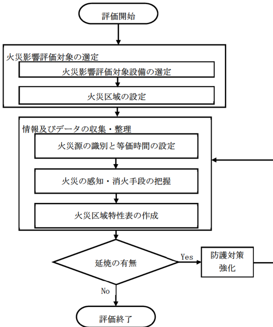
火災影響評価フロー
