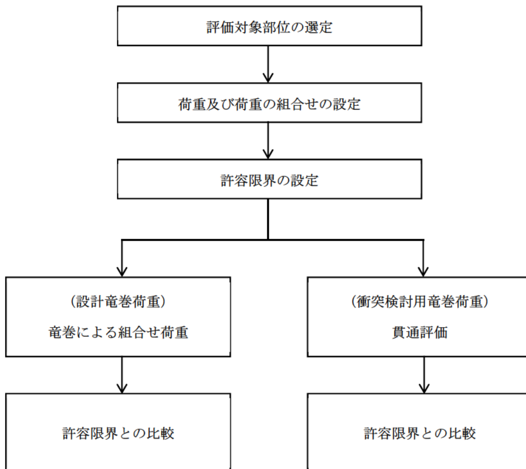
図1 設計荷重に対する強度評価のフロー図
