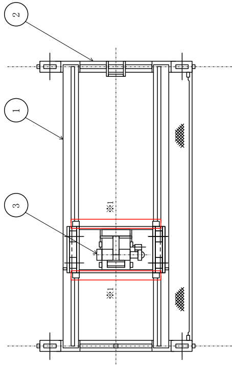
平面図
