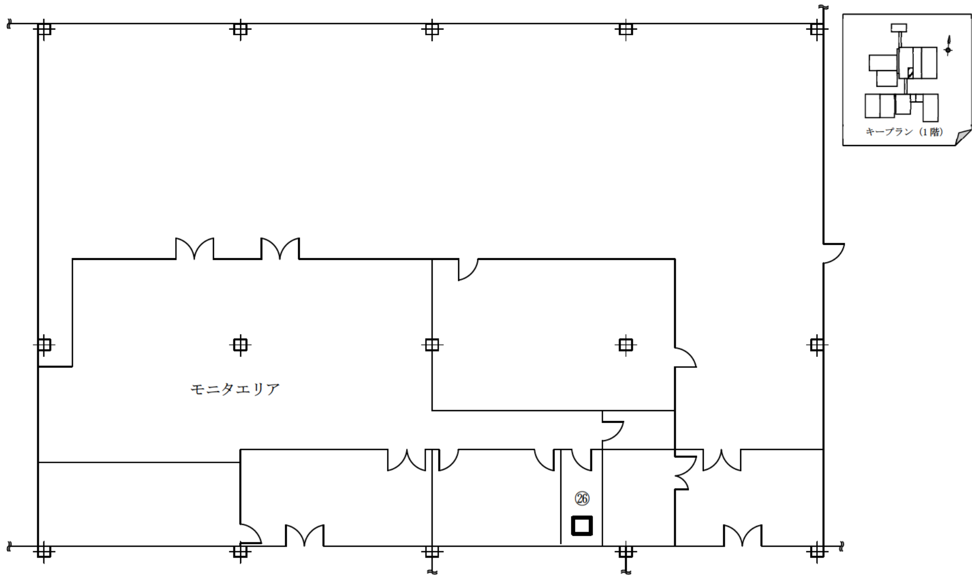
図 2.4.1 液体廃棄物の廃棄設備 機器配置概略図 (4 / 7)
