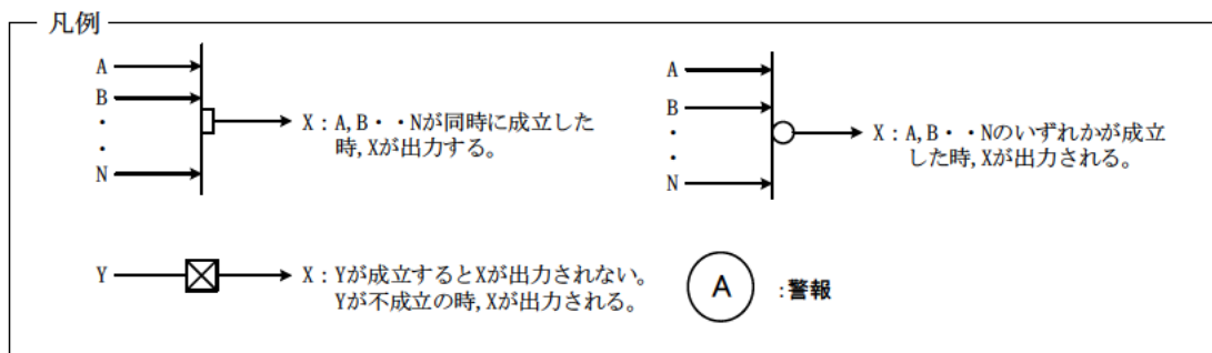
図-1-2-26 均質・ブレンディング設備 インターロック (2号均質ページ系コールドトラップ) (地震発生時の加熱停止のインターロック)
