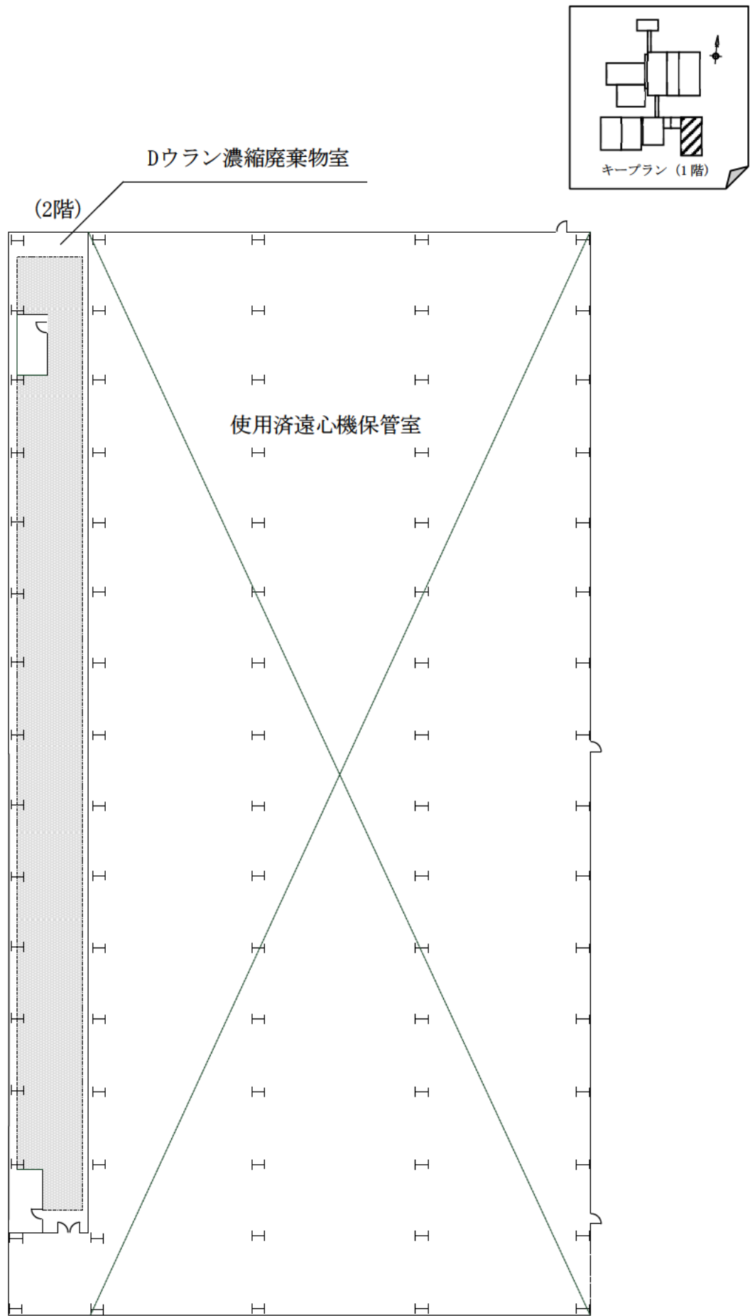
図 2.5.4 固体廃棄物の廃棄設備 機器配置概略図 (固体廃棄物保管廃棄区画)
