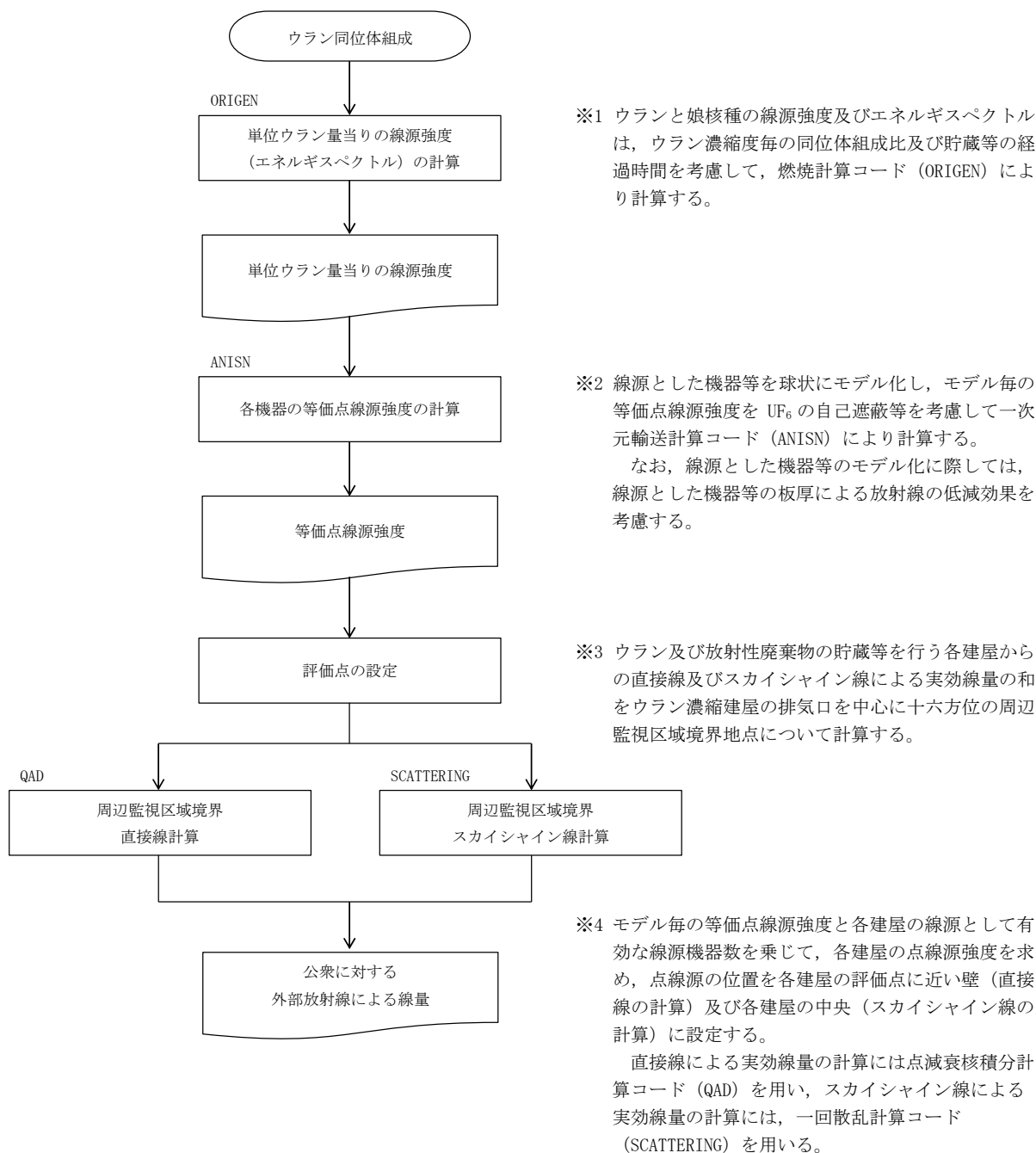
図ー1 直接線・スカイシャイン線の線量評価手順
