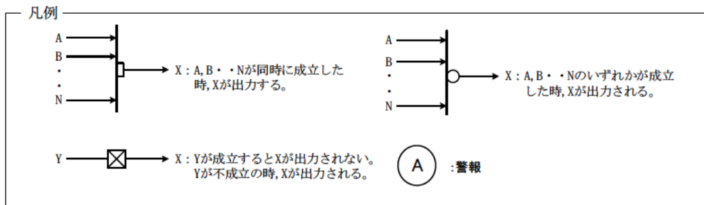
図-1-2-22 均質・ブレンディング設備 インターロック (2号サンプル小分け装置) (地震発生時の加熱停止のインターロック)
