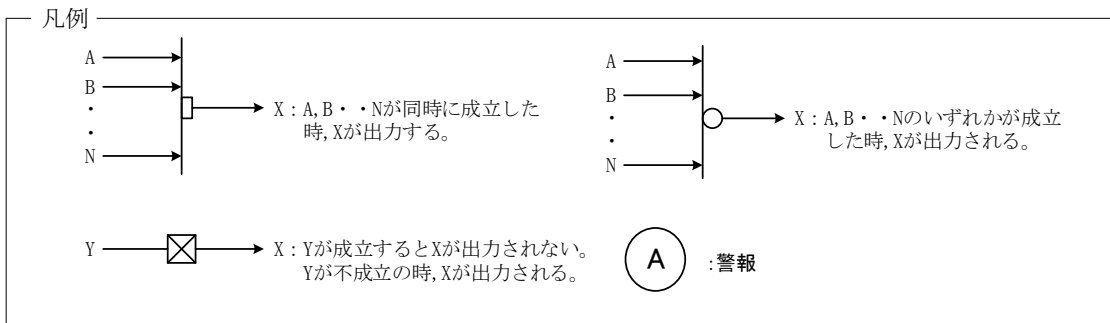
図-1-2-2(2/2) 均質・ブレンド設備 インターロック (2号均質槽F) (工程用モニタ HF 濃度高による UF 6 漏えい拡大防止のインターロック)
