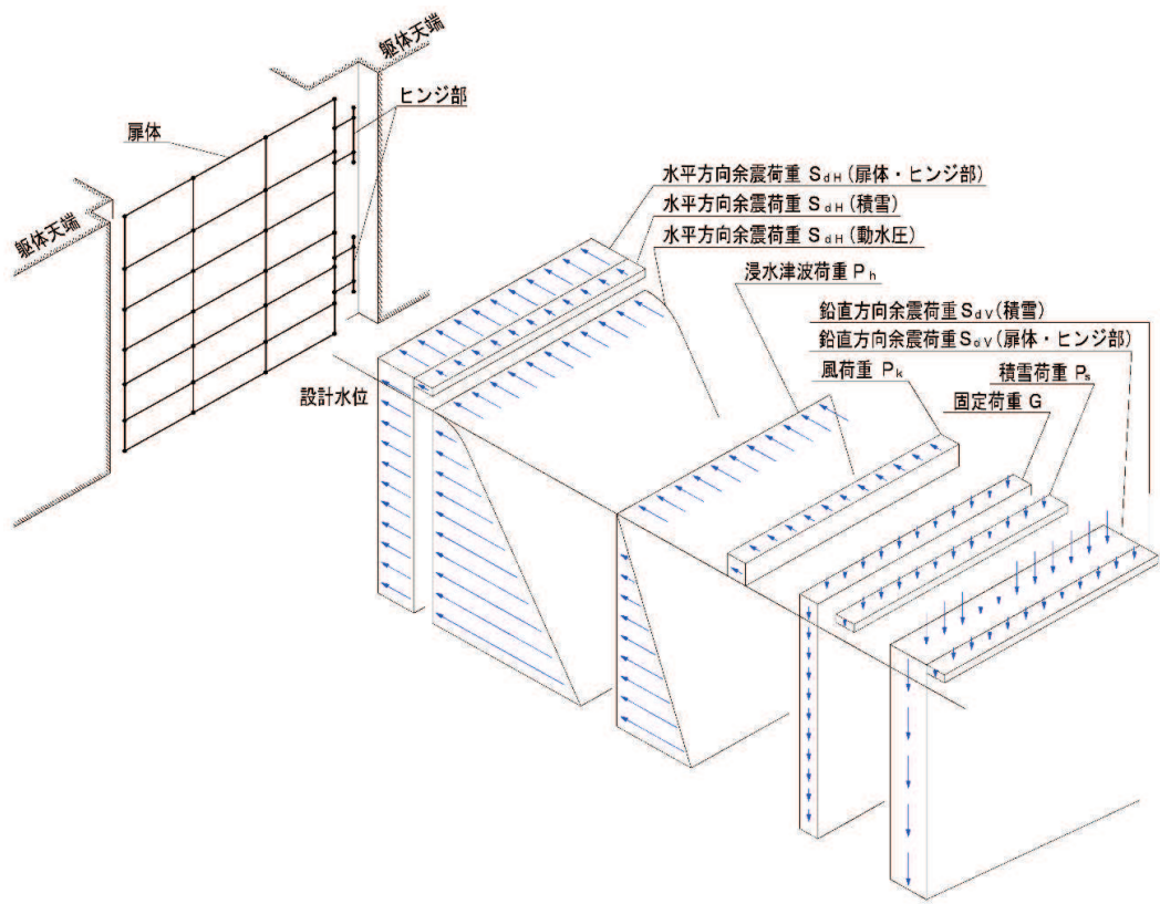
図 3.5-21 静的解析概念図 (荷重作用図)
