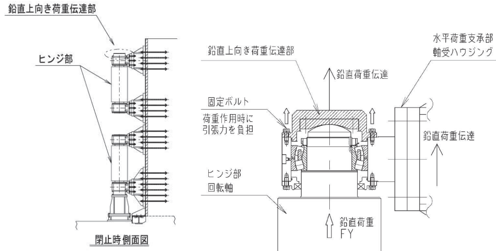
図 3.5-43 鉛直上向き荷重伝達部の概要図
