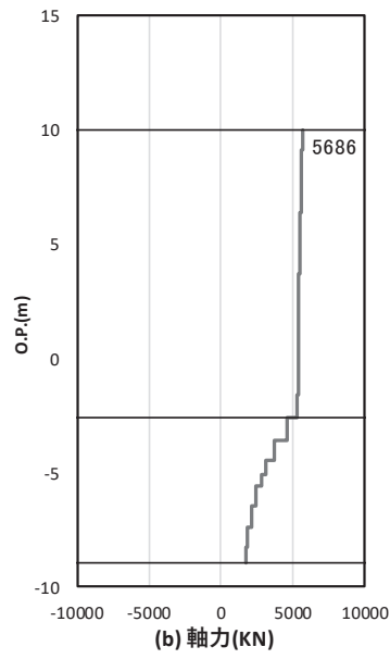
図 4.1-41 基礎地盤の支持性能照査時刻での軸力（押し込み） （鋼桁 2，基礎 1，S d-D 2（--），t = 25.44s） 解析ケース②：地盤物性のばらつき（+1σ）を考慮した解析ケース
