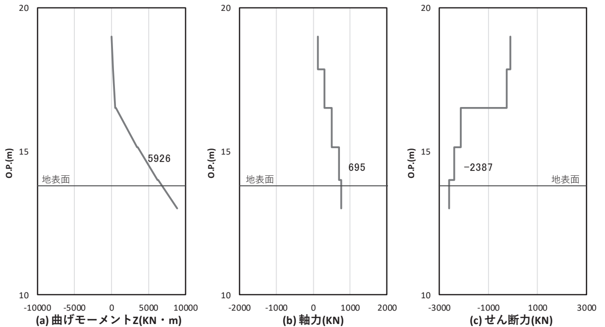
図 4.1-24 コンクリート及び鉄筋のせん断破壊に対する照査における照査時刻での断面力
