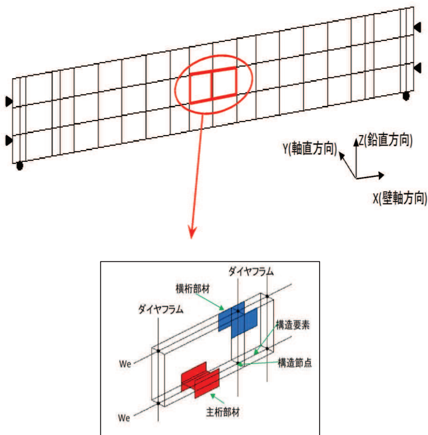
図 3.5-37(1) 鋼桁評価モデルの概念
