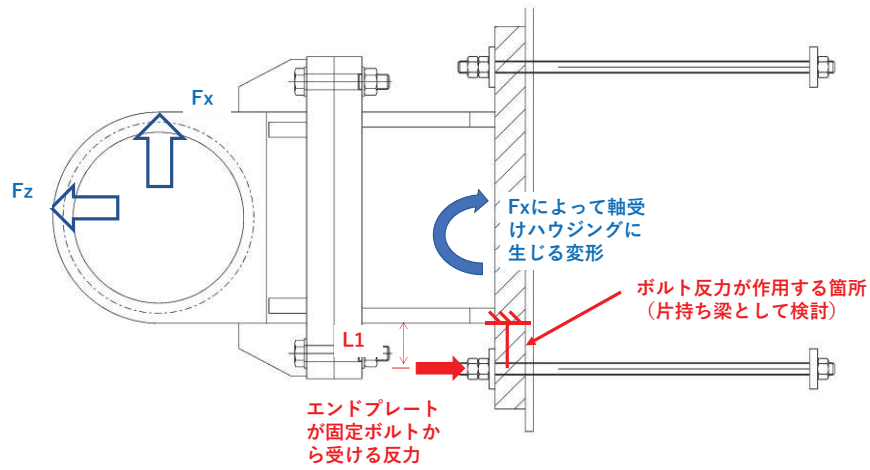
図 3.8-36 ヒンジ部エンドプレートの検討イメージ
