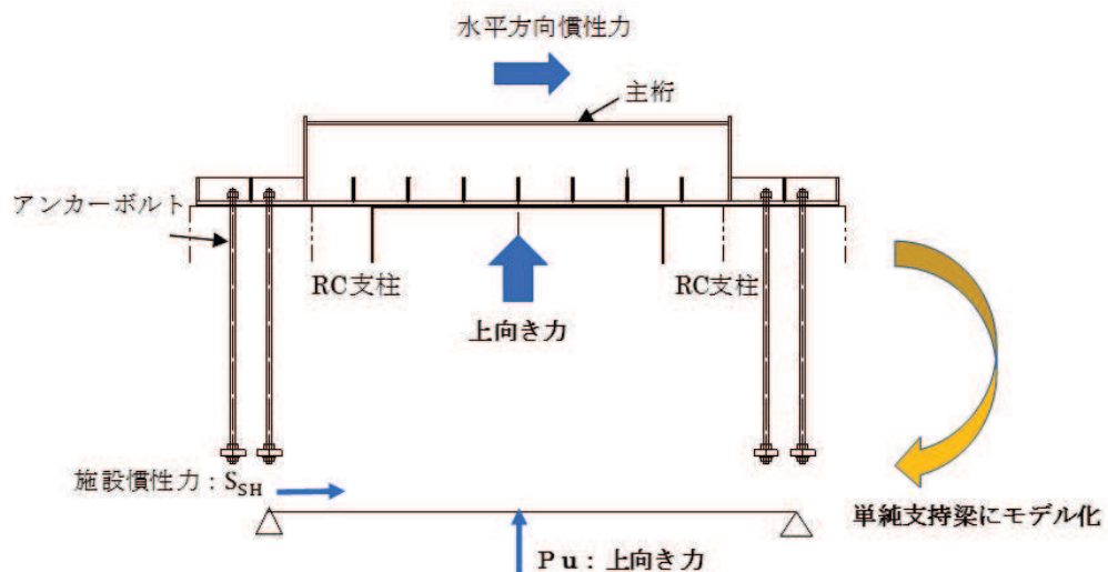
図 3.5-28 解析モデル図
