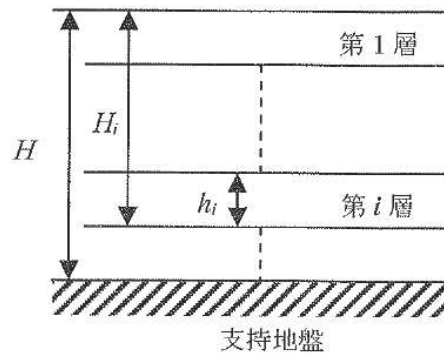
図 3.5-29 群杭係数の設定に用いる各層の概略図
