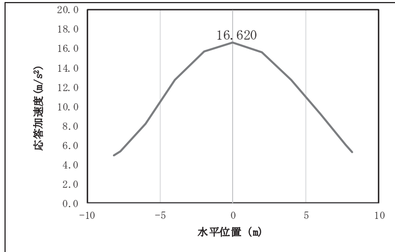
図 4.1-12(2) 鋼桁の水平応答震度分布 (鋼桁 6, S d-D 2 (-+) )
