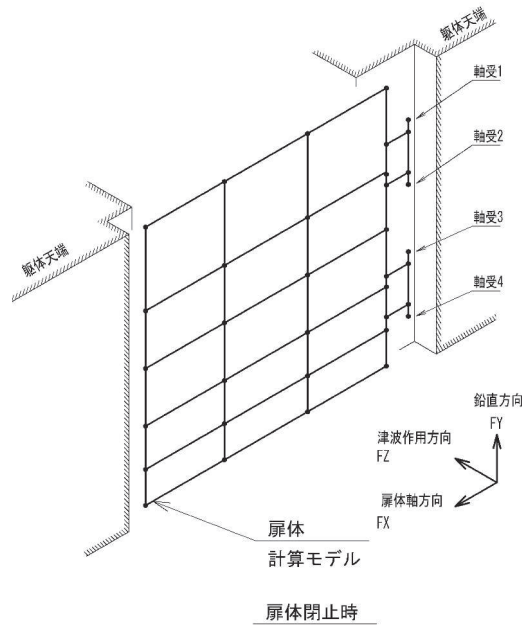
図 3.5-23 鋼製扉の計算モデル概要図
