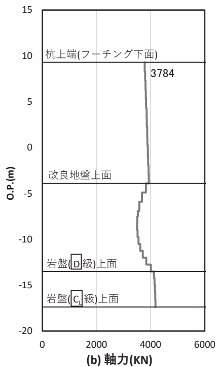
図 4.1-20 基礎地盤の支持性能照査時刻での軸力（押し込み時） （鋼製扉 3， S d - D 2（++）， t = 23.56s） 解析ケース②：地盤物性のばらつき（+1σ）を考慮した解析ケース
