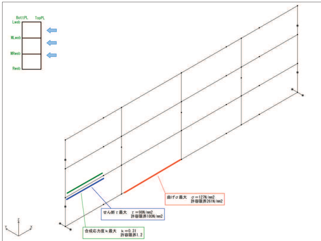
図 4.1-5(1) 鋼桁の曲げ・軸力系の破壊及びせん断破壊に対する最大照査値発生箇所（鋼桁 5）
