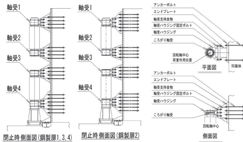
図 3.5-24 水平荷重支承部の概要図
