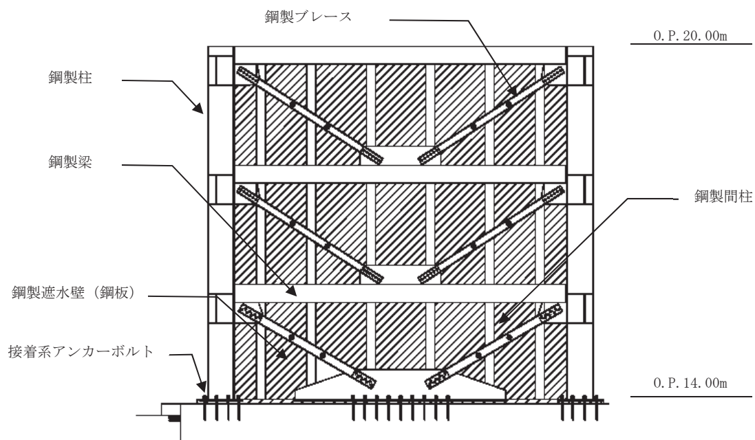
図 1-3 A - A 正面図
