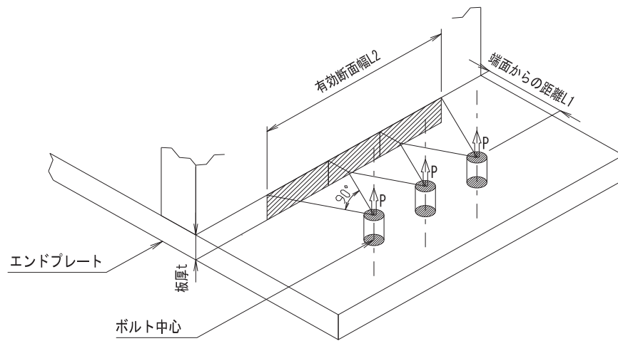
図 3.8-37 軸受ハウジングエンドプレートの有効断面イメージ
