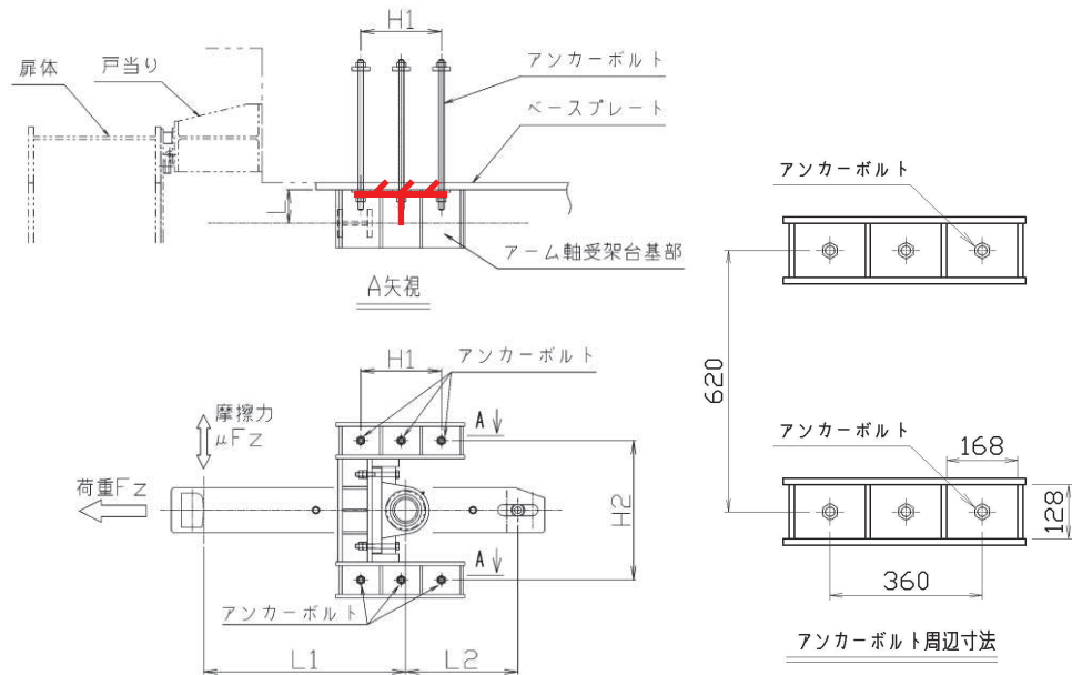
図 3.5-57 ベースプレート及びアンカーボルト周辺構造
