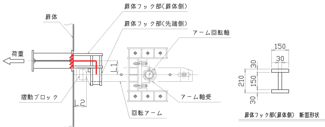
図 3.5-47 扉体フック部（扉体側）構造概要及び計算モデル概念図
