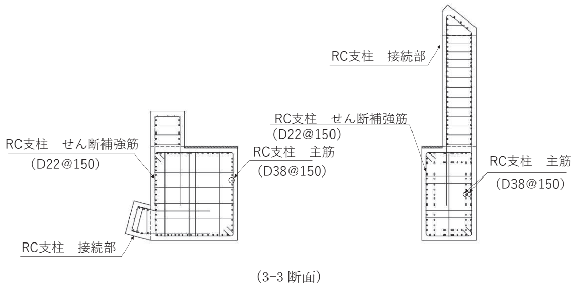
図 2.2-10 (2) RC 支柱配筋概要図 (鋼製扉 2 の例)
