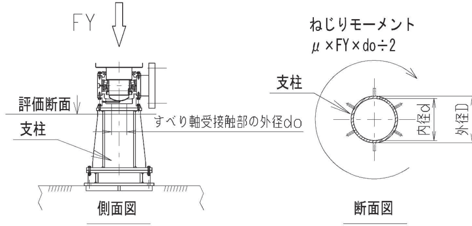
図 3.5-42 支柱の構造概要
