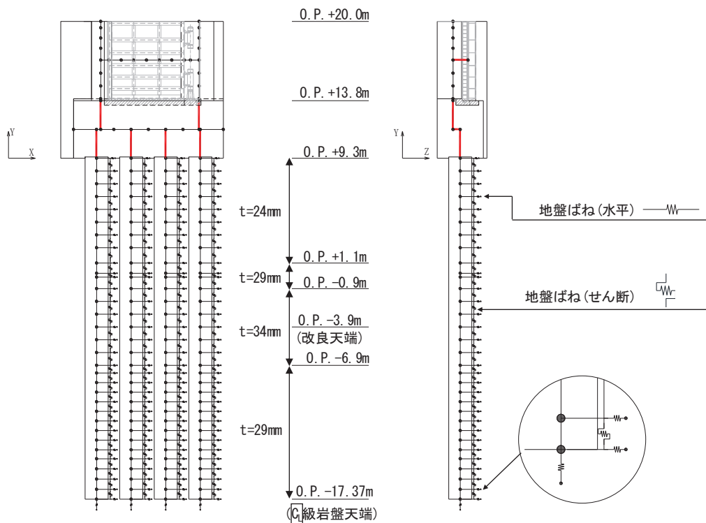
図 3.5-16 静的解析モデル（鋼製扉 3 の例）
