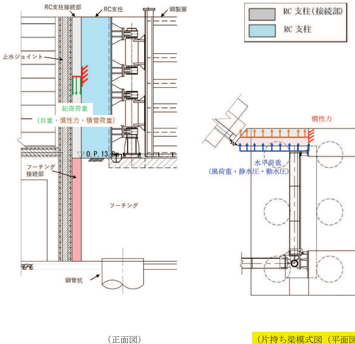
図3.5-62 RC支柱接続部照査用モデル概念図
