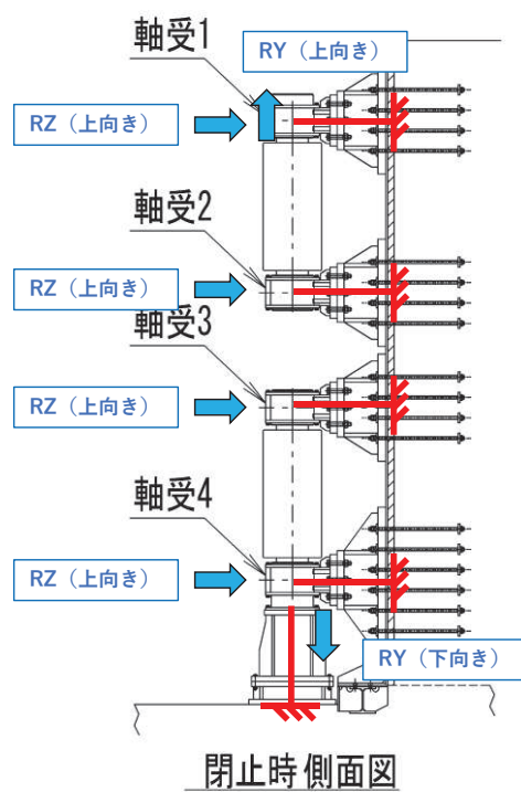
図 3.5-25 ヒンジ水平荷重支承部に伝達する荷重と評価用モデルのイメージ図
