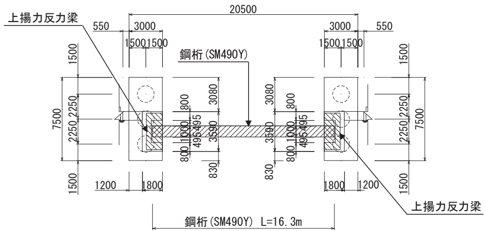
図 2.2-9(1) 鋼製遮水壁（鋼桁 6） 正面図及び断面図
