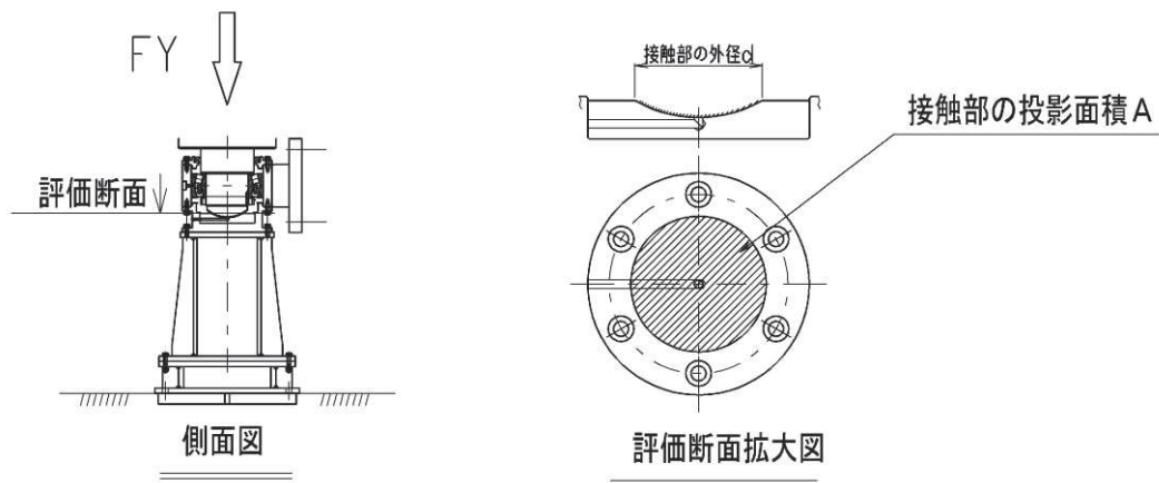
図 3.5-41 すべり軸受の構造概要図
