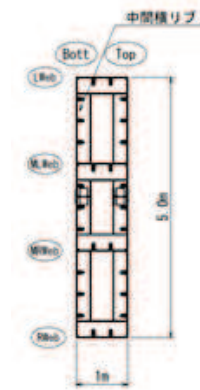
(中間横リブ)
