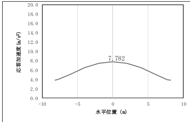
図 4.1-12(7) 鋼桁の鉛直応答震度分布 (鋼桁 6, S d-D 2 (+-))
