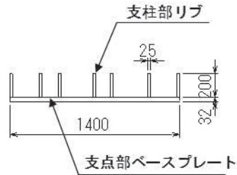
図 3.5-62 評価断面概念図
