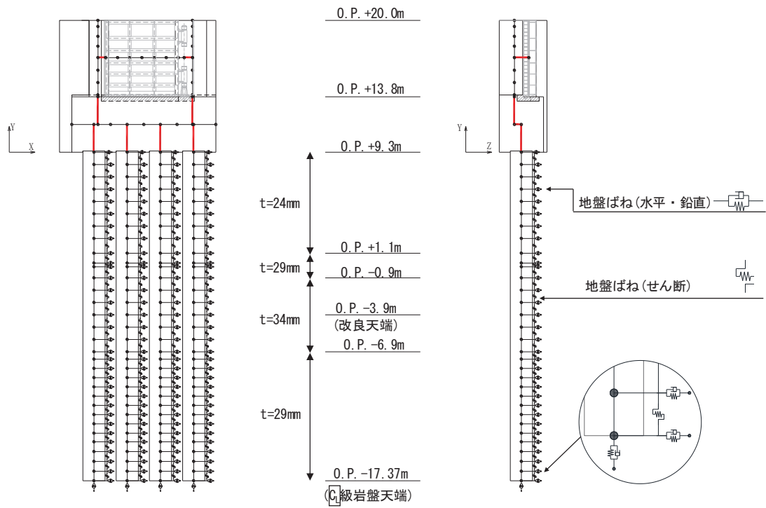
図 3.5-17 固有値解析モデル (鋼製扉 3 の例)
