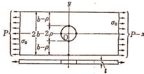
図 3.5-50 応力集中係数の計算モデル概要図
