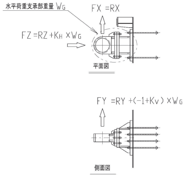
図 3.5-26 評価に用いる荷重の概要図
