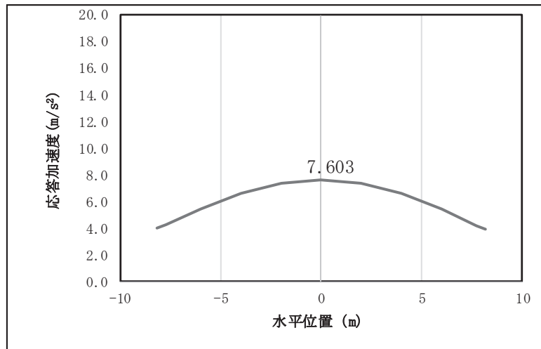
図 4.1-12(8) 鋼桁の鉛直応答震度分布 (鋼桁 6, S d-D 2 (--))
