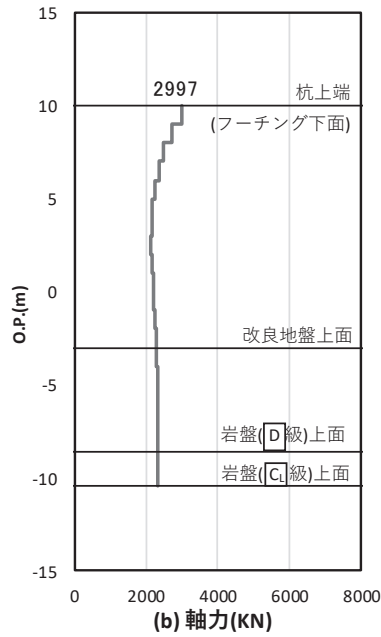
図 4.1-51(1) 基礎地盤の支持性能照査時刻での軸力 (押し込み) (鋼桁 5, 基礎 1, S d-D 2 (-+), t=25.40s) 解析ケース②: 地盤物性のばらつき (+1σ) を考慮した解析ケース
