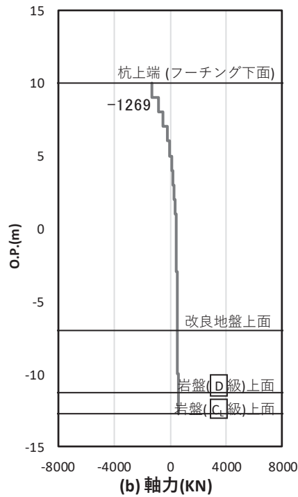
図 4.1-52 (2) 基礎地盤の支持性能照査時刻での軸力 (引き抜き)
