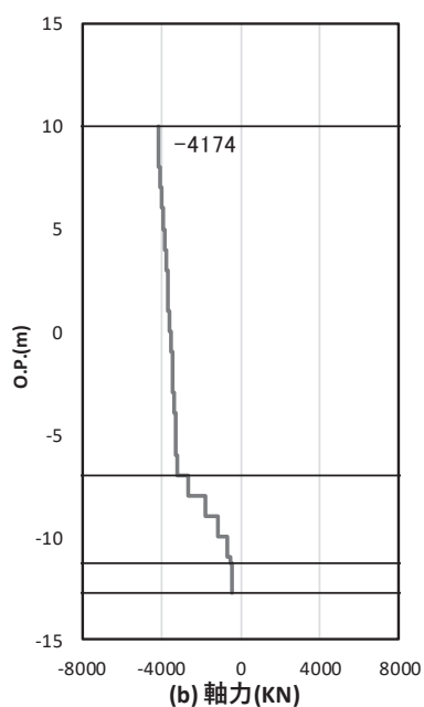
図 4.1-50 基礎地盤の支持性能照査時刻での軸力（引き抜き） （鋼桁 6，基礎 1，S d-D 2（-+），t = 25.48s） 解析ケース②：地盤物性のばらつき（+1σ）を考慮した解析ケース
