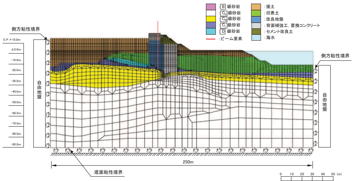
図 5.3-2(2) 解析モデル (防潮堤 (鋼管式鉛直壁) 断面②)
