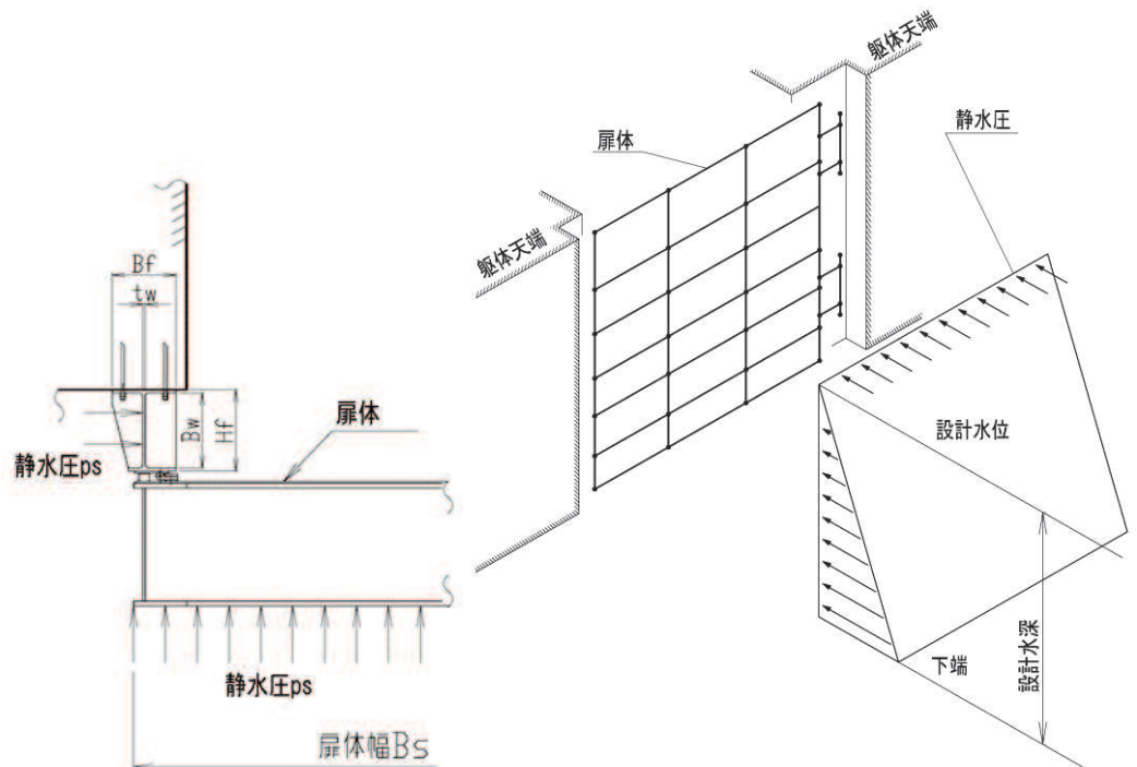
図 3.5-60(2) 戸当り（側部）の評価に用いた荷重の概要図
