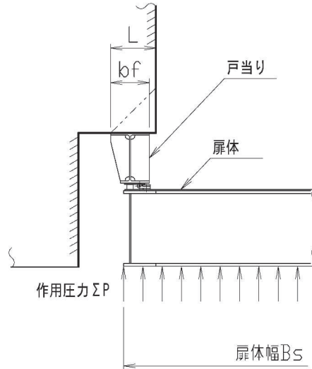
図 3.5-60 戸当りコンクリートの発生応力度の計算諸元に関する概要図
