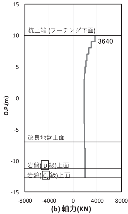
図 4.1-52 (1) 基礎地盤の支持性能照査時刻での軸力 (押し込み)
