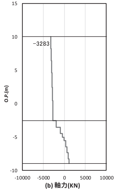
図 4.1-42 基礎地盤の支持性能照査時刻での軸力（引き抜き） （鋼桁 2，基礎 1，S d-D 2（++），t = 25.44s） 解析ケース②：地盤物性のばらつき（+1σ）を考慮した解析ケース
