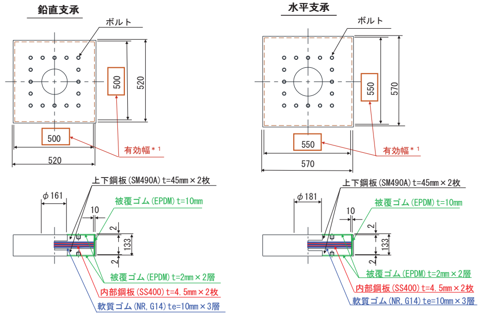
(鋼桁 1, 4)
