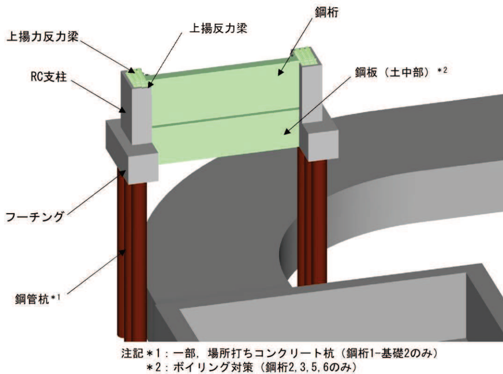
(全体図)
