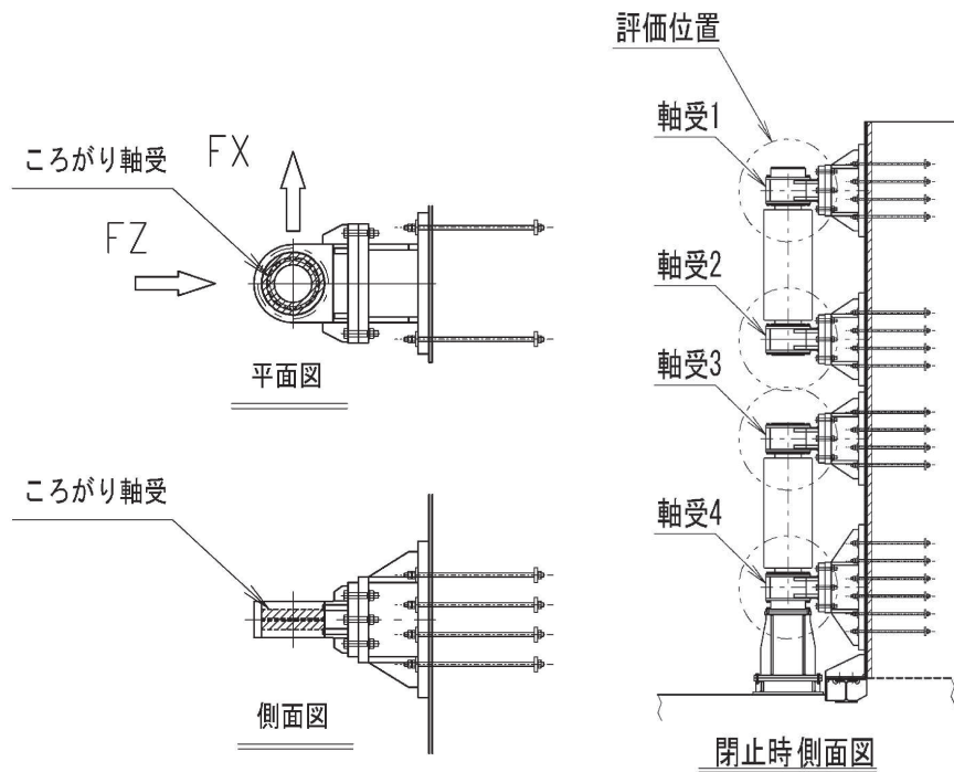
図 3.5-27 ころがり軸受の作用荷重の概要図
