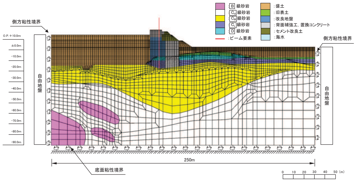
図 5.3-2(3) 解析モデル (防潮堤 (鋼管式鉛直壁) 断面③)
