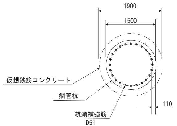
図 3.5-67 仮想鉄筋コンクリート断面概念図
