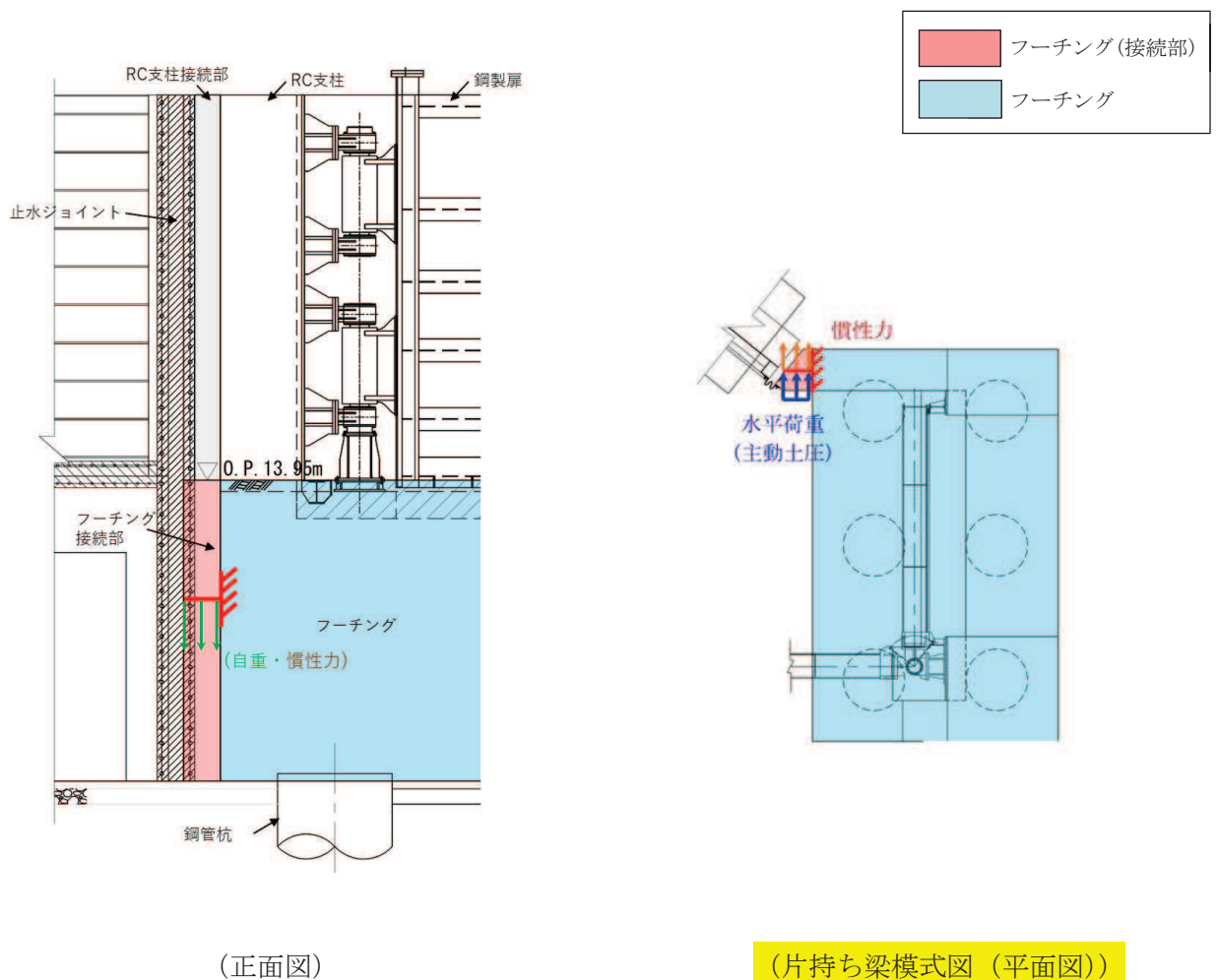
図 3.5-65 フーチング接続部照査用モデル概念図
