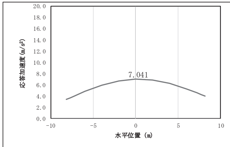
図 4.1-11(5) 鋼桁の鉛直応答震度分布 (鋼桁 5, S d-D 2 (++) (改良幅 2D 未満) 考慮)
