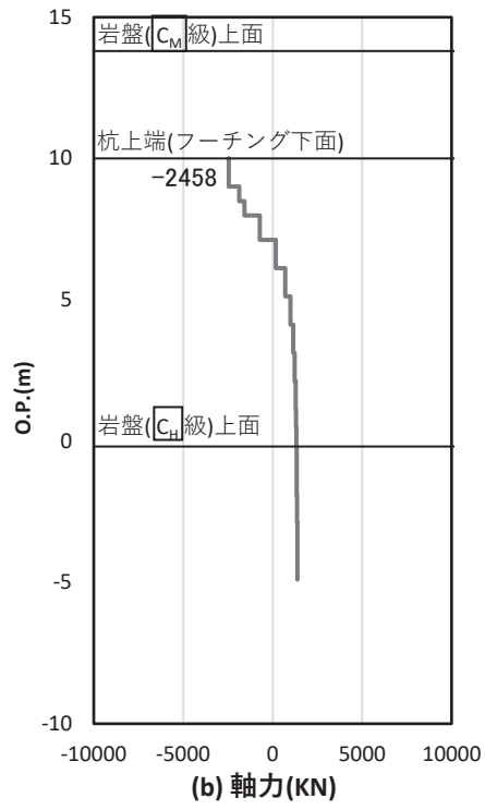
図 4.1-21 基礎地盤の支持性能照査時刻での軸力（引き抜き時） （鋼製扉 2， S d - D 2（+-）， t = 13.38s） 解析ケース③：地盤物性のばらつき（-1σ）を考慮した解析ケース
