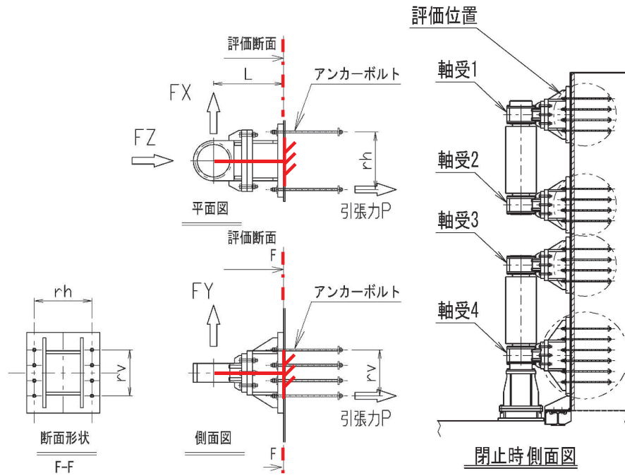
図 3.5-39 アンカーボルトの概要図
