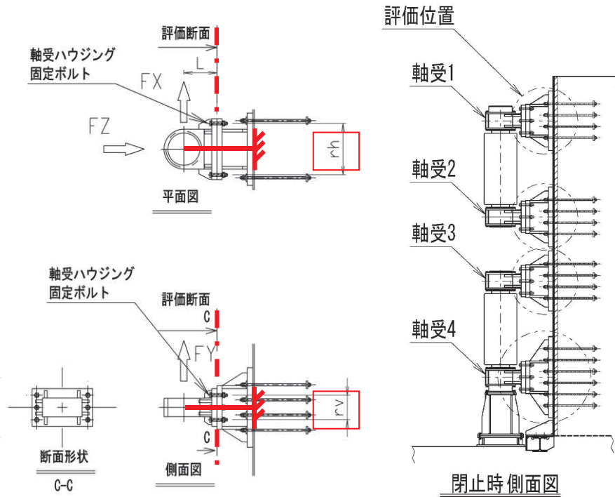
図 3.5-30 軸受ハウジング固定ボルトの概要図
