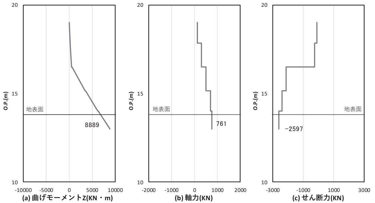
図 4.1-23 コンクリート及び鉄筋の曲げ・軸力系の破壊に対する照査における 曲げモーメント最大時刻での断面力
