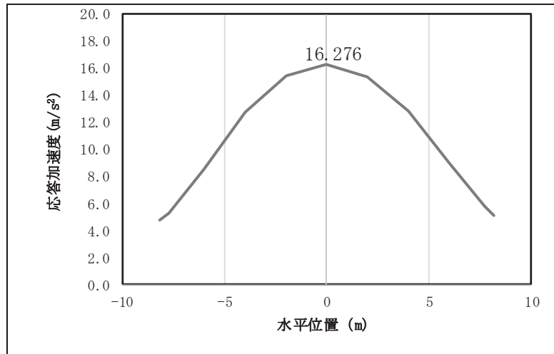
図 4.1-12(1) 鋼桁の水平応答震度分布 (鋼桁 6, S d-D 2 (++) )
