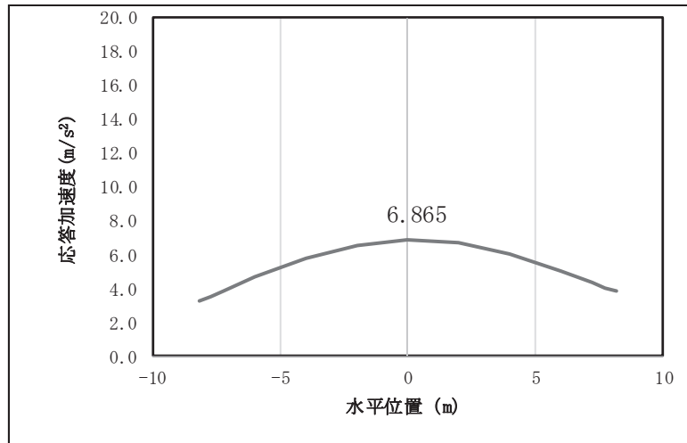
図 4.1-11(7) 鋼桁の鉛直応答震度分布 (鋼桁 5, S d-D 2 (+-) (改良幅 2D 未満) 考慮)
