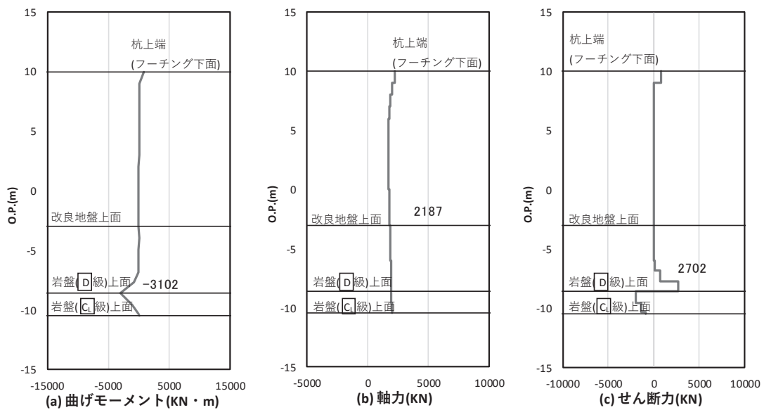
図 4.1-40 鋼管杭のせん断破壊に対する照査における照査時刻での断面力 (鋼桁 5, 基礎 2, S d-D 2 (++) , t =25.50s) 解析ケース②: 地盤物性のばらつき (+1σ) を考慮した解析ケース
