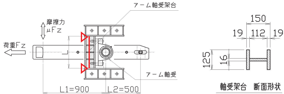
図 3.5-55 アーム軸受架台周辺構造及び断面形状
