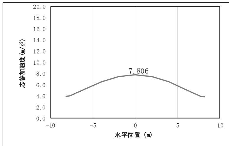
図 4.1-12(6) 鋼桁の鉛直応答震度分布 (鋼桁 6, S d-D 2 (-+))
