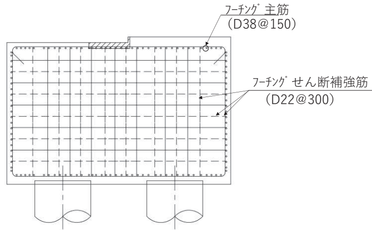
(1-1 断面)
