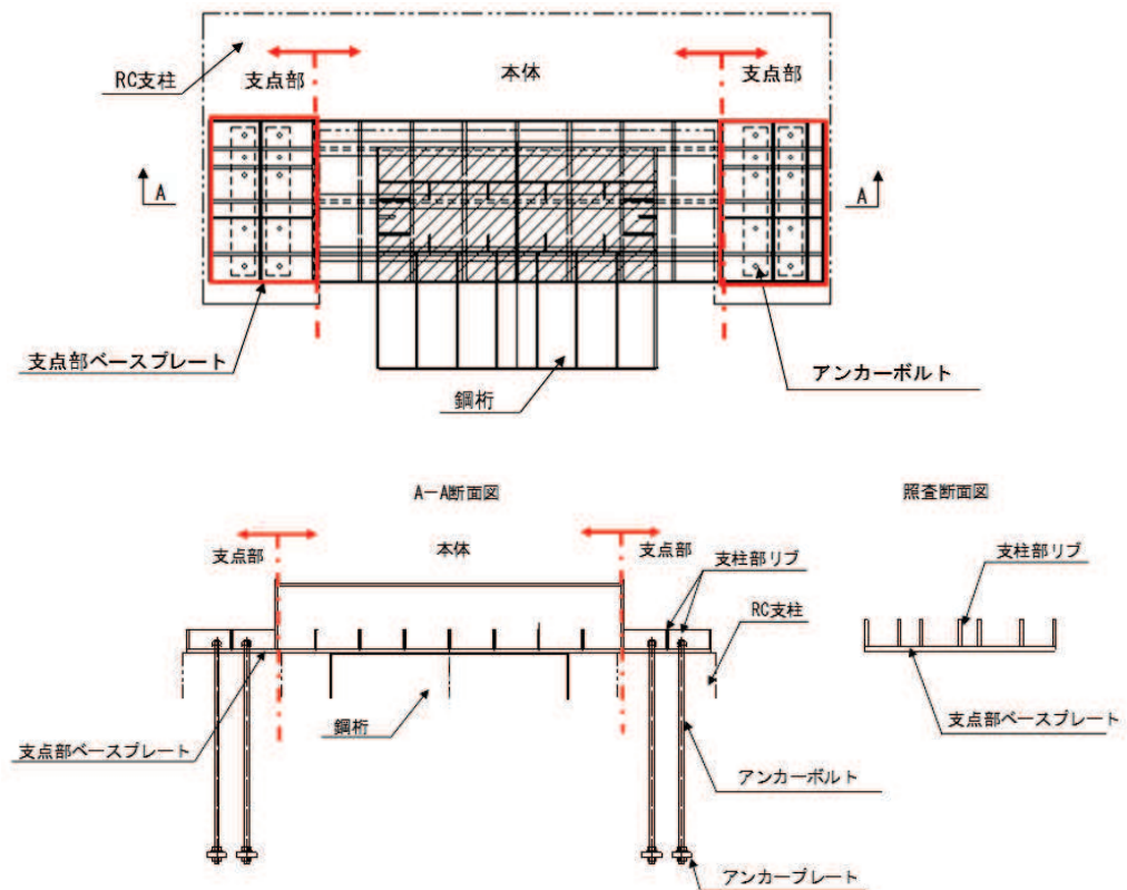
図 3.5-59 ベースプレート概要図
