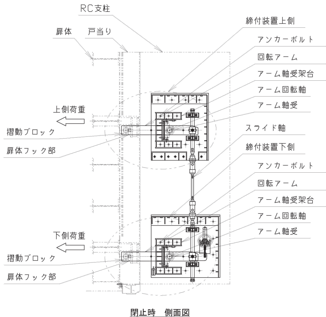
図 3.5-44 締付装置側面 概要図
