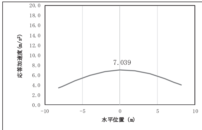
図 4.1-11(8) 鋼桁の鉛直応答震度分布 (鋼桁 5, S d-D 2 (--)) (改良幅 2D 未満) 考慮)
