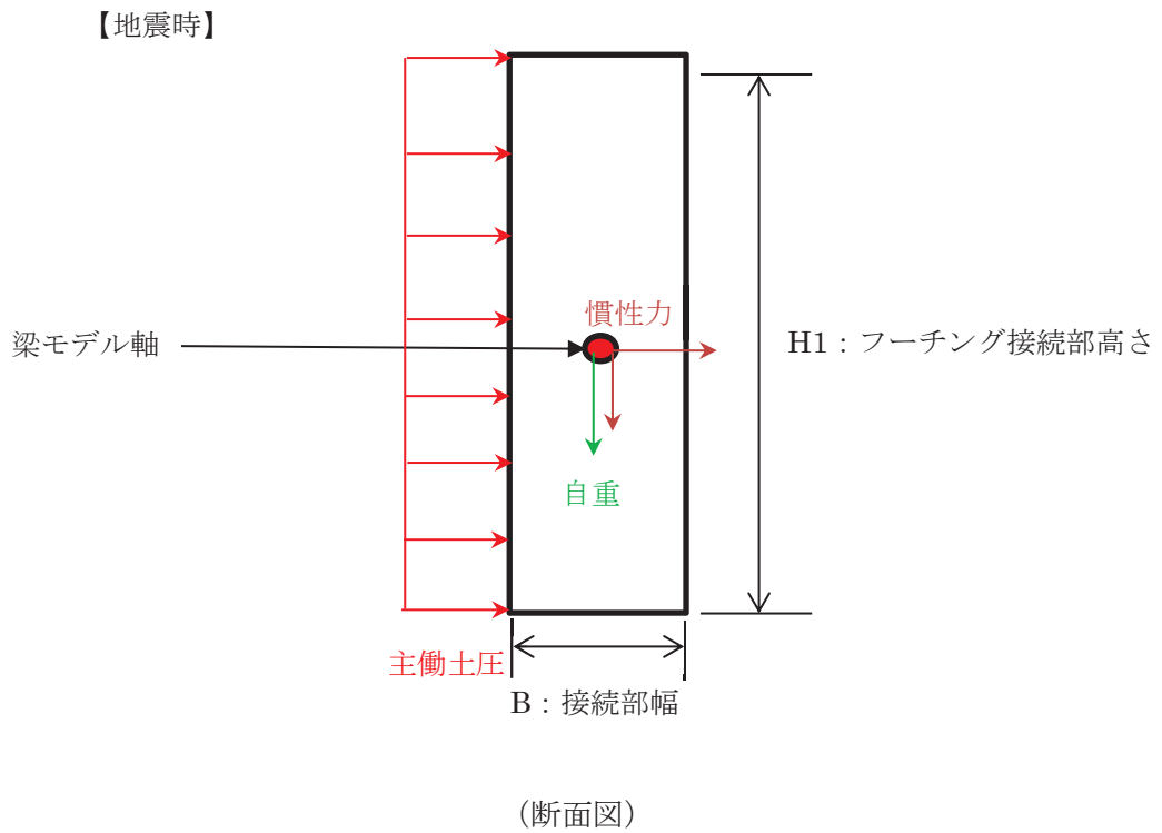
図 3.5-66 フーチング（接続部）作用荷重イメージ図
