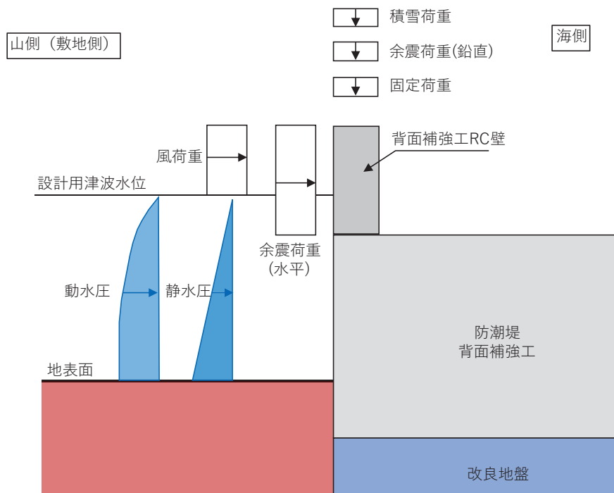
図 5.2-1(2) 荷重の概念図 (重畳時)
