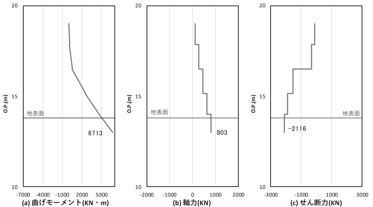
図 4.1-21 鉄筋の曲げ・軸力系の破壊に対する照査における
