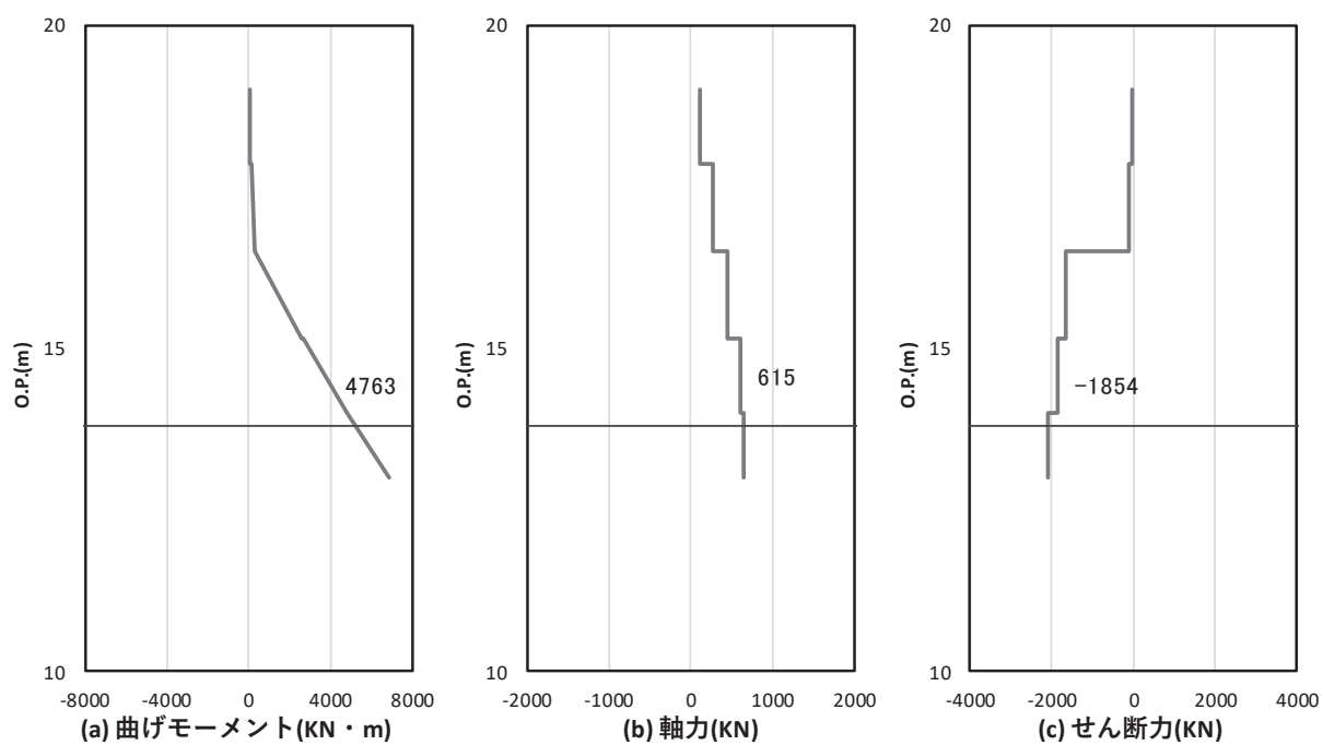
図 4.1-19(3) コンクリート及び鉄筋のせん断破壊に対する照査における照査時刻での断面力 (鋼桁 6, 基礎 2, S d-D 2 (-+), t = 13.72s ) 解析ケース②: 地盤物性のばらつき ( +1\sigma ) を考慮した解析ケース
