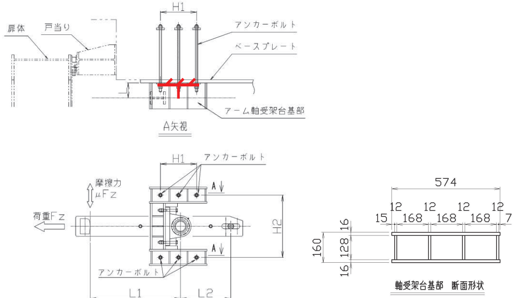
図 3.5-56 アーム軸受架台基部周辺構造及び断面形状
