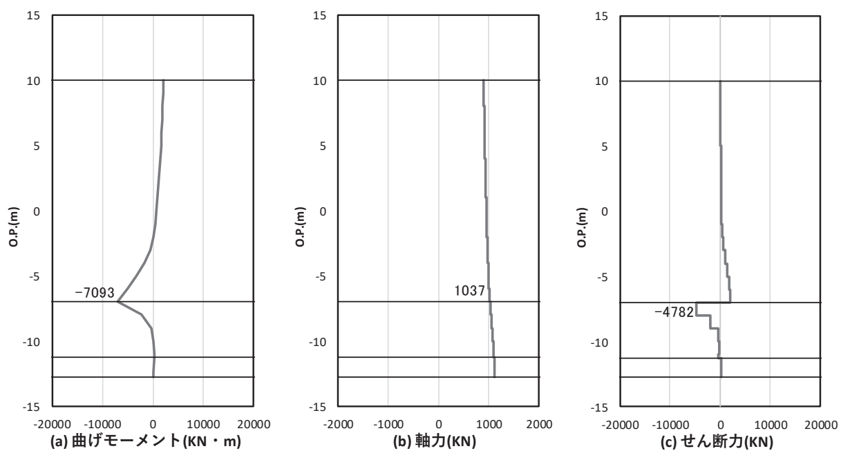
図 4.1-38 鋼管杭のせん断破壊に対する照査における照査時刻での断面力 (鋼桁6, 基礎1, S d-D 2 (-+), t = 13.44s) 解析ケース②: 地盤物性のばらつき (+1σ) を考慮した解析ケース
