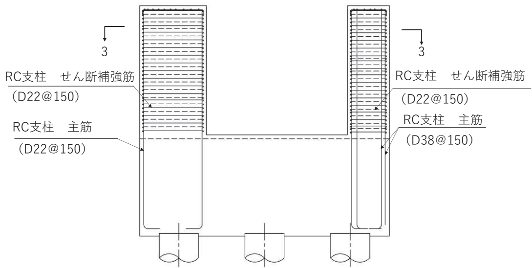
(1-1 断面)
