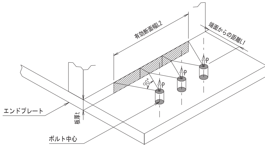
図 3.8-33 軸受ハウジングエンドプレートの有効断面イメージ
