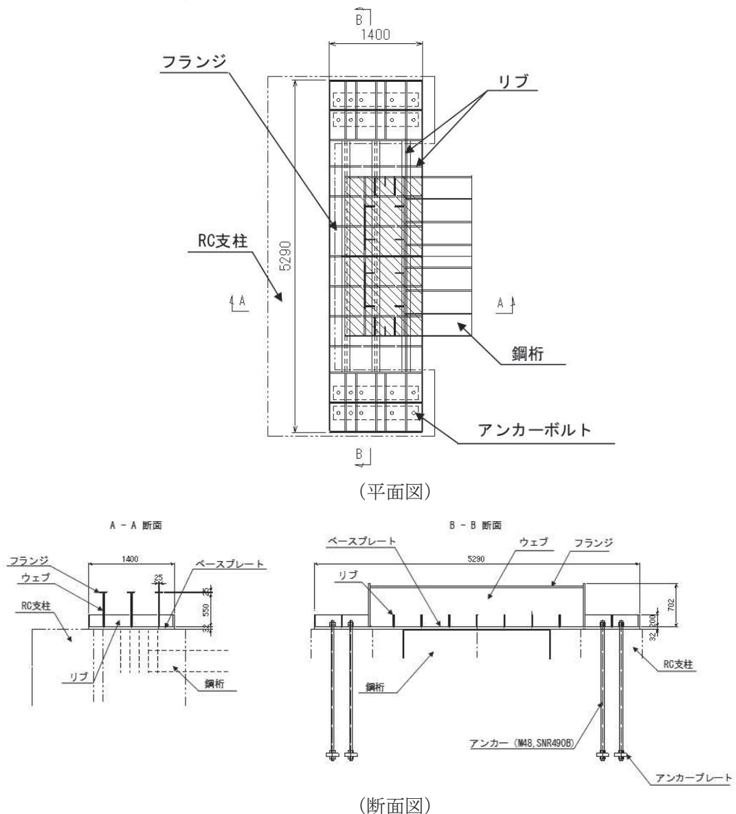
図 3.5-55 上揚力反力梁構造概要
