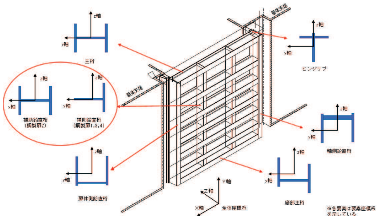
図 3.5-19 扉体の構造概要図
