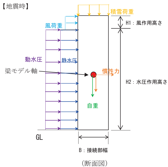
図 3.5-63 RC 支柱接続部作用荷重イメージ図 (断面図)
