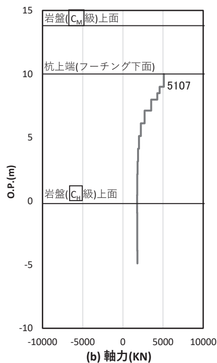
図 4.1-19 基礎地盤の支持性能照査時刻での軸力（押し込み時） （鋼製扉 2， S d - D 2（+-）， t = 26.88s） 解析ケース③：地盤物性のばらつき（-1σ）を考慮した解析ケース
