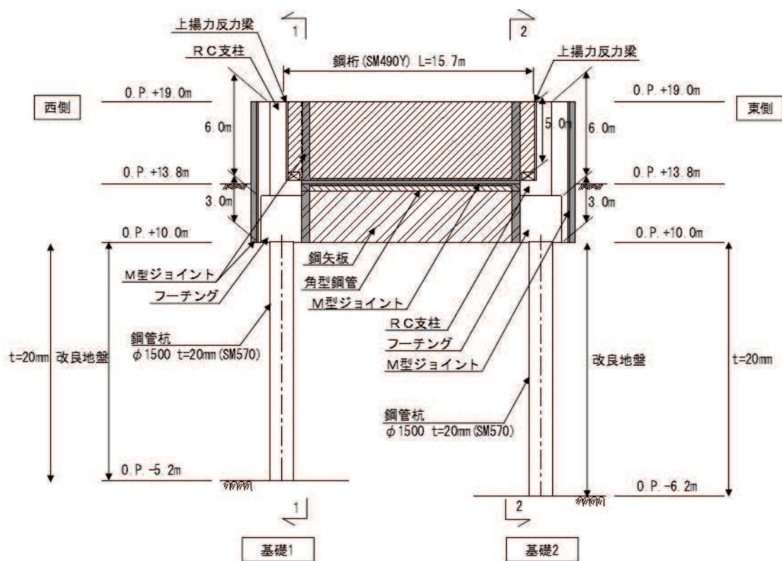
(正面図)
