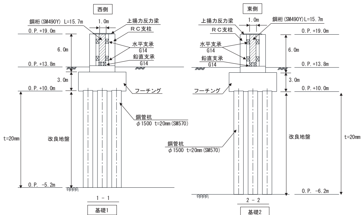
(断面図)
