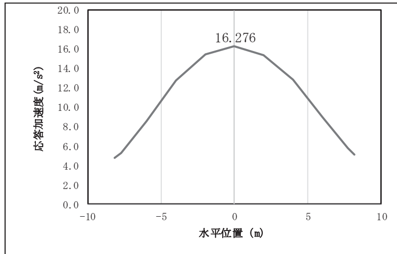
図 4.1-12(4) 鋼桁の水平応答震度分布 (鋼桁 6, S d-D 2 (---))
