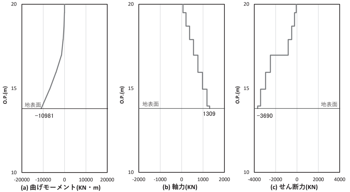
図 4.1-11(1) コンクリート及び鉄筋の曲げ・軸力系の破壊に対する照査における 最大曲げモーメント発生時刻での断面力 (鋼製扉 3, S d - D 2 (—), t = 25.56s)
