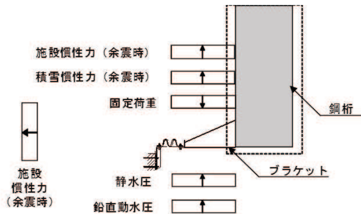
図 3.5-45 作用荷重図
