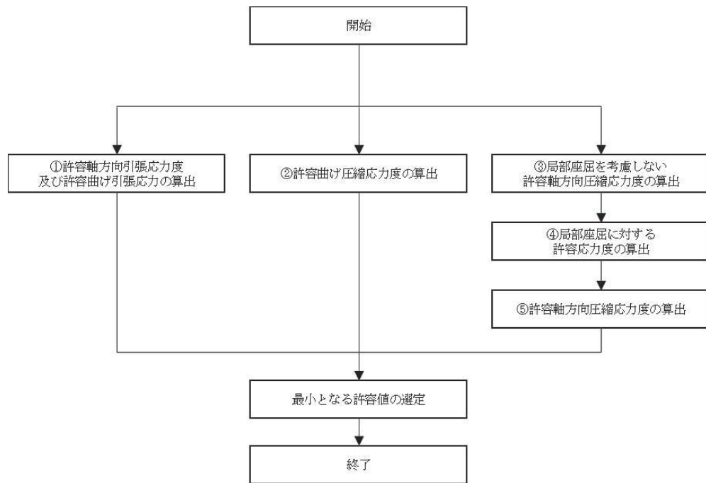
図 3.4-2 鋼桁の許容限界算定フロー
