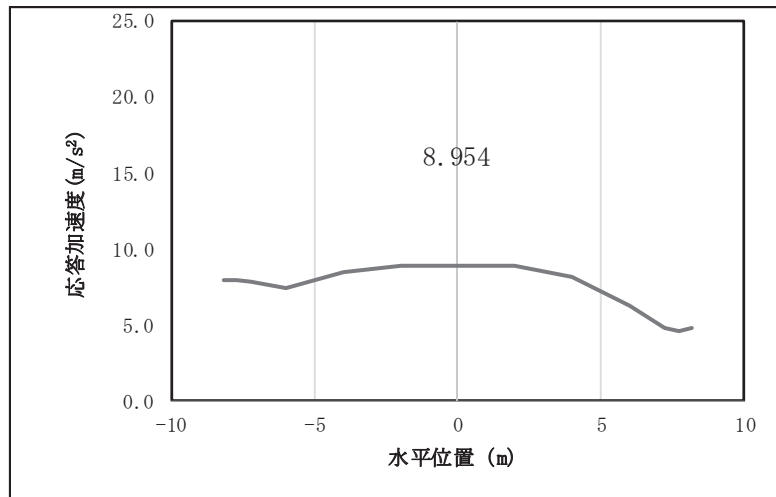
図 4.1-11(2) 鋼桁の水平応答震度分布 (鋼桁 5, S d-D 2 (-+) (改良幅 2D 未満) 考慮)
