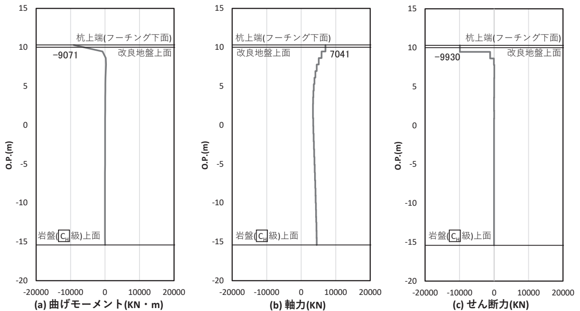
図 4.1-28(2) 場所打ちコンクリート杭のせん断破壊に対する照査における照査時刻での断面力 (鋼桁 1, 基礎 2, S d-D 2 (-+), t=23.66s)
