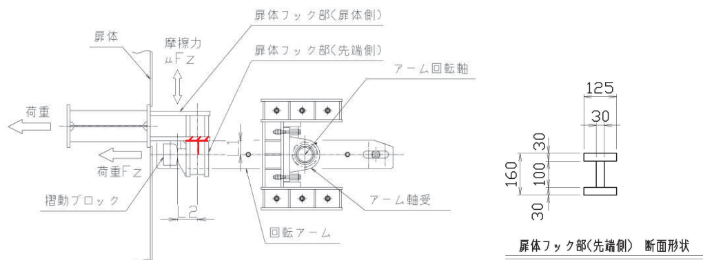
図 3.5-46 扉体フック部（先端側）構造概要及び計算モデル概念図
