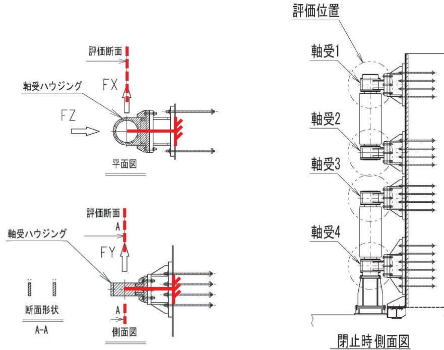
図 3.5-28 軸受ハウジング円筒部の外形図
