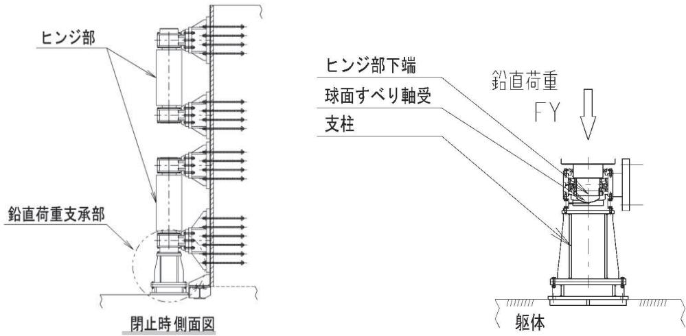
図 3.8-40 鉛直荷重支承部の構造概要
