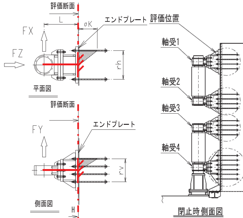
図 3.5-38 エンドプレートコンクリート支圧応力度に関する概要図
