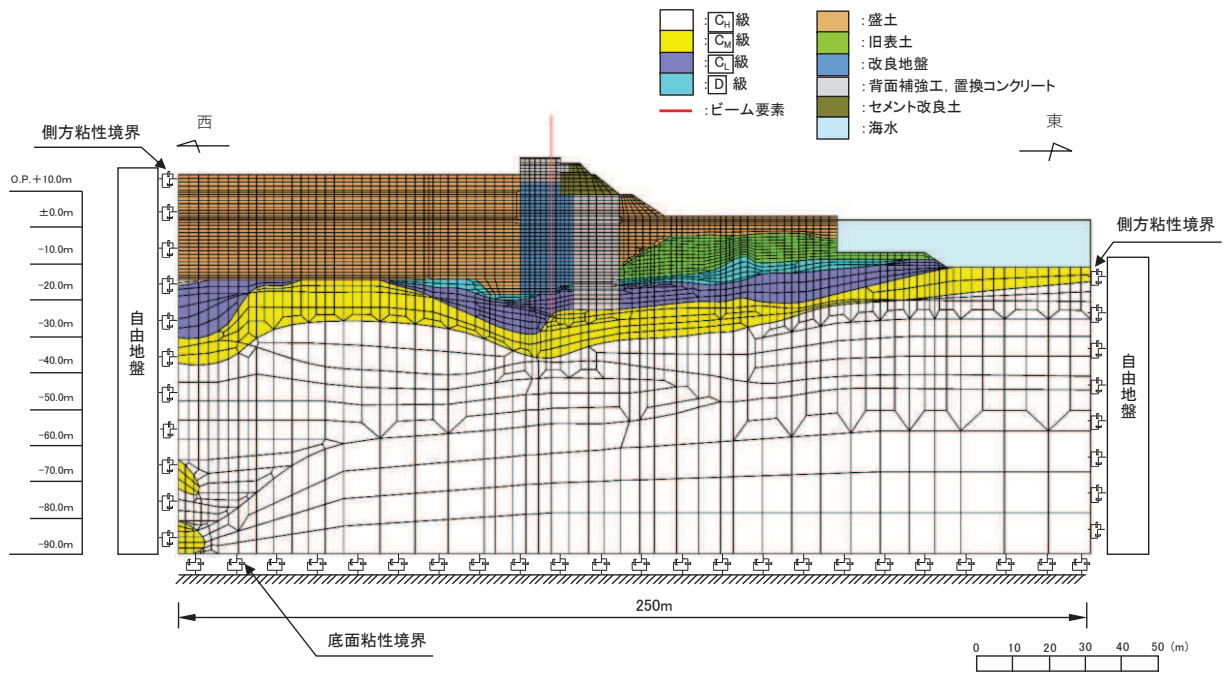
図 5.3-2(1) 解析モデル (防潮堤 (鋼管式鉛直壁) 断面①)
