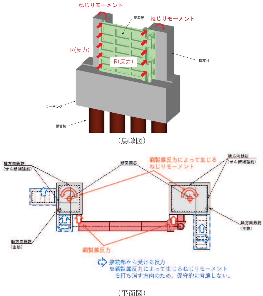
図 3.5-61 RC支柱へのねじりモーメント(反力)作用イメージ
