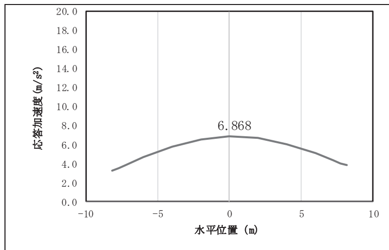
図 4.1-11(6) 鋼桁の鉛直応答震度分布 (鋼桁 5, S d-D 2 (-+) (改良幅 2D 未満) 考慮)
