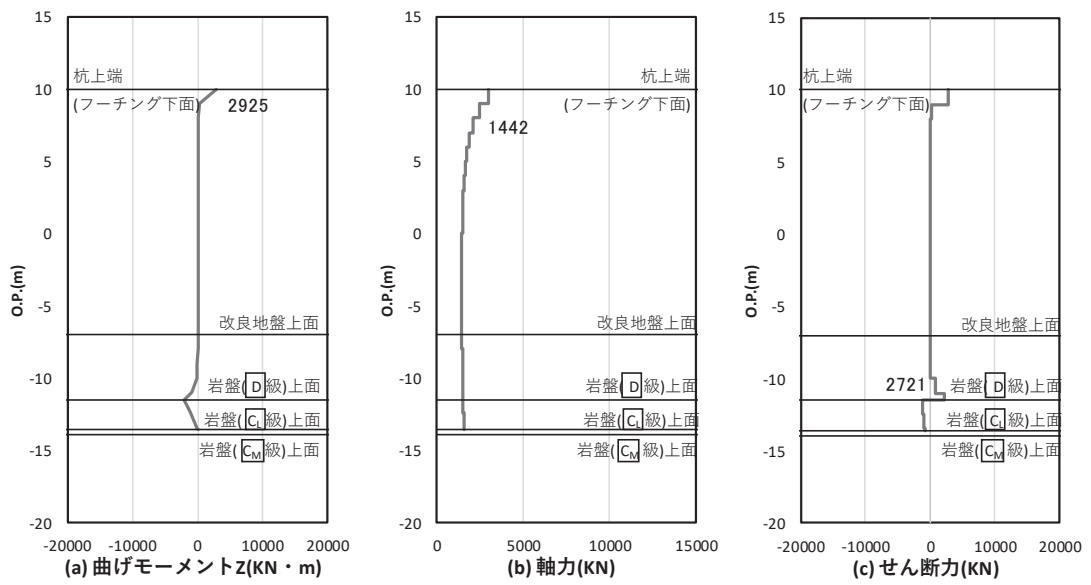
図 4.1-42 鋼管杭のせん断破壊に対する照査における照査時刻での断面力 (鋼桁 6, 基礎 1, S d-D 2 (+), t=14.07s) 解析ケース②: 地盤物性のばらつき (+1σ) を考慮した解析ケース
