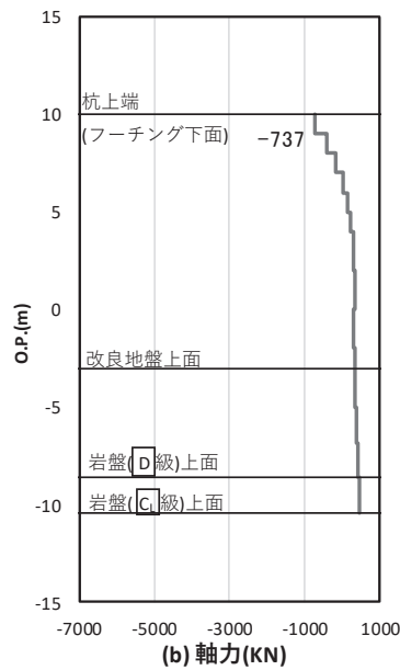
図 4.1-51(2) 基礎地盤の支持性能照査時刻での軸力 (引き抜き) (鋼桁 5, 基礎 2, S d-D 2 (++) , t=25.53s) 解析ケース③: 地盤物性のばらつき (+1σ) を考慮した解析ケース
