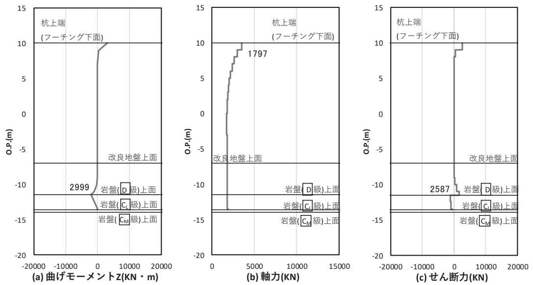
図 4.1-41 鋼管杭の曲げ・軸力系の破壊に対する照査における照査時刻での断面力 (鋼桁 6, 基礎 2, S d-D 2 (++) , t = 14.07s)
