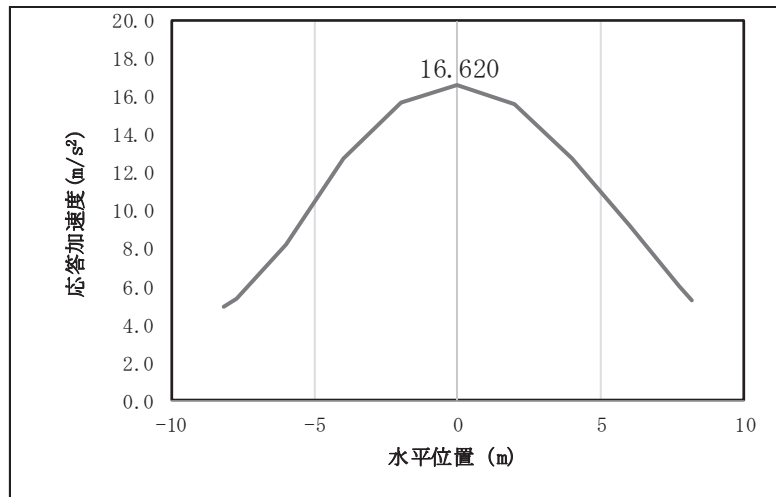
図 4.1-12(3) 鋼桁の水平応答震度分布 (鋼桁 6, S d-D 2 (+-) )
