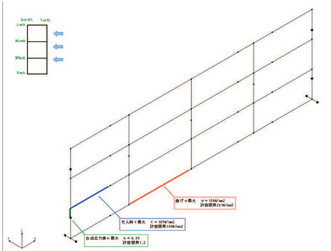
図 4.1-6(1) 鋼桁の曲げ・軸力系の破壊及びせん断破壊に対する 最大照査値発生個所（鋼桁 6）
