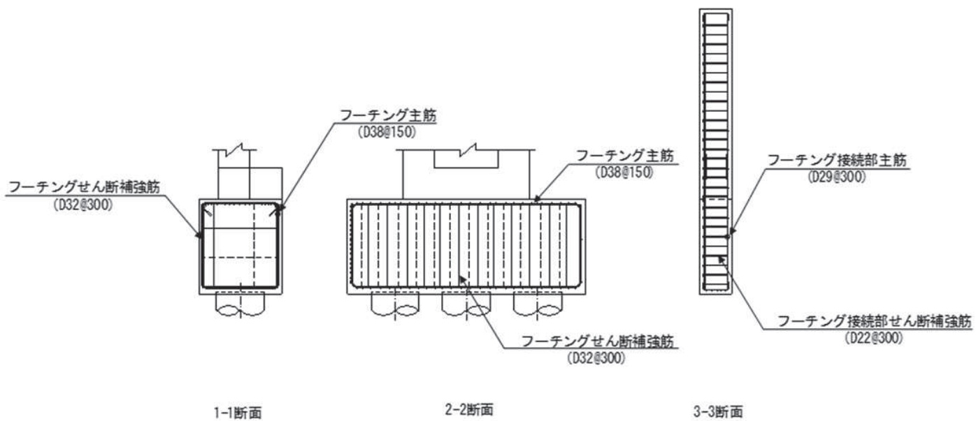
図 2.2-14 鋼製遮水壁（鋼桁）のフーチング配筋概要図
