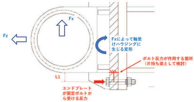
図 3.8-32 軸受ハウジングエンドプレートの検討イメージ
