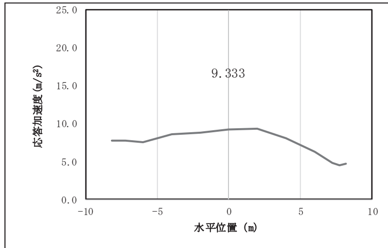
図 4.1-11(1) 鋼桁の水平応答震度分布 (鋼桁 5, S d-D 2 (++) (改良幅 2D 未満) 考慮)
