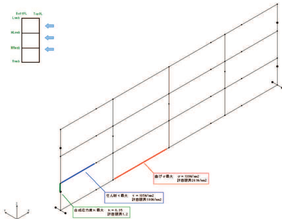
図 4.1-6(2) 鋼桁の曲げ・軸力系の破壊及びせん断破壊に対する 最大照査値発生個所（鋼桁 6）（地盤改良（改良幅 2D 未満）考慮）
