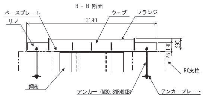
(断面図)
