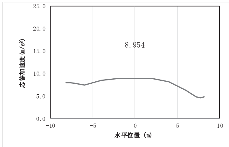
図 4.1-11(3) 鋼桁の水平応答震度分布 (鋼桁 5, S d-D 2 (+) (改良幅 2D 未満) 考慮)
