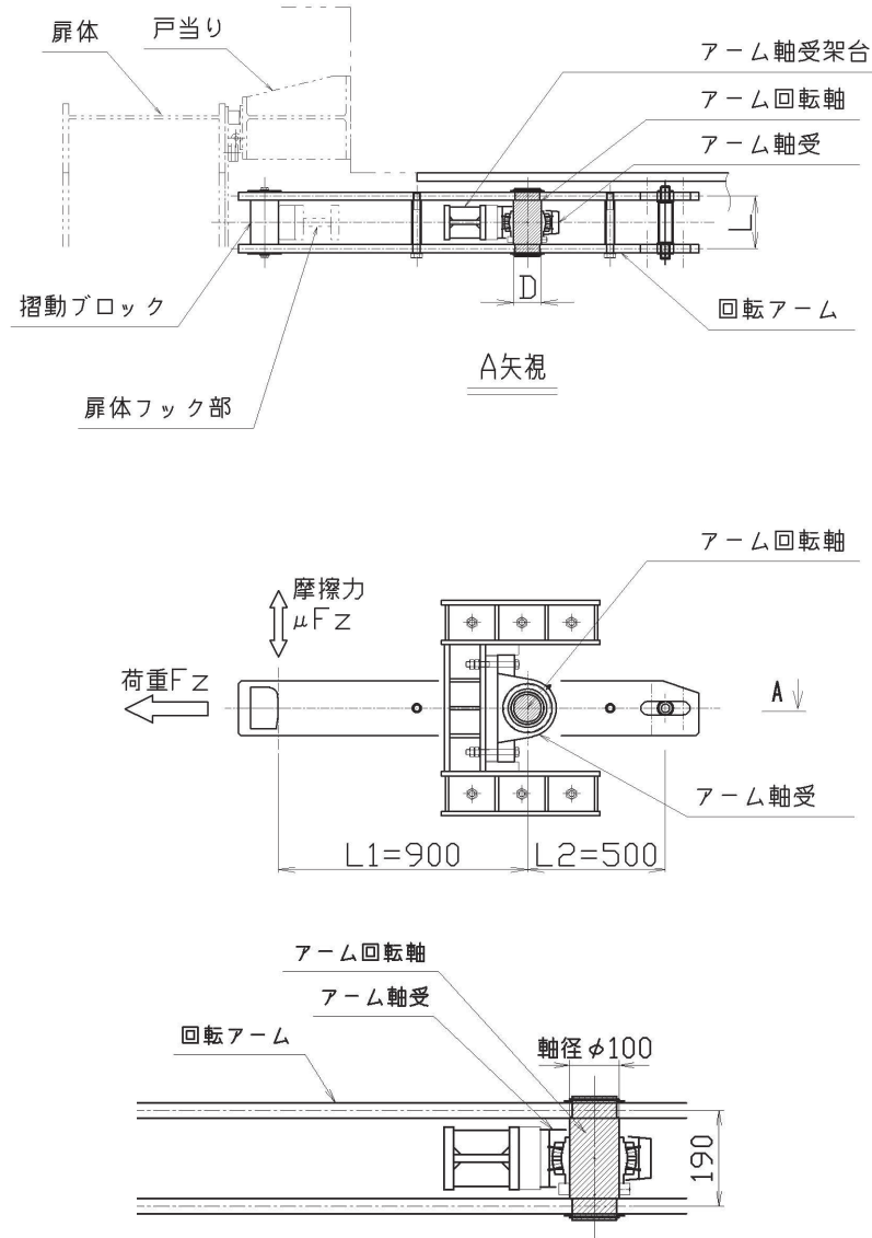
図 3.5-52 アーム回転軸周辺構造
