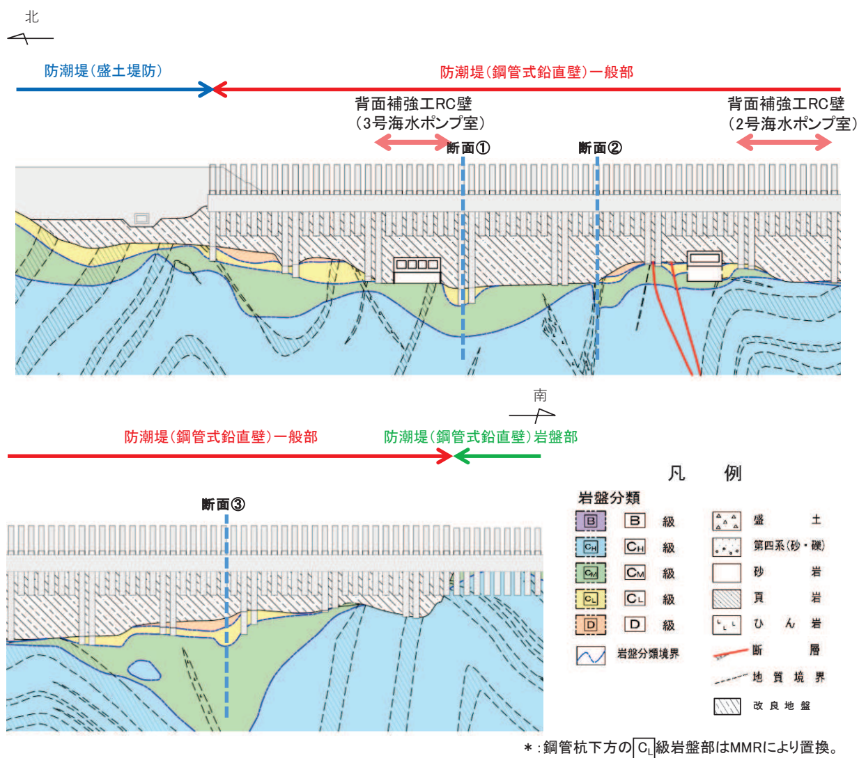
図 5.3-1(2) 地震応答解析の実施位置 (防潮堤縦断面図)
