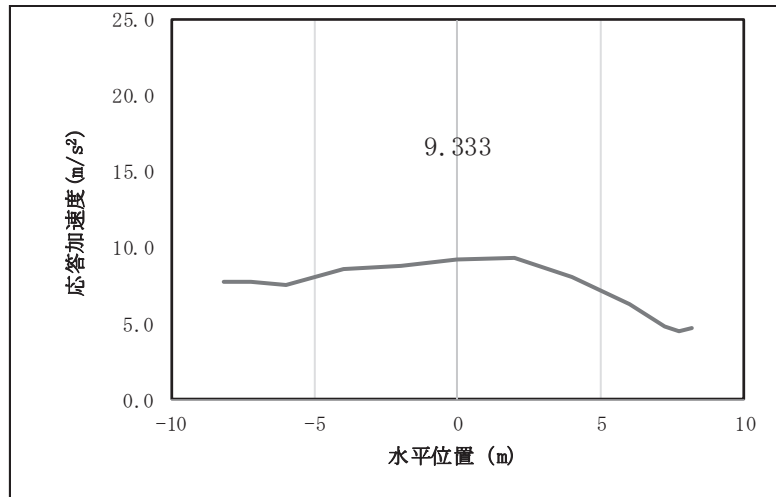
図 4.1-11(4) 鋼桁の水平応答震度分布 (鋼桁 5, S d-D 2 (--) (改良幅 2D 未満) 考慮)
