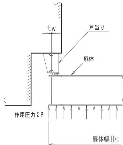
図 3.5-59 戸当り腹板の発生応力度の計算諸元に関する概要図
