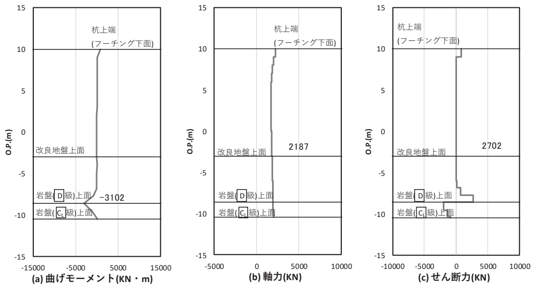
図 4.1-39 鋼管杭の曲げ・軸力系の破壊に対する照査における照査時刻での断面力 (鋼桁 5, 基礎 2, S d-D 2 (++) , t = 25.50s)
