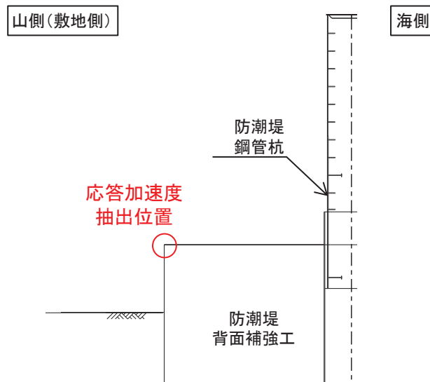
図 5.3-2 応答加速度の抽出位置
