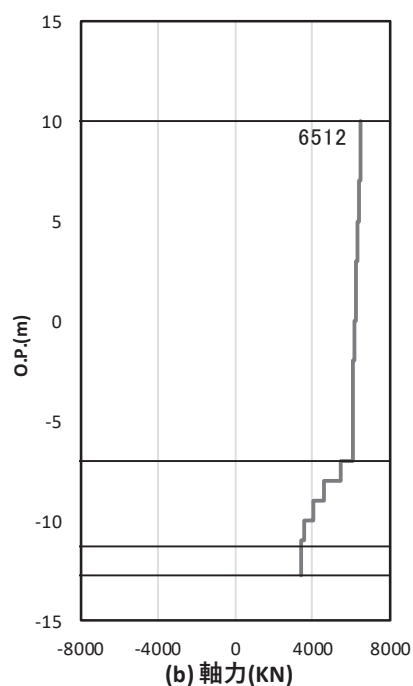
図 4.1-49 基礎地盤の支持性能照査時刻での軸力（押し込み） （鋼桁 6，基礎 1，S d-D 2（-+），t = 25.50s） 解析ケース②：地盤物性のばらつき（+1σ）を考慮した解析ケース
