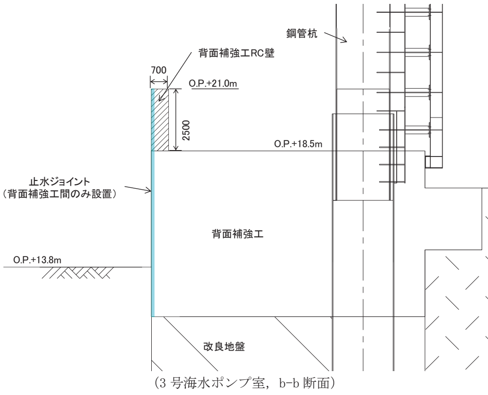
図 1-2(2) 防潮堤背面補強工部の構造概要図 (断面図)
