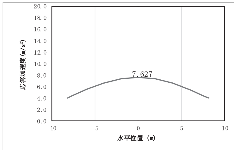
図 4.1-12(5) 鋼桁の鉛直応答震度分布 (鋼桁 6, S d-D 2 (++))
