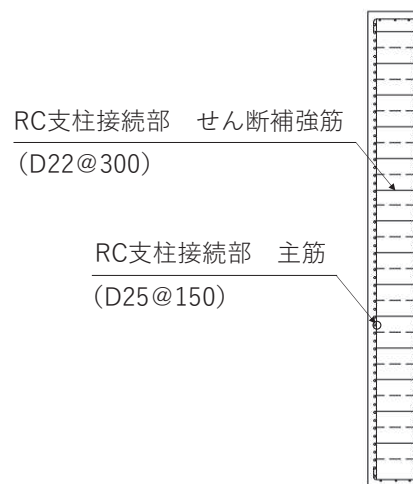
(2-2 断面)
