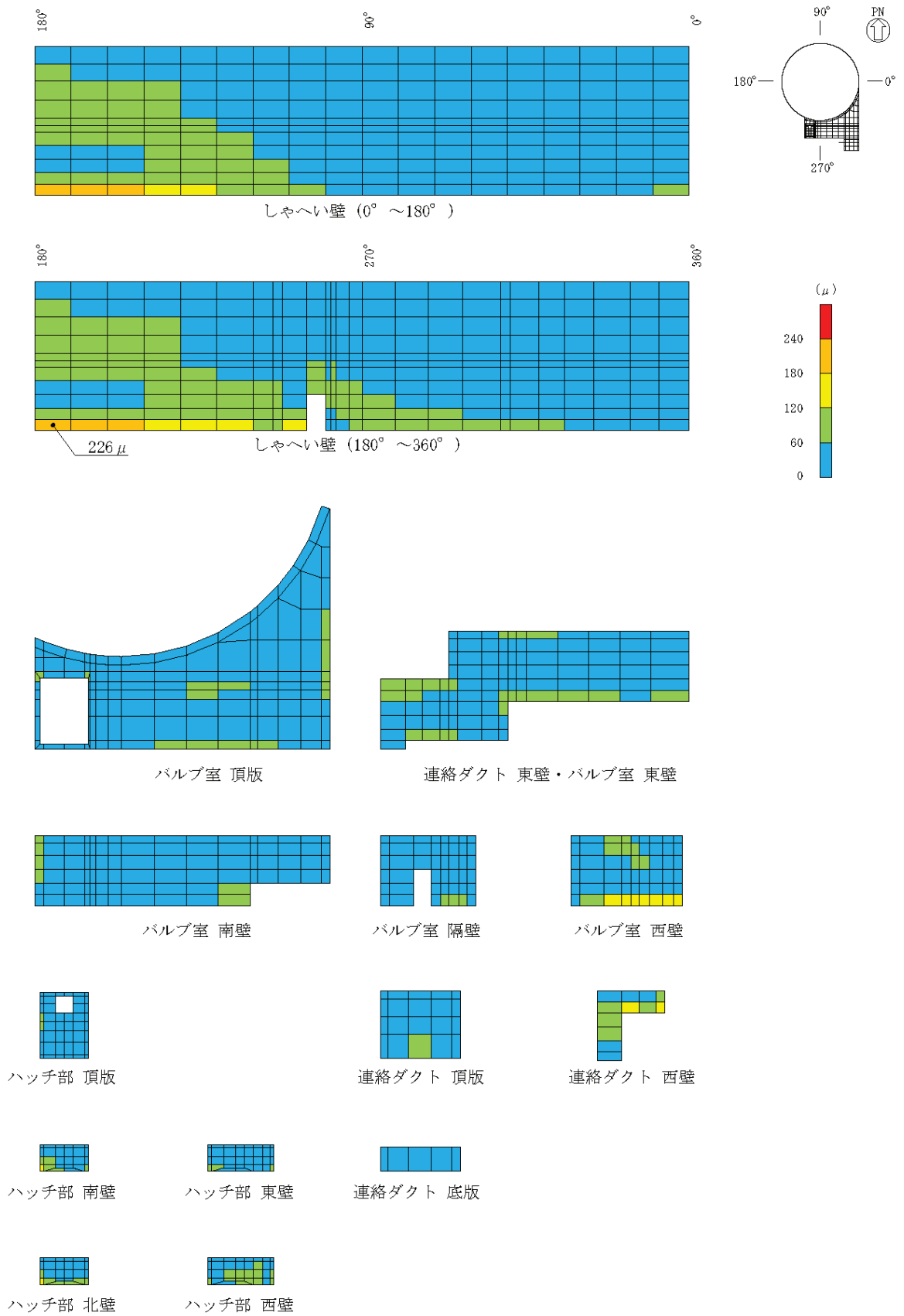
図 6-12 曲げ・軸力系の破壊に対する照査値最大時のひずみ分布図 (コンクリート) (しやへい壁 (地中部), 解析ケース①, S s - D 2 (-+), t=25.11s, 東西)
