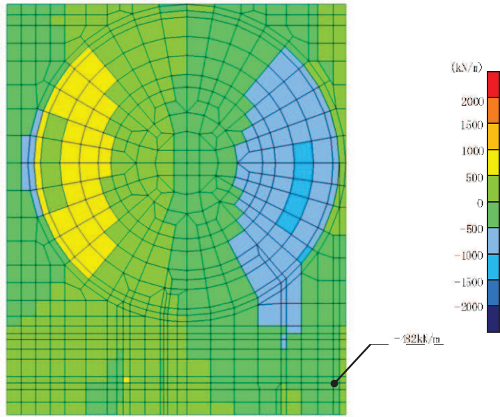
図 6-16(5) 曲げ・軸力系の破壊に対する照査値最大時の断面力分布図 (面内せん断力 (ken/m) : N_{x,y} ) (解析ケース②, S_s - D 2 (++) , t=6.86s , 南北)
