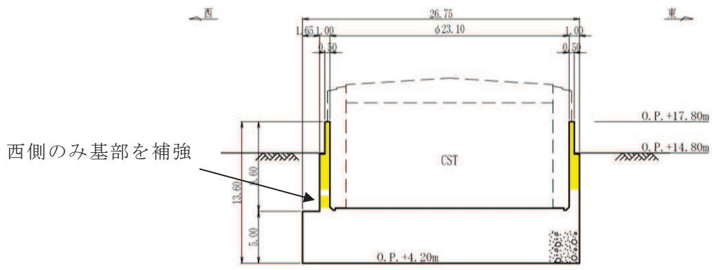
図 3-2(3) CCb による耐震補強箇所 (B-B 断面)
