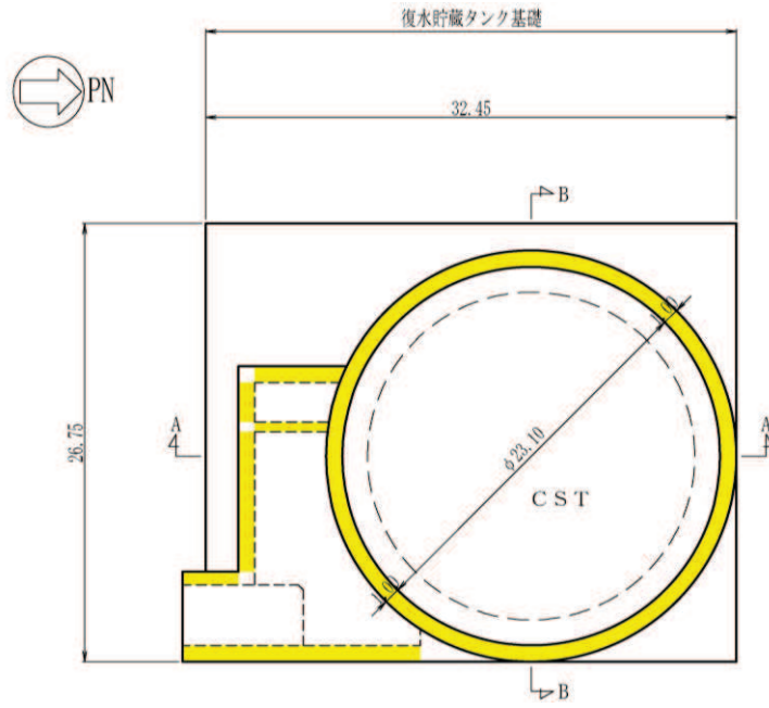
図 3-2(1) CCb による耐震補強箇所 (平面図)
