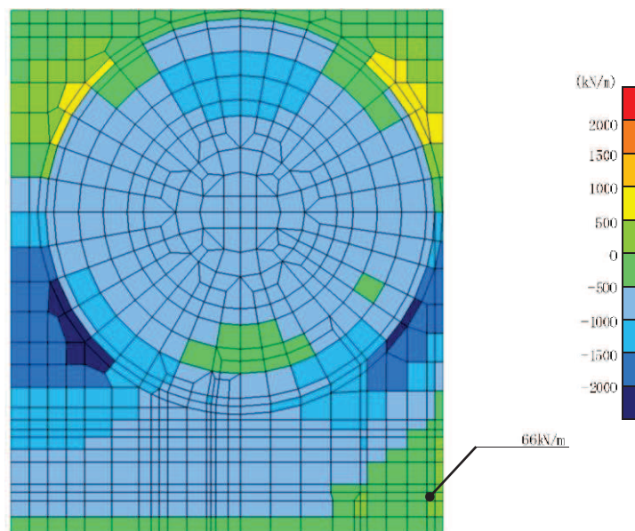
図 6-16(4) 曲げ・軸力系の破壊に対する照査値最大時の断面力分布図 (軸力 (ken/m) : N_y ) (解析ケース②, S_s - D 2 (++) , t=6.86s , 南北)
