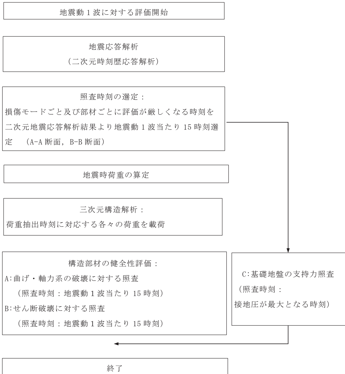
図 2-1 耐震評価フロー（基本フロー（地震動 1 波に対する評価フロー））
