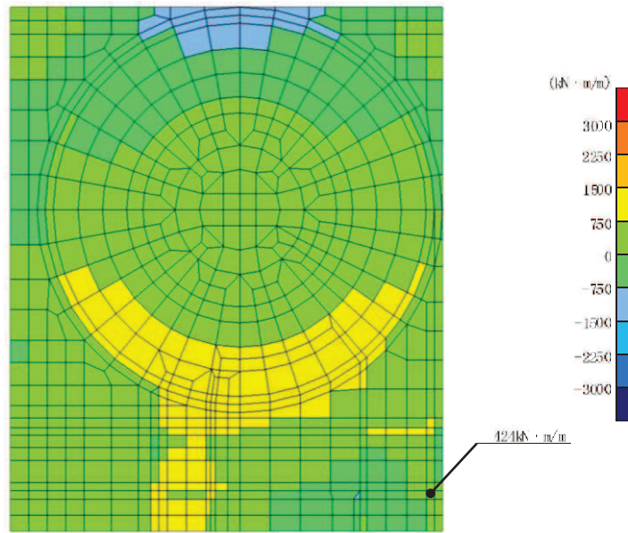
図 6-16(1) 曲げ・軸力系の破壊に対する照査値最大時の断面力分布図 (曲げモーメント (ken · m/m) : M_x ) (解析ケース②, S s - D 2 (++) , t=6.86s, 南北)
