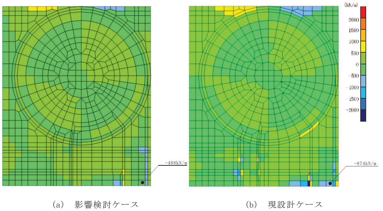
図 3-4(6) 基礎版の断面力分布図 (せん断力 (kN/m) : Q_x )
