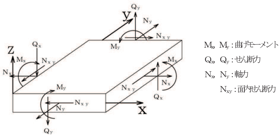
図 6-8 シェル要素における断面力の方向
