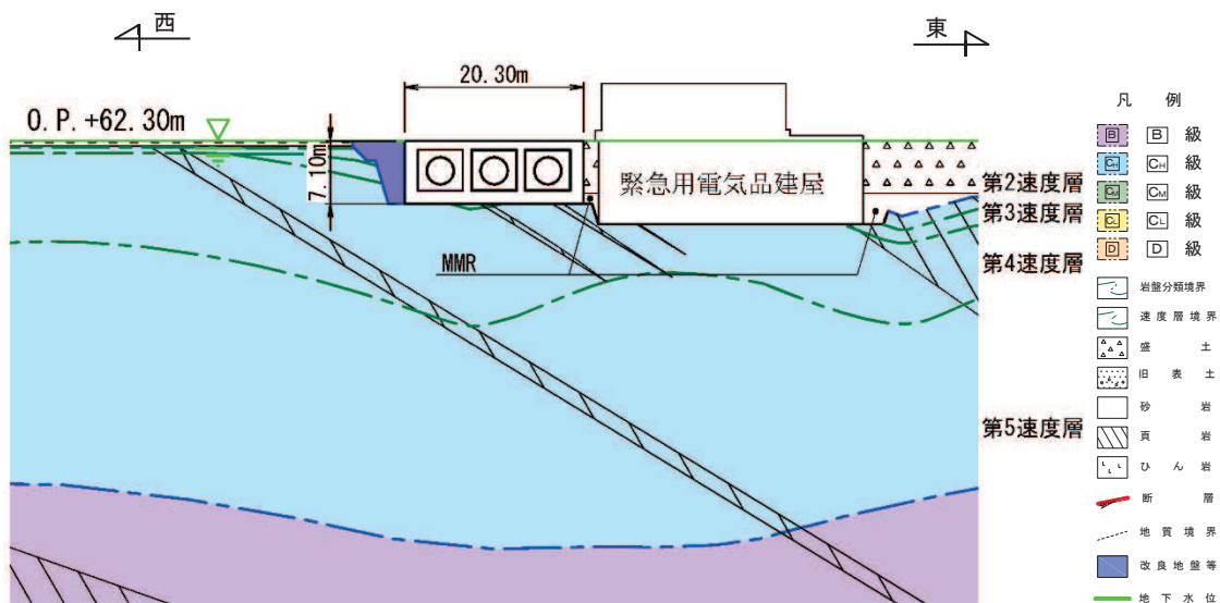
図 2-8 (2) ガスタービン発電設備軽油タンク室 地震時荷重算出用地質断面図 (B-B 断面, 東西)
