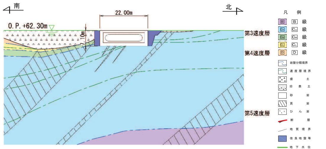
図 2-10(1) 設計用地下水位 (A-A 断面, 南北)
