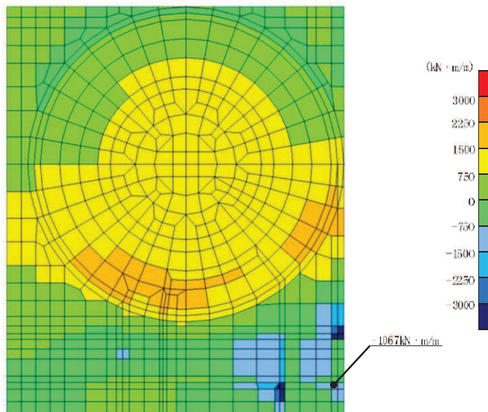
図 6-16(2) 曲げ・軸力系の破壊に対する照査値最大時の断面力分布図 (曲げモーメント (ken · m/m) : M_y ) (解析ケース②, S s - D 2 (++) , t=6.86s, 南北)
