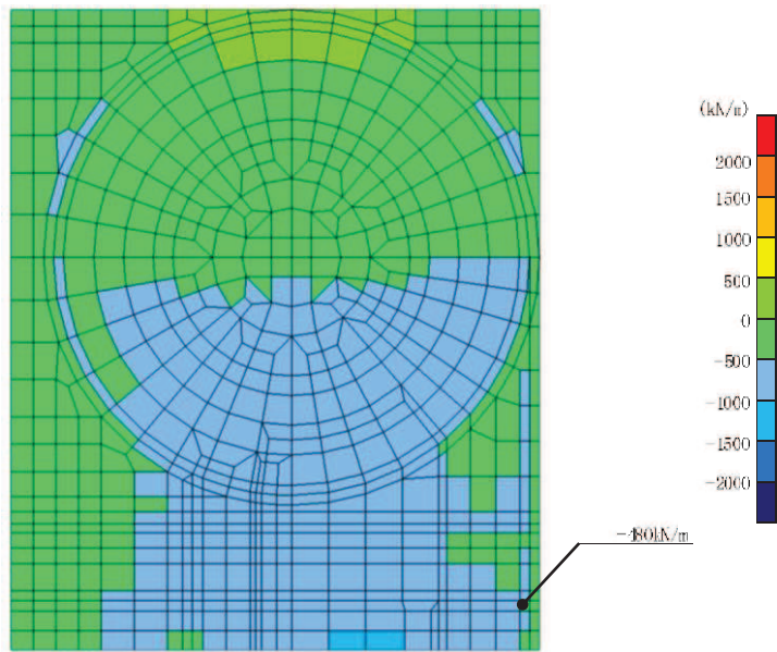
図 6-16(3) 曲げ・軸力系の破壊に対する照査値最大時の断面力分布図 (軸力 (ken/m) : N_x ) (解析ケース②, S_s - D 2 (++) , t=6.86s , 南北)
