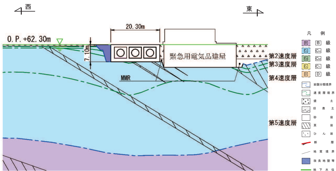
図 2-10(2) 設計用地下水位 (B-B 断面, 東西)
