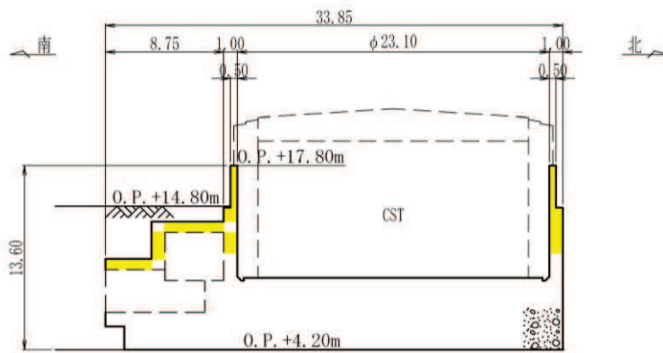
図 3-2(2) CCb による耐震補強箇所 (A-A 断面)
