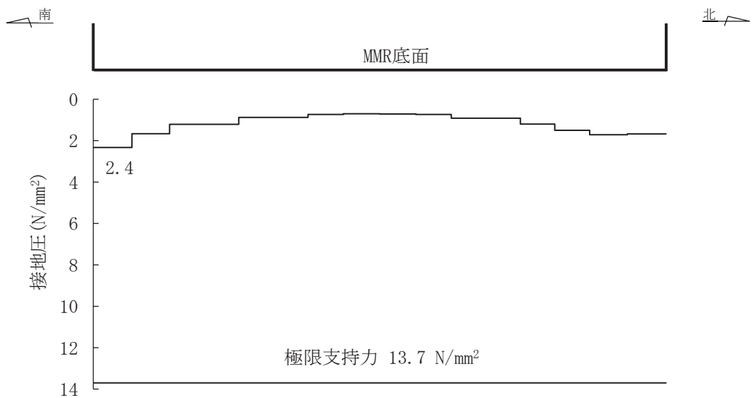
図 6-48(2) 基礎地盤の最大接地圧分布図（断面③）（有効応力解析） （解析ケース⑨', S s -F3 (++)）
