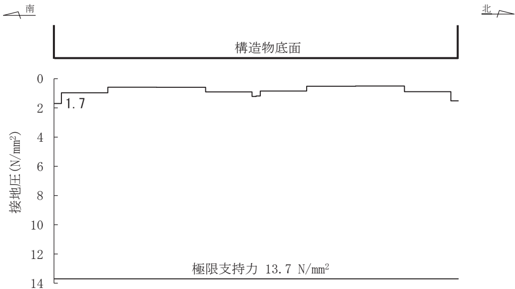
図 6-52(2) 基礎地盤の最大接地圧分布図（断面⑦）（有効応力解析） （解析ケース⑥'，S s -D1（-+））
