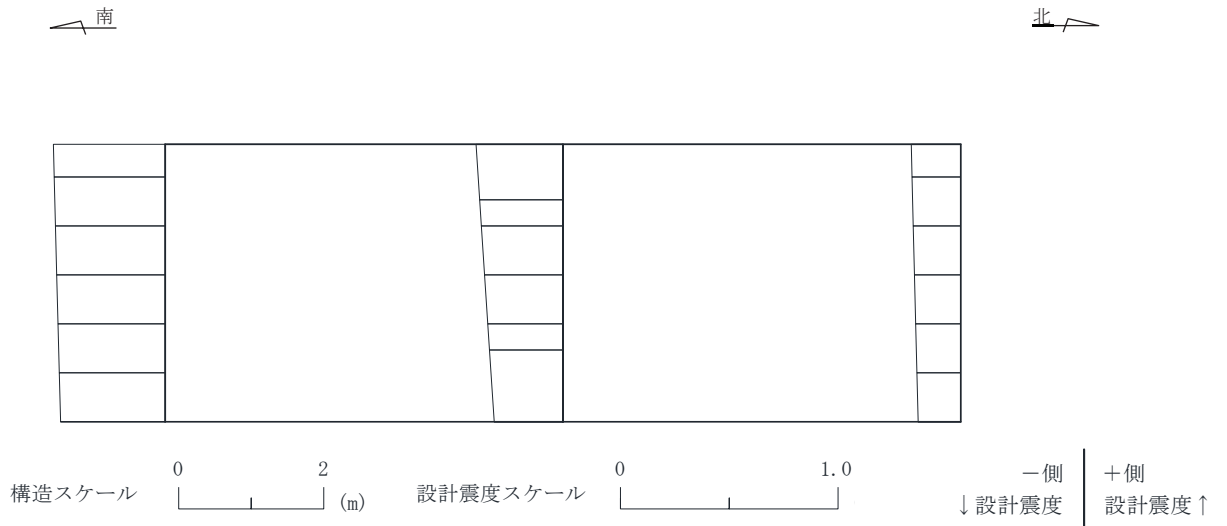
図 6-2(2) 作用荷重分布図 (設計震度分布) (全応力解析) (断面③ : 直線部, 解析ケース③, S_s - N1 (++) )
