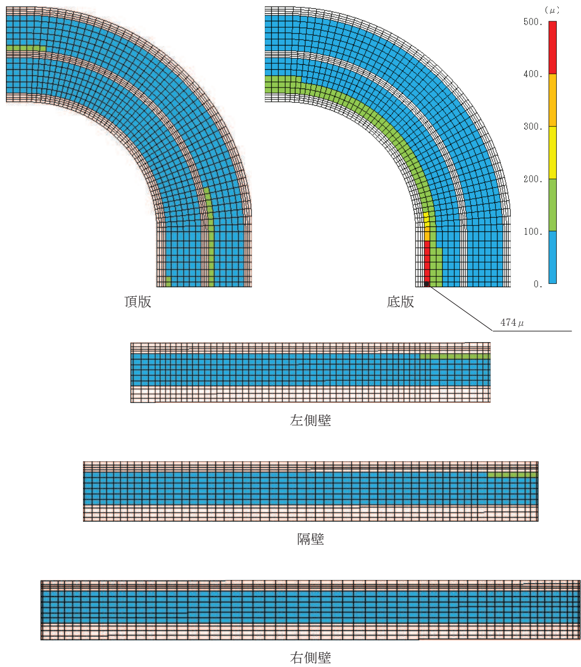
図 6-32(2) 曲げ・軸力系の破壊に対する照査値最大時のひずみ分布図 (鉄筋 : 有効応力解析) (曲線部, 底版, 解析ケース⑧', S_s - N1 (-+) )
