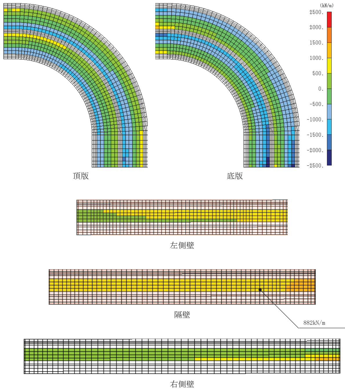
図 6-43(2) せん断破壊に対する照査値最大時の断面力分布図 (有効応力解析)
