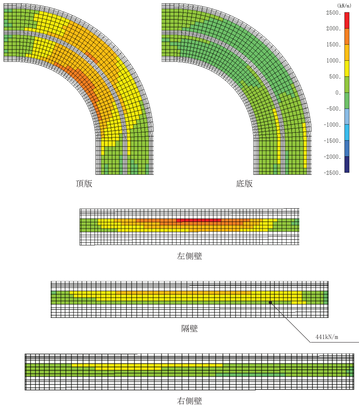
図 6-42(2) せん断破壊に対する照査値最大時の断面力分布図 (有効応力解析)
