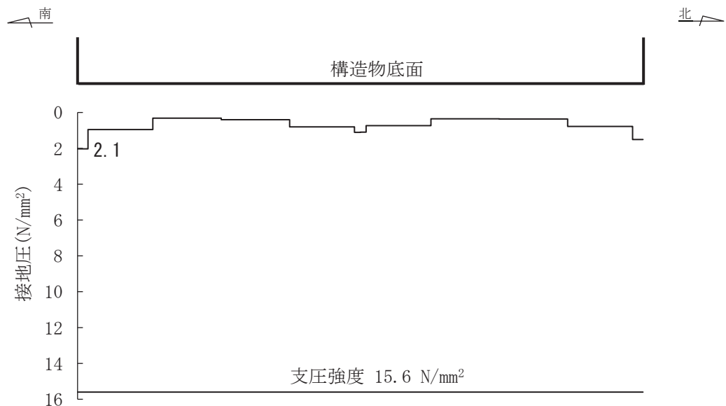
図 6-57(2) MMR (既設) の最大接地圧分布図 (断面⑥) (有効応力解析) (解析ケース⑧', S s -N1 (-+))
