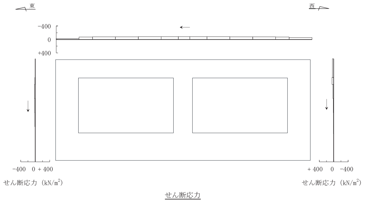
図 6-7(3) 作用荷重分布図 (直応力及びせん断応力) (有効応力解析)
