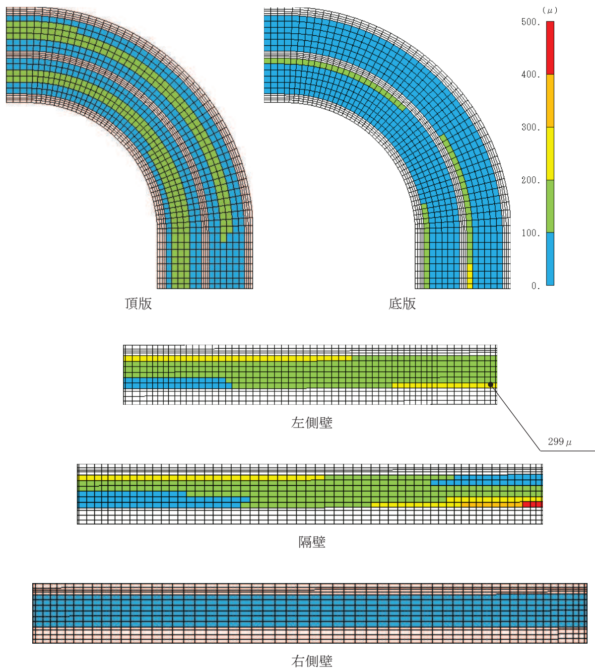
図 6-31(1) 曲げ・軸力系の破壊に対する照査値最大時のひずみ分布図 (コンクリートの圧縮ひずみ：全応力解析) (曲線部，隔壁，解析ケース③，S s - N 1 (++) )
