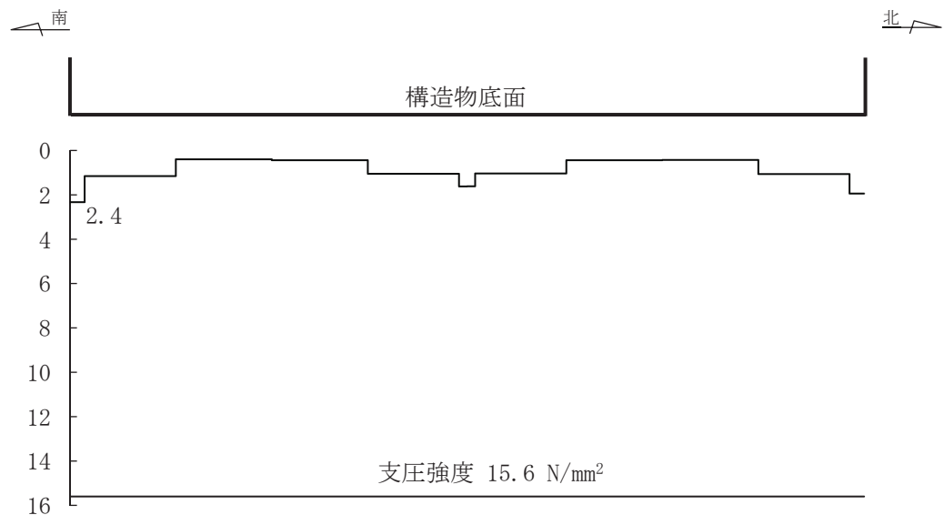
図 6-57(1) MMR (既設) の最大接地圧分布図 (断面⑥) (全応力解析) (解析ケース①, S s -D1 (++) )
