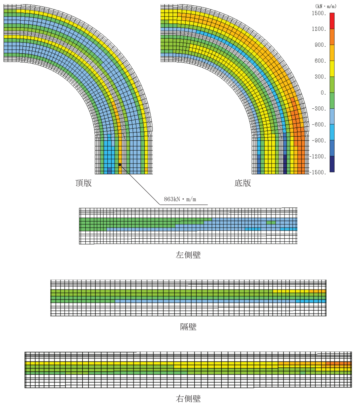
図 6-39(1) せん断破壊に対する照査値最大時の断面力分布図 (全応力解析)
