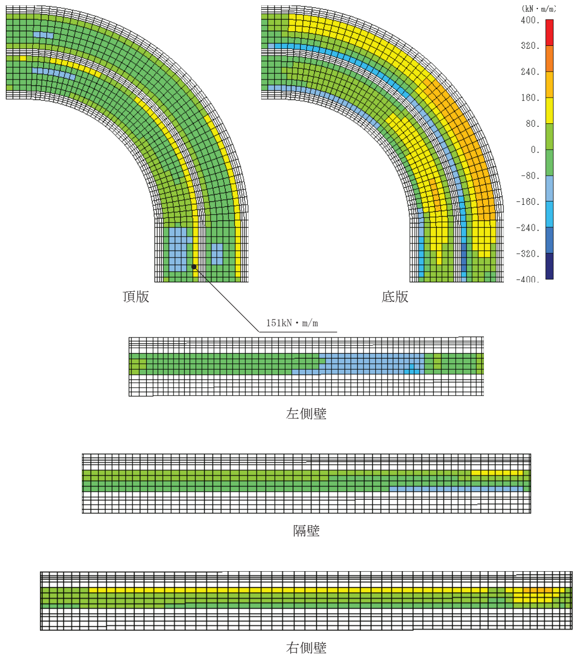
図 6-40(1) セン断破壊に対する照査値最大時の断面力分布図 (全応力解析) (曲げモーメント (kN · m/m) : M_y ) (曲線部, 頂版, 解析ケース③, S s - N 1 (++) )
