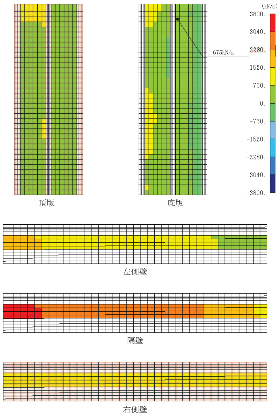
図 6-35(1) セン断破壊に対する照査値最大時の断面力分布図 (全応力解析)
