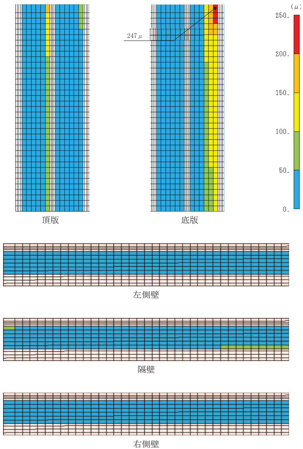
図 6-28(1) 曲げ・軸力系の破壊に対する照査値最大時のひずみ分布図 (鉄筋: 全応力解析) (直線部, 底板, 解析ケース③, S s - N 1 (++) )
