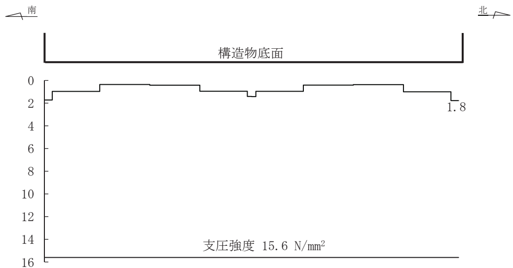
図 6-55(1) MMR (既設) の最大接地圧分布図 (断面④) (全応力解析) (解析ケース①, S s -D2 (++) )
