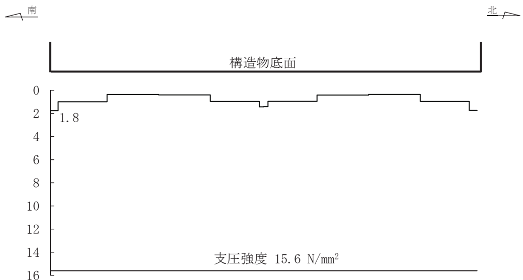
図 6-55(2) MMR (既設) の最大接地圧分布図 (断面④) (有効応力解析) (解析ケース①, S s -D2 (-+))
