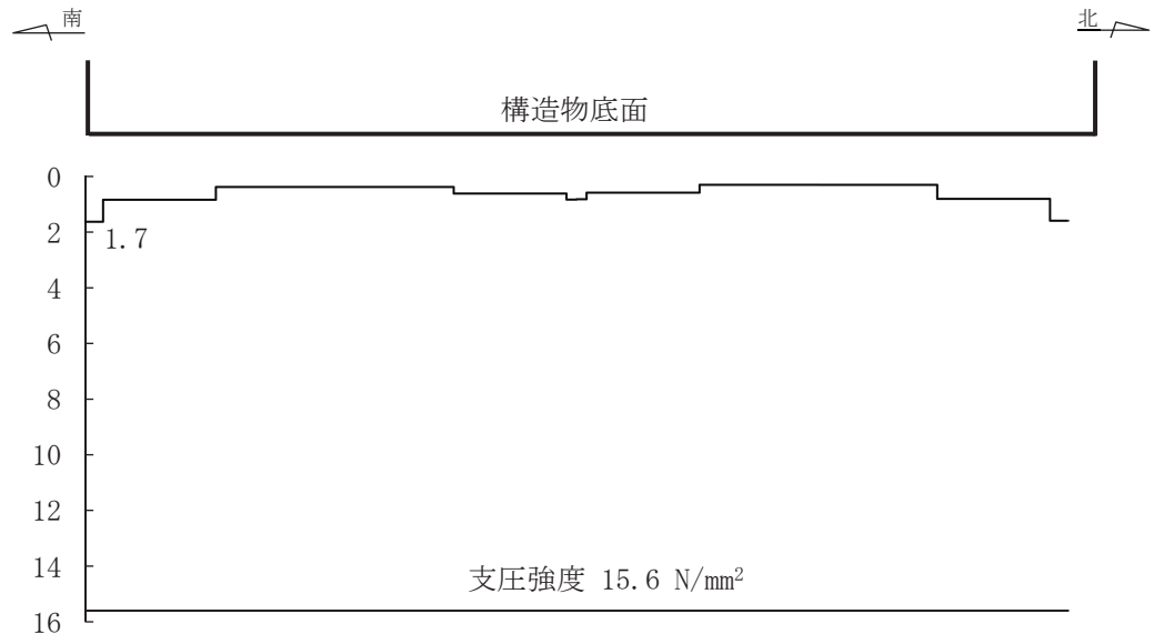
図 6-53(1) MMR (既設) の最大接地圧分布図 (断面②) (全応力解析) (解析ケース①, S s -D2 (-+))
