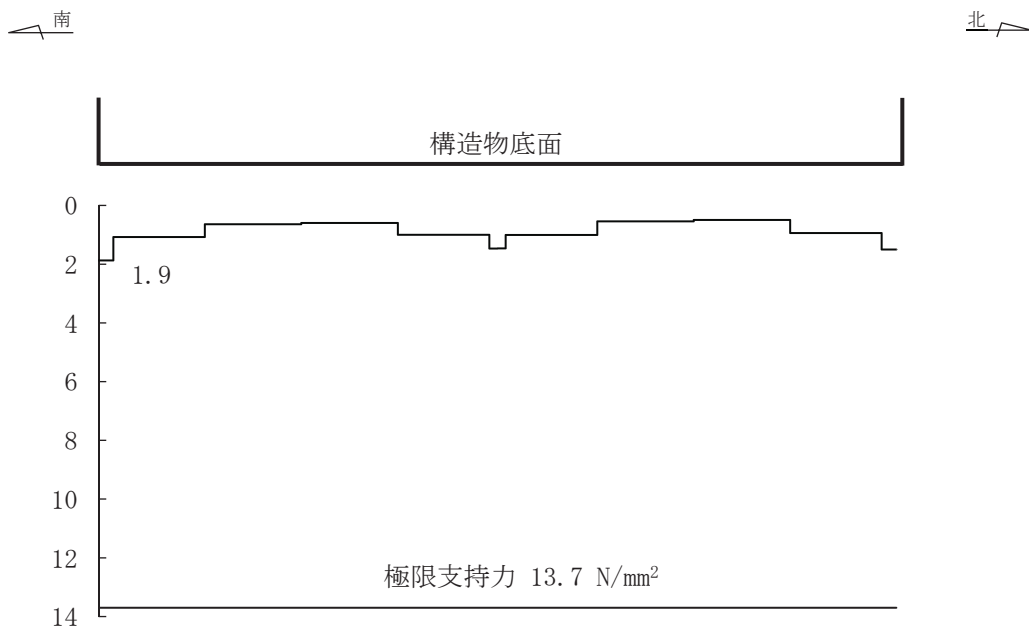
図 6-52(1) 基礎地盤の最大接地圧分布図（断面⑦）（有効応力解析） （解析ケース①，S s -D2（++））
