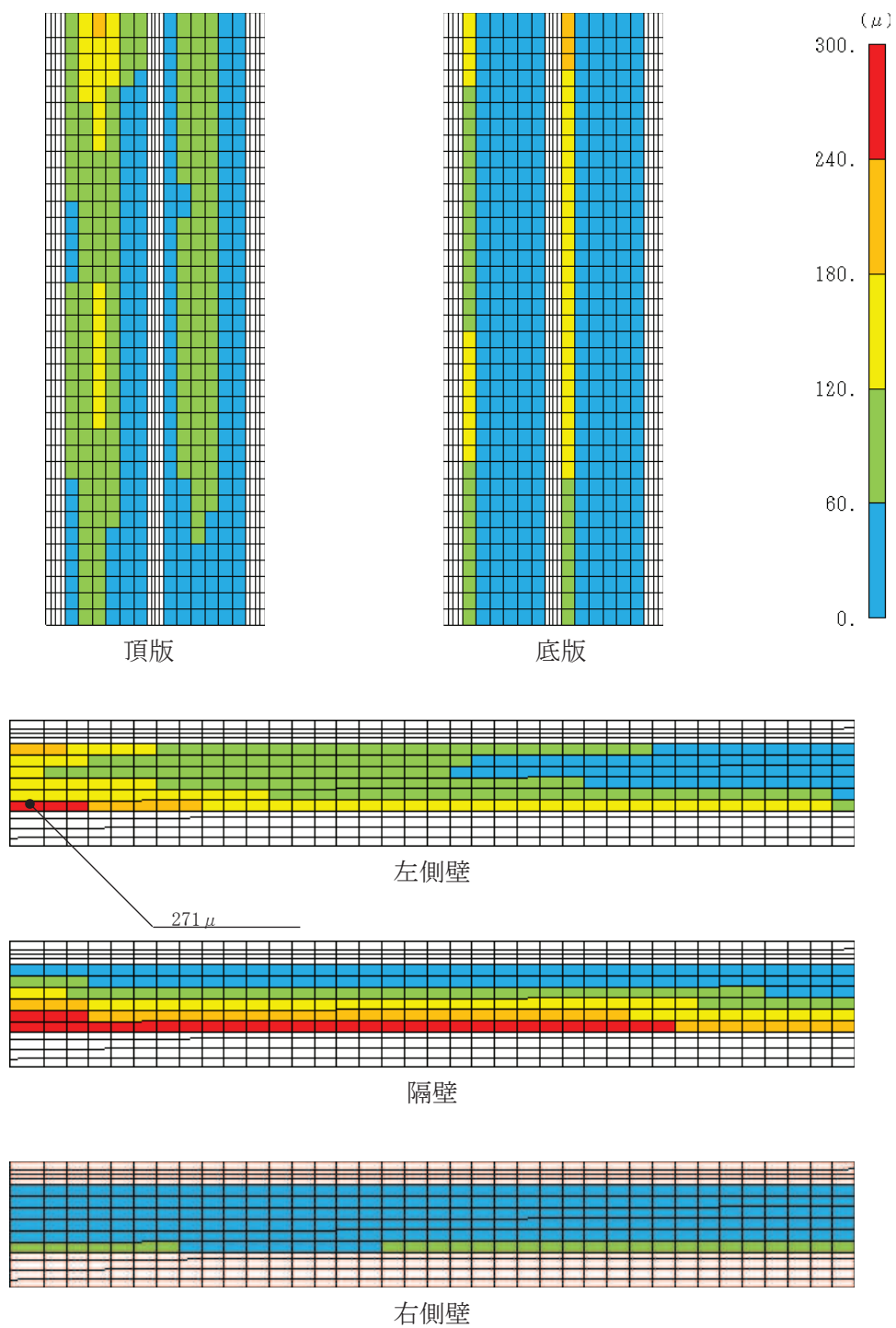
図 6-27(1) 曲げ・軸力系の破壊に対する照査値最大時のひずみ分布図 (コンクリートの圧縮ひずみ：全応力解析) (直線部，左側壁，解析ケース③， S_s - N1 (++) )
