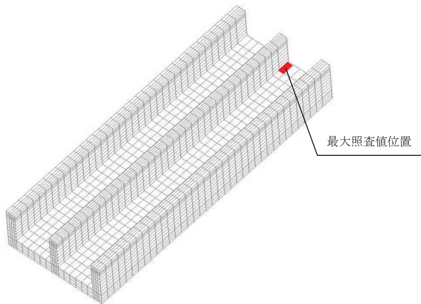
図 6-24 Ccb 工法適用部材におけるせん断破壊に対する最大照査値位置図 (直線部)
