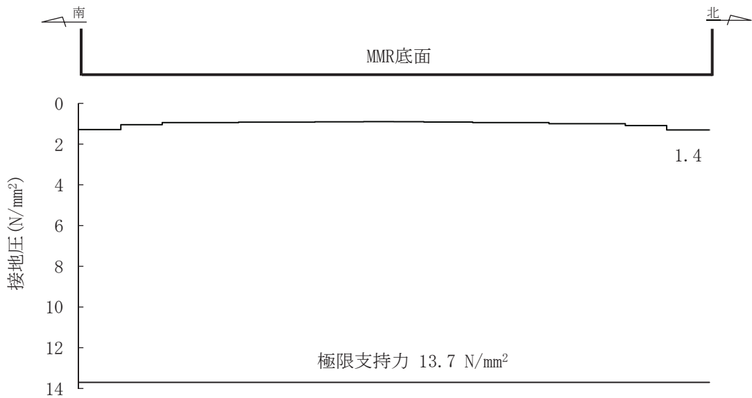
図 6-49(1) 基礎地盤の最大接地圧分布図（断面④）（全応力解析） （解析ケース①，S s -D2（-+））
