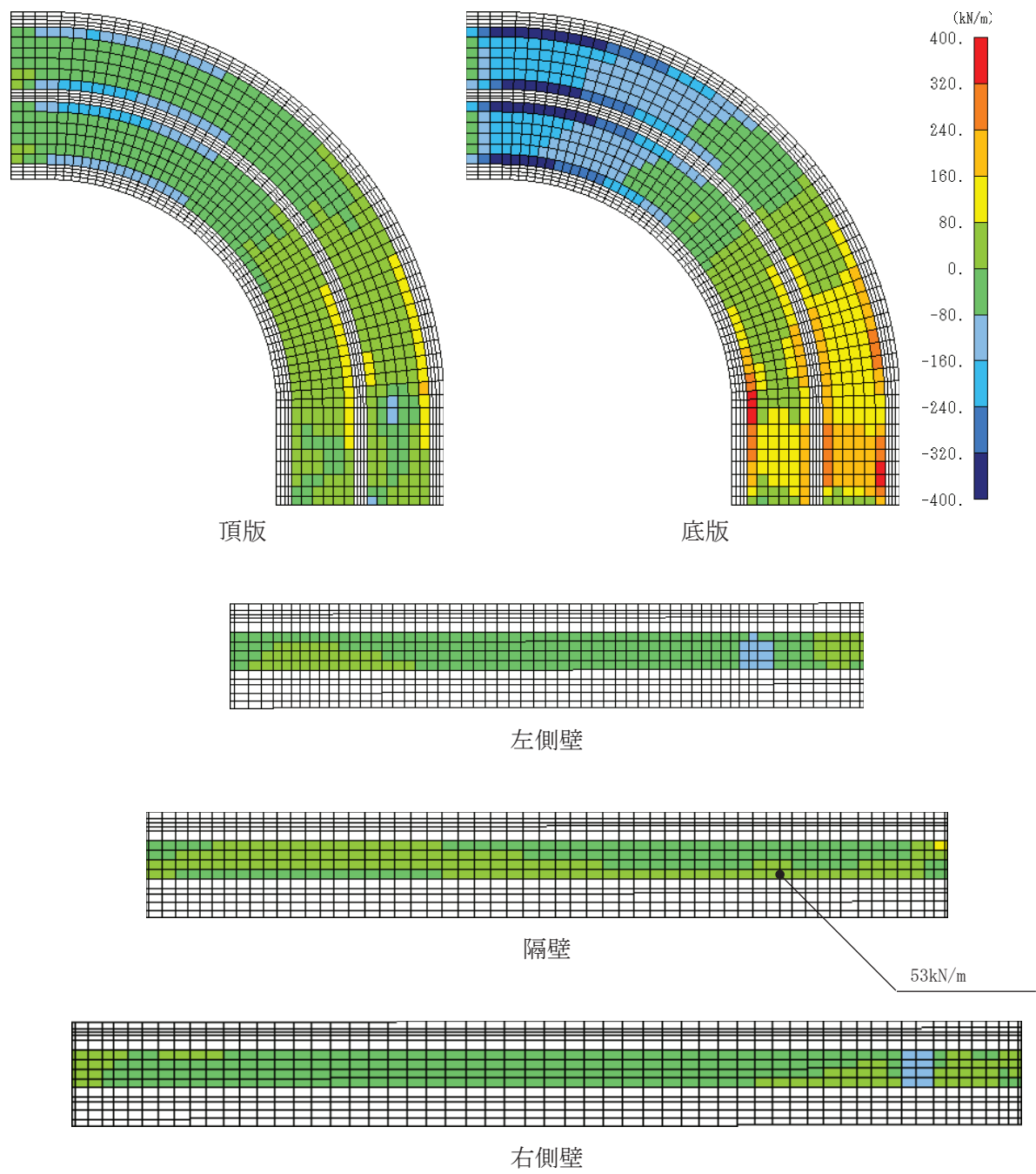
図 6-44(2) せん断破壊に対する照査値最大時の断面力分布図 (有効応力解析) (せん断力 (kN/m) : Q_y ) (曲線部, 隔壁, 解析ケース③, S_s - N1 (-+))
