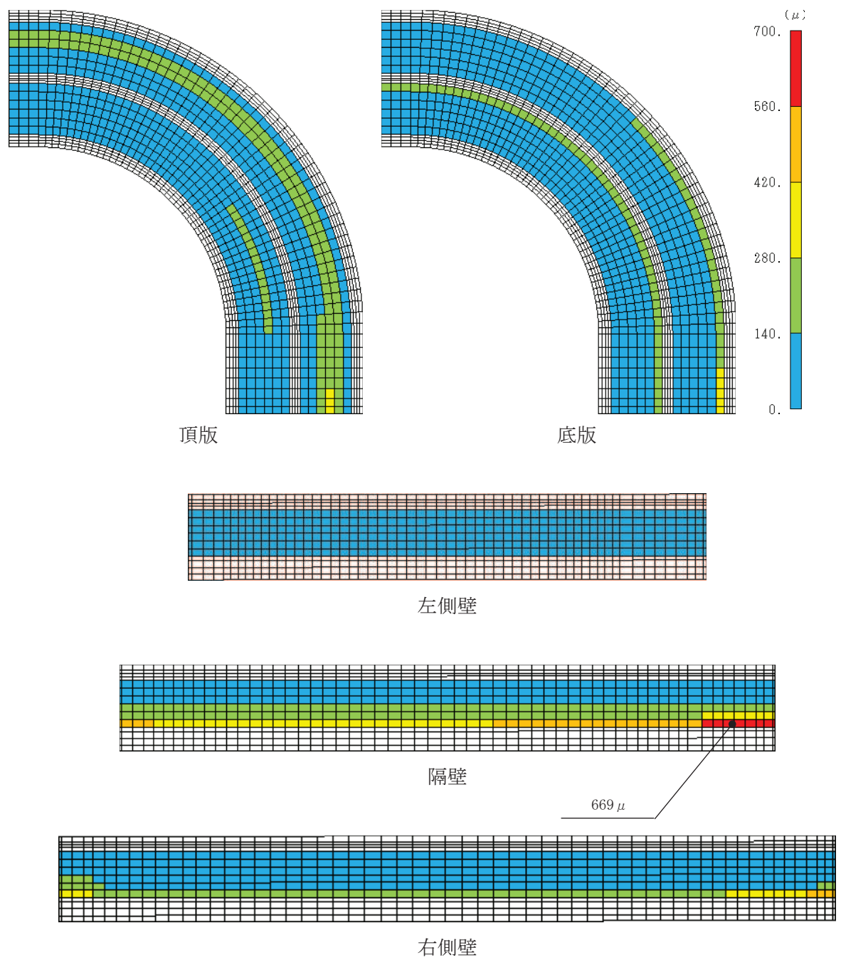
図 6-30(2) 曲げ・軸力系の破壊に対する照査値最大時のひずみ分布図 (コンクリートの圧縮縁ひずみ：有効応力解析) (曲線部，隔壁，解析ケース⑧'， S_s - N1 (-+) )
