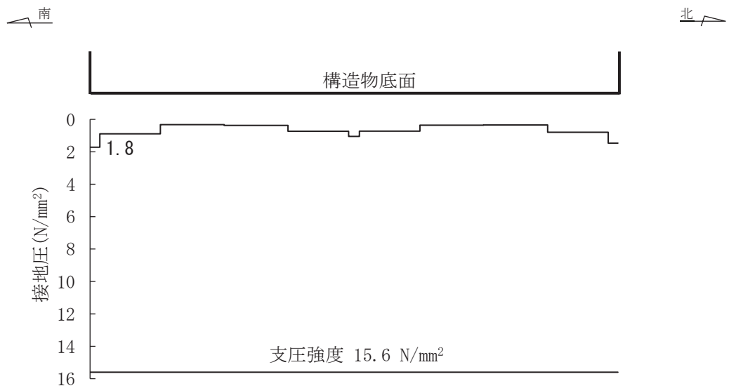
図 6-54(2) MMR (既設) の最大接地圧分布図 (断面③) (有効応力解析) (解析ケース⑥', S s -D2 (++))
