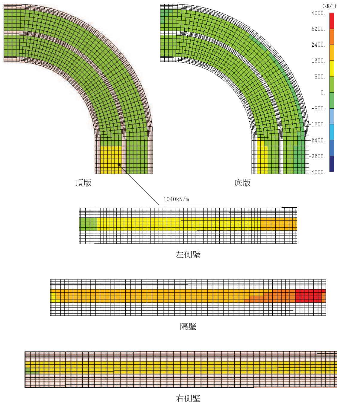
図 6-41(1) せん断破壊に対する照査値最大時の断面力分布図 (全応力解析)
