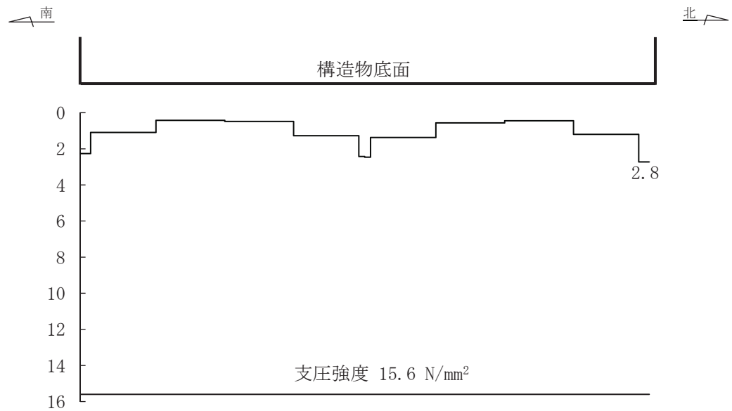
図 6-56(2) MMR (既設) 最大接地圧分布図 (断面⑤) (有効応力解析) (解析ケース③, S s -N1 (-+))
