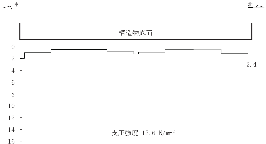
図 6-54(1) MMR (既設) の最大接地圧分布図 (断面③) (全応力解析) (解析ケース①, S s -D1 (-+))
