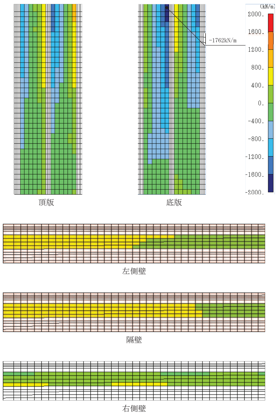
図 6-37(2) せん断破壊に対する照査値最大時の断面力分布図 (有効応力解析)
