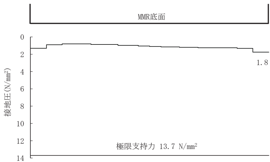
図 6-50(2) 基礎地盤の最大接地圧分布図（断面⑤）（有効応力解析） （解析ケース③，S s -N1（-+））
