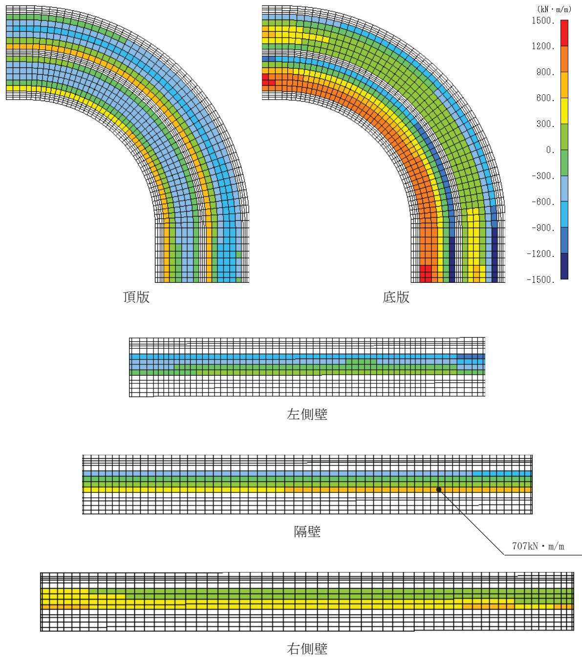
図 6-39(2) せん断破壊に対する照査値最大時の断面力分布図 (有効応力解析) (曲げモーメント (kN · m/m) : M_x ) (曲線部, 隔壁, 解析ケース③, S_s - N1 (-+))
