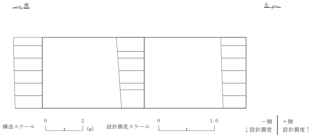
図 6-1(2) 作用荷重分布図 (設計震度分布) (全応力解析) (断面② : 直線部, 解析ケース③, S_s - N1 (++) )
