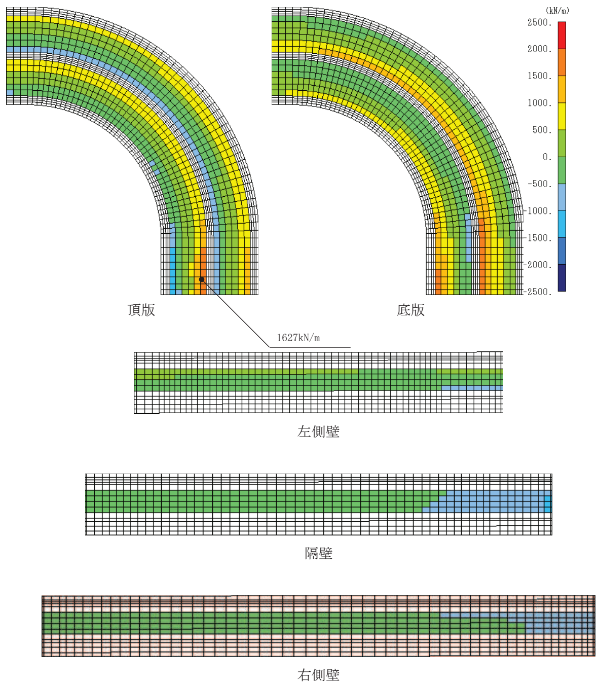
図 6-43(1) せん断破壊に対する照査値最大時の断面力分布図 (全応力解析)
