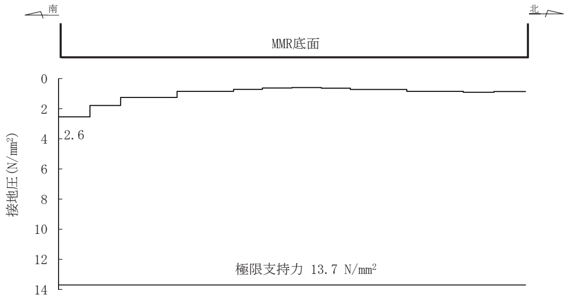
図 6-47(1) 基礎地盤の最大接地圧分布図（断面②）（全応力解析） （解析ケース①， S s -F2（++））
