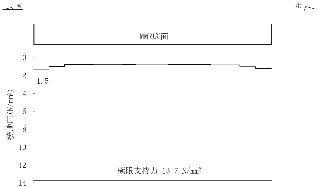
図 6-51(1) 基礎地盤の最大接地圧分布図（断面⑥）（全応力解析） （解析ケース①, S s -D2 (-+)）
