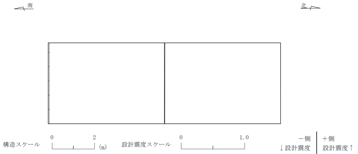
図 6-3(2) 作用荷重分布図 (設計震度分布) (全応力解析) (断面④ : 直線部, 解析ケース③, S_s - N1 (++) )
