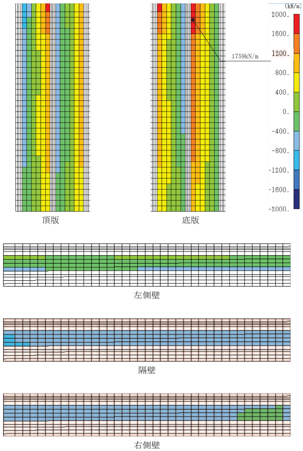
図 6-37(1) せん断破壊に対する照査値最大時の断面力分布図 (全応力解析) (せん断力 (kN/m) : Q_x ) (直線部, 底板, 解析ケース③, S_s - N1 (++) )
