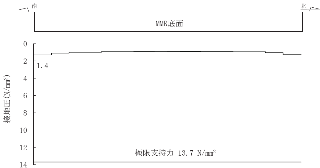
図 6-49(2) 基礎地盤の最大接地圧分布図（断面④）（有効応力解析） （解析ケース④，S s -F3（++））
