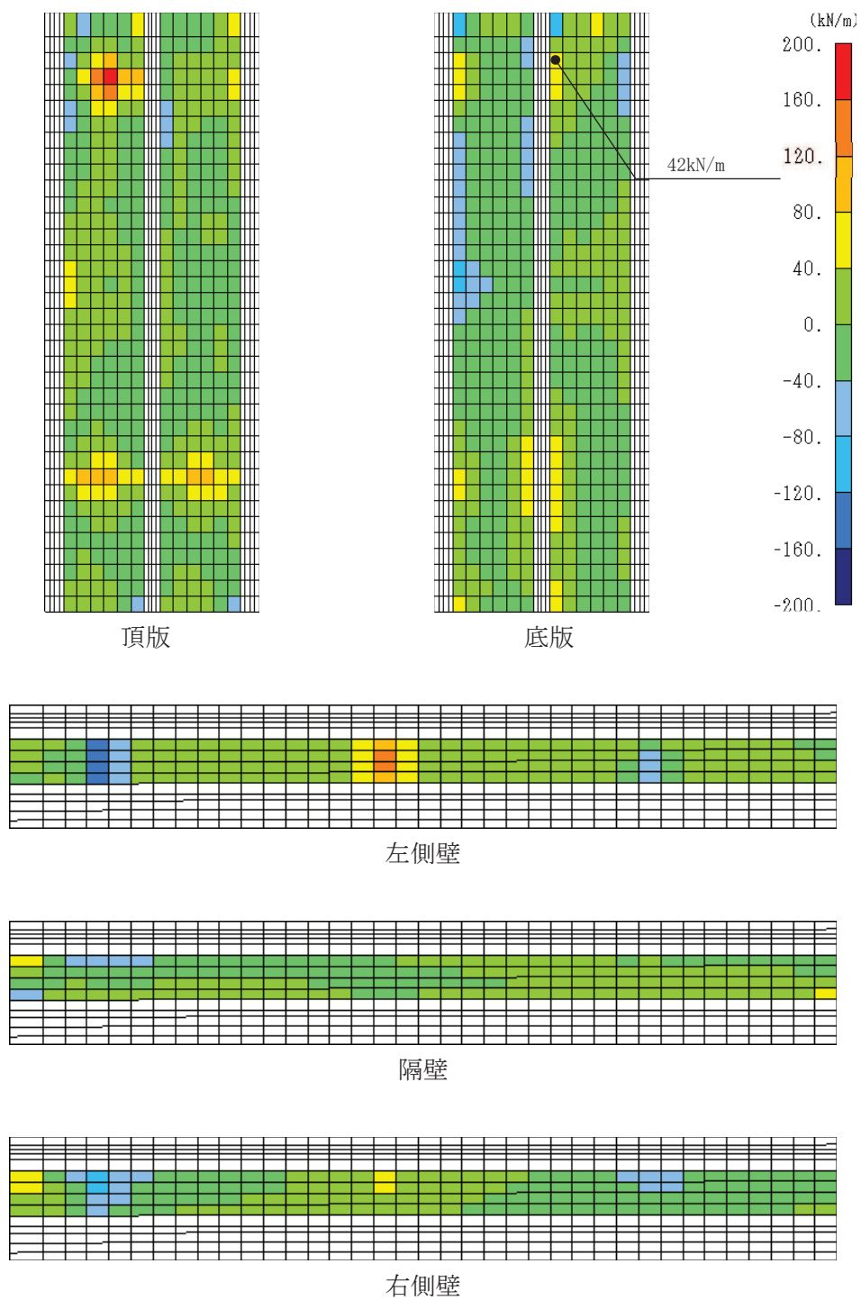
図 6-38(1) セン断破壊に対する照査値最大時の断面力分布図 (全応力解析) (せん断力 (kN/m) : Q_y ) (直線部, 底板, 解析ケース③, S_s - N1 (++) )
