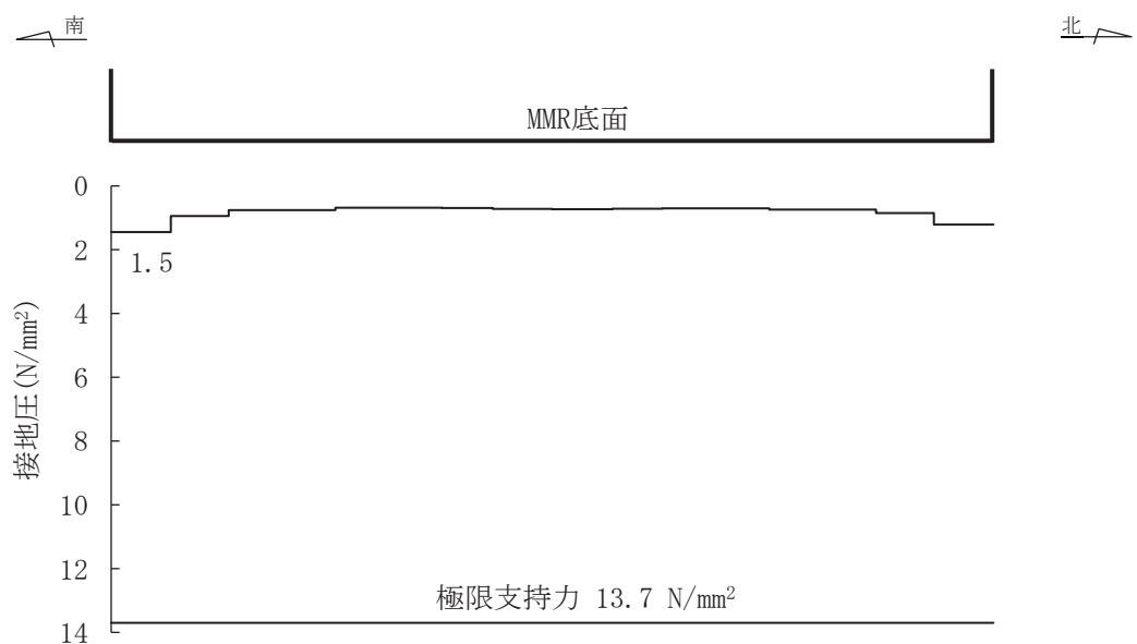
図 6-51 (2) 基礎地盤の最大接地圧分布図（断面⑥）（有効応力解析） （解析ケース⑥'， S s -F3（++））
