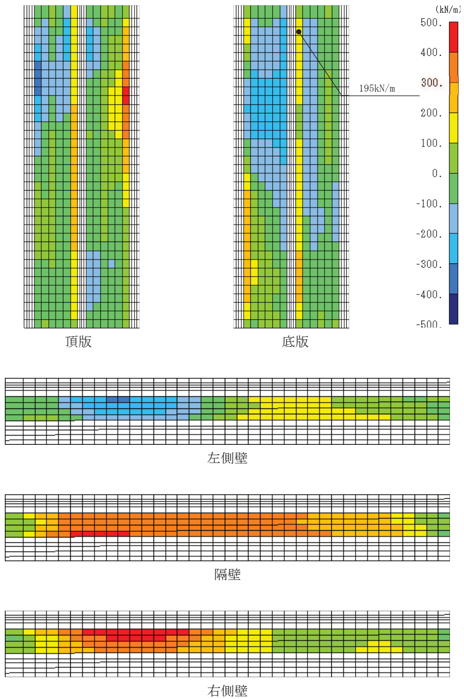
図 6-36(1) せん断破壊に対する照査値最大時の断面力分布図 (全応力解析) (軸力 (kN/m) : N_y ) (直線部, 底板, 解析ケース③, S_s - N1 (++) )
