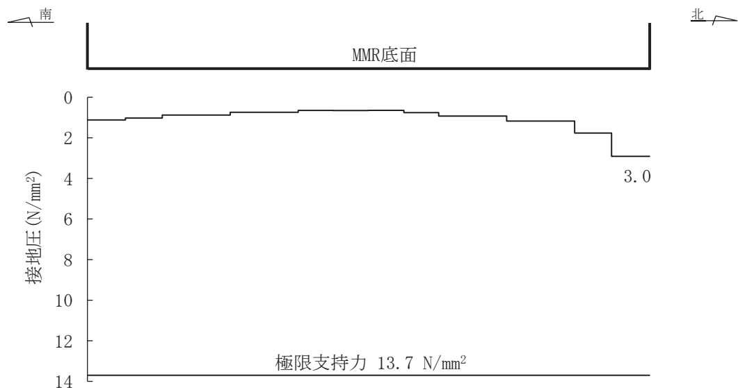
図 6-47(2) 基礎地盤の最大接地圧分布図（断面②）（有効応力解析） （解析ケース⑥'，S s -D1（-+））
