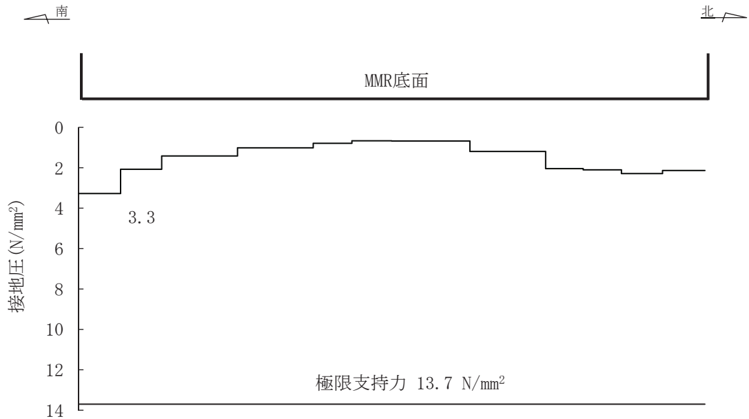
図 6-48(1) 基礎地盤の最大接地圧分布図（断面③）（全応力解析） （解析ケース①，S s -F1（-+））
