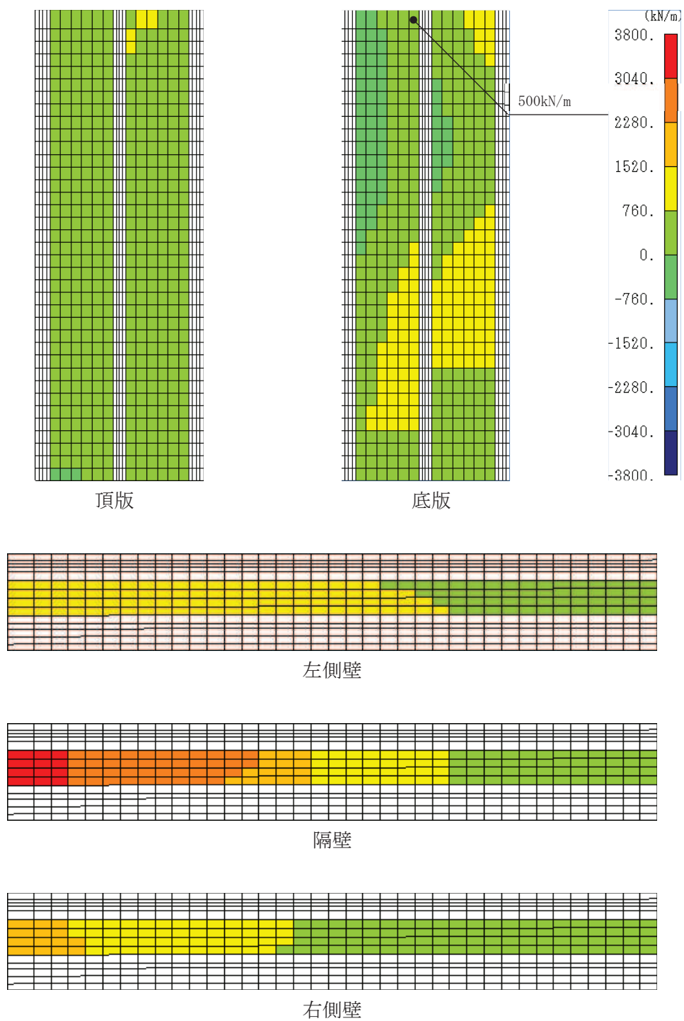
図 6-35(2) せん断破壊に対する照査値最大時の断面力分布図 (有効応力解析)
