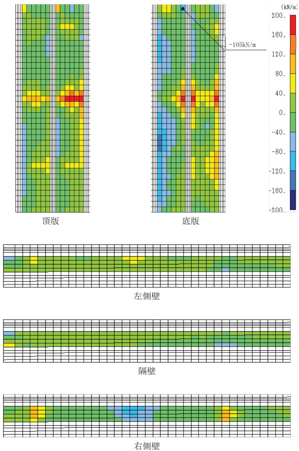
図 6-38(2) せん断破壊に対する照査値最大時の断面力分布図 (有効応力解析)
