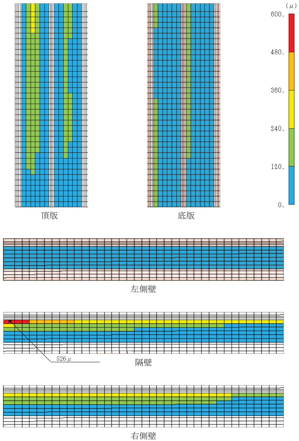
図 6-26(1) 曲げ・軸力系の破壊に対する照査値最大時のひずみ分布図* (コンクリートの圧縮縁ひずみ：全応力解析) (直線部，隔壁，解析ケース③， S_s - N1 (+ +) )
