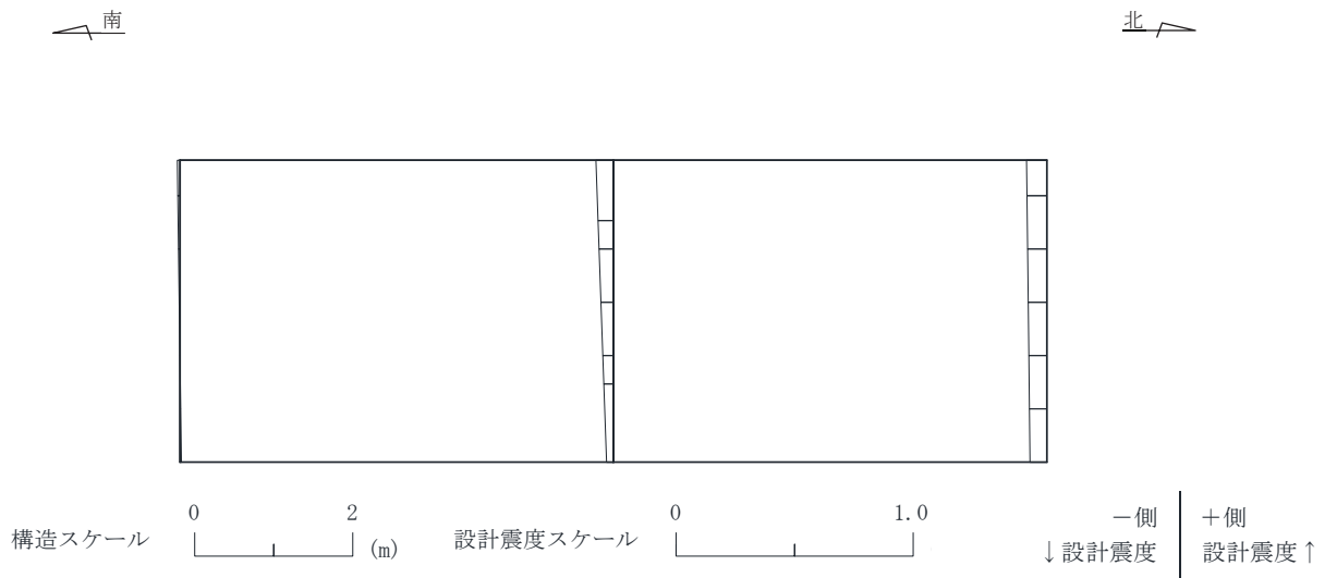
図 6-4(2) 作用荷重分布図 (設計震度分布) (全応力解析) (断面⑤ : 直線部, 解析ケース③, S_s - N1 (++) )
