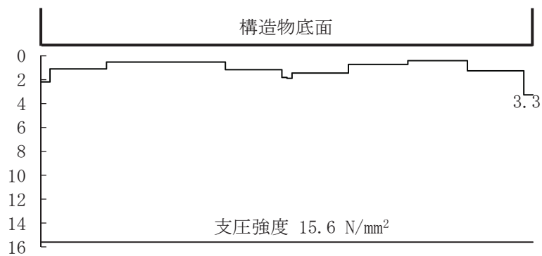
図 6-56(1) MMR (既設) 最大接地圧分布図 (断面⑤) (全応力解析) (解析ケース③, S s -N1 (++) )
