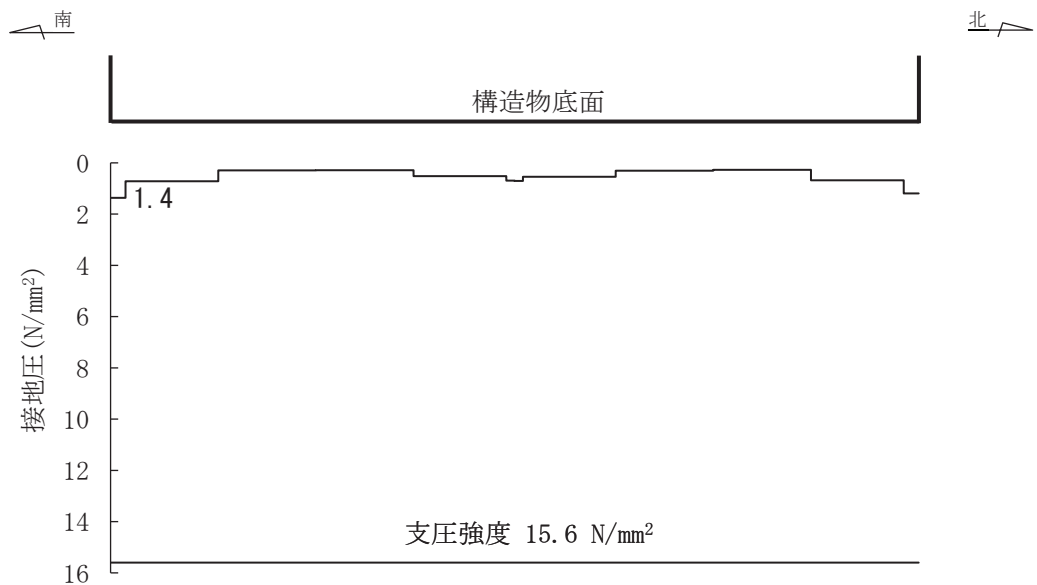
図 6-53(2) MMR (既設) の最大接地圧分布図 (断面②) (有効応力解析)
