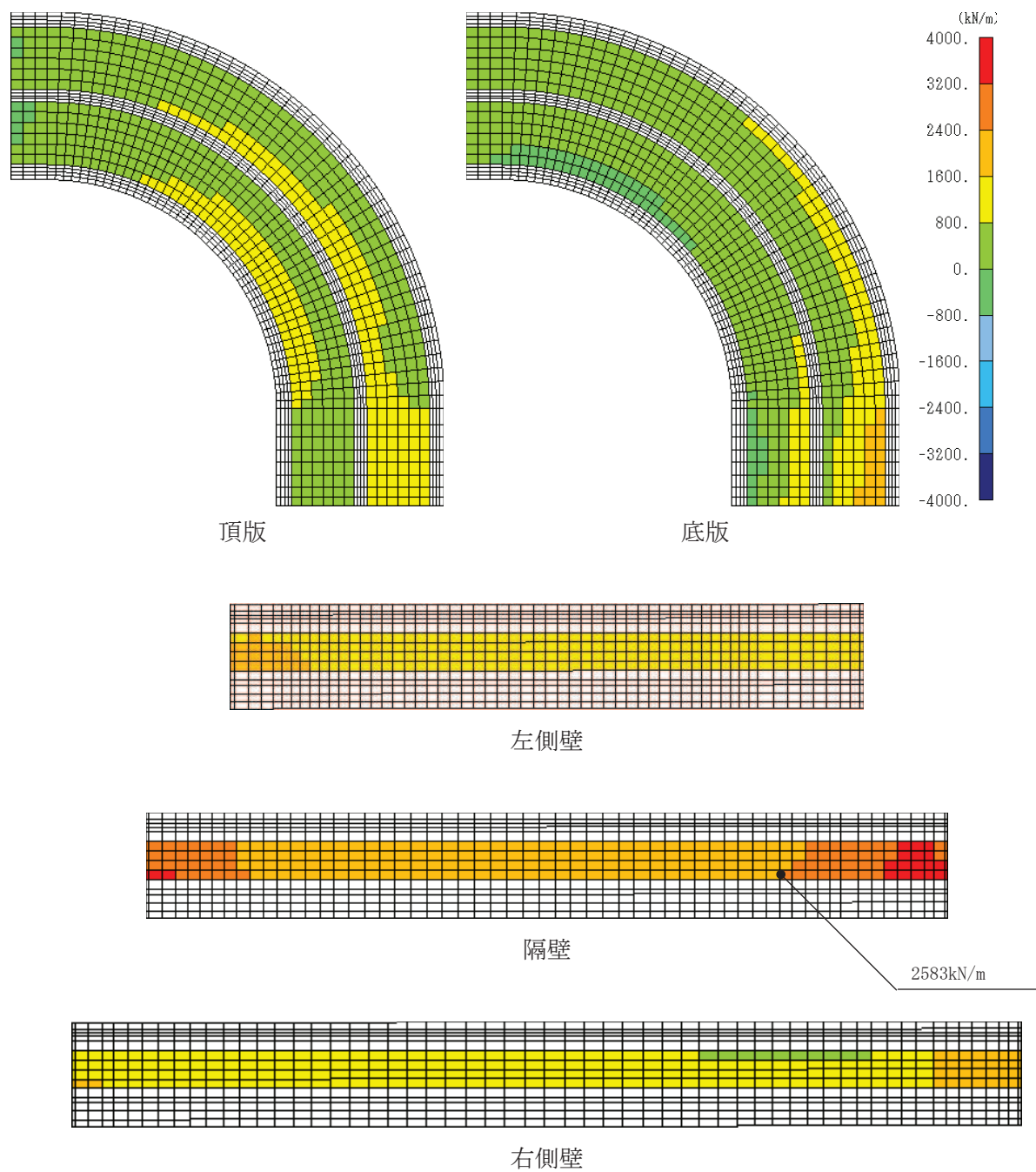
図 6-41(2) せん断破壊に対する照査値最大時の断面力分布図 (有効応力解析)
