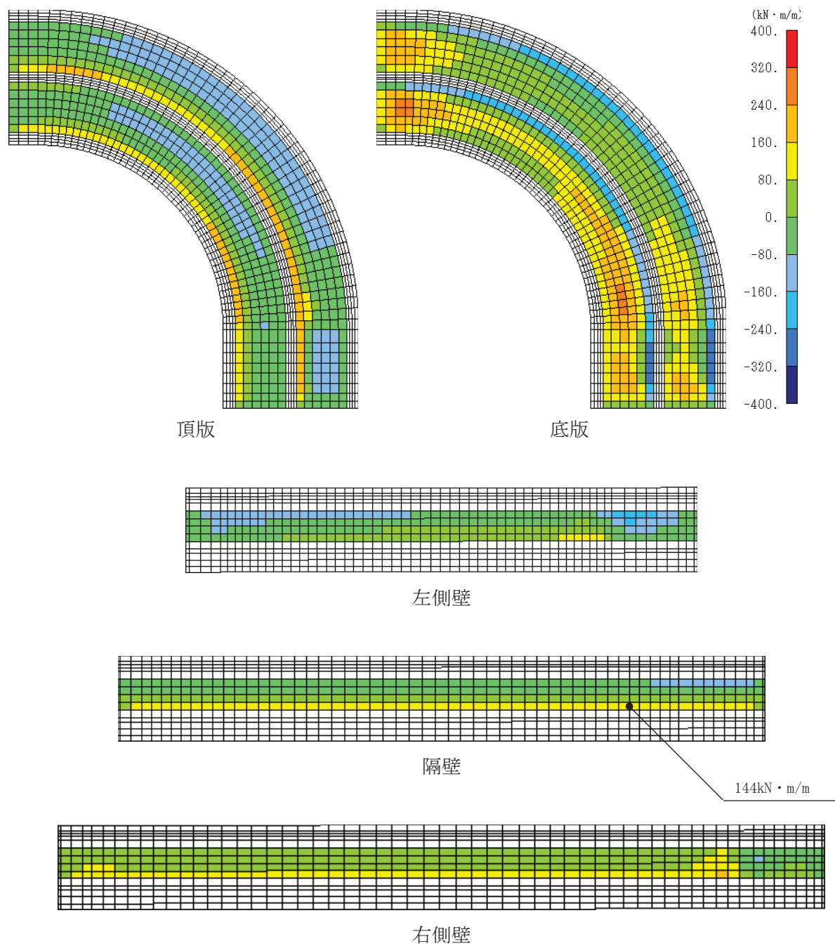
図 6-40(2) せん断破壊に対する照査値最大時の断面力分布図 (有効応力解析) (曲げモーメント (kN・m/m) : M_y ) (曲線部, 隔壁, 解析ケース③, S_s - N1 (一十))
