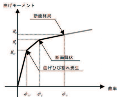
図3-21 鉄筋コンクリート部材のM- \phi 関係 (土木学会マニュアルより引用)
