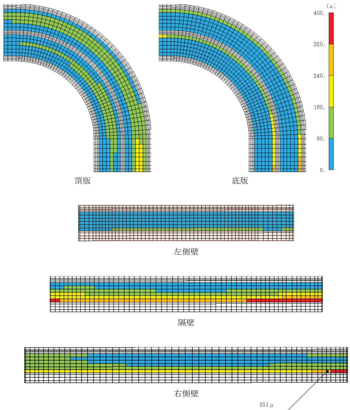
図 6-31(2) 曲げ・軸力系の破壊に対する照査値最大時のひずみ分布図 (コンクリートの圧縮ひずみ：有効応力解析) (曲線部，右側壁，解析ケース⑧'，S s - N 1 (-+))
