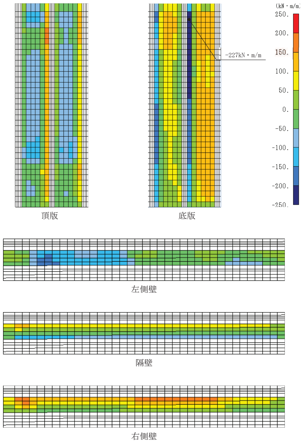
図 6-34(1) せん断破壊に対する照査値最大時の断面力分布図 (全応力解析) (曲げモーメント ( \text{kN} \cdot \text{m}/\text{m} ) : M_y ) (直線部, 底板, 解析ケース③, S_s - N1 (++) )
