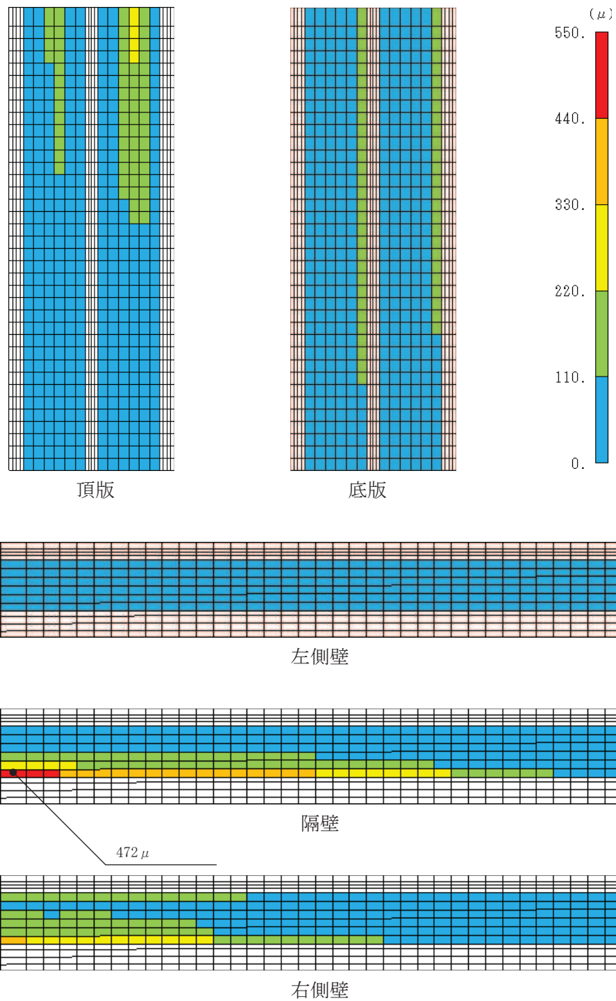
図 6-26(2) 曲げ・軸力系の破壊に対する照査値最大時のひずみ分布図* (コンクリートの圧縮縁ひずみ：有効応力解析) (直線部，隔壁，解析ケース⑧'， S_s - F3 (++) )
