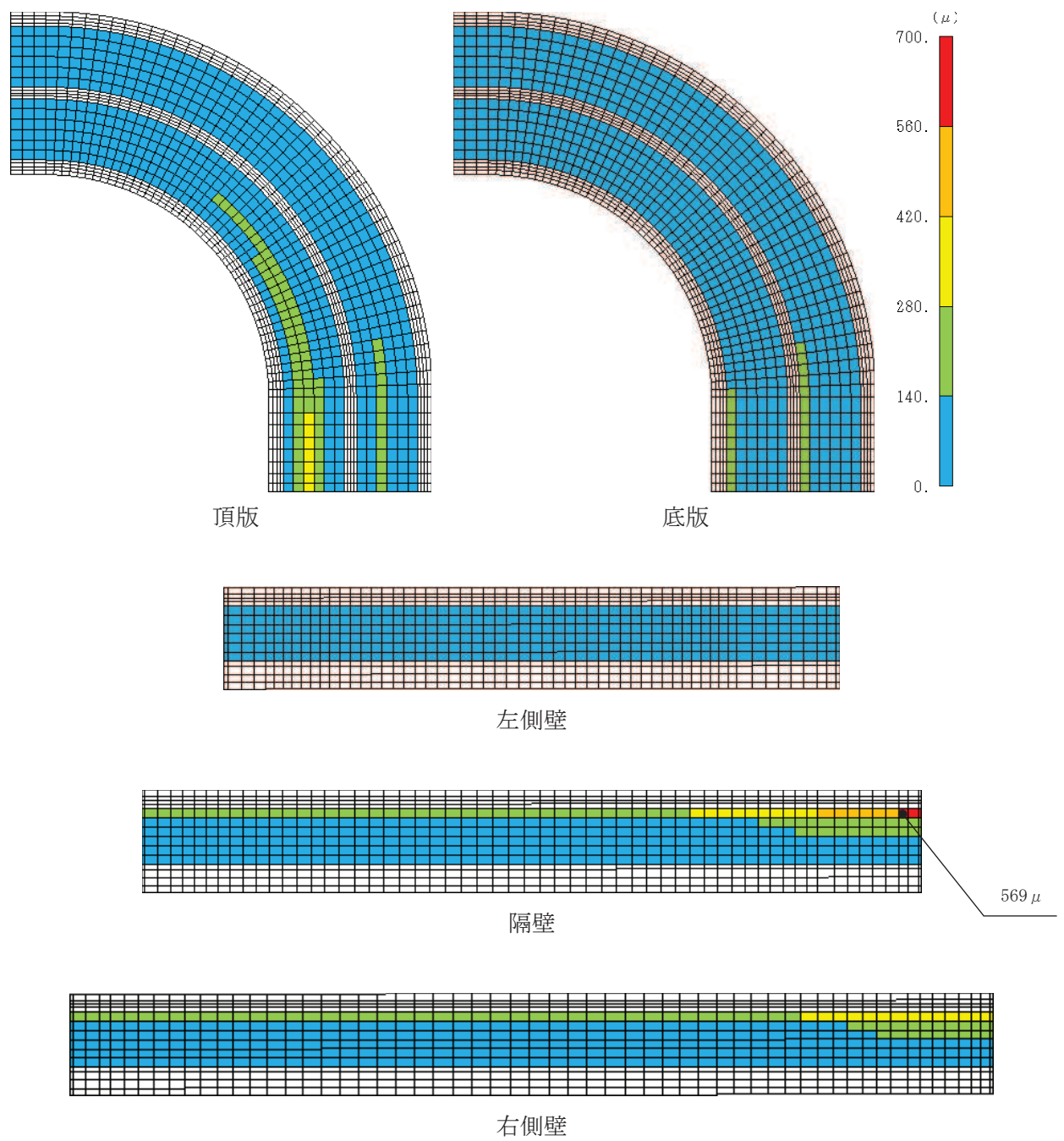
図 6-30(1) 曲げ・軸力系の破壊に対する照査値最大時のひずみ分布図 (コンクリートの圧縮縁ひずみ：全応力解析) (曲線部，隔壁，解析ケース③， S_s - N1 (++) )
