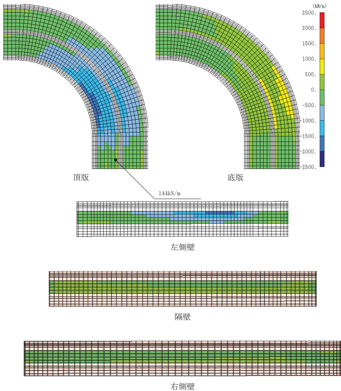
図 6-42 (1) せん断破壊に対する照査値最大時の断面力分布図 (全応力解析)
