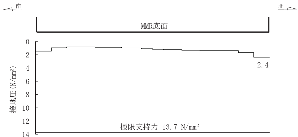
図 6-50(1) 基礎地盤の最大接地圧分布図（断面⑤）（全応力解析） （解析ケース③， S s -N1（++））
