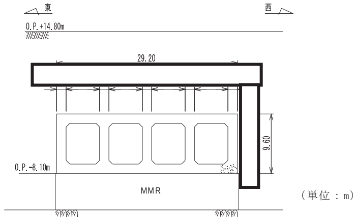
図 3-3-14 取水路（漸拡部）断面図（A-A）
