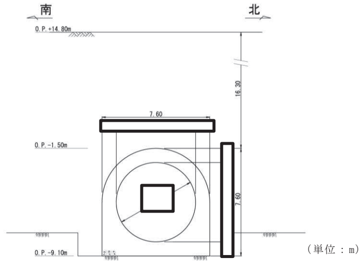
図 3-3-8 排気筒連絡ダクト断面図（土砂部，A-A）
