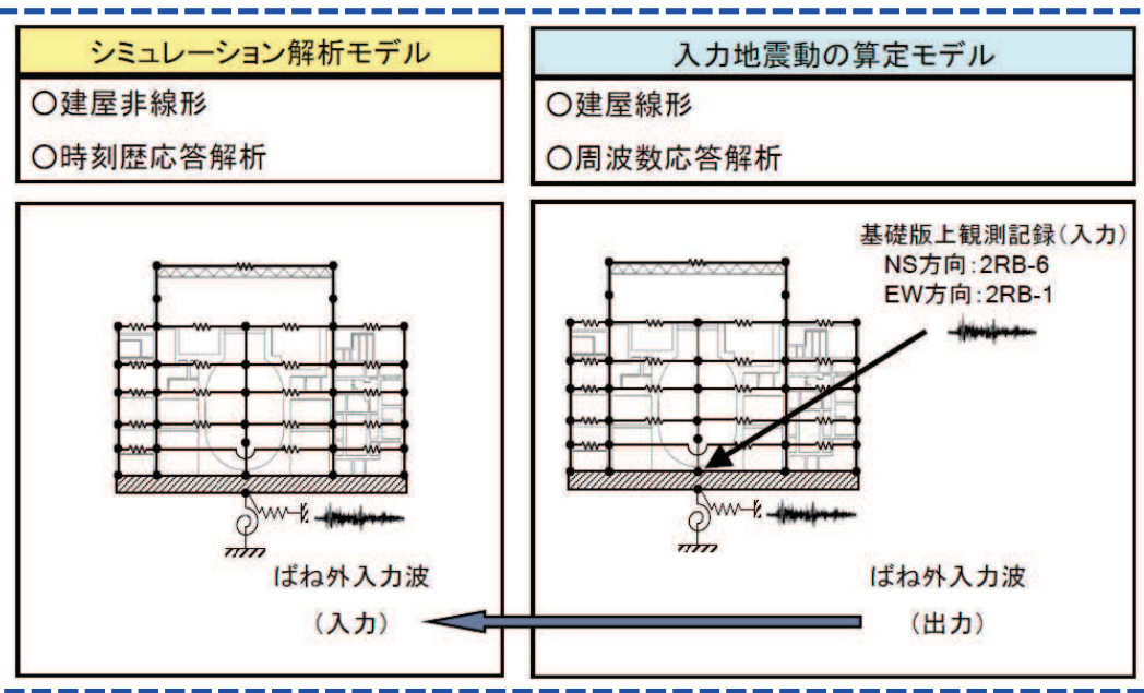
入力地震動の算出概念図(第475回審査会合(2017年6月15日) 資料1-4抜粋)
