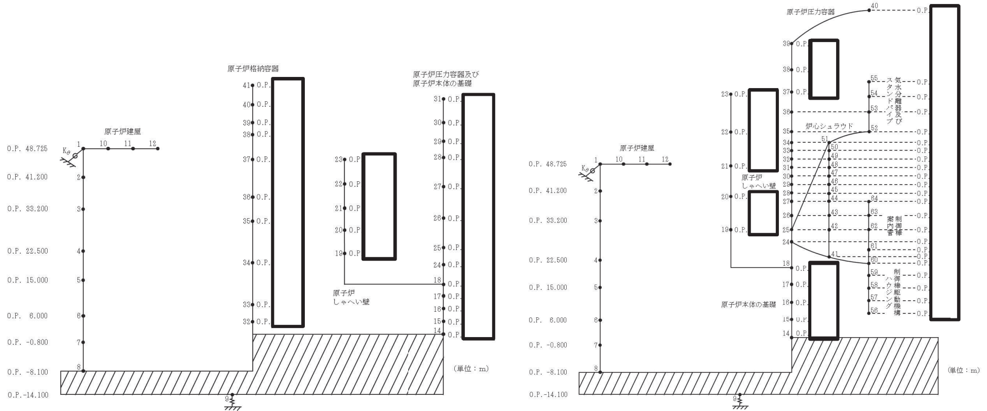
鉛直方向解析モデル(大型機器系)
