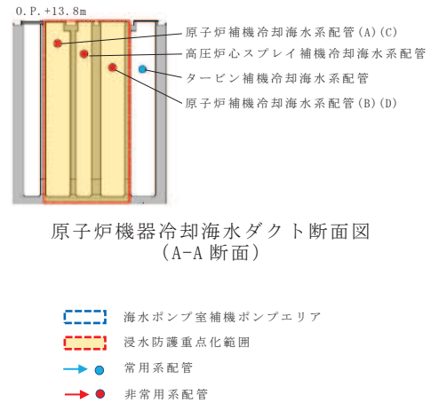
図 3-36 海水ポンプ室補機ポンプエリアの浸水防護重点化範囲及び断面図
