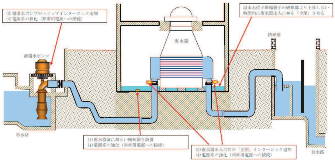
図 3-30 タービン建屋における循環水系配管からの溢水の評価方針の概要
