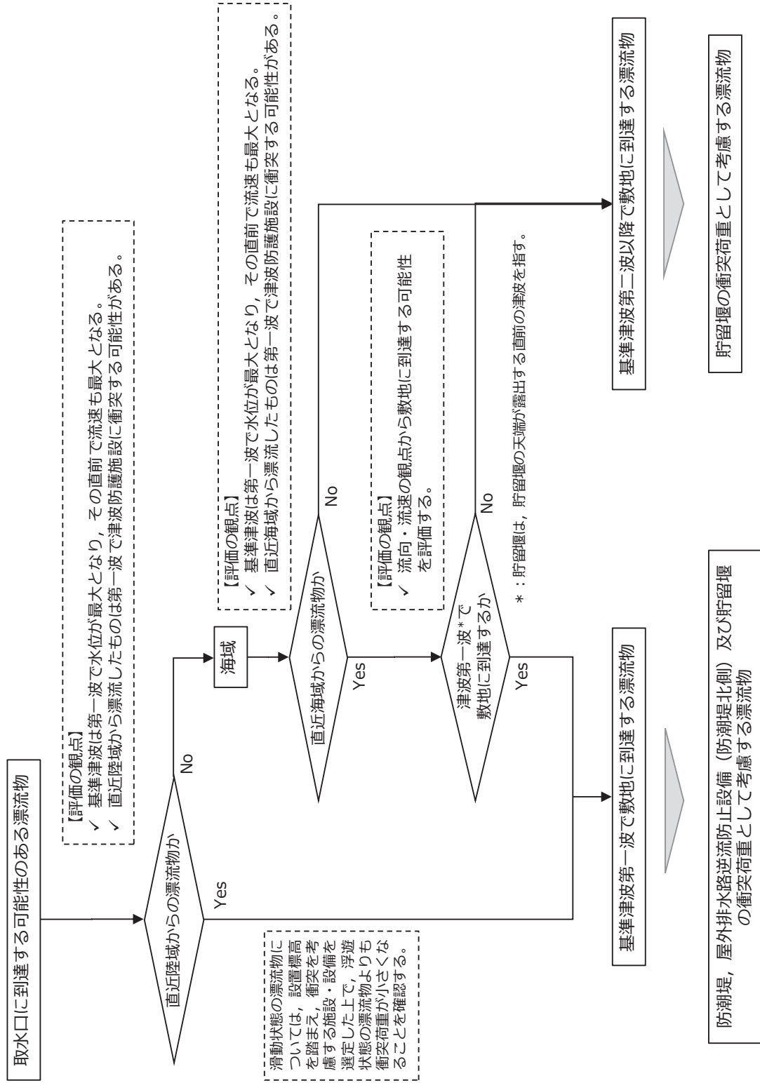
図 3-48 津波防護施設の機能に対する影響評価フロー
