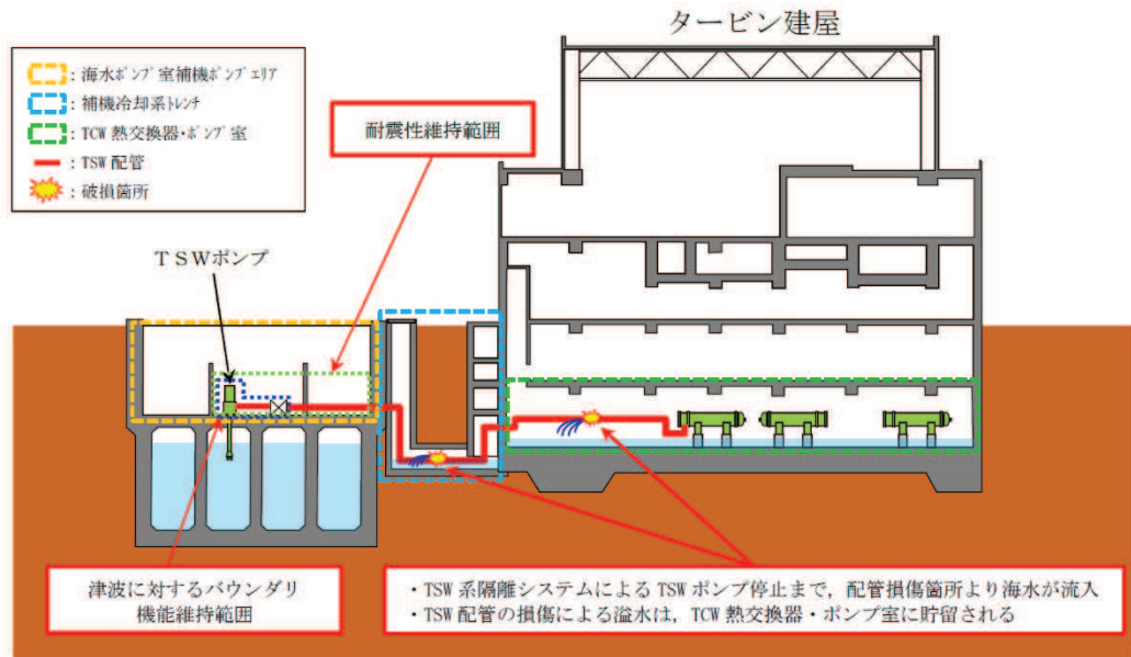
図 3-32 タービン補機冷却海水系配管からの溢水の評価方針の概要
