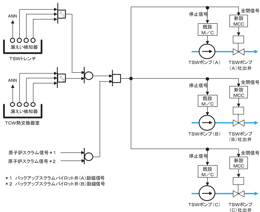
図 3-33 タービン補機冷却海水系隔離システムの概要
