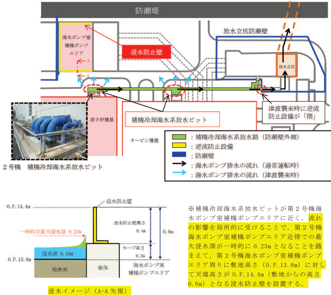
図 3-41 補機冷却海水系放水路からの溢水概要
