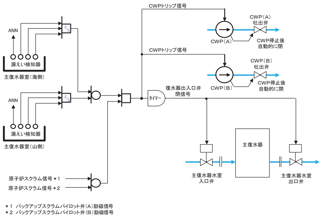
図 3-31 循環水系隔離システムの概要
