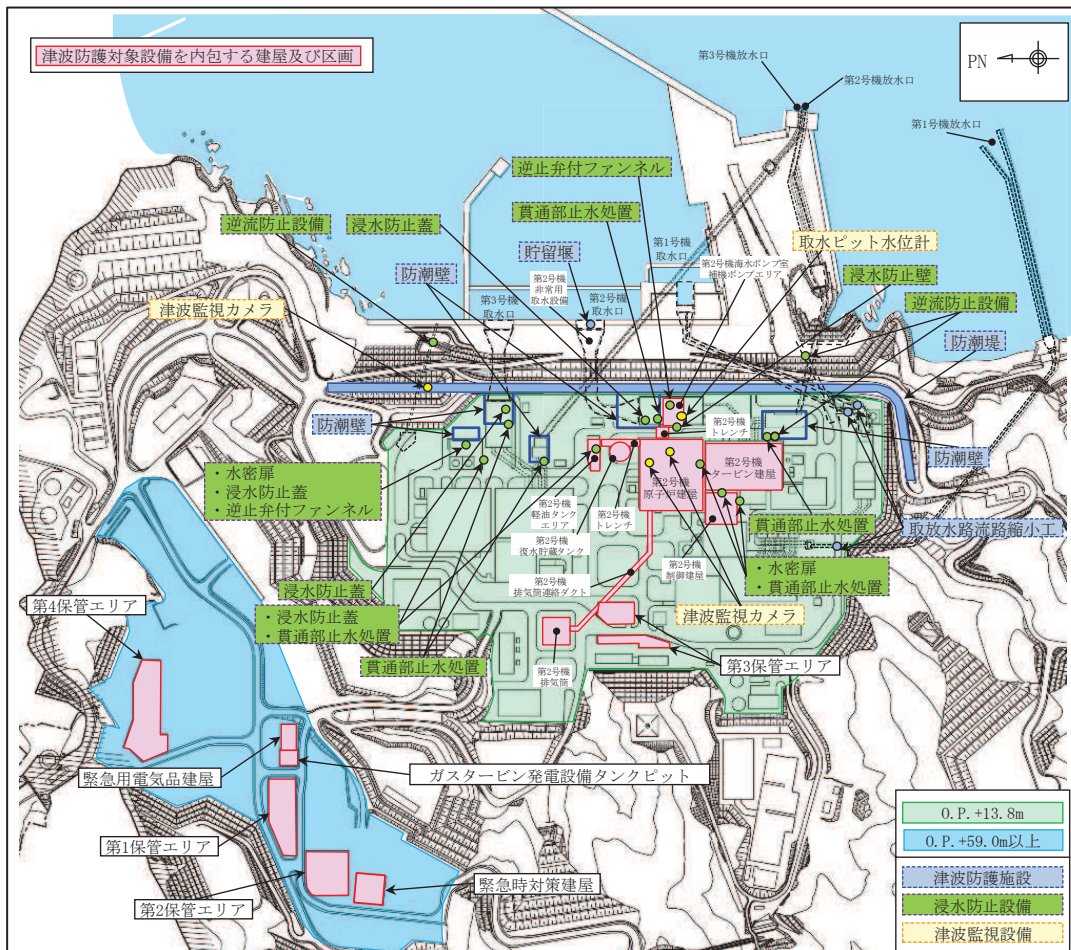
図 3-1 津波防護に関する施設の配置
