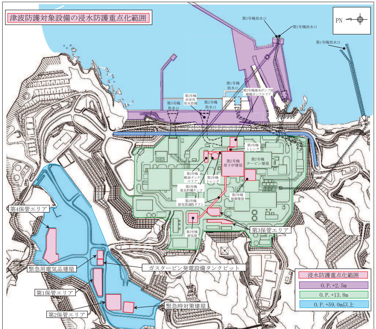
図 3-34 浸水防護重点化範囲
