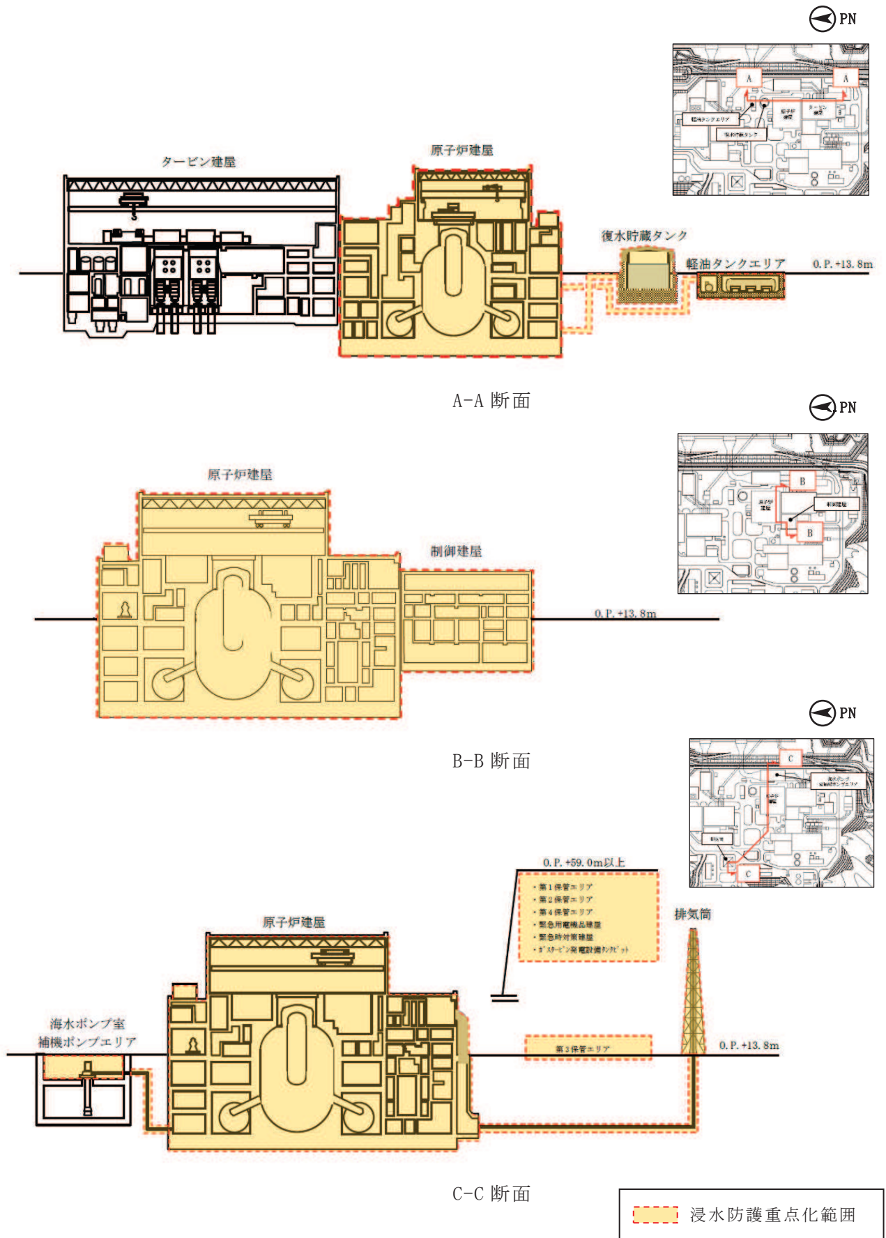
図 3-35 建屋断面概略及び浸水防護重点化範囲
