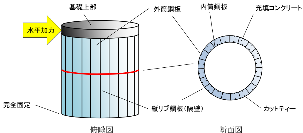
図 1 鋼コンクリート製の原子炉本体基礎を模擬した試験体のイメージ
