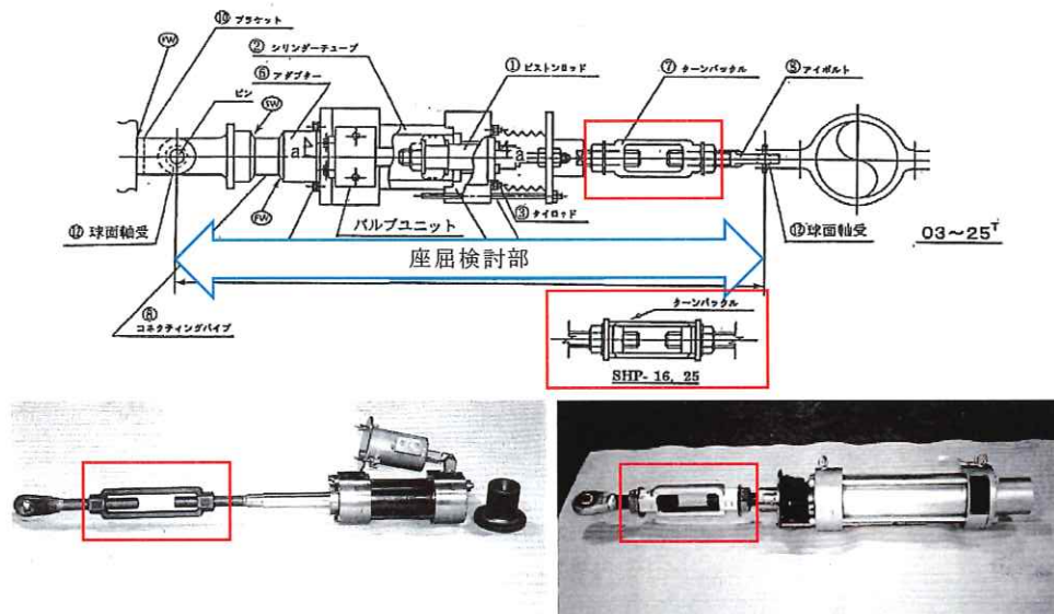
図1 SHP型オイルスナップの概略構造及びターンバックル部
