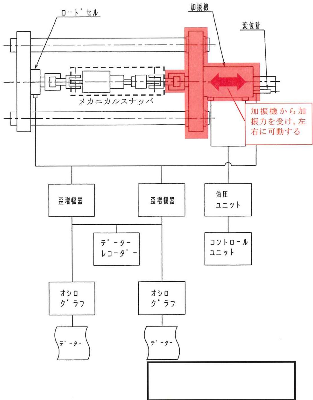
図 4-5 振動試験装置の概要
