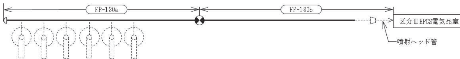
区分ⅢHPCS電気品室消火系 ハロン1301貯蔵容器
