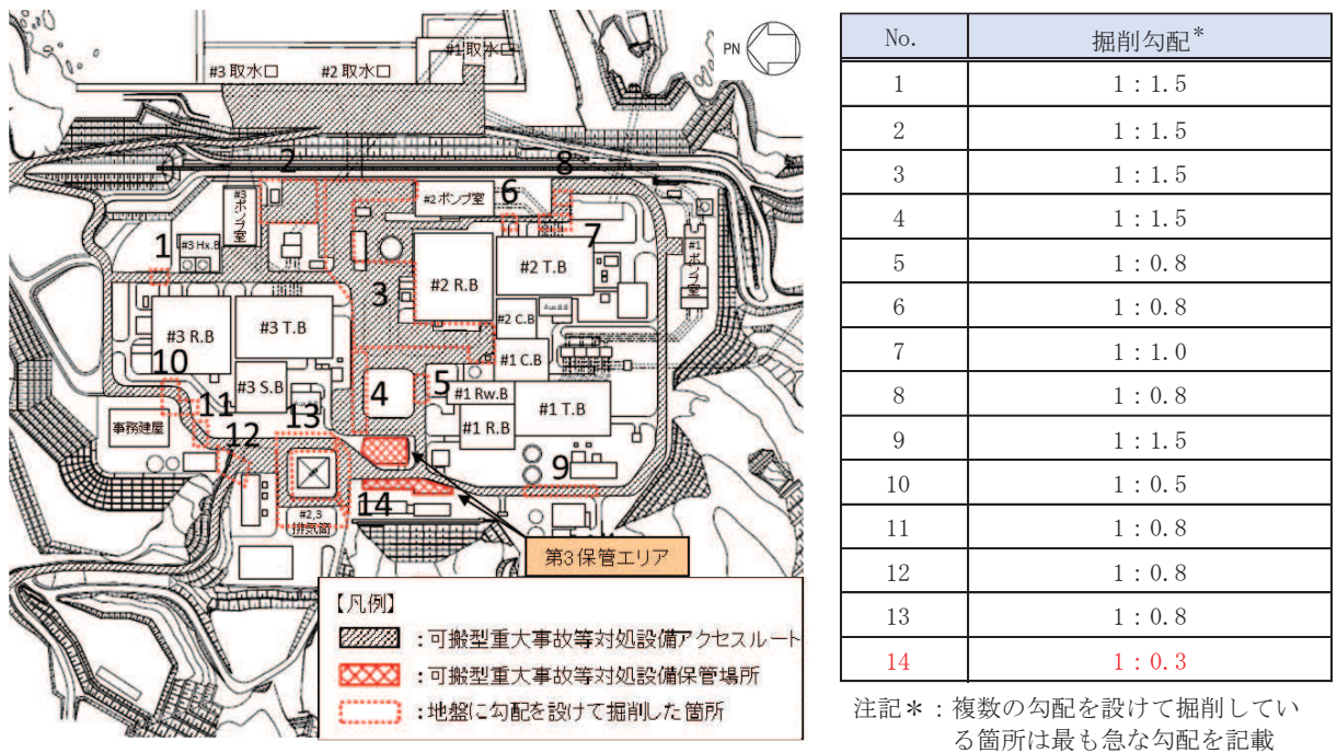
図 8.1-9 地山に勾配を設けて掘削した箇所の抽出結果
