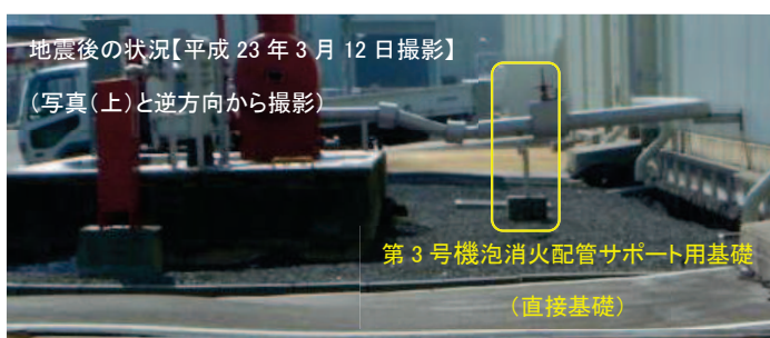
写真⑥' 沈下発生状況
