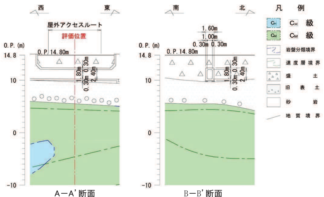
図 8.3-12 地質断面図
