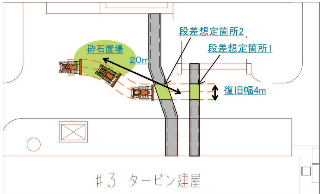
図 10.1-2 仮復旧の方法
