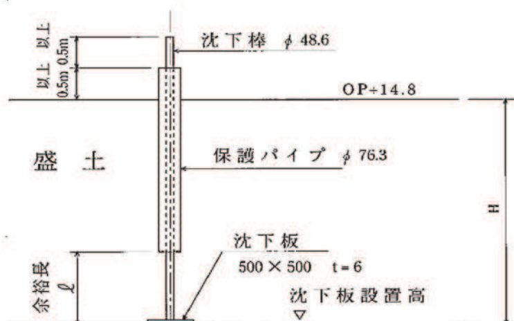
図7.2-1 沈下棒の構造
