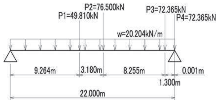
図 8.6-24 H形鋼に発生するせん断力及び接地圧が最大となる場合の荷重図
