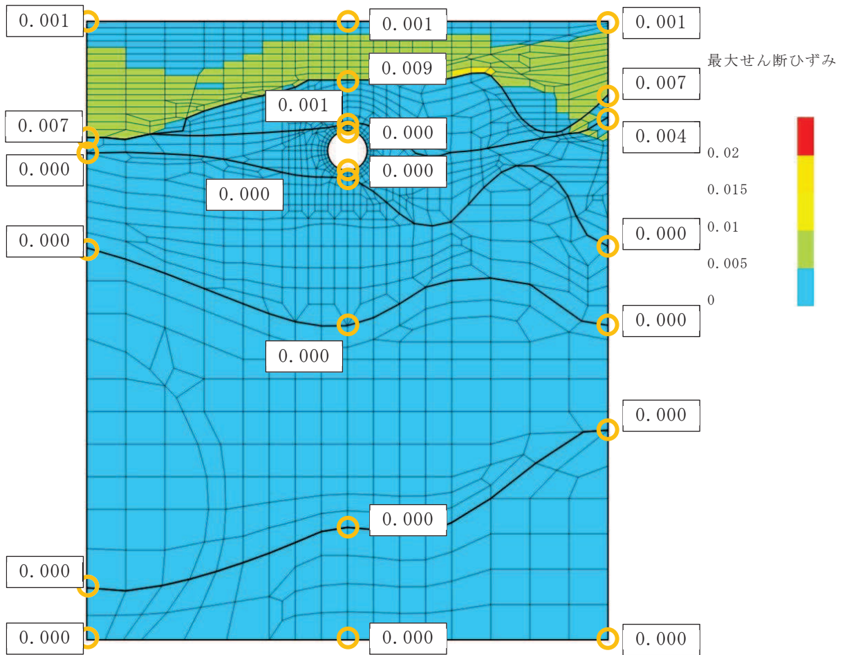
図 4-4(3) 排気筒連絡ダクト岩盤部（断面⑤）における最大せん断ひずみ分布図 （全応力解析， S_s - D 2 （-+）ケース④）
