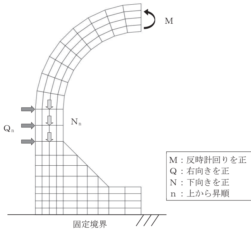
図 5-18 材料非線形解析における荷況 (側壁)
