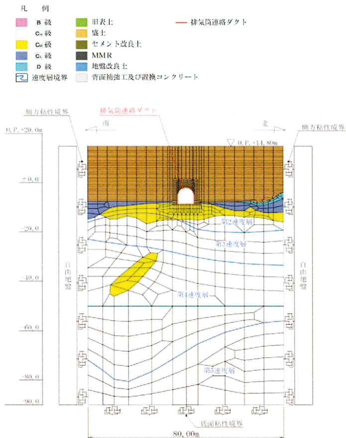
(b) 地震応答解析モデル図
