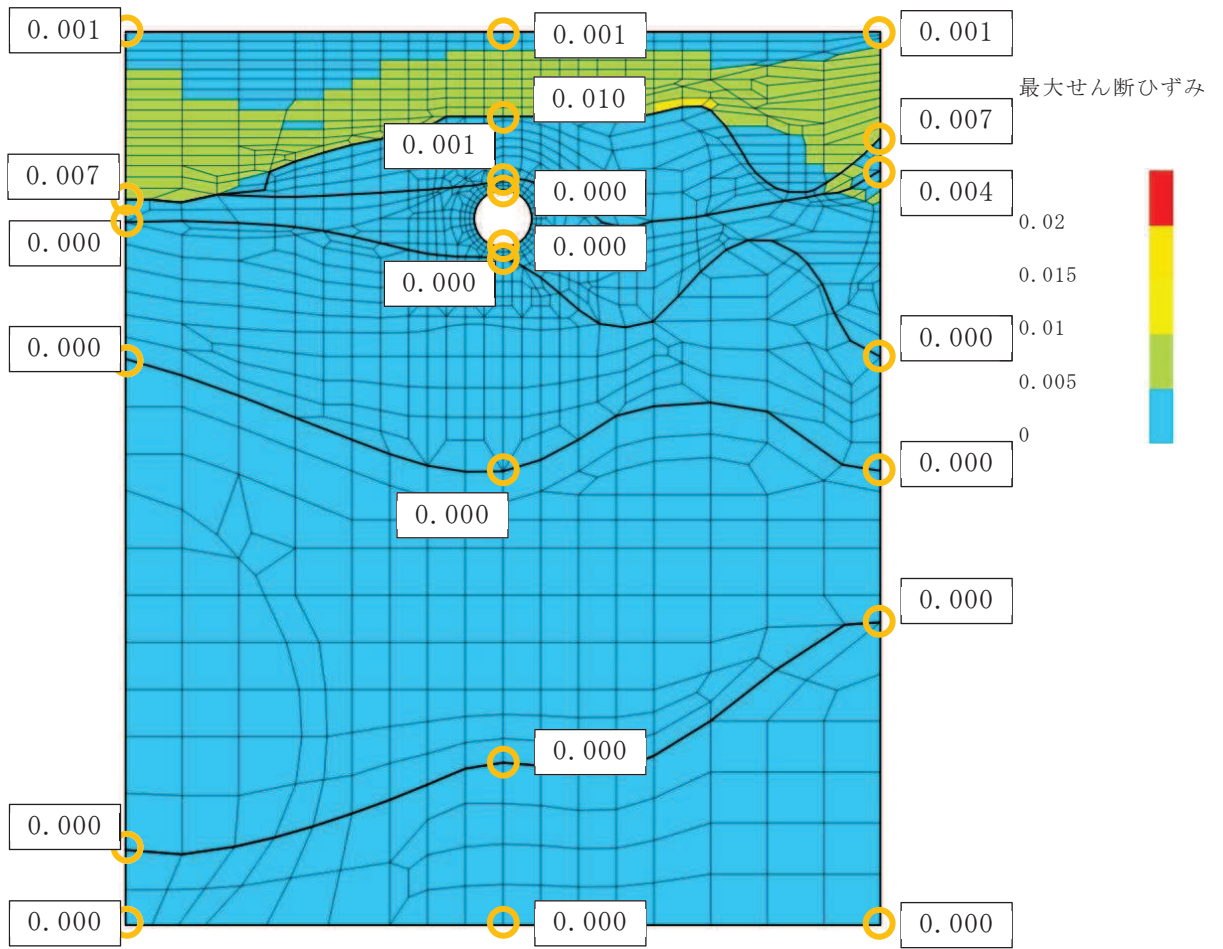
図 4-5(3) 排気筒連絡ダクト岩盤部 (断面⑤) における最大せん断ひずみ分布図 (全応力解析, S_s - D2 (-+) ケース③)
