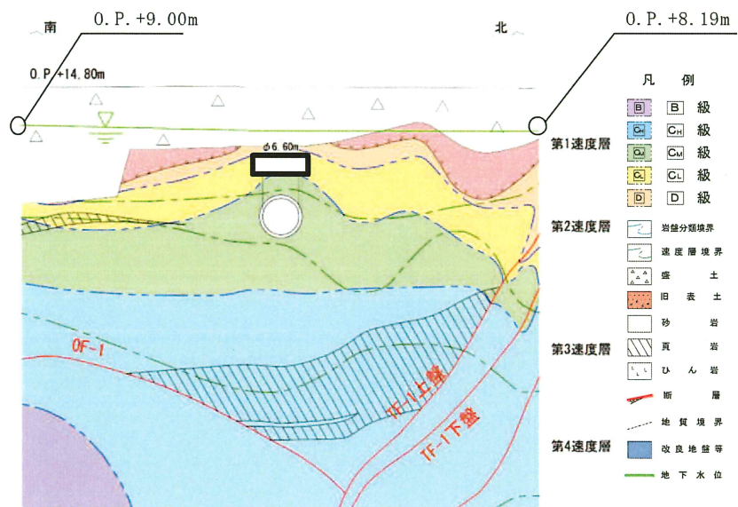
図 2-2 排気筒連絡ダクト岩盤部（断面⑤）における地質断面図
