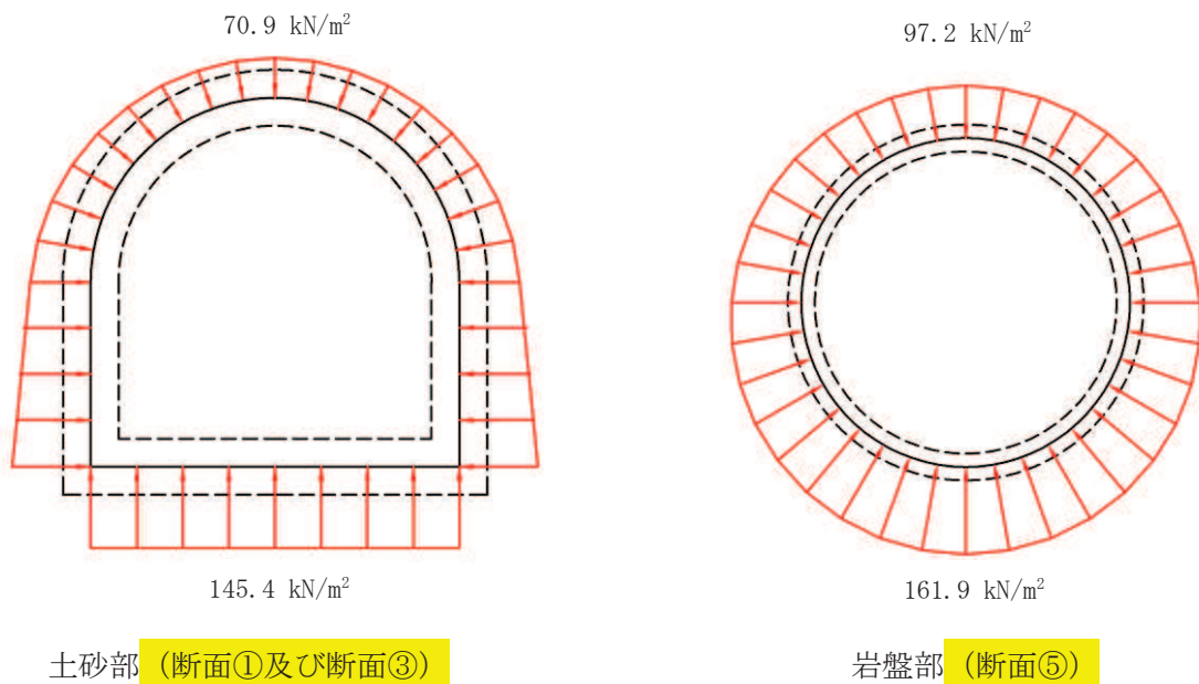
図3-22 外水圧図
