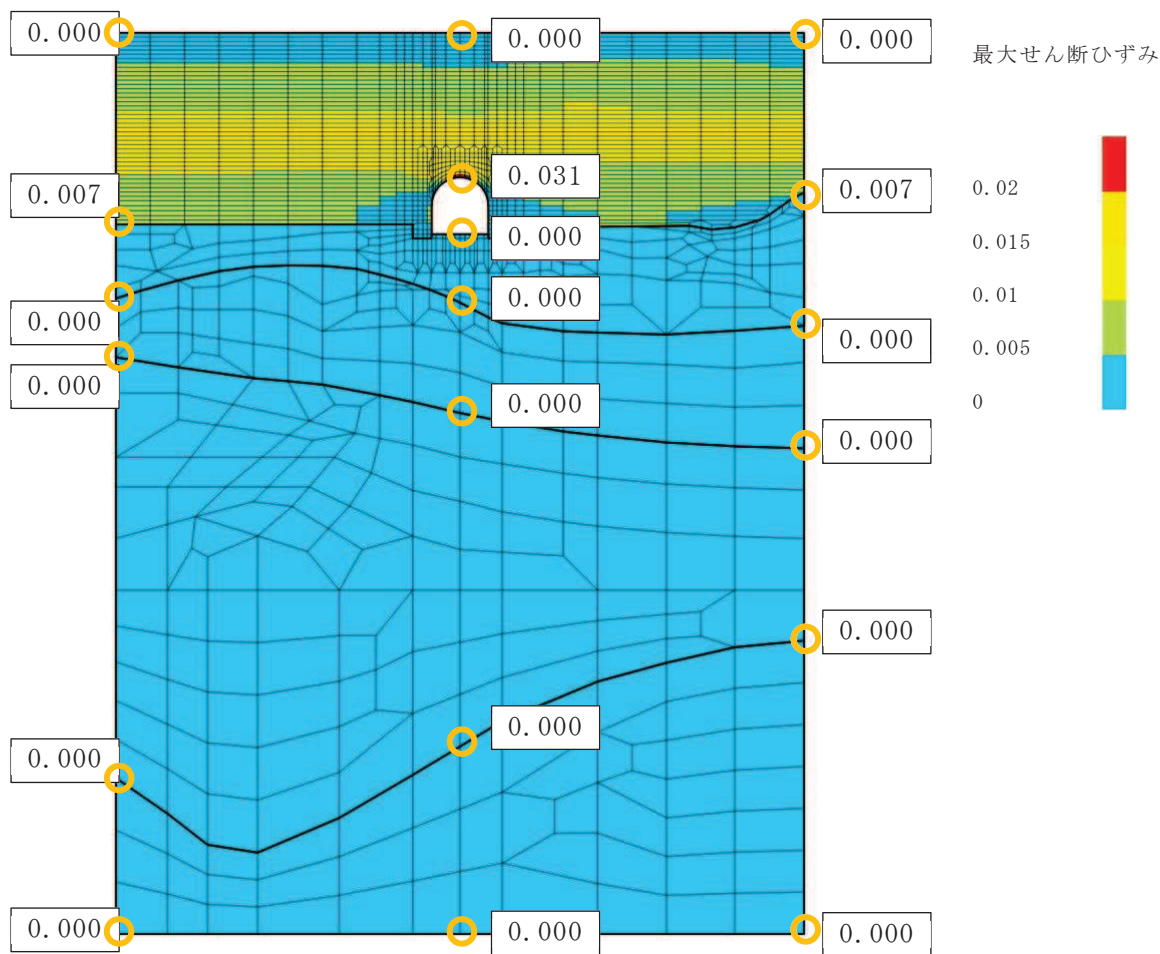
図 4-2(3) 排気筒連絡ダクト土砂部（断面①）における最大せん断ひずみ分布図 （全応力解析， S_s - N1 （++）ケース④）
