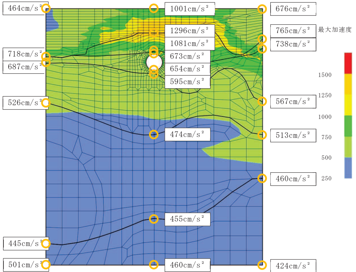
図 4-5(1) 排気筒連絡ダクト岩盤部 (断面⑤) における最大加速度分布図 (全応力解析, S_s - D2 (-+) ケース③)
