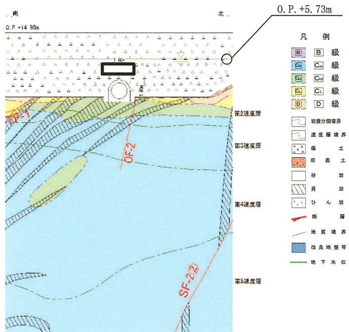
(a) 評価対象地質断面図
