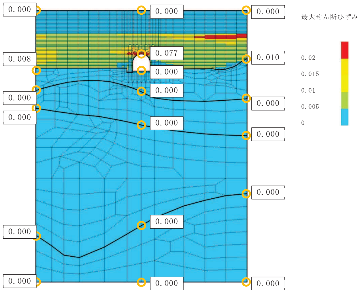
図 4-3(3) 排気筒連絡ダクト土砂部 (断面①) における最大せん断ひずみ分布図 (有効応力解析, S_s - D_3 (-+) ケース⑦)
