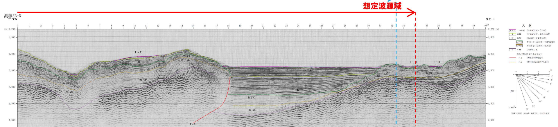
音波探査記録と解析図(測線3B-5)
