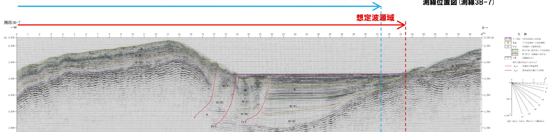
音波探査記録と解析図(測線3B-7)
