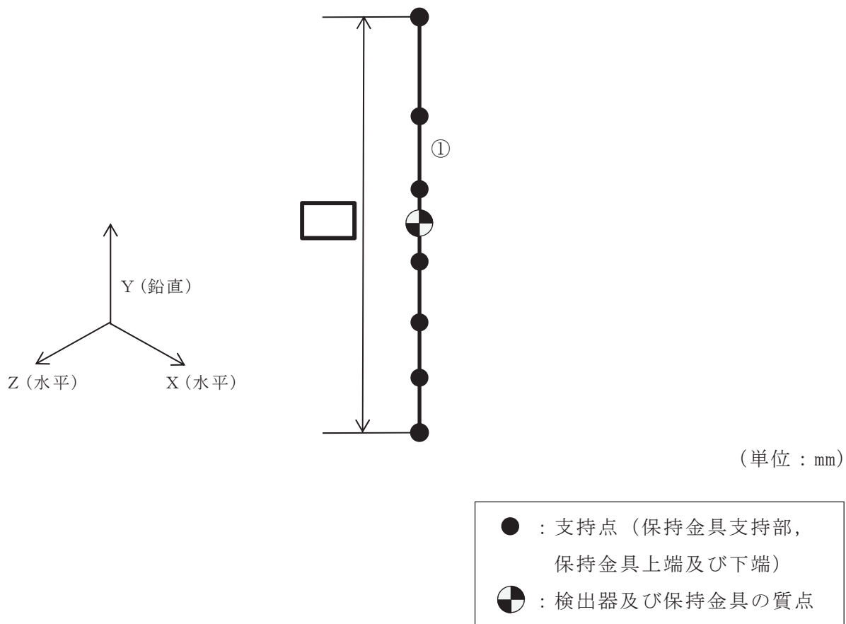
図 4-1 主蒸気管放射線モニタ解析モデル
