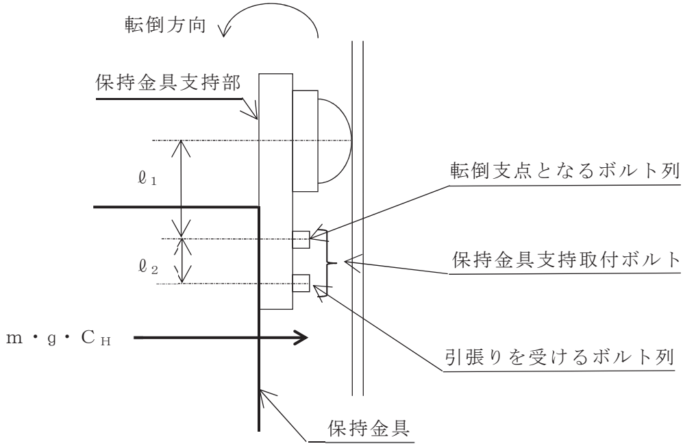
図5-1 計算モデル
