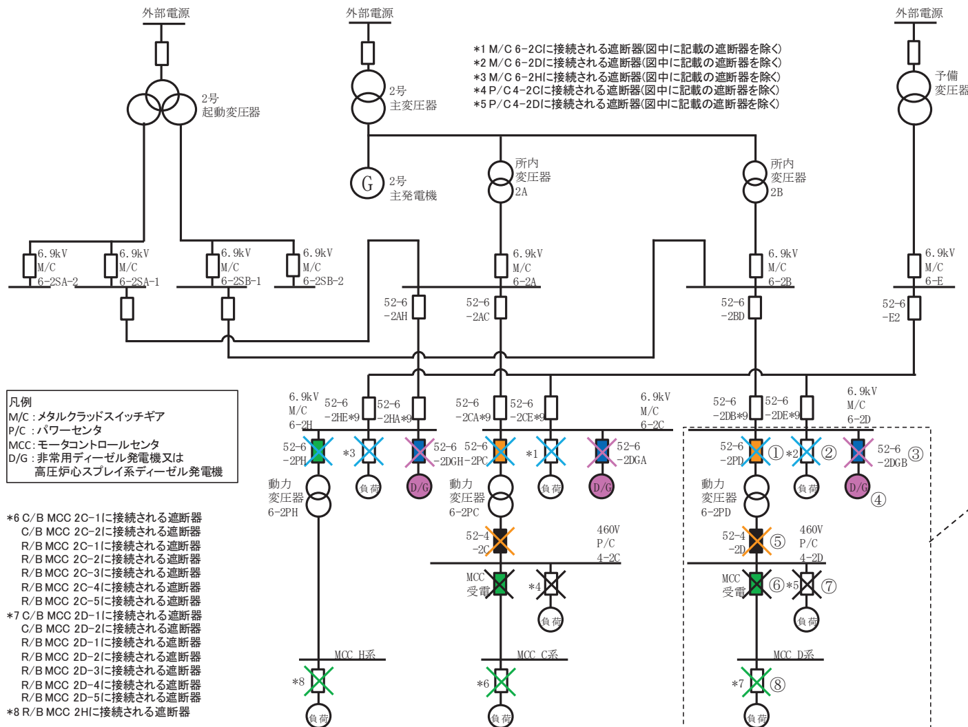
図 3.3 HEAF 対策が必要な電気盤系統図 (2/2) (非常用ディーゼル発電機又は高圧炉心スプレイ系ディーゼル発電機からの給電時)
