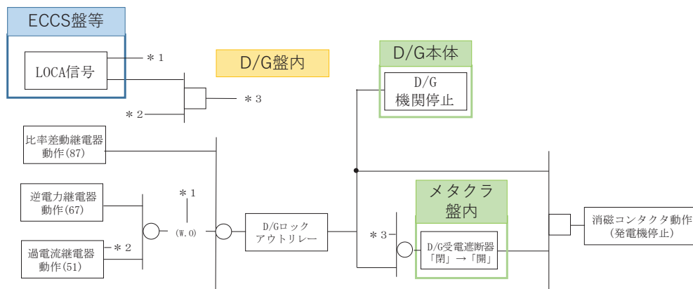
図 2-1 既設インターロック
