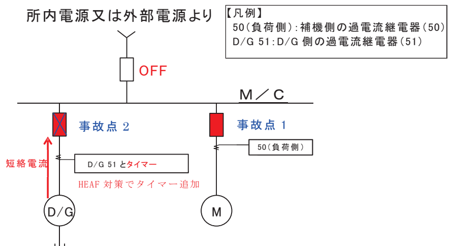
図 2-3 M/C への D/G 給電時の電源構成 (HEAF 対策後)
