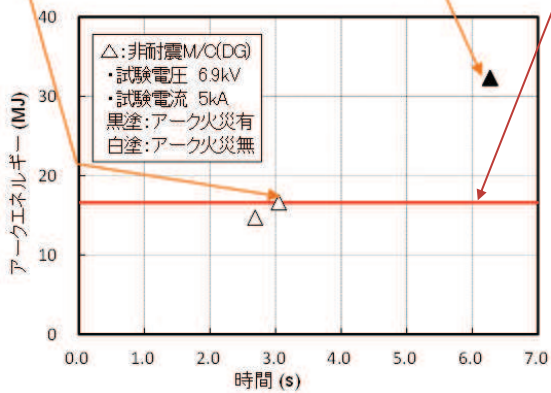
図 5.3.4 M/C(D/G) 試験結果
