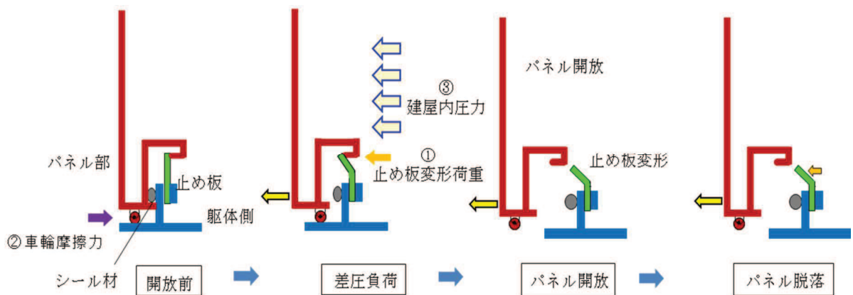
図 3-1 原子炉建屋 BOP 開放のメカニズム
