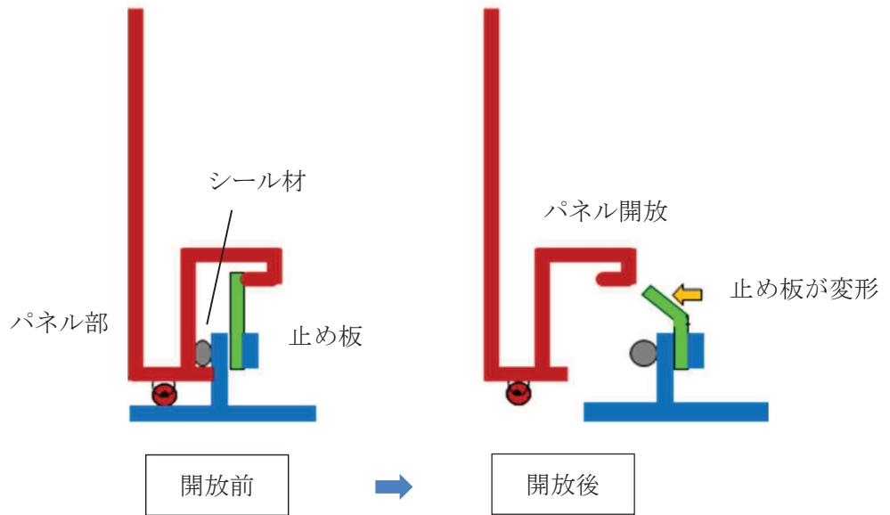
図 2-1 原子炉建屋 BOP の構造と作動原理
