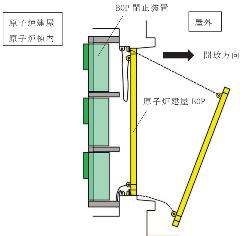
図1-1 原子炉建屋BOPとBOP閉止装置の配置関係
