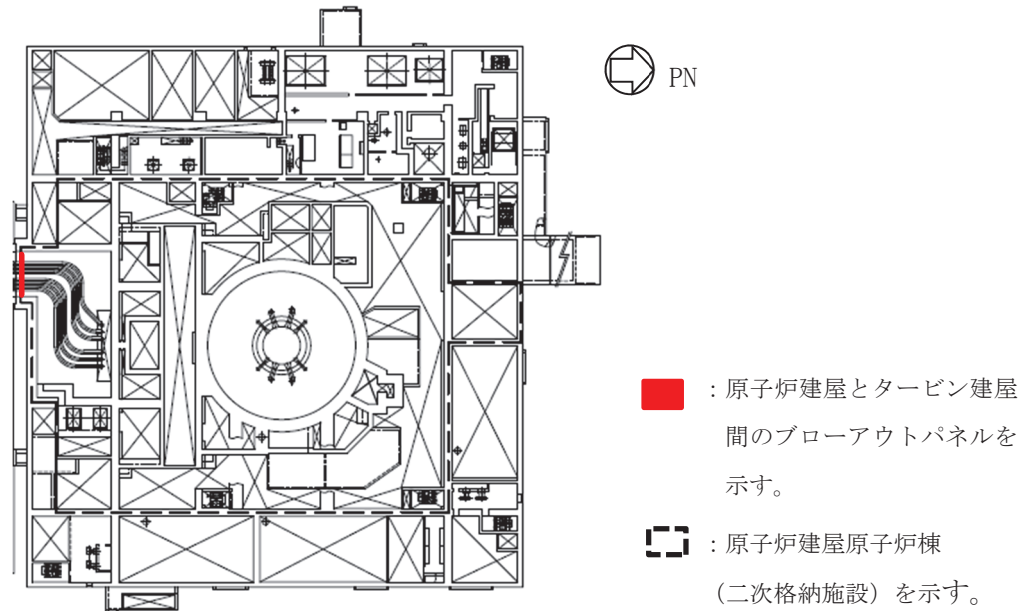
原子炉建屋原子炉棟地上中 2 階 概略平面図 (0. P. 19. 10m)
