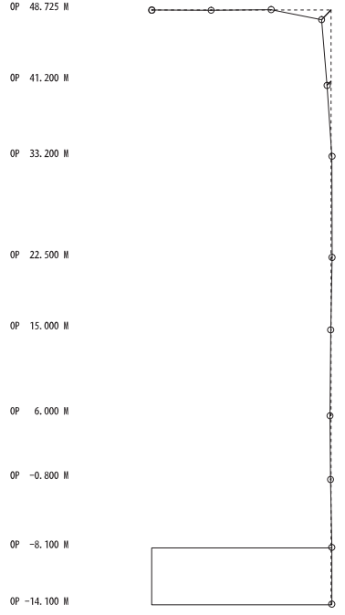
7次モード
