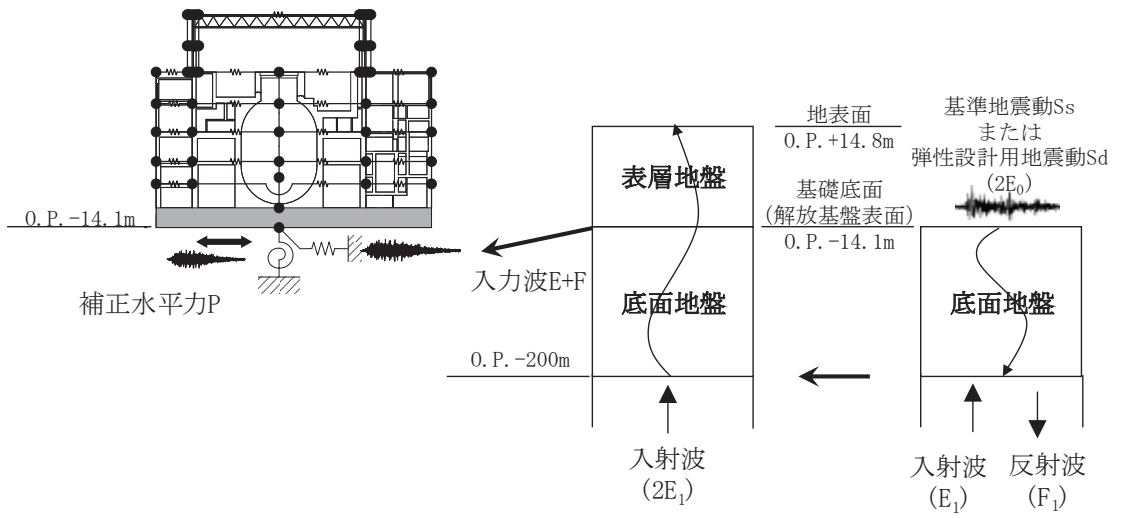
図 3-10 地震応答解析モデルに入力する地震動の概念図（水平方向）
