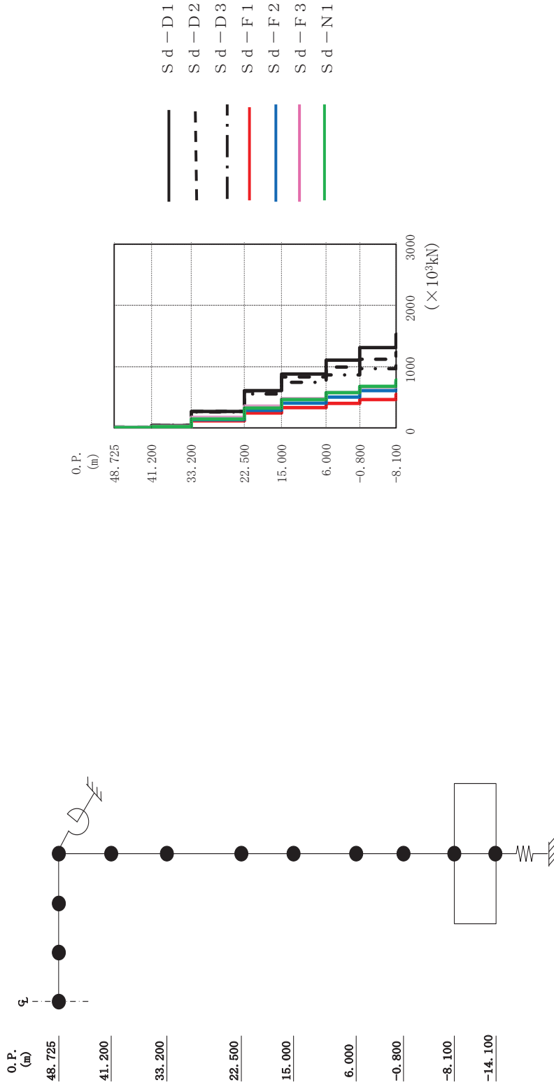
图 4-25 最大応答軸力 (弾性設計用地震動 S d , 鉛直方向)
