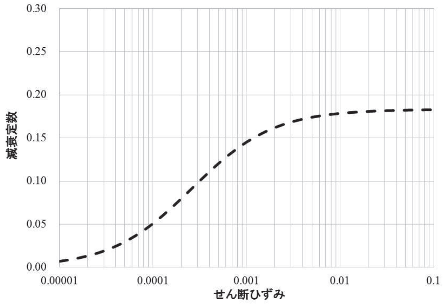
図 3-9 h - \gamma 曲線
