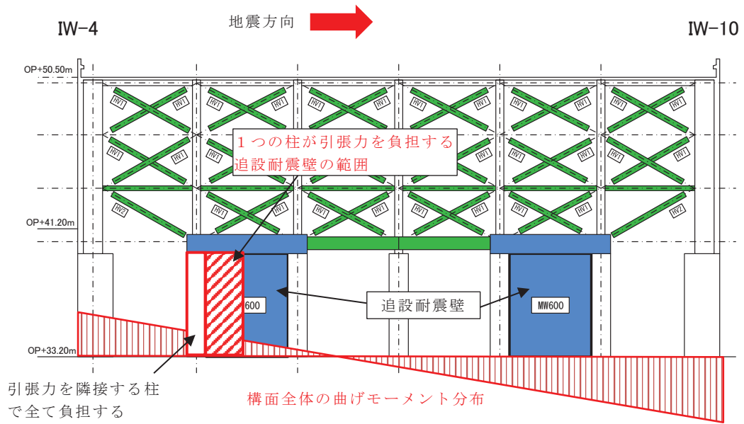
図 3-6 曲げモーメントに対する追設耐震壁の設計手法の概要
