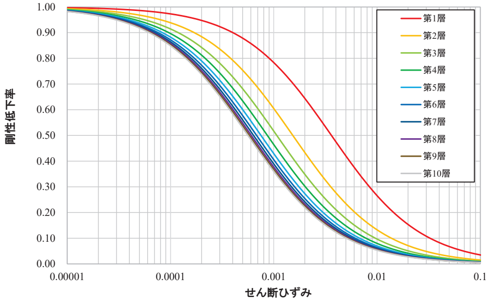
図 3-8 G/G_0 - \gamma 曲線
