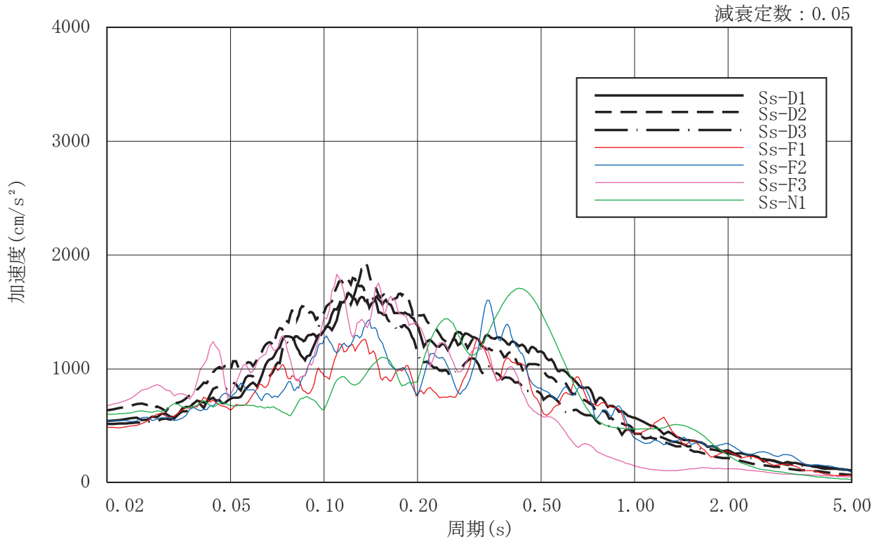
図 3-11 (1) 入力地震動の加速度応答スペクトル (基準地震動 S_s , O.P.-14.1m)
