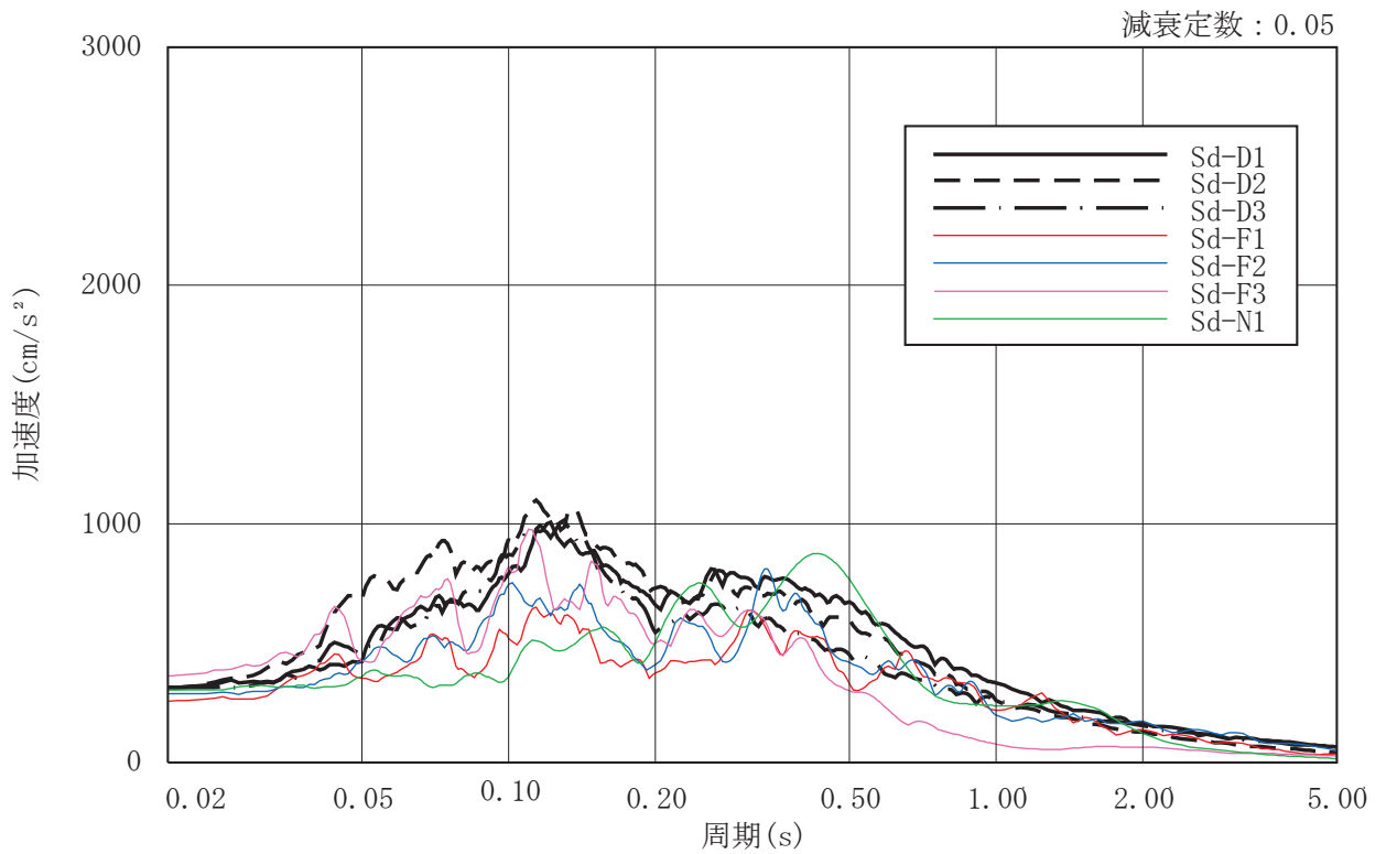
図 3-11 (2) 入力地震動の加速度応答スペクトル (弾性設計用地震動 S_d , O.P.-14.1m)
