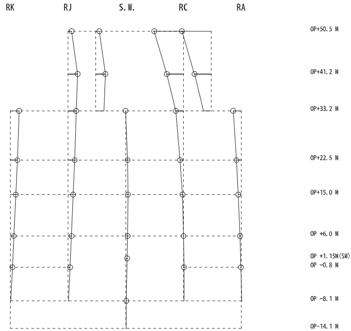
3 次モード
