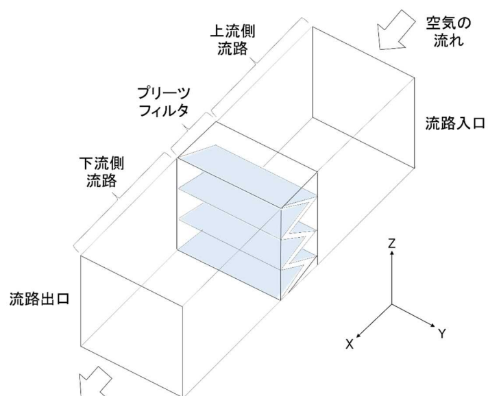
図1 プリーツフィルタ及び流路の概略図
