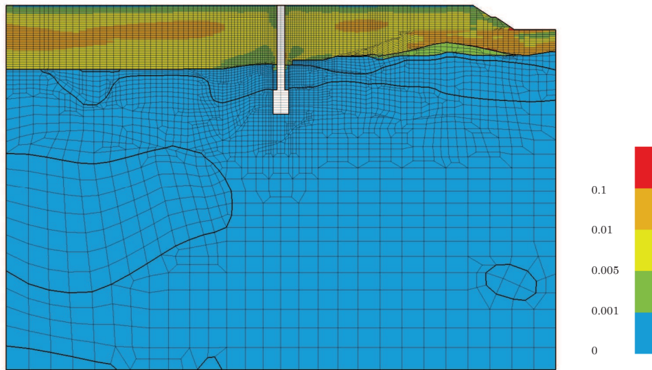
図 4-34(19) 最大せん断ひずみ分布 (No. 4 揚水井戸, S s - N 1 (一十), 解析ケース①) (全応力解析)
