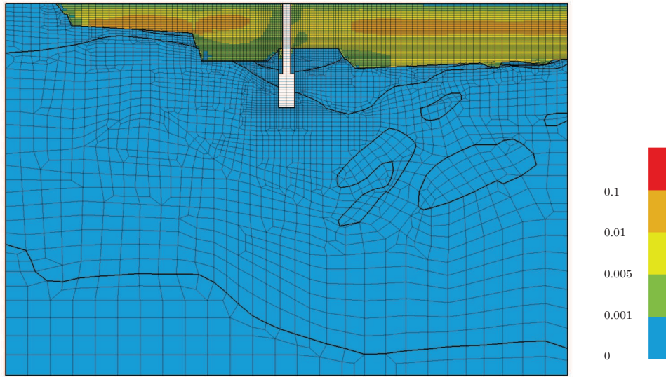
図 4-34(3) 最大せん断ひずみ分布 (No.1 揚水井戸, S s - N 1 (一+), 解析ケース②) (全応力解析)
