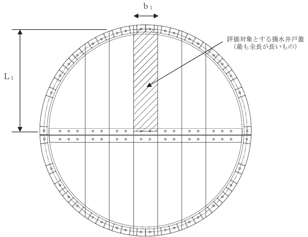
図 5-1 評価の対象とする揚水井戸蓋
