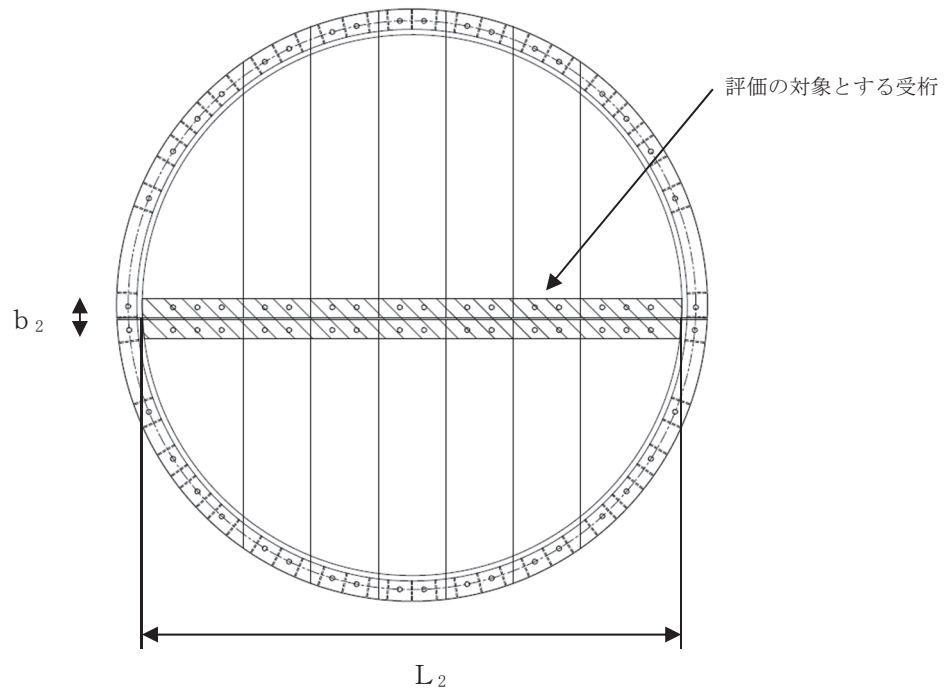
図 5-2 評価の対象とする受桁
