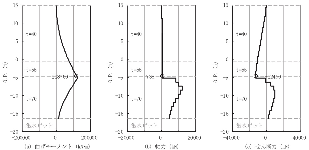
図 4-1(2) 排水シャフト 軸方向照査における曲げ・軸力系の破壊に対する評価時刻での断面力 (No.1 揚水井戸 (板厚 t=55\text{mm} ), S s -N1 (++) , 7.77s)
