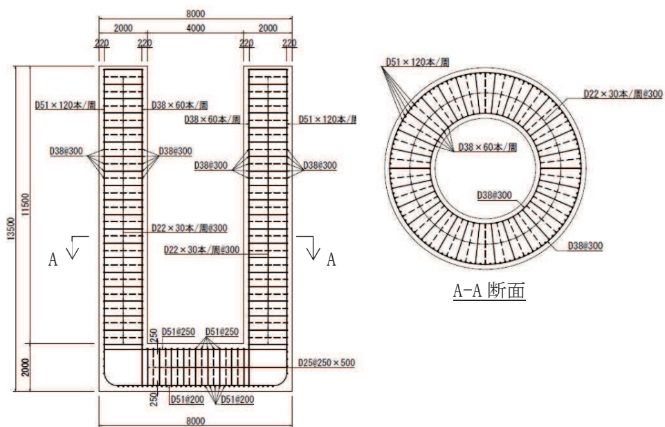
図 1 ( 2 ) No.2 揚水井戸 概略配筋図
