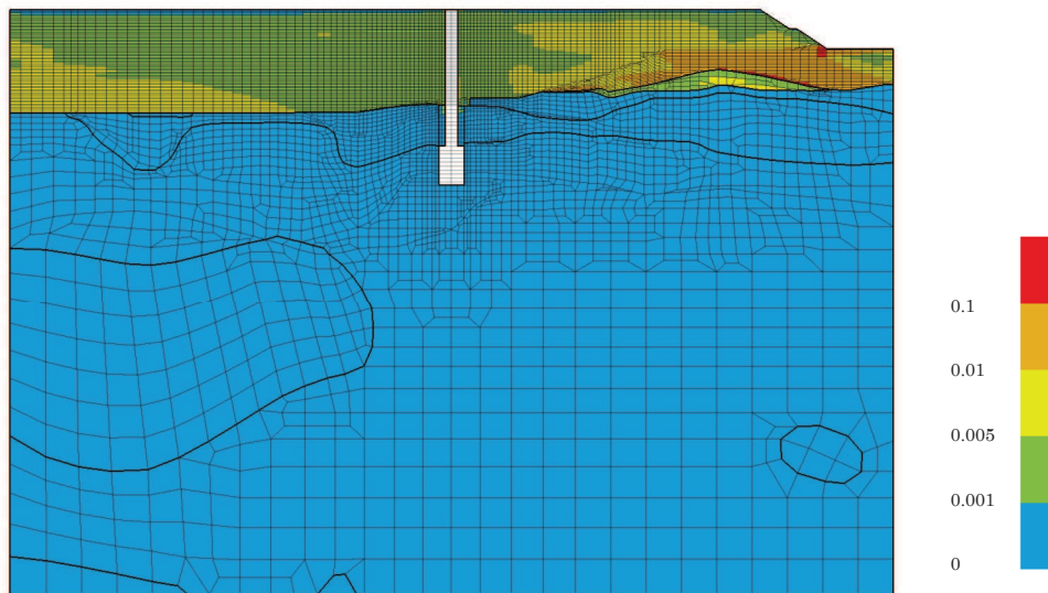
図 4-34(20) 最大せん断ひずみ分布 (No. 4 揚水井戸, S s - D 2 (一十), 解析ケース③) (全応力解析)
