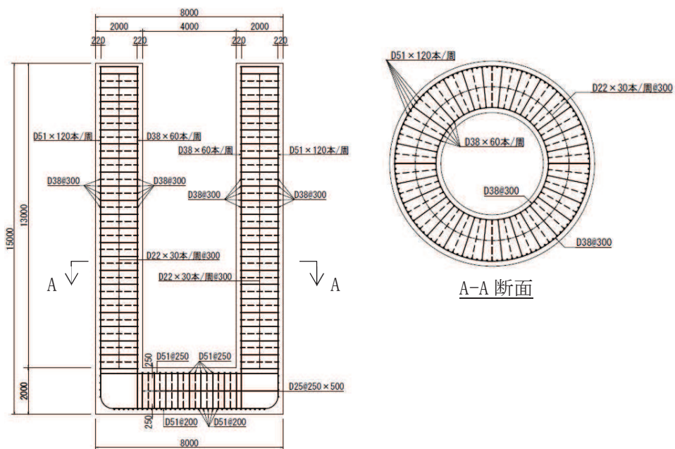
図 1 ( 1 ) No.1 揚水井戸 概略配筋図
