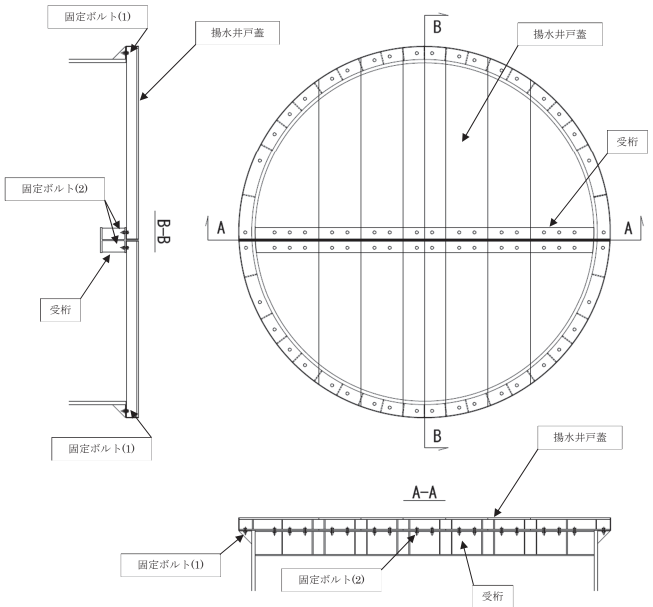
図 3-1(2) 評価対象部位 (No. 3, No. 4 揚水井戸蓋)
