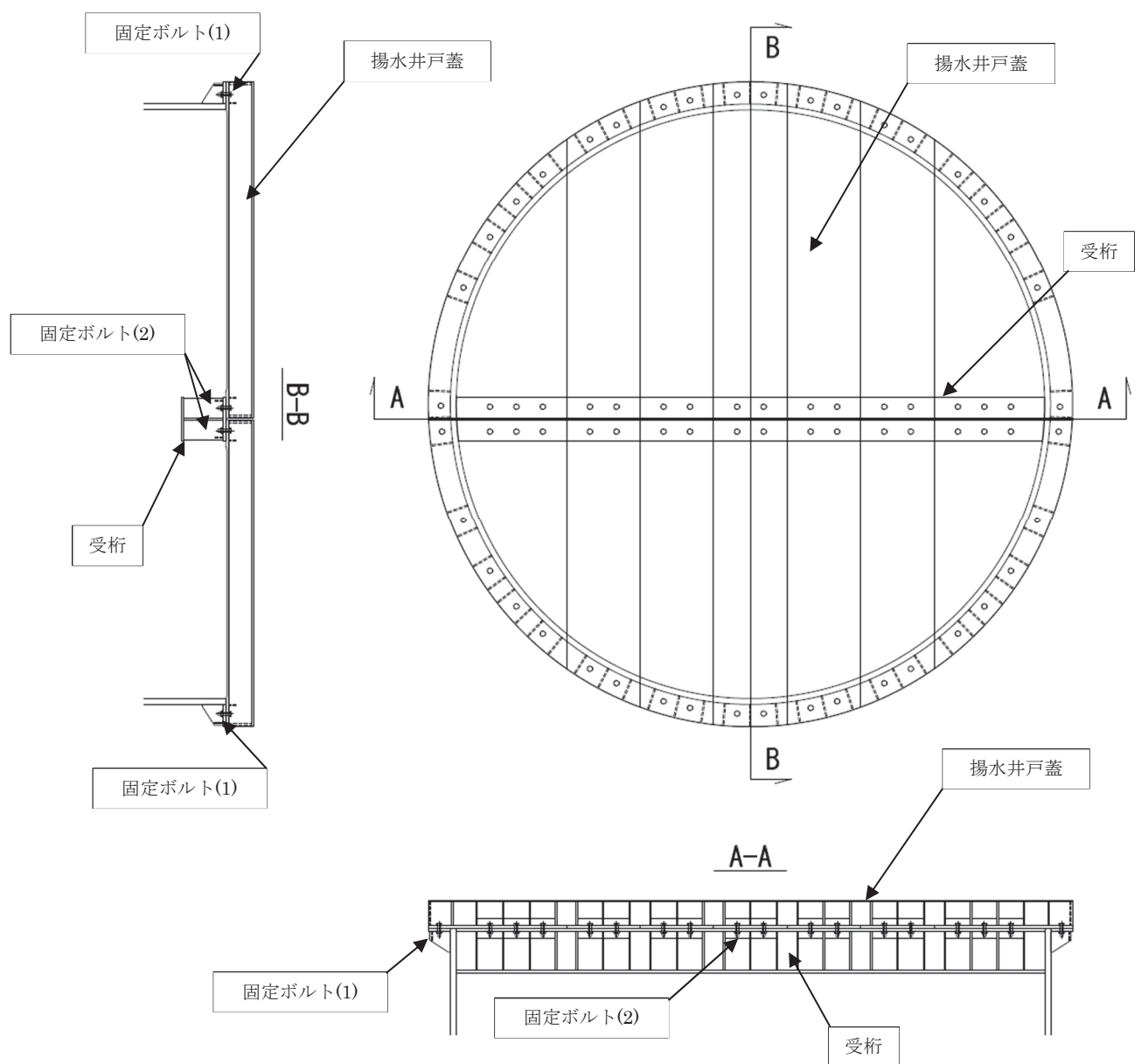
図3-1(1) 評価対象部位 (No. 1, No. 2 揚水井戸蓋)
