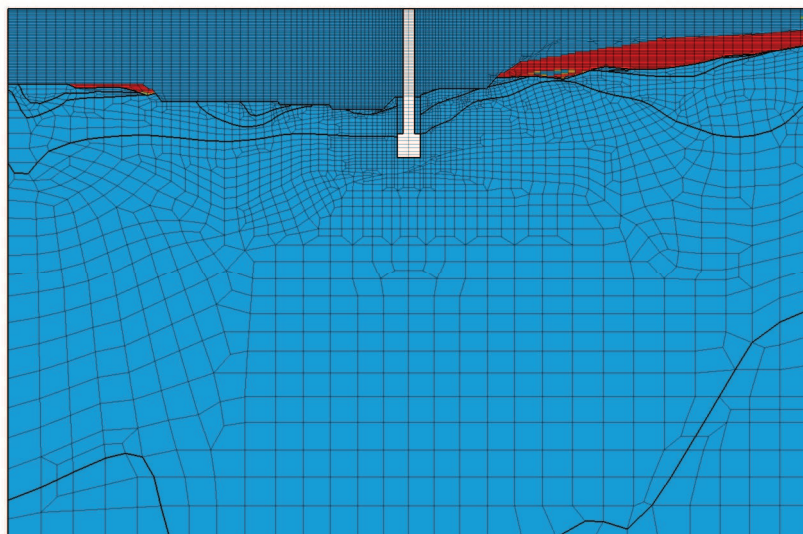
図 4-35(9) 最大過剰間隙水圧比分布 (No. 3 揚水井戸, S_s - N 1 (一十), 解析ケース①)
