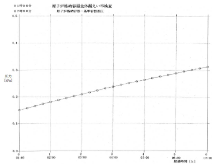
図 4.3.8-4 差圧測定結果
