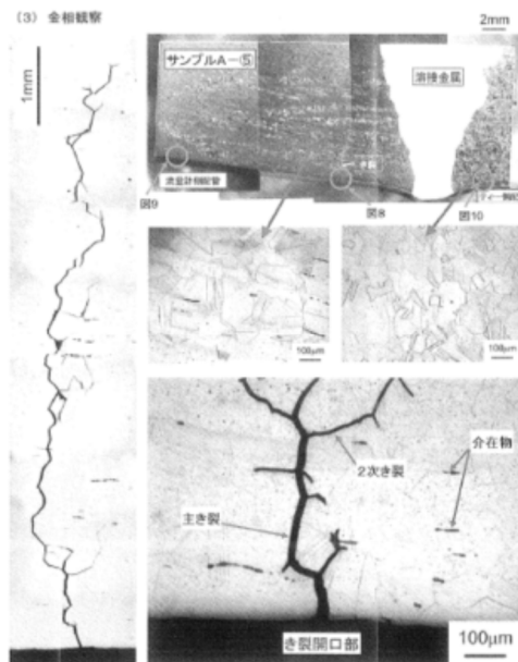
図7 き裂部の全体(左図)及びシュウ酸エッチング後の金属組織(右側図)
