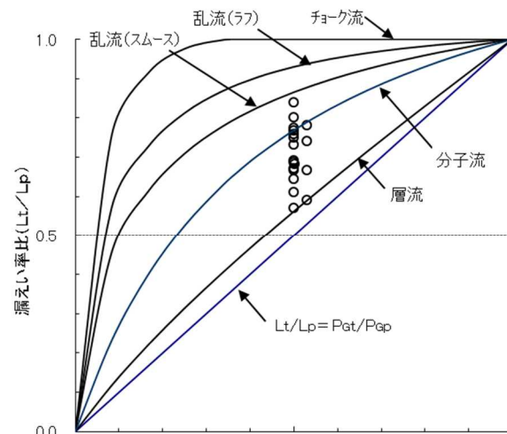
解説図 2-10.1 圧力比と漏えい率比の関係 (実機)
