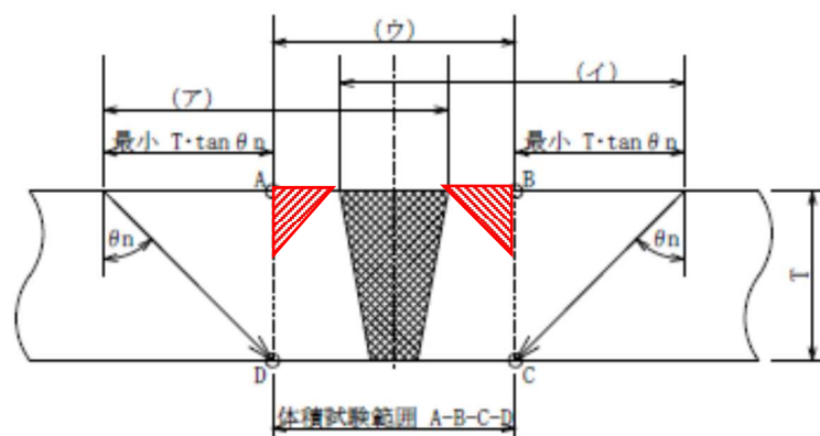
(1) 直射法 (0.5 スキップ) で試験する場合
