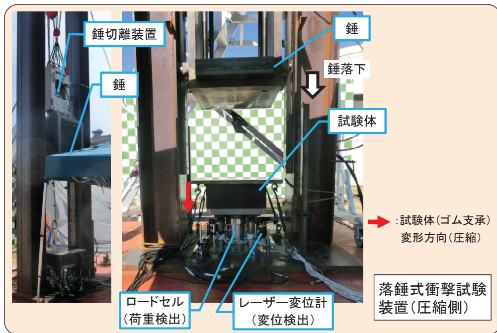
参考図1-2 試験装置外観
