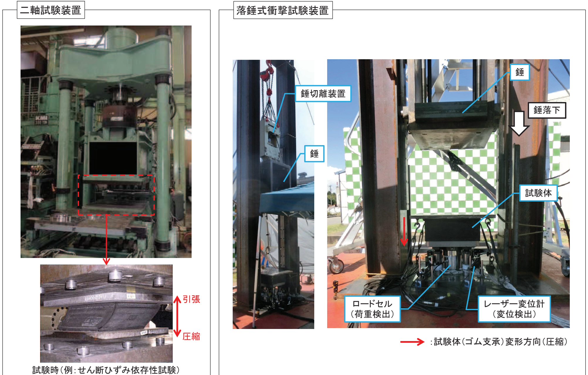
図3-2 試験装置外観
