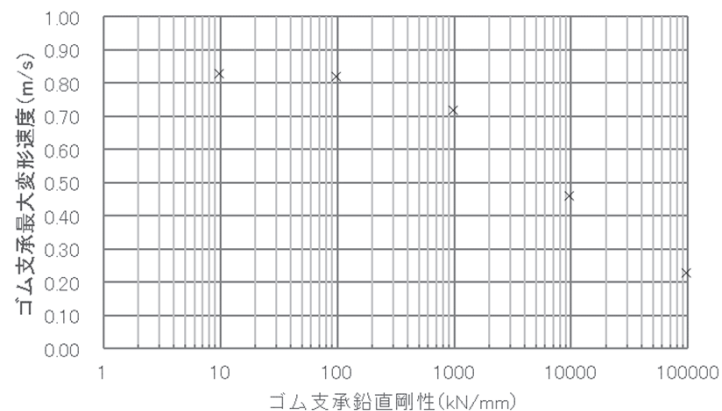
参考図1-1 ゴム支承の鉛直剛性と最大変形速度の関係
