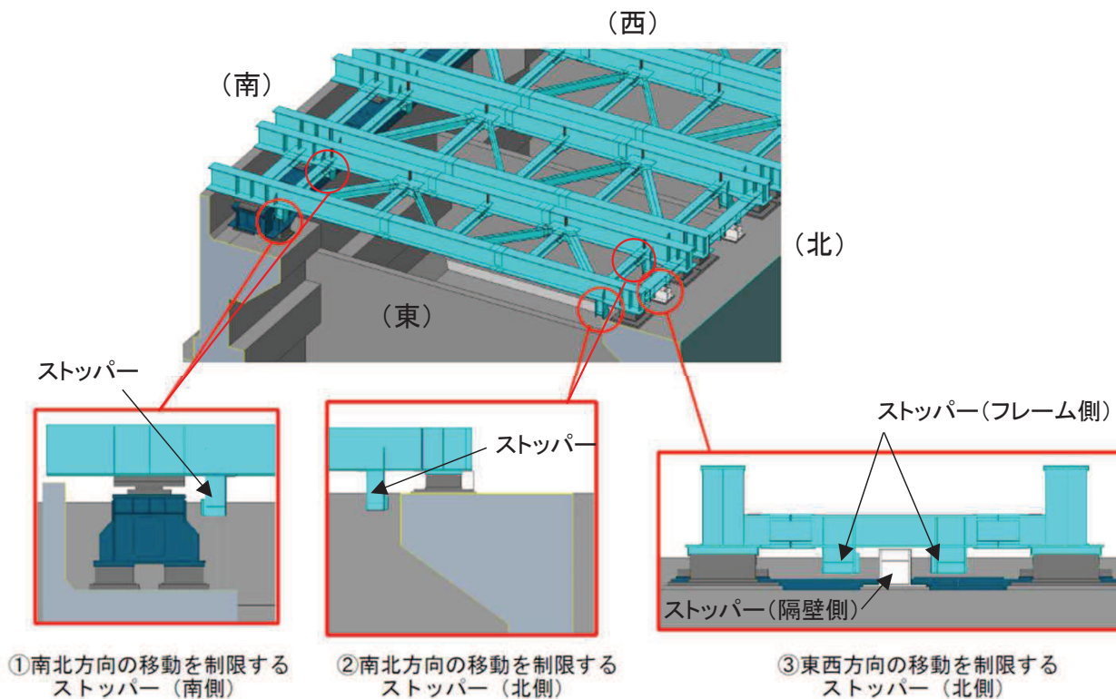
参考図3-1 ストッパーの設置位置及び構造概要
