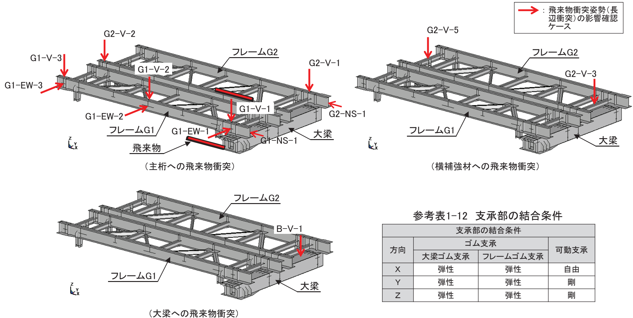
参考図1-5 解析モデル及び解析ケース
