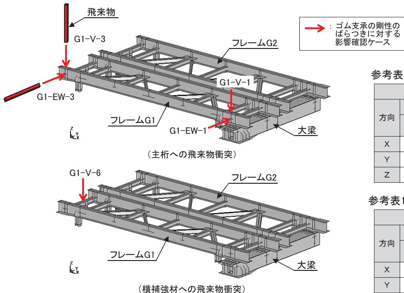
参考図1-4 解析モデル及び解析ケース
