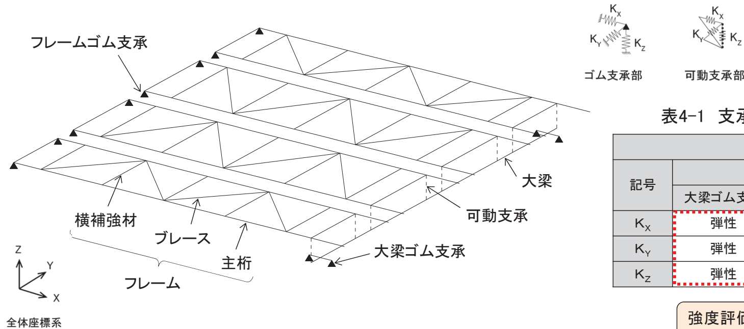
図4-2 耐震評価における解析モデル図
