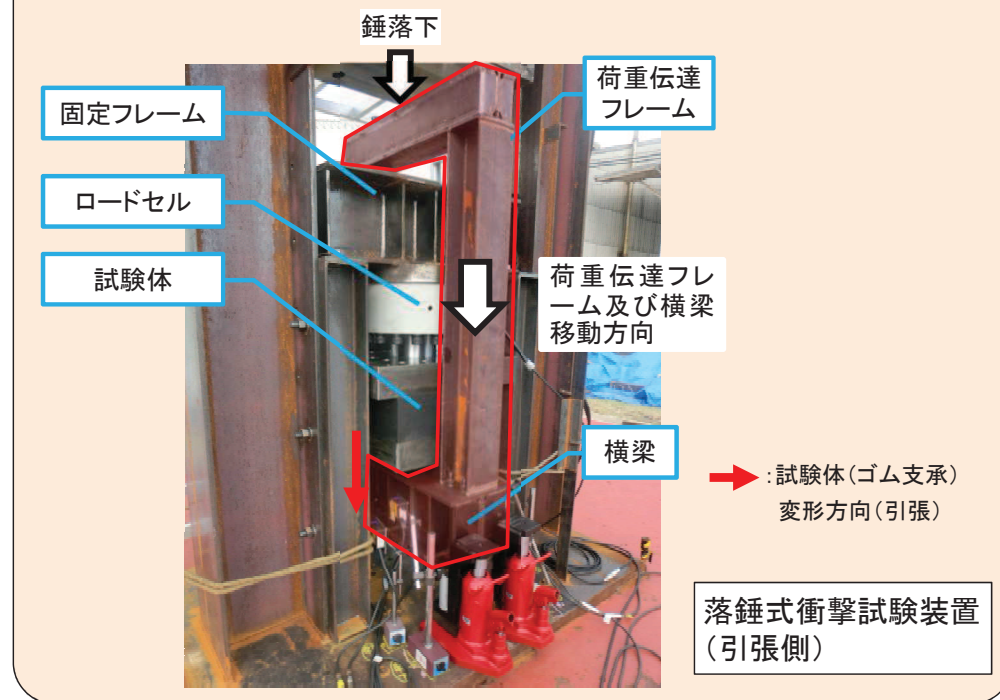
参考図1-2 試験装置外観
