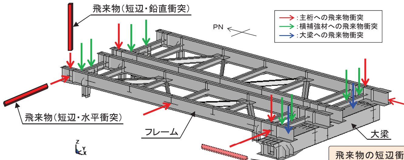
図3-1 解析モデル及び飛来物衝突位置図
