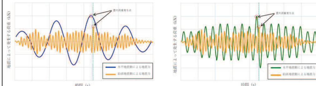
免震型の施設(水平方向の固有周期が4秒の例)
