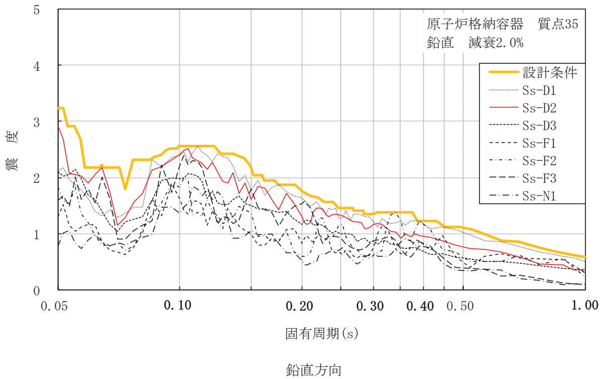
図 2-1 設計条件と基本ケースの床応答曲線の比較 (原子炉格納容器)
