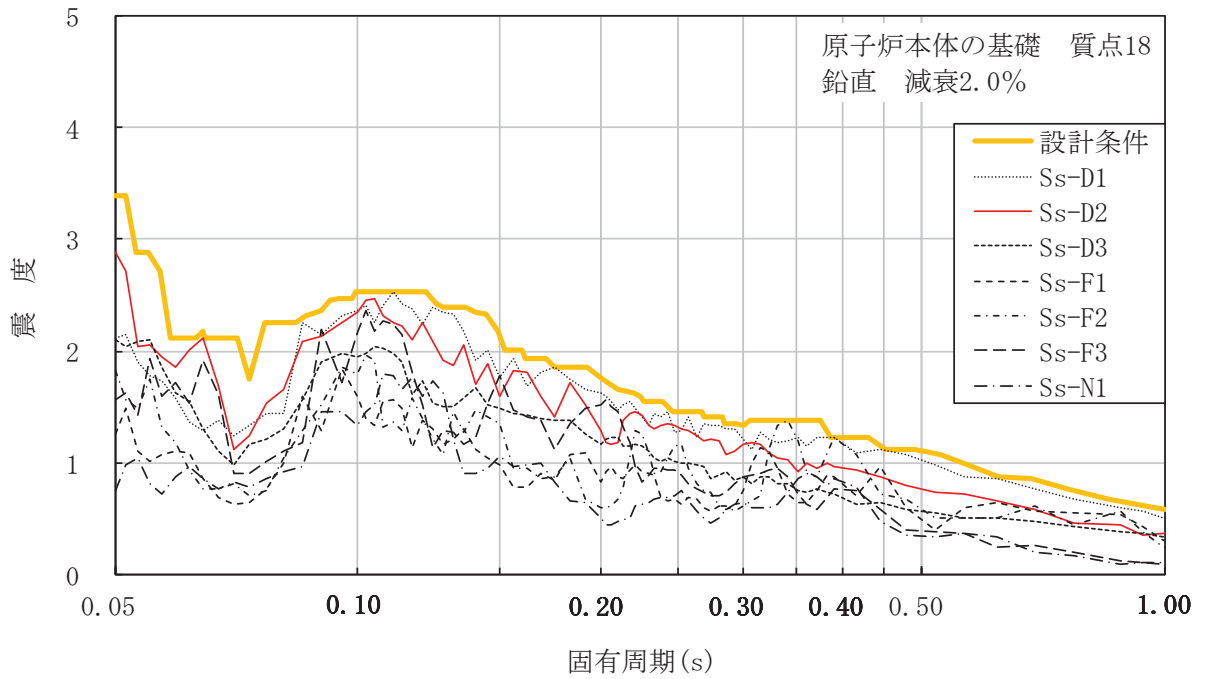
図 2-2 設計条件と基本ケースの床応答曲線の比較 (原子炉本体の基礎)
