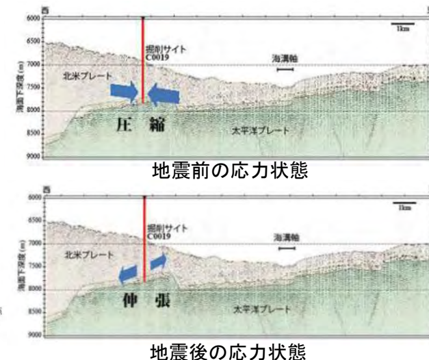
2011年東北地方太平洋沖地震震源域の応力状態変化模式図 JAMSTEC (2013) (18)
