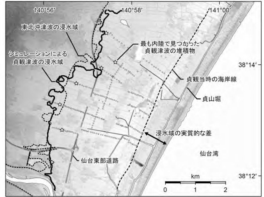
仙台平野における貞観津波 (869年) と2011年東北地方太平洋沖地震に伴う津波の浸水域の比較 菅原ほか (2013) (21)
