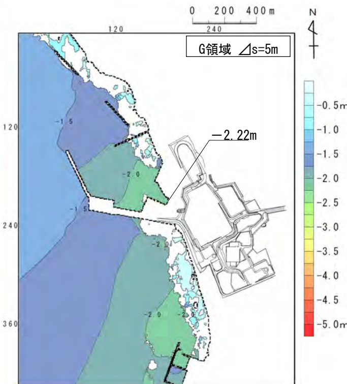
最大水位下降量分布
