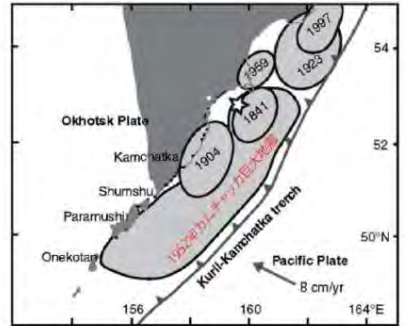
図2 カムチャツカ沖で発生した最近の巨大地震の震源域 (Fedotov et al., 1982)。右は1952年カムチャツカ巨大地震の震源を示す。Maclussey et al.(2010)の図に追記した。
