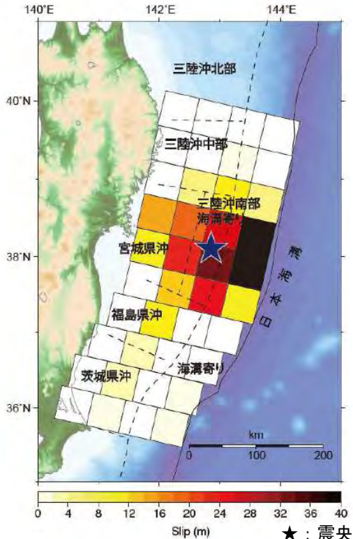
★: 震央 津波波形のインバージョンによる2011年東北地方太平洋沖地震のすべり分布 佐竹 (2011) (19)
