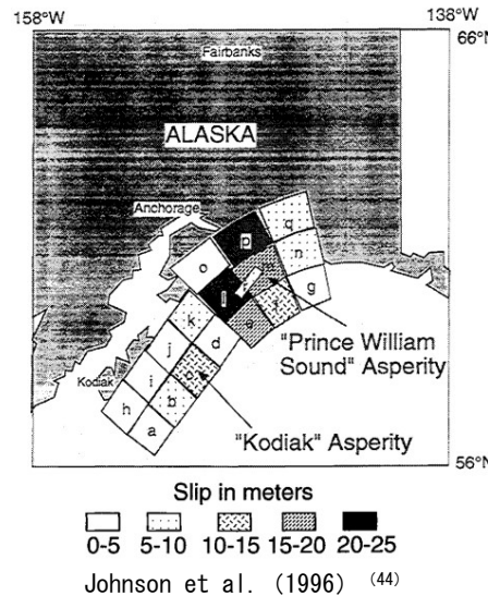
【1964年アラスカ・アリユーション】
