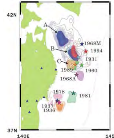
青森県東方沖及び岩手県沖北部におけるアスペリティの活動パターンと地震規模の関係 Yamanaka and Kikuchi (2004) (82) 、永井ほか (2001) (83)
