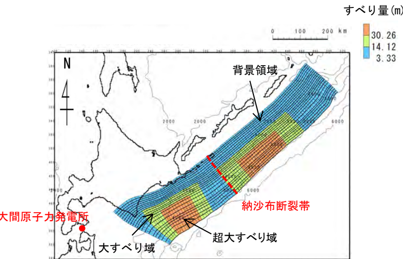
基準波源モデル①-2 (十勝沖・根室沖から色丹島沖及び択捉島沖の広域の津波特性を考慮した特性化モデル)
