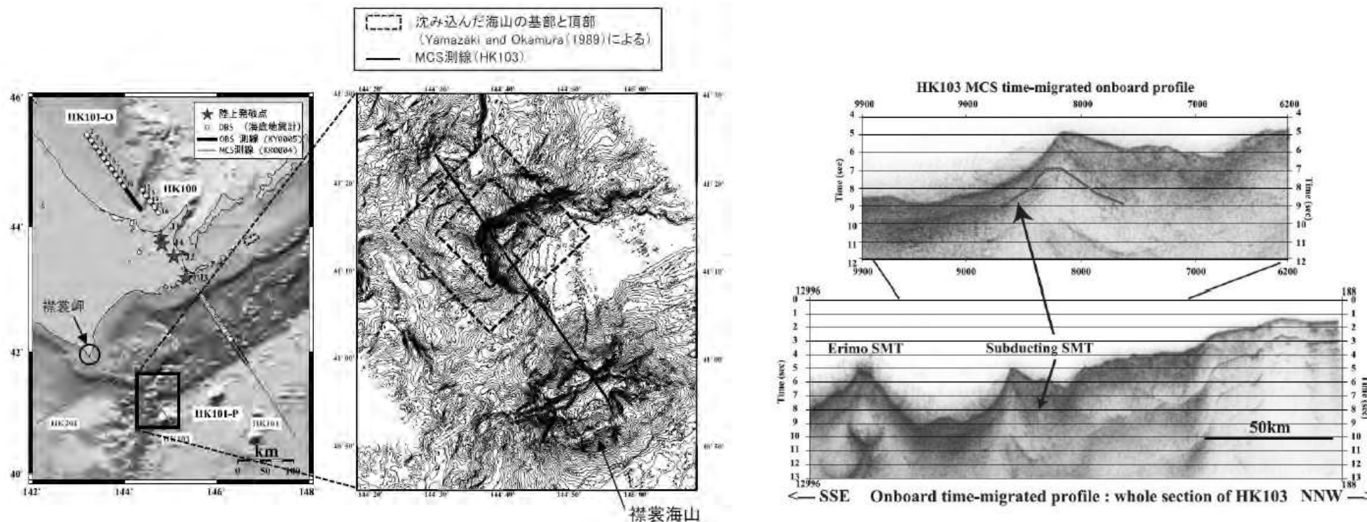
襟裳海山及び沈み込む海山直上のプロファイル (MCS処理記録 (測線: HK103) ) 木戸ほか (2002) (115)
