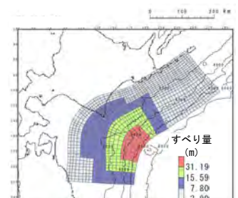
基準波源モデル⑥
