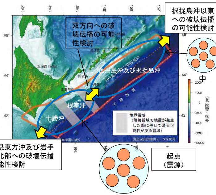
地震調査研究推進本部 (2017a) (79) に一部加筆
