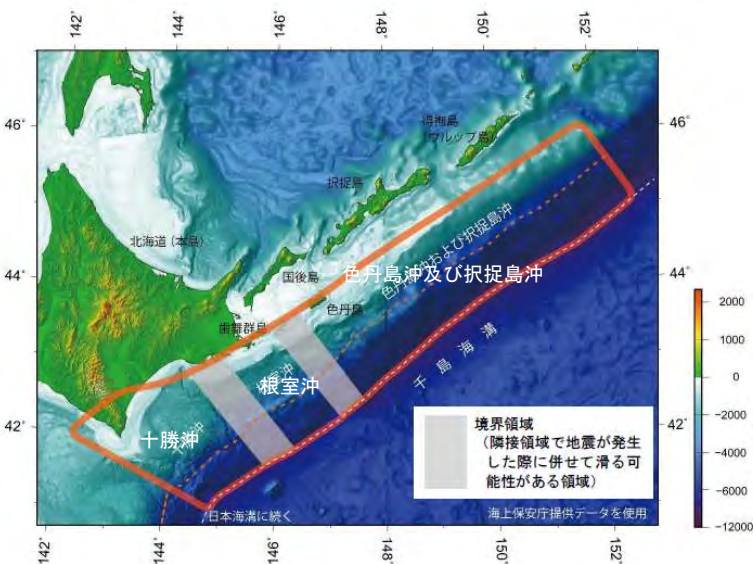
千島海溝沿いの評価対象領域※ 地震調査研究推進本部 (2017a) (79) に一部加筆
