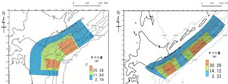
基準波源モデル①-1
