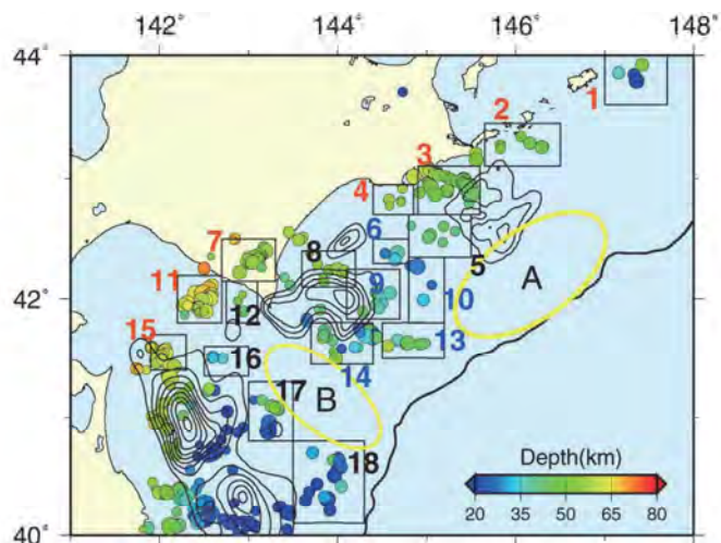
第1図. 北海道南東沖の小繰り返し地震グループの分布 (丸印). 丸の色はグループの地震の平均の深さを示す、コンターは Yamanaka and Kikuchi (2004) (8) による M7 以上の地震のすべり量分布. 矩形は第3図で平均の積算すべりを推定した領域を示す. 黄色楕円は繰り返し地震活動が低い場所.
