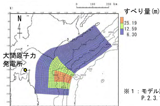
岩手県沖北部から青森県東方沖の破壊特性を考慮した特性化モデル※1
