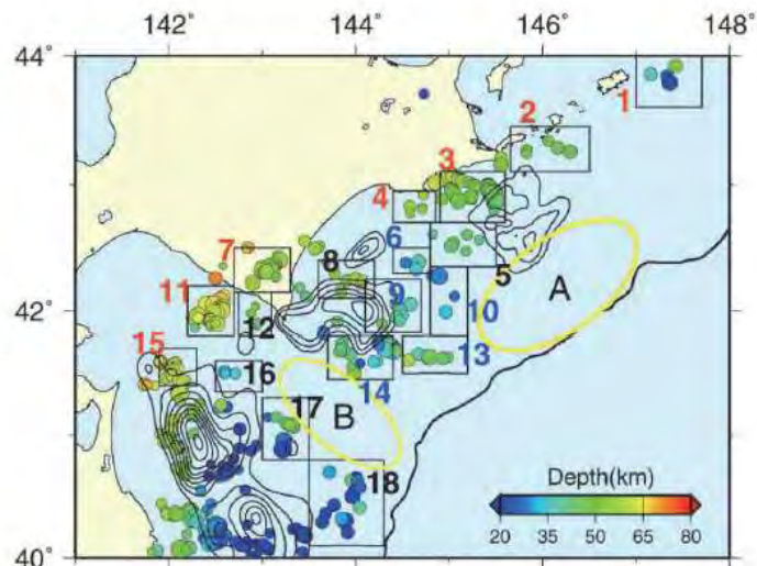
第1図. 北海道南東沖の小繰り返し地震グループの分布 (丸印). 丸の色はグループの地震の平均の深さを示す。コンターはYamanaka and Kikuchi (2004) (82) によるM7以上の地震すべり量分布。矩形は第3図で平均の積算すべりを推定した領域を示す。黄色楕円は繰り返し地震活動が低い場所。
