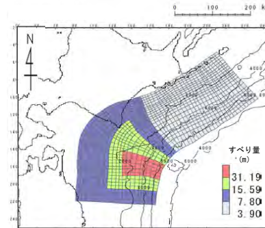
基準波源モデル③
