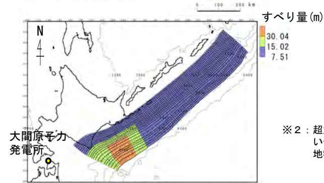
十勝沖・根室沖から色丹島沖及び択捉島沖の破壊特性を考慮した特性化モデル※2
