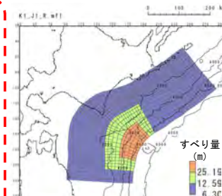
基準波源モデル⑤
