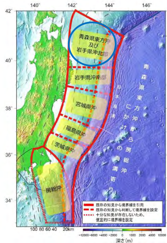
三陸沖から房総沖にかけての評価対象領域の区分け 地震調査研究推進本部 (2019) (78)に一部加筆
