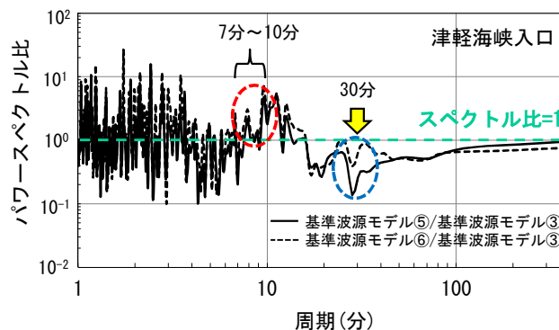
基準波源モデル③と基準波源モデル⑤⑥との比較
