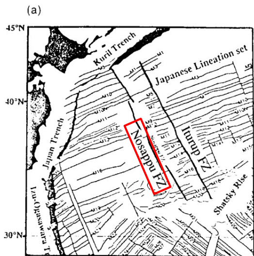
地磁気異常 Kasahara et al. (1997) (97) に一部加筆
