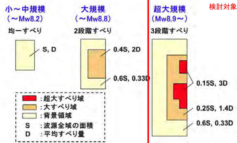
微視的波源特性に係る波源領域内の空間的すべり分布の設定方法 杉野ほか（2014） (80) に一部加筆
