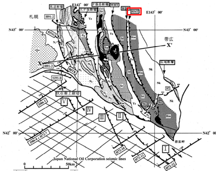
図1 日高衝突帯ならびに前縁褶曲・衝上断層帯の地質概略と主な反射法地震探査測線図。X-X'は図2の断面位置を示す。伊藤ら(1999)を改変。 【地質】主として、地質調査所(1982, 1996)による。Nk: 中の川層群, Hm: 日高変成岩類(主帯), Po: ボロシリ・オフィオライト(西帯), Id: イドンナップ帯, Yz: 蝦夷層群, Sr: 空知層群, Km: 神威古潭変成岩類, Sn: 沙流川層群(ニセウ層), Pg: 古第三系, N1~N3: 地質調査所(1982)と同じ。Qv: 第四紀火山岩類。 【測線】H4・96・97: 日高深部構造反射法探査, 85NG・86TK: 浅野ら(1990), Y97: 伊藤ら(1998), その他の測線は石油公団(1973, 1987, 1993, 1996)。
