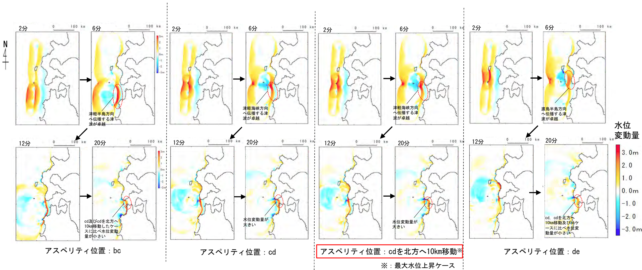
スナップショット \Delta s=2500m 領域 (地震発生～20分後)
