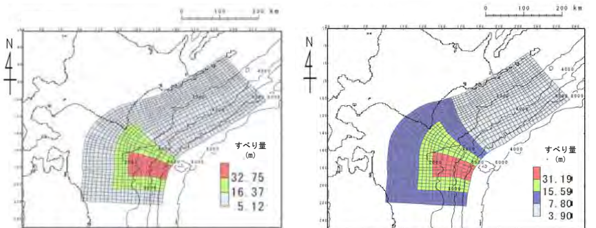
基準波源モデル②
