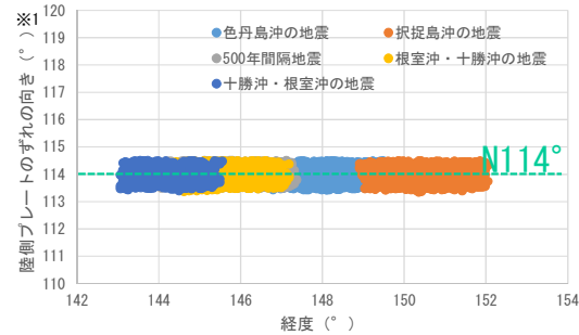
千島海溝沿い
