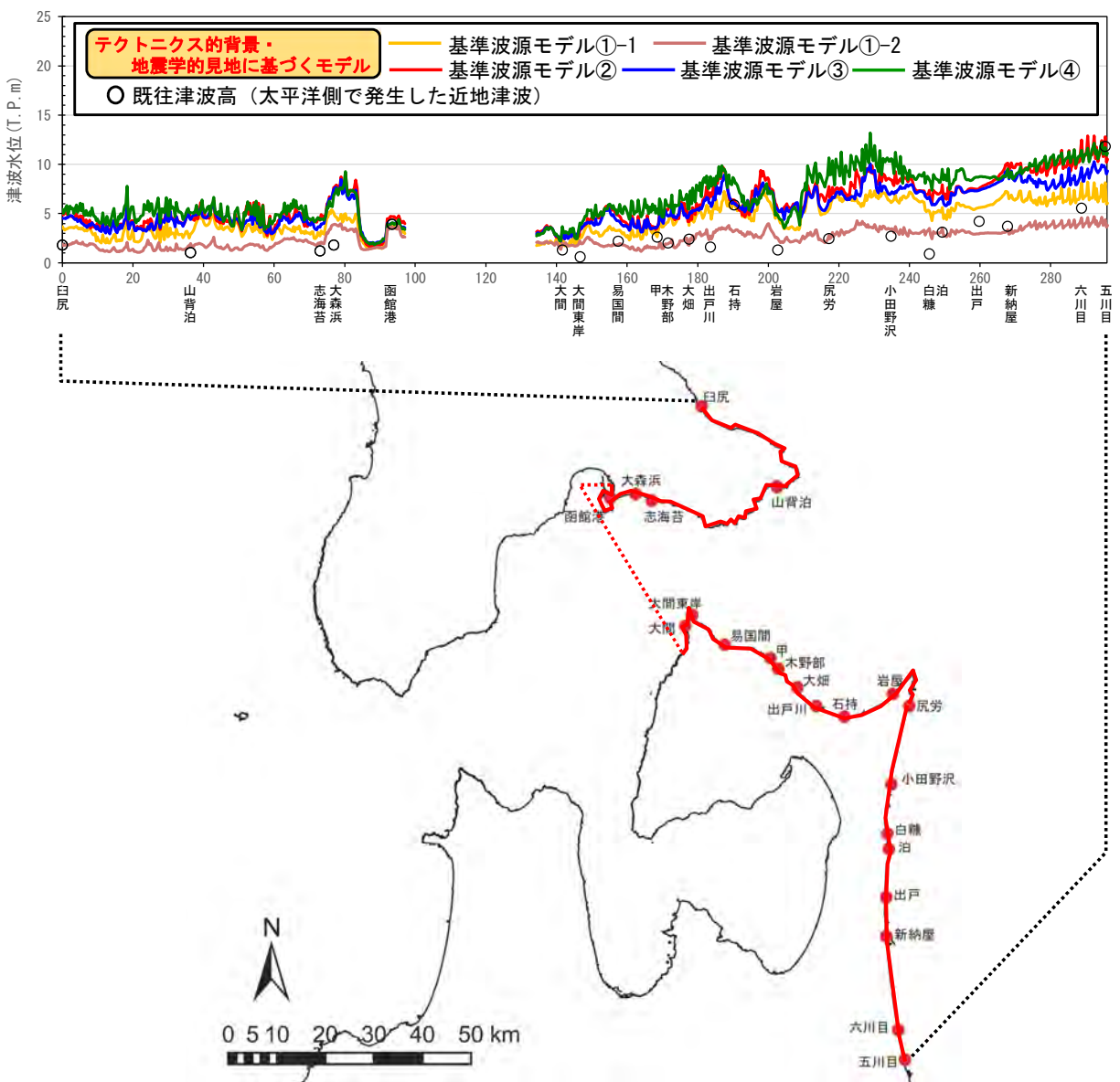
基準波源モデル①~④の計算津波高と太平洋側既往津波高との比較
