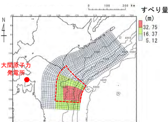
(基準波源モデル②)
