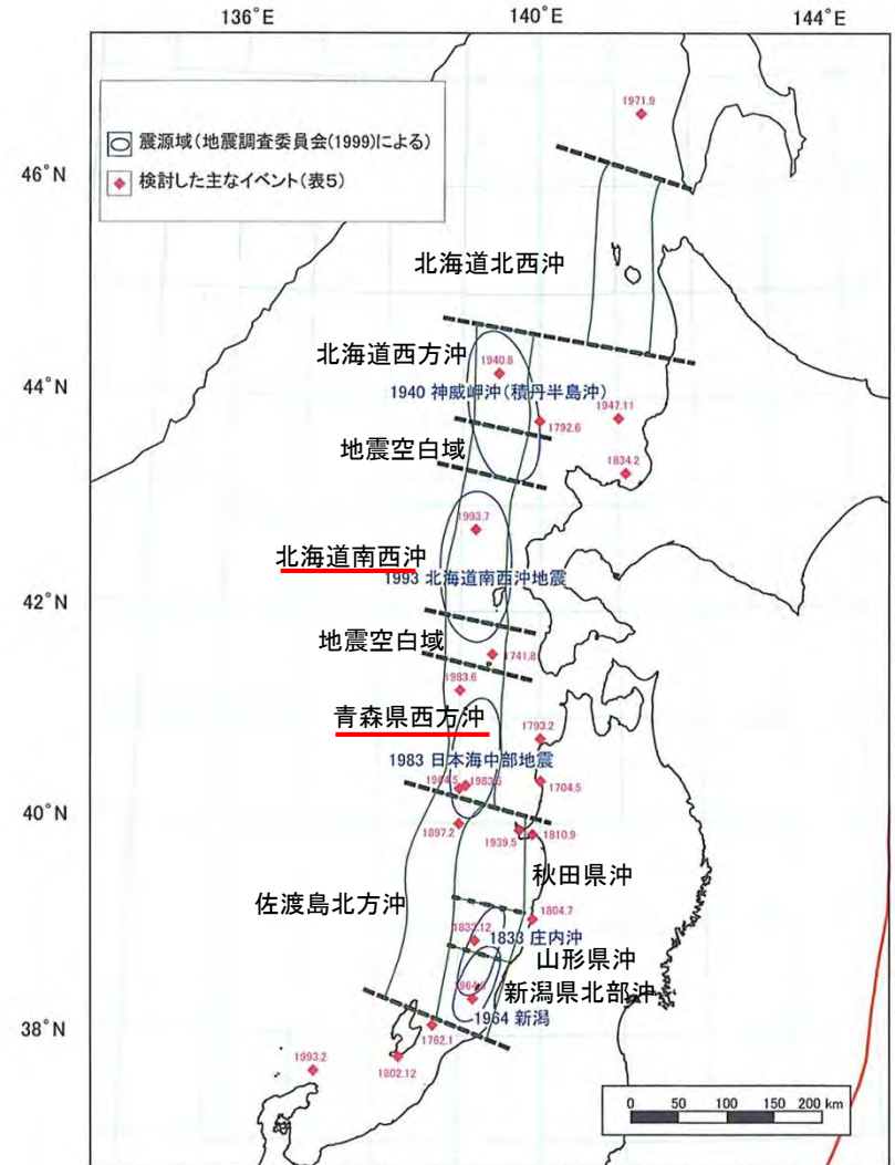
日本海東縁部における主な地震の震源域と地震調査研究推進本部（2003） (50) で検討対象としたイベント
