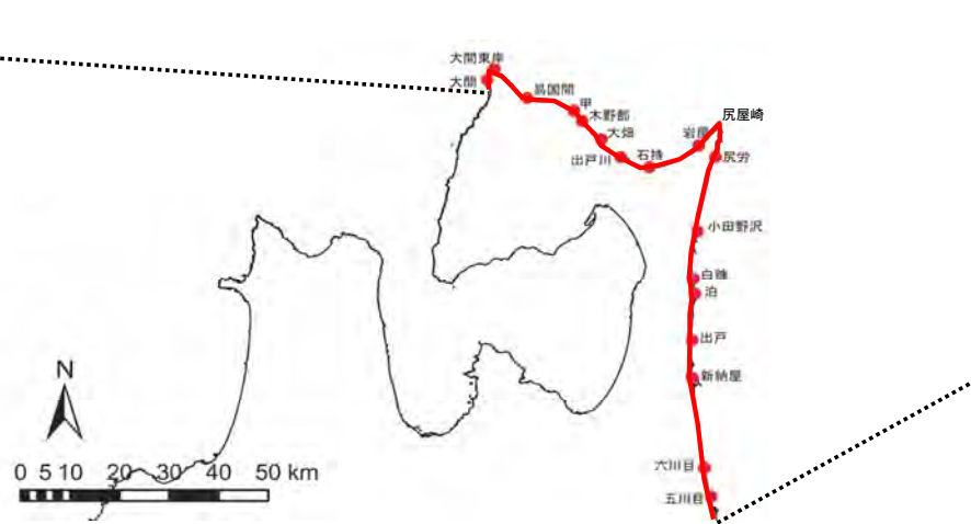
青森県北部太平洋沿岸の海岸線位置における基準波源モデル①～⑥と内閣府(2020)による日本海溝(三陸・日高沖)モデルの想定津波群との比較
