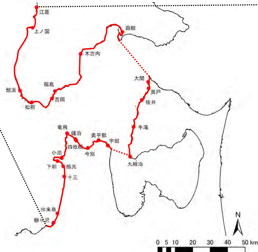
日本海東縁部に想定される地震に伴う津波の計算津波高と既往津波高等との比較
