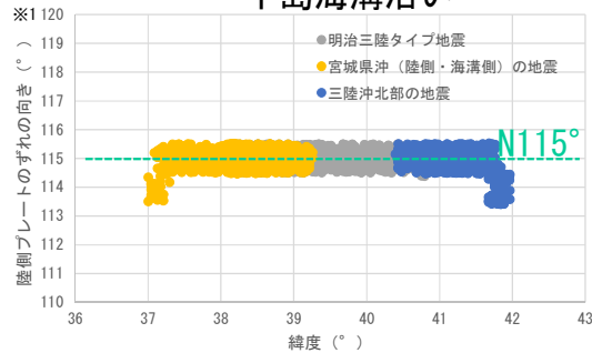
日本海溝沿い
