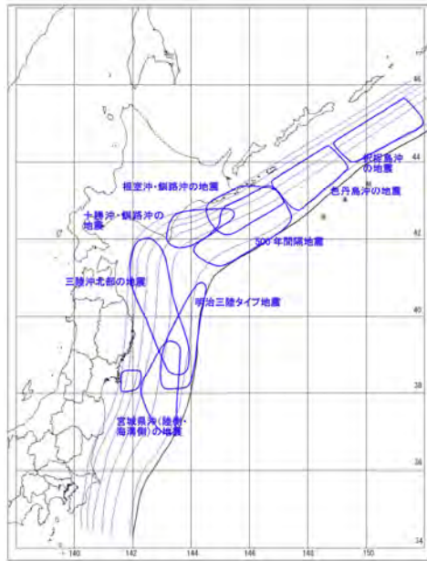
津波を発生させる断層領域 (津波の断層域) の模式図 中央防災会議 (2006) (10)
