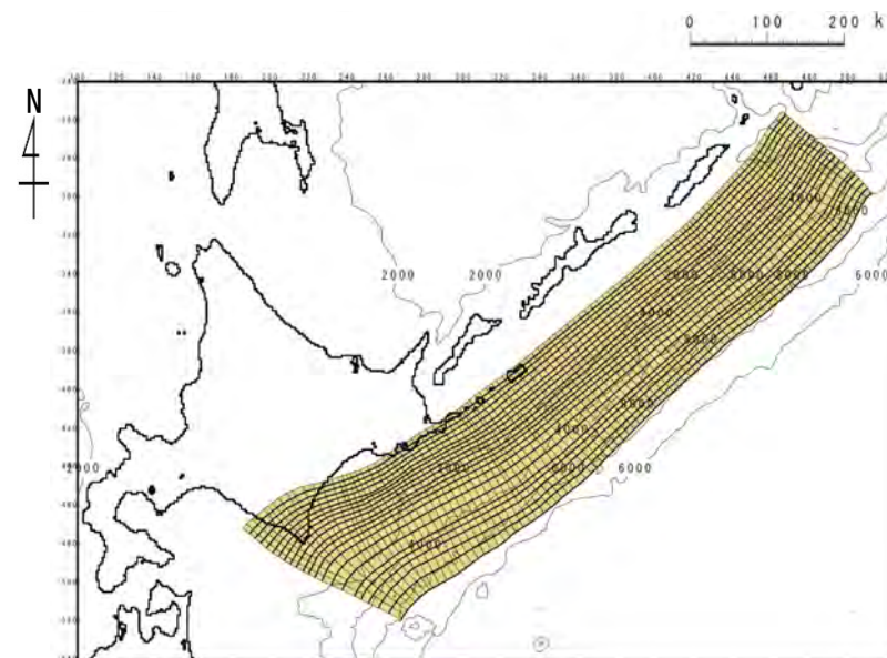
十勝沖・根室沖から色丹島沖及び択捉島沖
