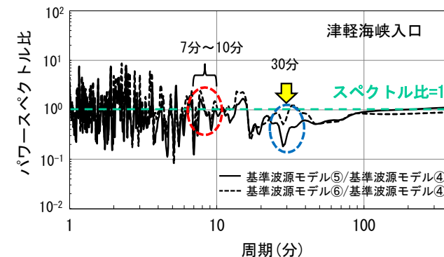
基準波源モデル④と基準波源モデル⑤⑥との比較
