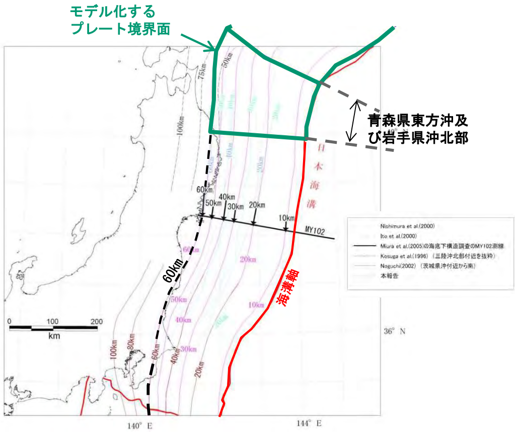
微小地震の震源分布に基づくプレート境界面の推定等深線 (三陸沖～房総沖) 地震調査研究推進本部 (2012) (8) に一部加筆
