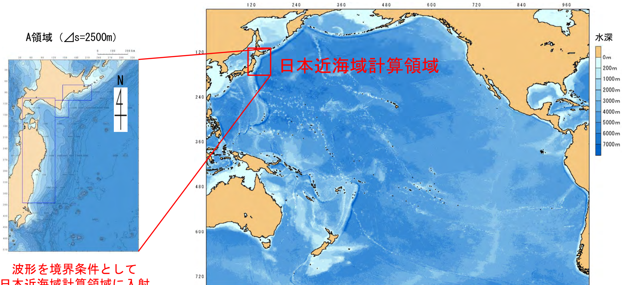
太平洋伝播計算領域 ( \Delta s=10分 )
