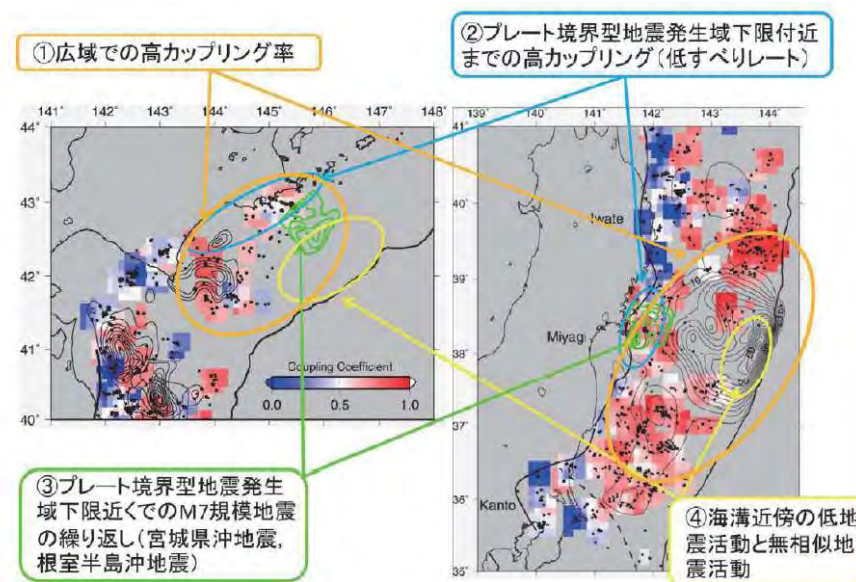
第2図. 北海道南東沖 (左) および東北地方東方沖 (右) の繰り返し地震分布 (黒丸) およびそれにより推定したプレート間カップリング率 (カラー) の比較. カップリング率は 0.3^\circ \times 0.3^\circ のグリッドごとに、3つ以上の小繰り返し地震グループが存在する場所について推定した. 緑および黒のコンターは M7 以上の地震すべり量分布. 関東地方の沖の破線は、フィリピン海プレートの北東限.
