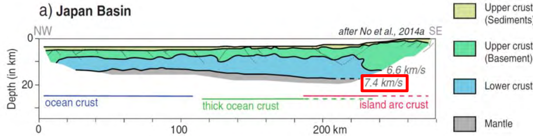
Van Horne et al. (2017) (72) に一部加筆
