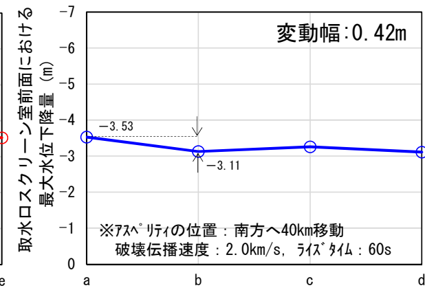
破壊開始点の位置 下降側 (基準波源モデル③)
