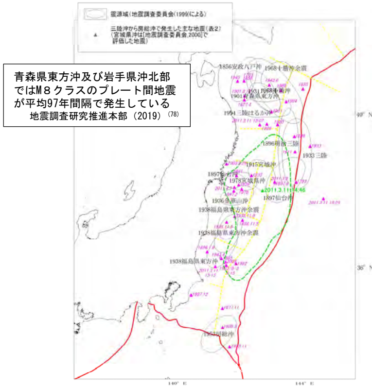
三陸沖から房総沖にかけての主な地震と主な震源域 地震調査研究推進本部 (2012) (8)
