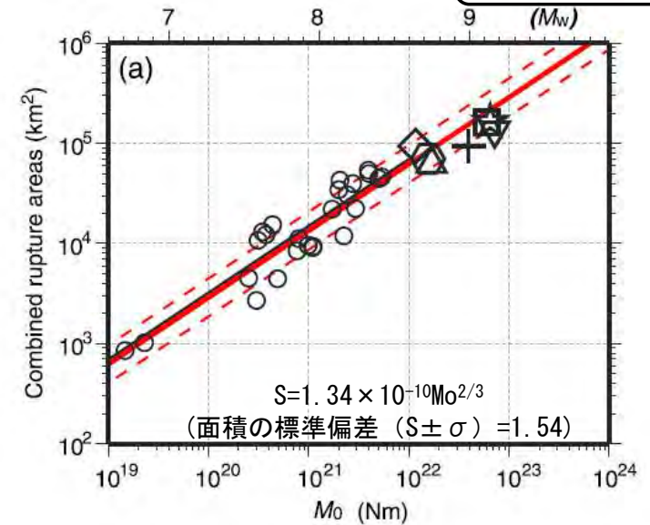
破壊領域 (S) と Mo の関係 Murotani et al. (2013) (119) に一部加筆
