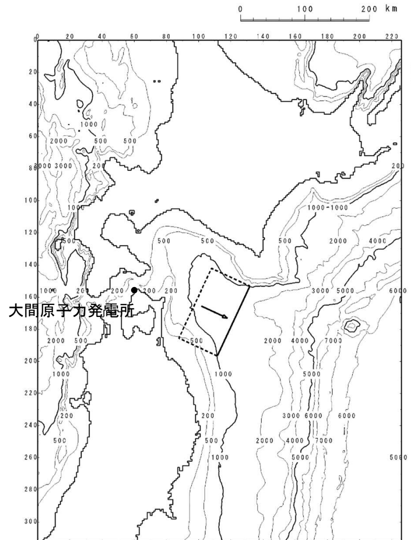
修正相田モデル
