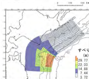
基準波源モデル④
