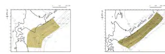
岩手県沖北部から十勝沖・根室沖
