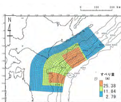
基準波源モデル①-1
