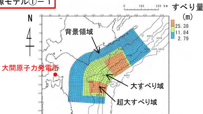
基準波源モデル①-1
