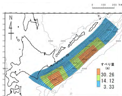
基準波源モデル①-2
