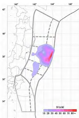
東北地方太平洋沖地震の地震時のすべり量の分布 地震調査研究推進本部 (2019) (78)
