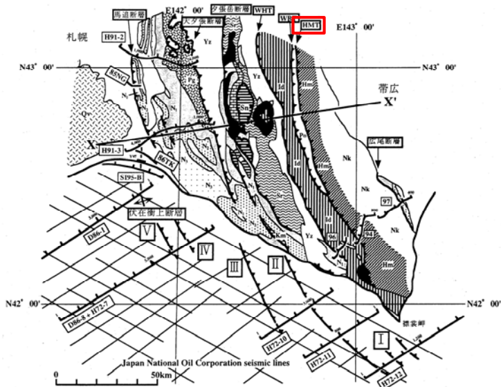
図1 日高衝突帯ならびに前縁褶曲・衝上断層帯の地質概略と主な反射法地震探査測線図。X-X'は図2の断面位置を示す。伊藤ら(1999)を改変。 【地質】主として、地質調査所(1982, 1996)による。Nk: 中の川層群, Hm: 日高変成岩類(主帯), Po: ポロシリ・オフィオライト(西帯), Id: イドナップ帯, Yz: 蝦夷層群, Sr: 空知層群, Km: 神威古潭変成岩類, Sn: 沙流川層ニセウ層, Pg: 古第三系, N1~N3: 地質調査所(1982)と同じ。Qv: 第四紀火山岩類。HMT: 日高主衝上断層, WBT: 西縁衝上断層, WHT: 日高西部断層群 【測線】84°96'37: 日高深部構造反射法探査, 85NG・86TK: 浅野ら(1990), Y97: 伊藤ら(1998), その他の測線は石油会社(1973, 1987, 1993, 1996)。
