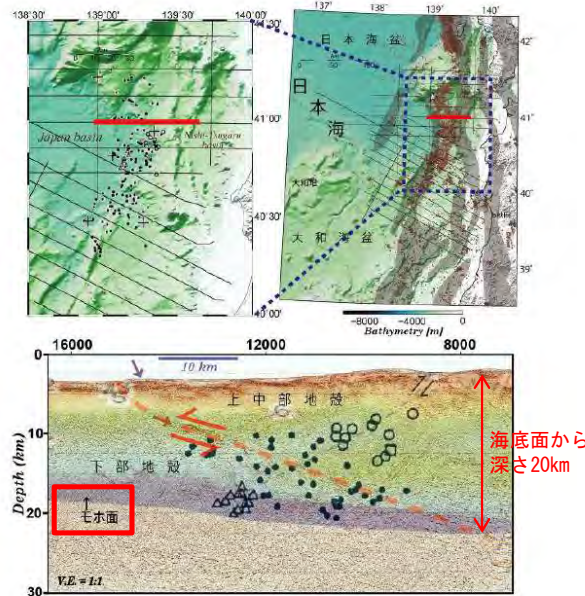
図5 (上) 測線図。赤線の範囲を下图に表示しました。右上图の震源分布は気象庁一元化震源と地震年報 23) による震源(深さ:0~50 km, 期間:2000~2011年、マグニチュード: M_j > 1 )。左上图の震源分布は海底地震観測と陸上観測網の統合処理で得られた余震分布 21) 。(下) マルチチャンネル反射法地震探査によって得られた深度断面と海底地震計による地震波速度構造と海陸統合処理によって得られた余震分布 21) の結果との比較。
