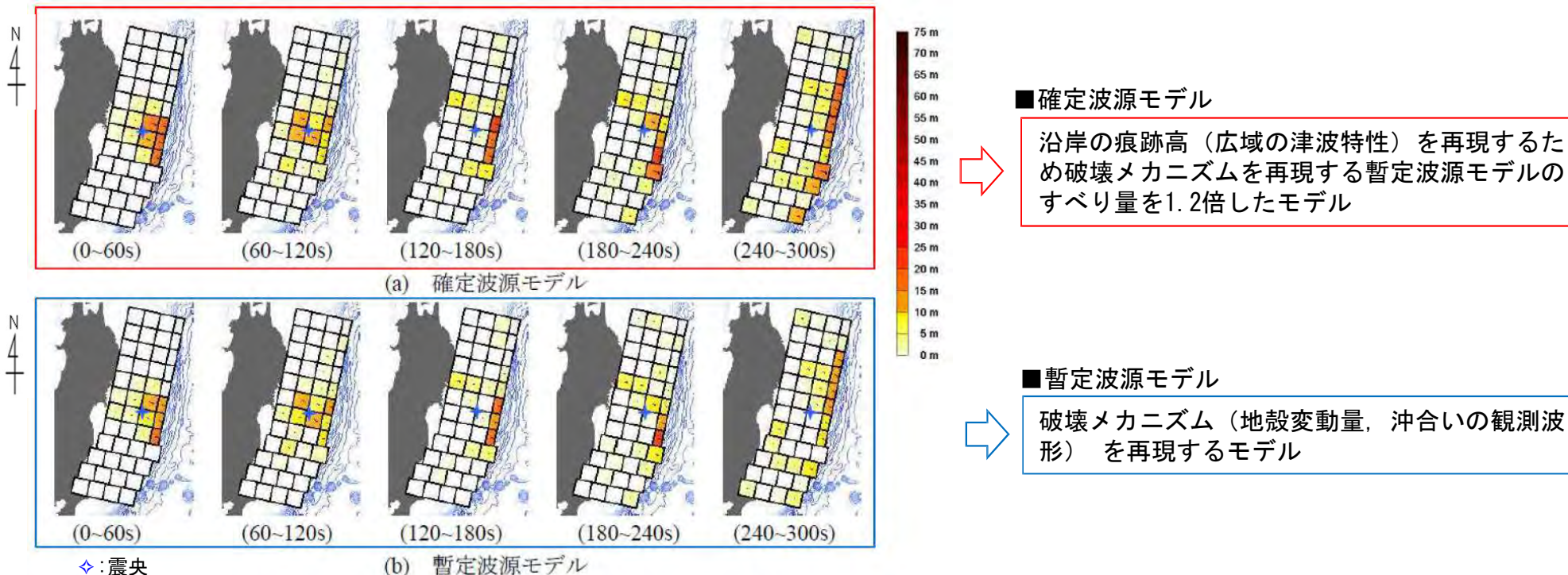
3.11地震を再現する津波波源モデルのすべり分布の経時変化 杉野ほか (2013) (101) に一部加筆
