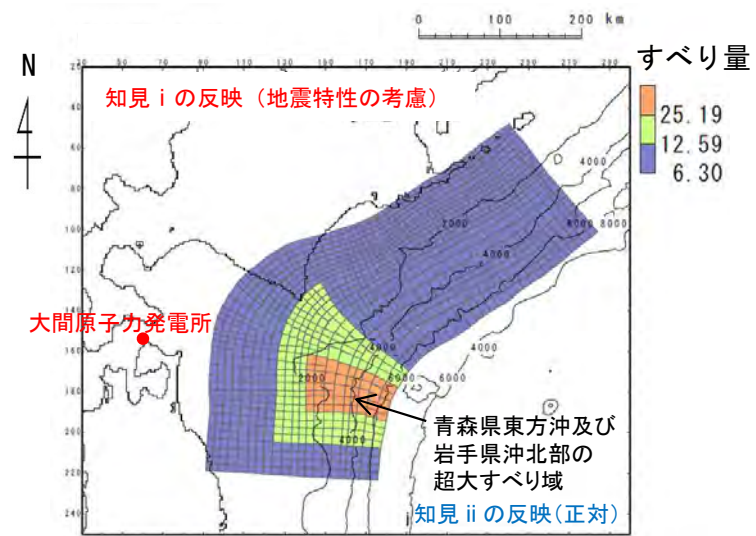
3.11地震における宮城県沖の破壊 特性を考慮した特性化モデルを参 考に設定した特性化モデル (P. 2.3.1-93)
