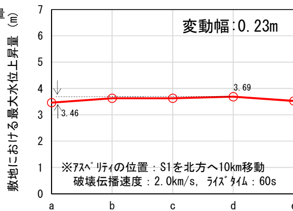
破壊開始点の位置 上昇側 (基準波源モデル⑥)
