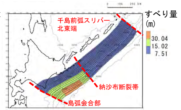
十勝沖・根室沖から色丹島沖及び択捉島沖の連動型地震
