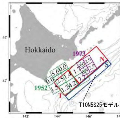
17世紀に発生した超巨大地震に伴う津波の再現モデル (Ioki and Tanioka (2016) (105) によるT10N5S25モデル) 地震調査研究推進本部 (2017a) (79) に一部加筆
