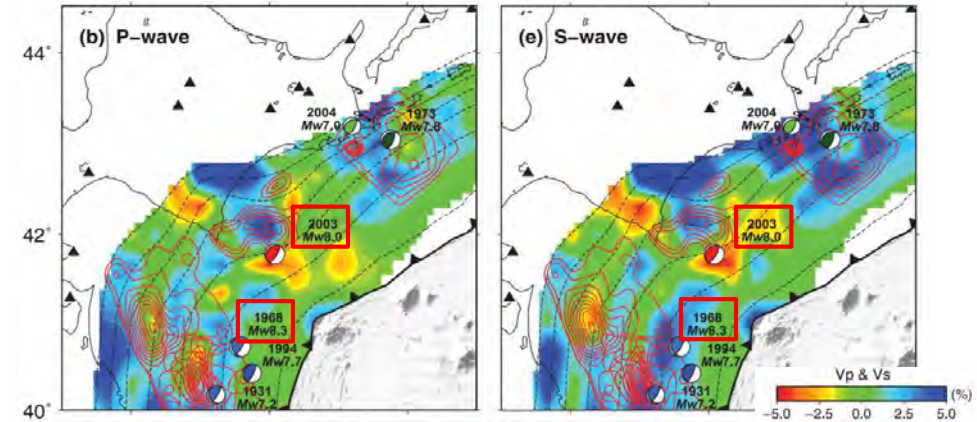
日本海溝・千島海溝島弧改造部付近の地震波トモグラフィと既往地震発生域の関係 Liu et al. (2013) (95) に一部加筆
