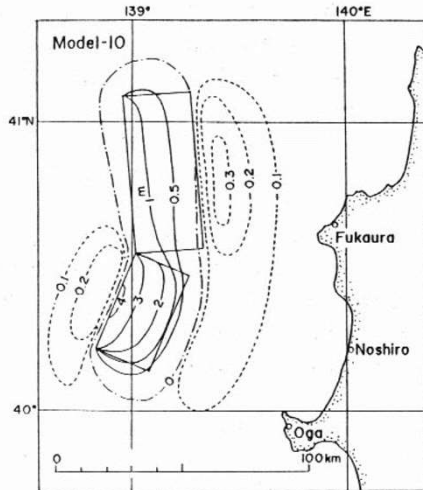
1983年日本海中部地震津波 断層モデル 相田 (1984) (75) に一部加筆
