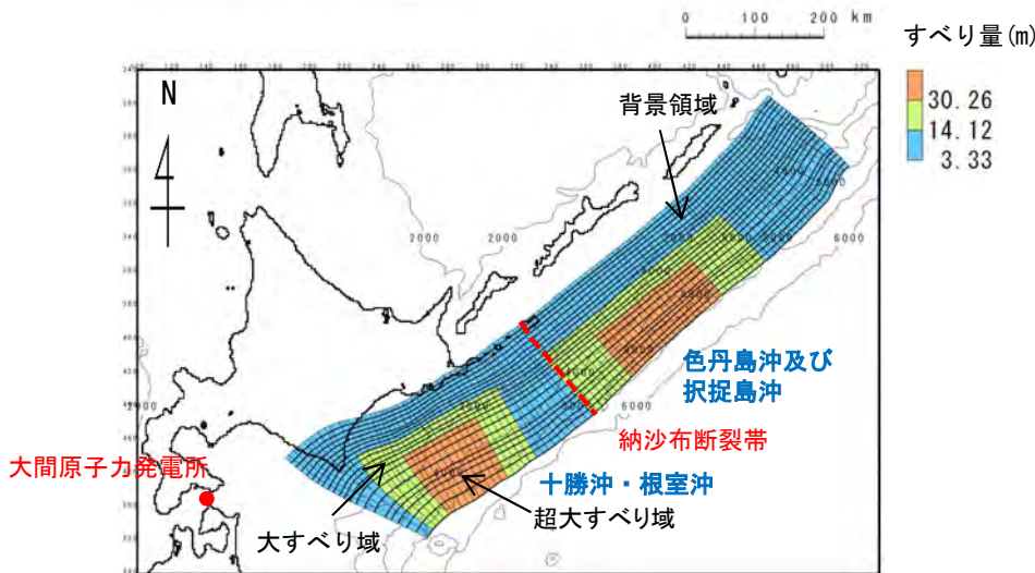
基準波源モデル①-2
