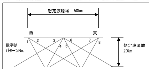
東西位置、傾斜角パターン 土木学会 (2016) (39) に一部加筆
