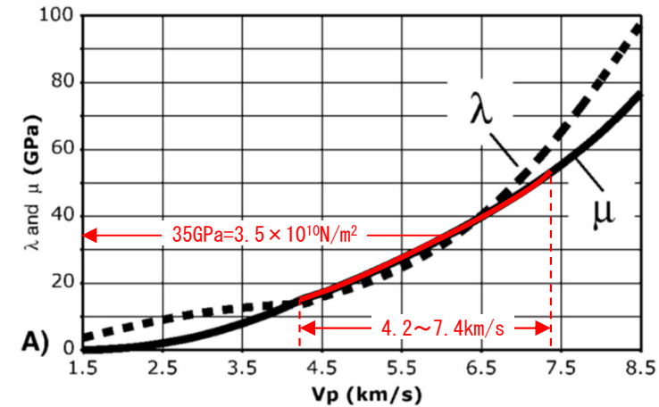
Brocher (2005) (74) に一部加筆
