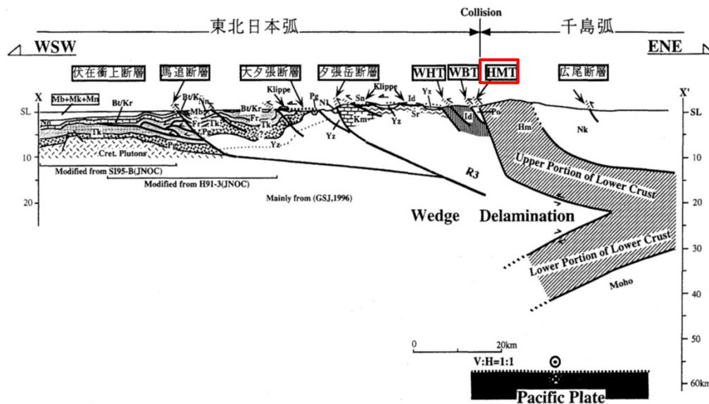
図2 日高衝突帯ならびに前縁褶曲・衝上断層帯の地下構造断面図。 断面線の位置は図1のX-X'。断面図下に主要な出典を示した。略称は図1に同じ。Ito et al. (1998) および伊藤ら(1999)を改変。 伊藤(2000) (93) に一部加筆
