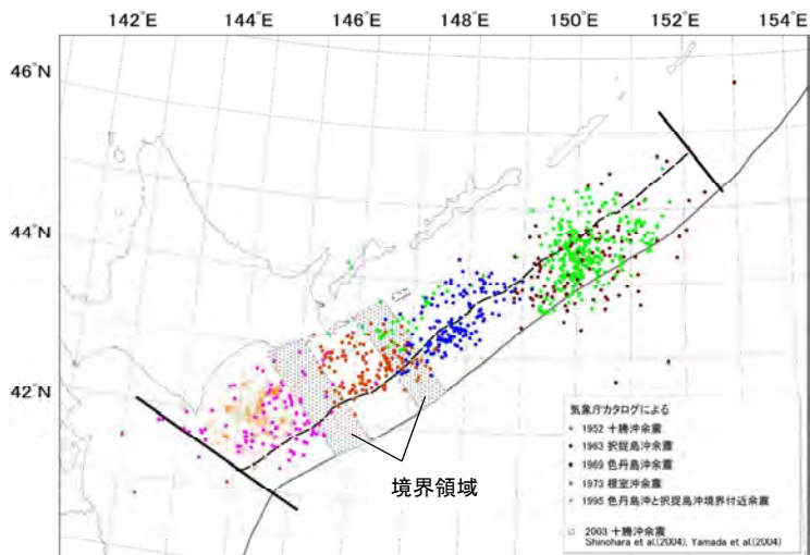
近年のプレート間巨大地震の余震分布 地震調査研究推進本部 (2017a) (79) に一部加筆
