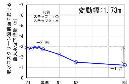
アスペリティの位置 下降側 (基準波源モデル⑥)
