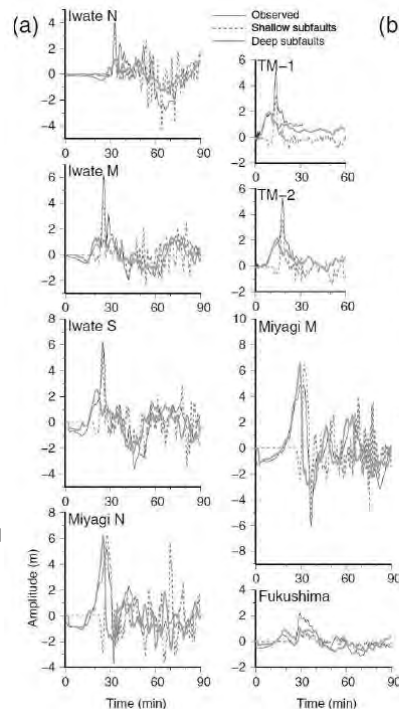
観測波形と計算波形の比較 3.11地震に伴う津波特性の分析 Satake et al. (2013) (102) に一部加筆
