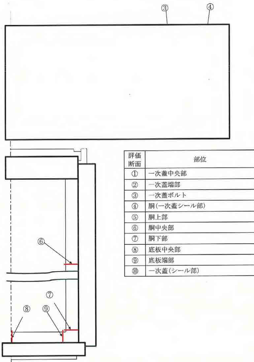
図 2.6.1-1 密封容器の応力評価位置
