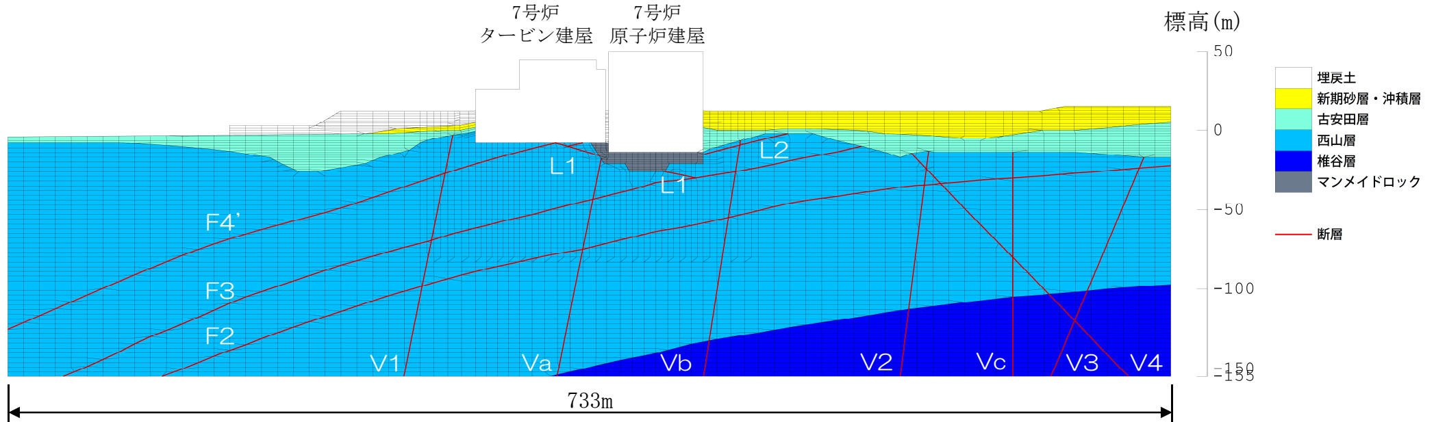
7号炉原子炉建屋 汀線直交断面 C-C'
