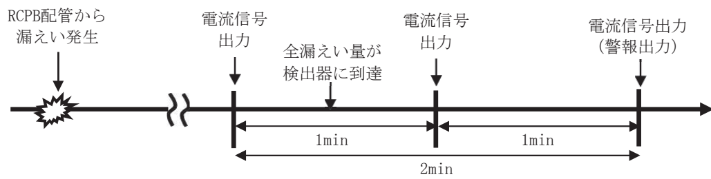
図1-2 ドライウェル送風機冷却コイルドレン流量測定装置の検出時間の考え方
