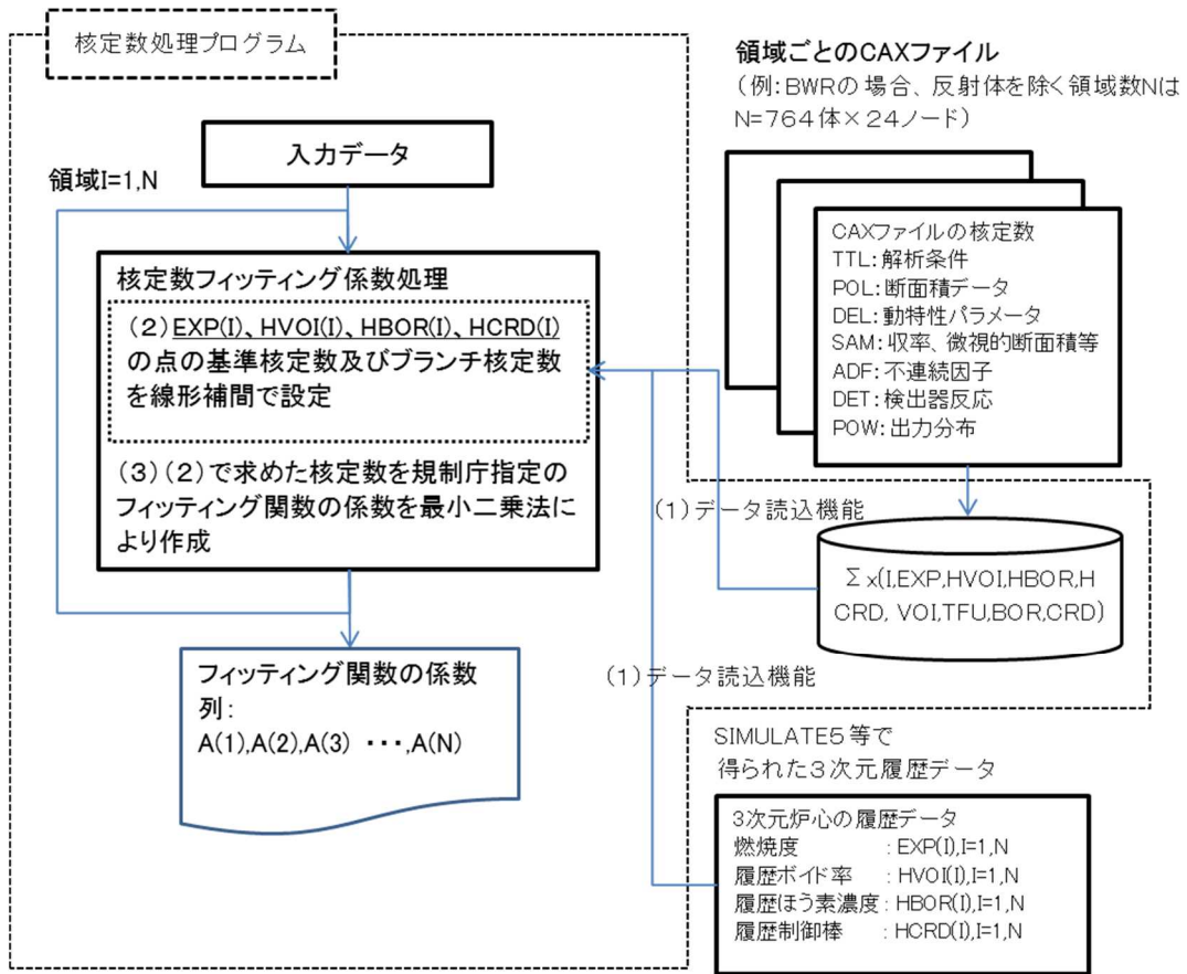
図1 多次元フィッティング方式の核定数処理の流れ
