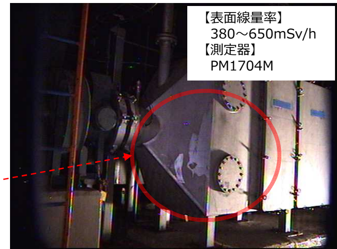
矢視(1)
