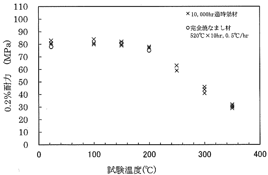
別紙 1-46 図 完全焼なまし処理材 (520°C×10hr 保持、0.5°C/hr 冷却) と長時間過時効熱処理材の比較 (0.2%耐力)
