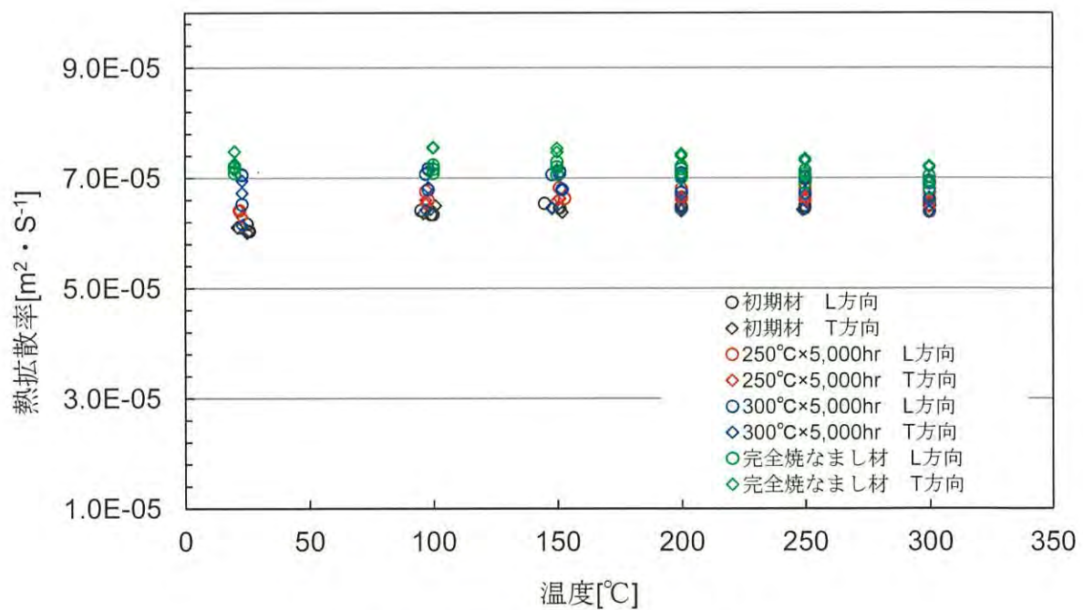
別紙 4-3 図 各温度における熱膨散率
