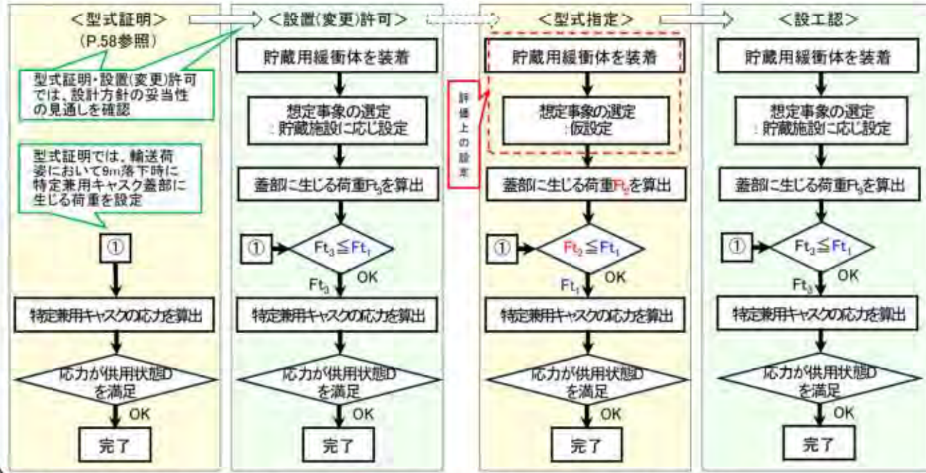
安全設計全般に係る設計方針の妥当性確認(安全評価)フロー (型式指定の前に設置(変更)許可が実施される場合)
