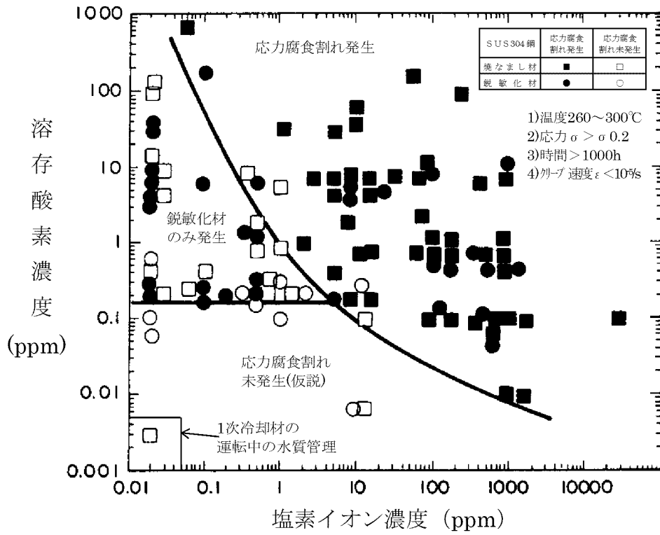
第 8-5 図 SUS304 鋼の応力腐食割れ発生におよぼす塩素イオン濃度及び溶解酸素濃度の限界量 (42)
