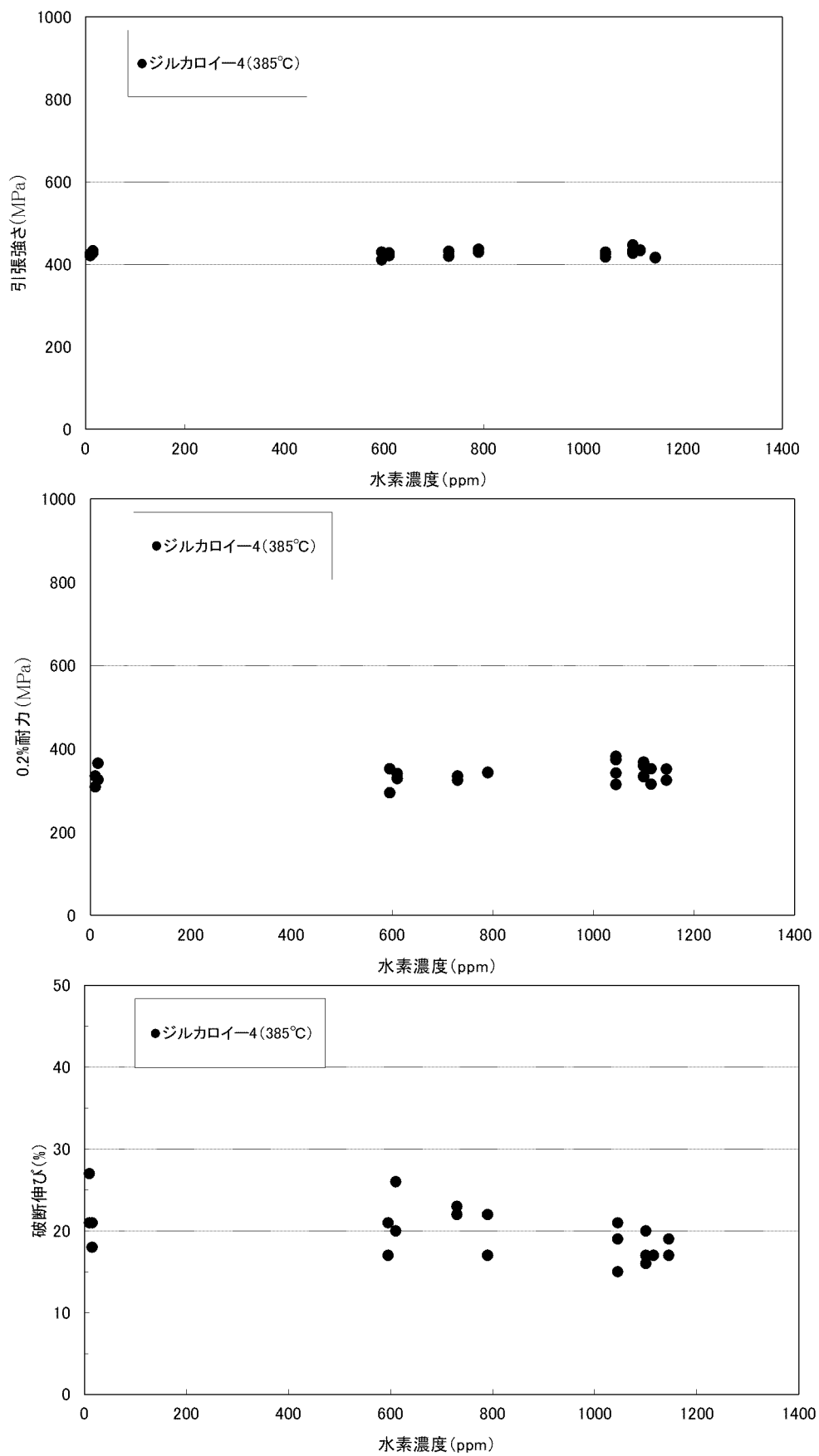
第5-2図 ジルカローイ-4 未照射被覆管の機械特性と水素濃度の関係
