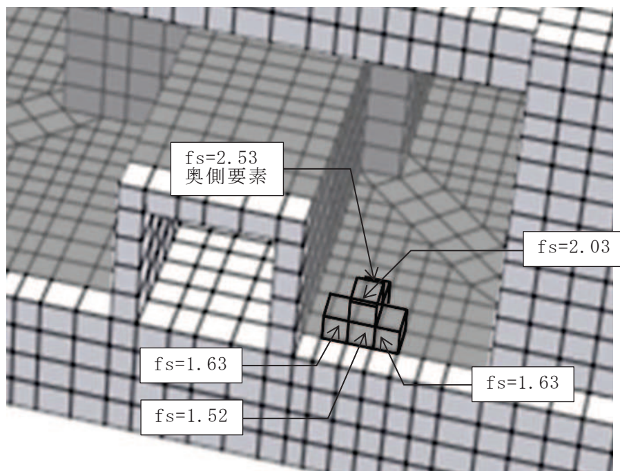
(b) 拡大図
