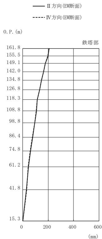
図 3-19(1) 最大応答変位 (S s ばらつき, ケース⑥)
