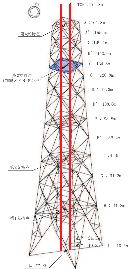
解析モデル
