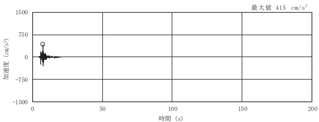
図 2-6(15) 入力地震動の加速度時刻歴波形
