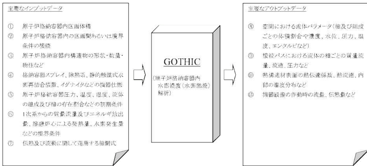
第1.15-90図 水素濃度評価の概要
