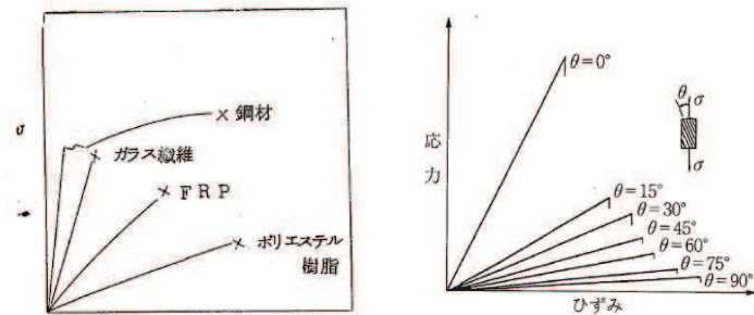
応力-ひずみ曲線 左:「基礎からわかるFRP(強化プラスチック協会編, 2016)」 右:「FRP成形入門講座(日本プラスチック加工技術協会)」
