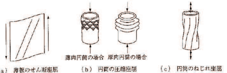
座屈変形の例
