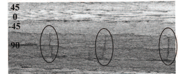
積層板に発生するトランスバースクラックの例
